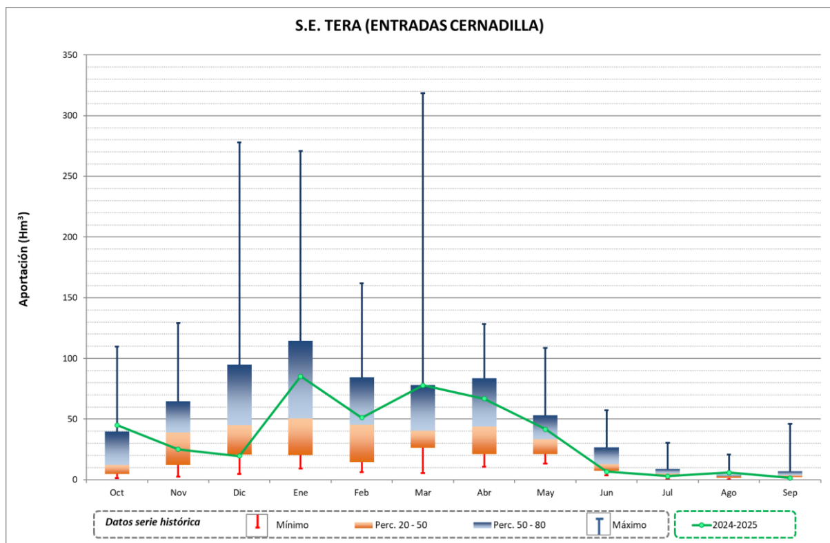
Figura 2. Gráfica del año hidrológico 2024-2025 en el sistema Tera
