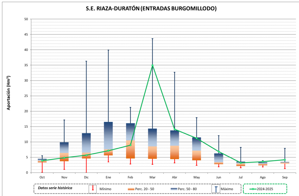
Figura 9. Gráficas del año hidrológico 2024-2025 en el sistema Rianza-Duración
