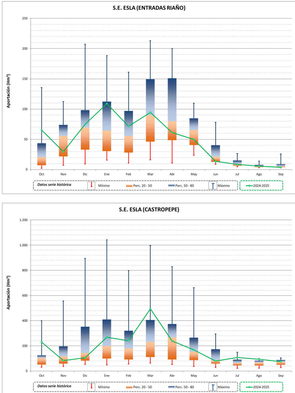
Figura 4. Gráficas del año hidrológico 2024-2025 en el sistema Esla
