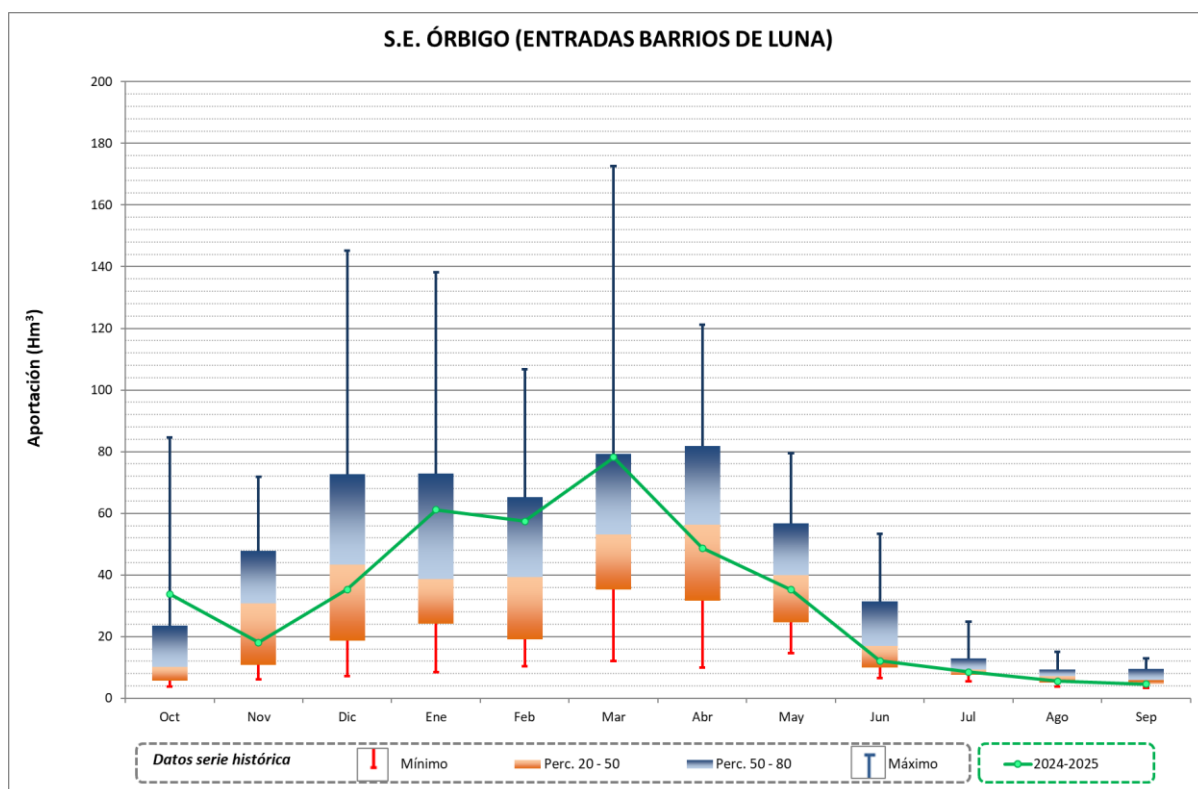
Figura 3. Gráficas del año hidrológico 2024-2025 en el sistema Órbigo
