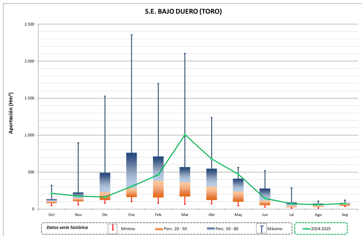
Figura 11. Gráfica del año hidrológico 2024-2025 en el sistema Bajo Duero
