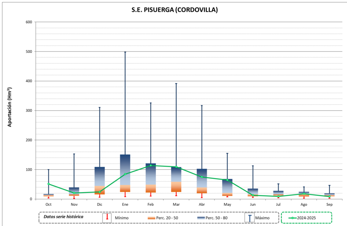
Figura 6. Gráficas del año hidrológico 2024-2025 en el sistema Pisuerga
