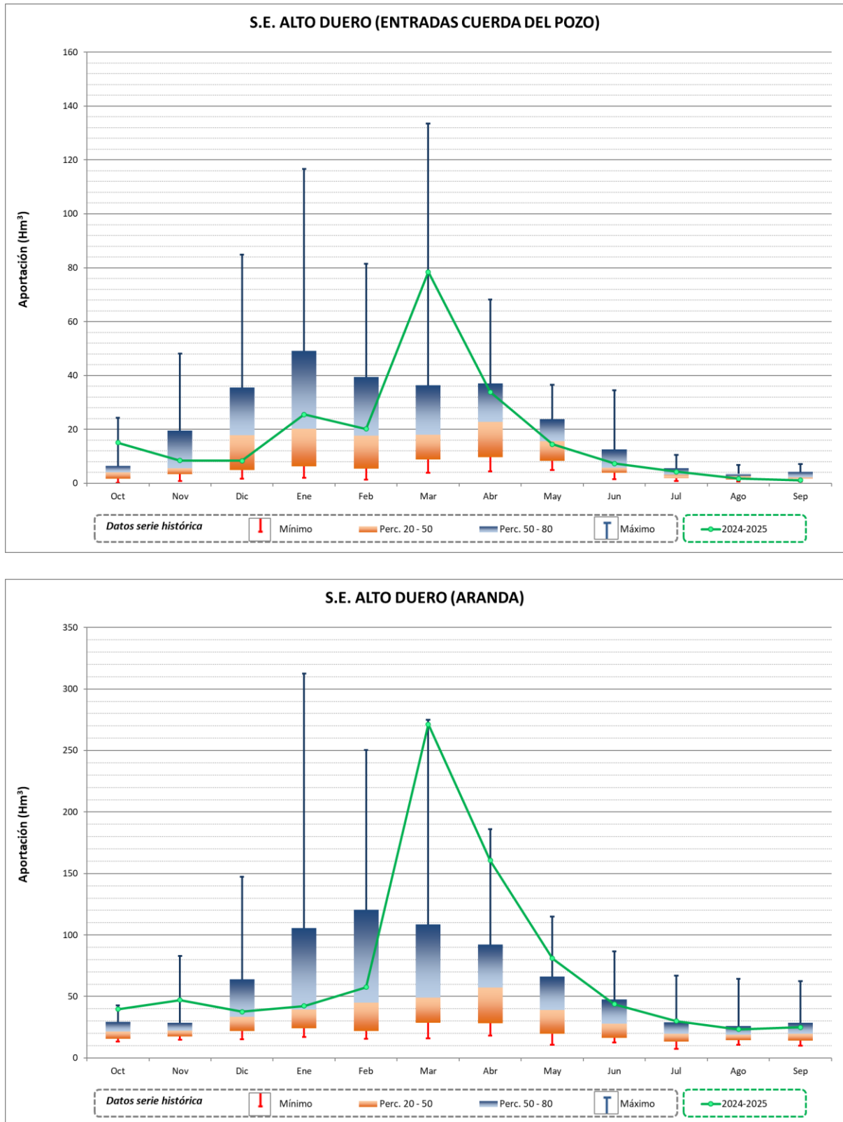
Figura 8. Gráficas del año hidrológico 2024-2025 en el sistema Alto Duero
