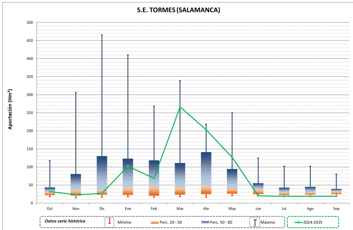
Figura 12. Gráficas del año hidrológico 2024-2025 en el sistema Tormes
