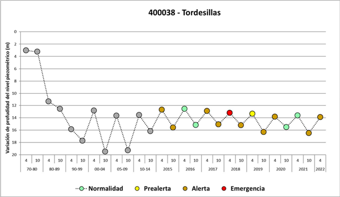
Figura 57. Evolución del Índice de estado de escasez en la MASub de Tordesillas
