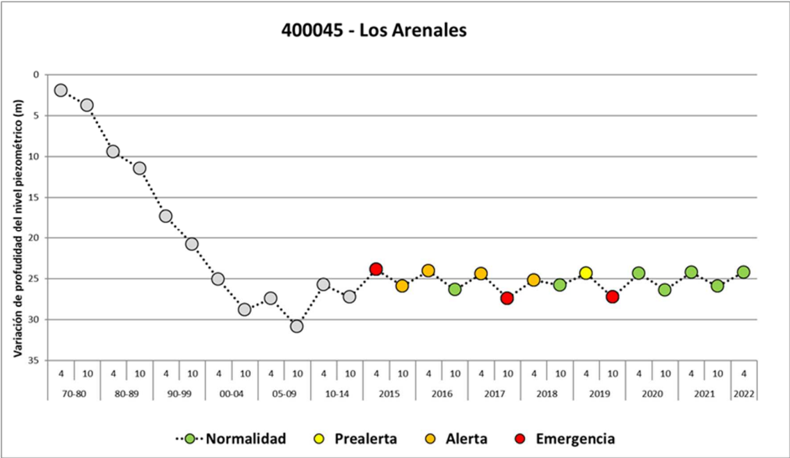
Figura 59. Evolución del Índice de estado de escasez en la MASub de Los Arenales
