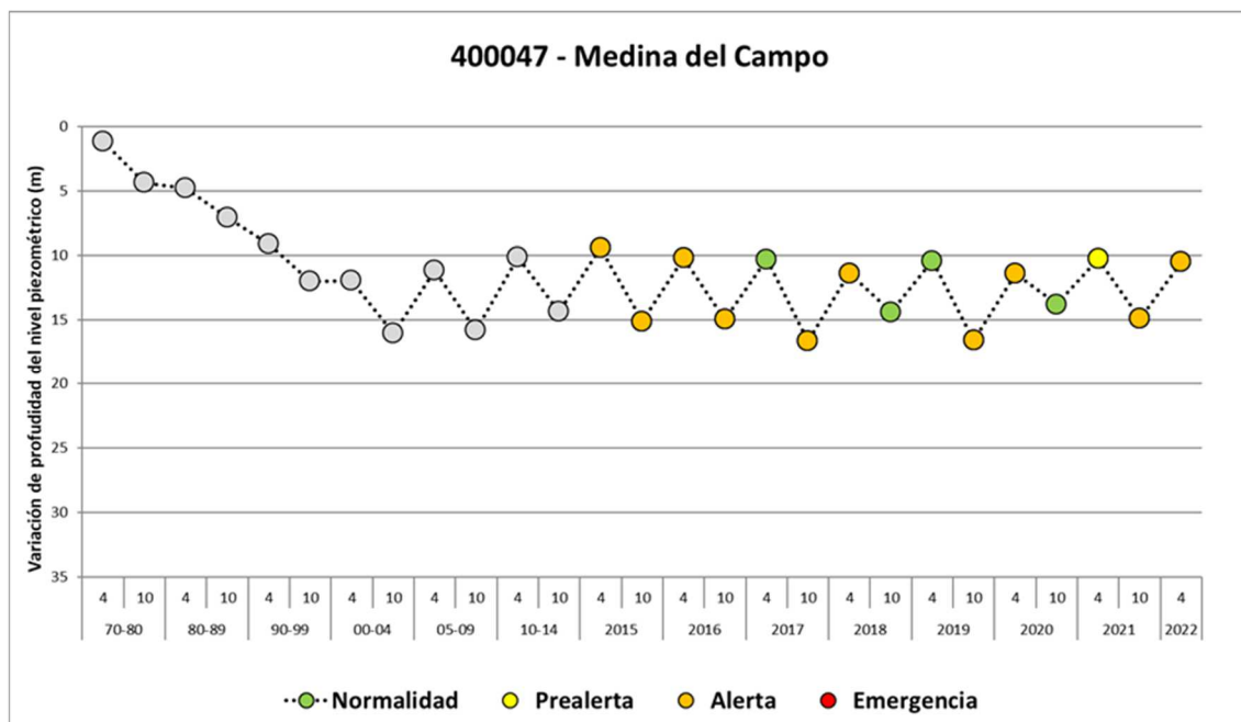
Figura 60. Evolución del Índice de estado de escasez en la MASub de Medina del Campo
