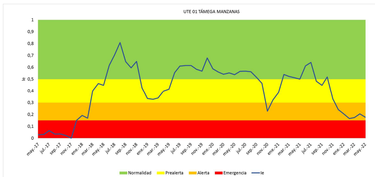
Figura 5. Evolución del Índice de estado de escasez en la UTE 01 Támea Manzanillas en los últimos 5 años
