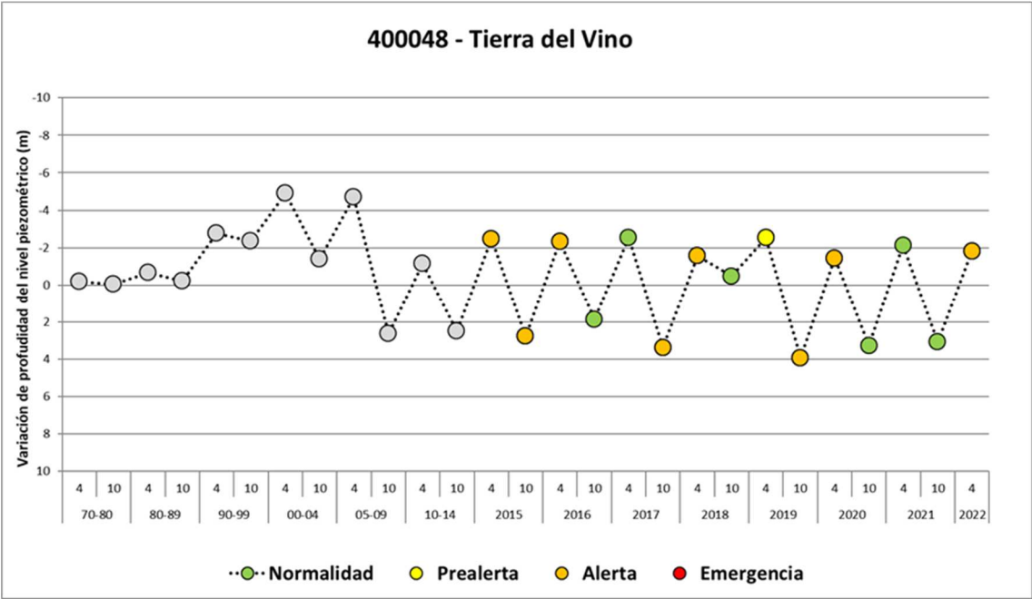
Figura 61. Evolución del Índice de estado de escasez en la MASub de Tierra del Vino
