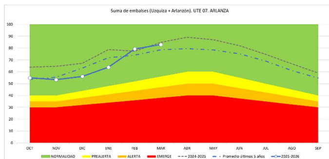
Figura 28. Umbrales mensuales para cada escenario de escasez en la UTE 07 Arlanza. Suma de embalses (Uzquiza-Arlanzón)
