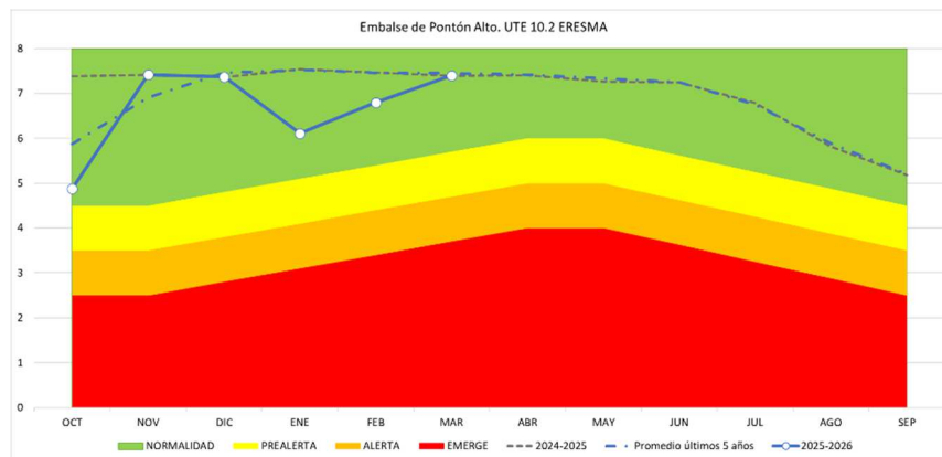
Figura 41. Umbrales mensuales para cada escenario de escasez en la UTE 10.2 Eresma. Embalse de Pontón Alto
