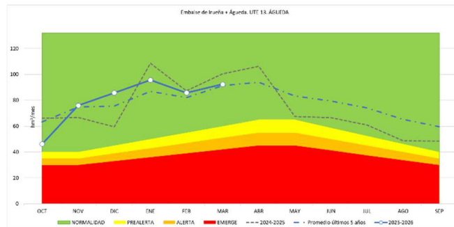
Figura 56. Umbrales mensuales para cada escenario de escasez en la UTE 13 Águeda. Embalse de Iruña-Águeda
