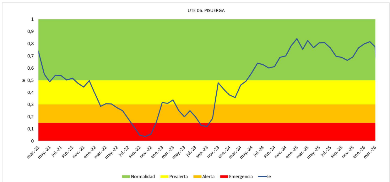
Figura 24. Evolución del Índice de estado de escasez en la UTE 06 Pisuegra en los últimos 5 años
