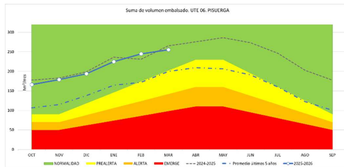
Figura 25. Umbrales mensuales para cada escenario de escasez en la UTE 06 Pisuegra. Suma de embalses(Aguilar de Campoo-Requejada-Cervera)
