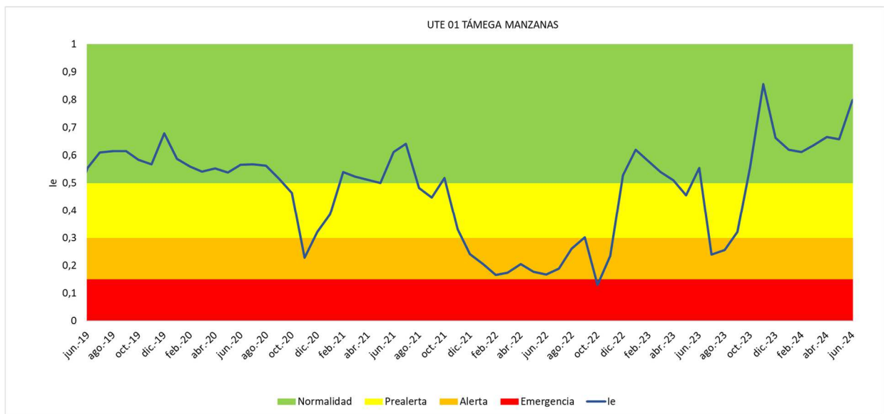
Figura 5. Evolución del Índice de estado de escasez en la UTE 01 Támeaga Manzanas en los últimos 5 años
