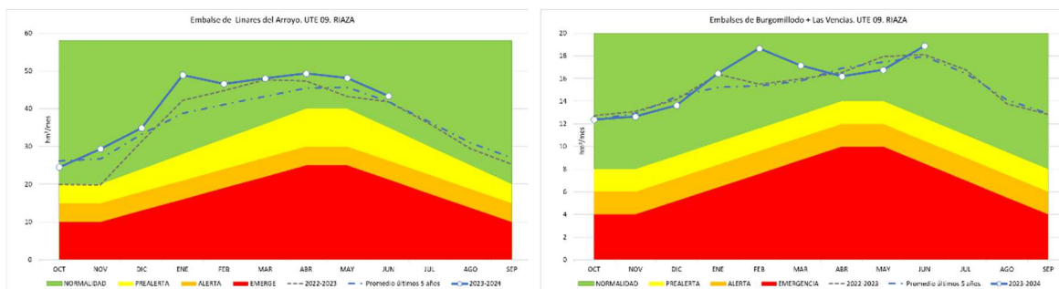
Figura 35. Umbrales mensuales para cada escenario de escasez en la UTE 09 Riaza Duratón
