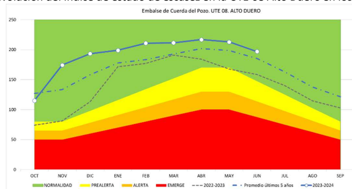
Figura 30. Evolución del Índice de estado de escasez en la UTE 08 Alto Duero en los últimos 5 años
