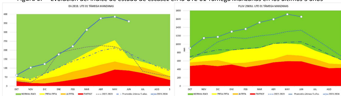
Figura 6. Umbrales mensuales para cada escenario de escasez en la UTE 01 Támeaga Manzanas
