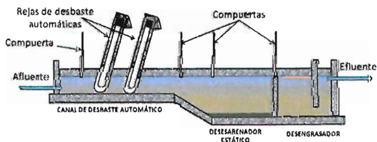
Esquema de pretratamiento con elementos de limpieza manual
