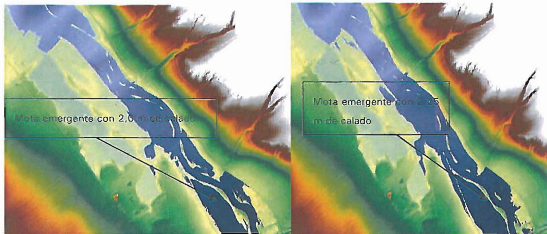
Ilustración 5 e Ilustración 6. Motas emergentes en dos láminas de inundación con diferentes calados
