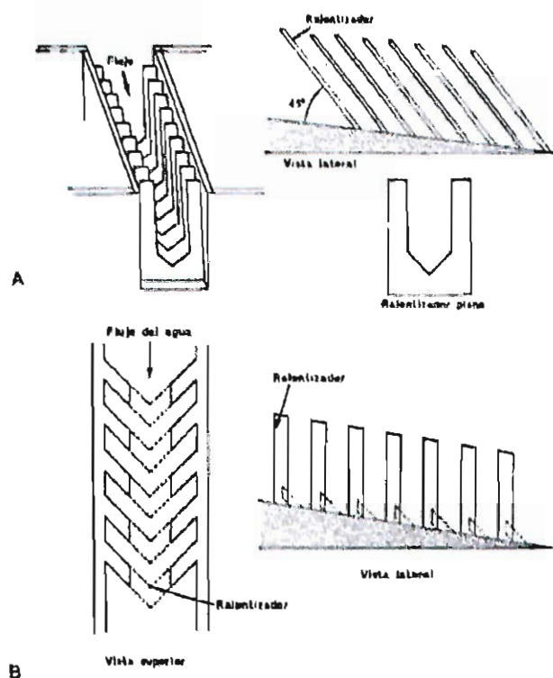
Sistema de deflectores-ralentizadores. A. Con ralentizadores planos. B. Con ralentizadores de tipo "Fatou". Fte: Cedex, 1998.
