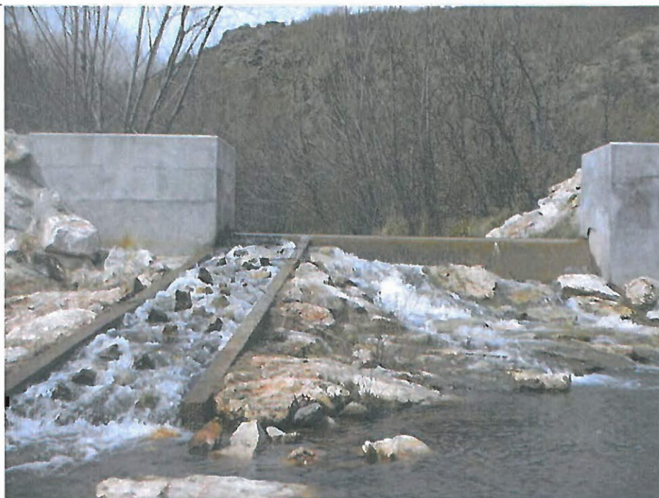
Escala para peces en el río Resoba, Palencia. Fte: Infraeco
