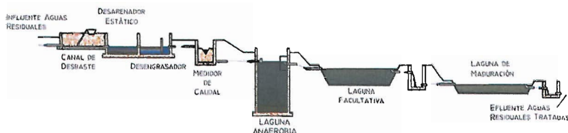
Esquema de un tratamiento de lagunaje
