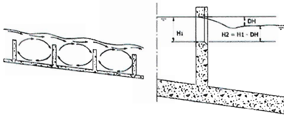
Vertido sumergido (H2) y vertido libre (DH). Estos pasos son menos selectivos, y por lo tanto pueden ser adecuados para los ciprínidos migradores. Fte: Larinier, 1992.
