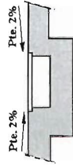
Detalle de drenaje
