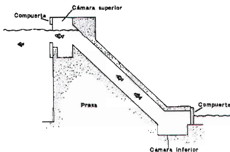
Esquema de esclusa típica para peces. Fte: Cedex, 1998.
