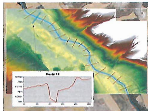
Ilustración 2: Secciones transversales en el cauce de estudio
