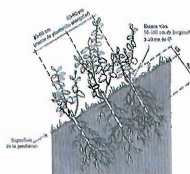
ESTACAS VIVAS
