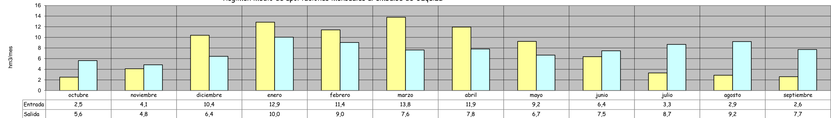
Régimen medio de aportaciones mensuales al embalse de Úzquiza
