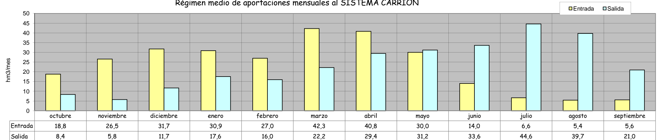
Régimen medio de aportaciones mensuales al SISTEMA CARRIÓN
