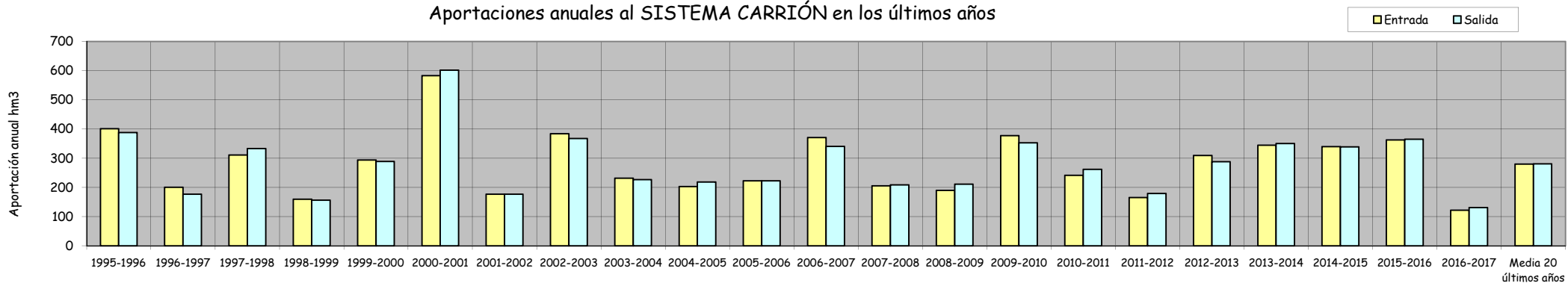
Aportaciones anuales al SISTEMA CARRIÓN en los últimos años
