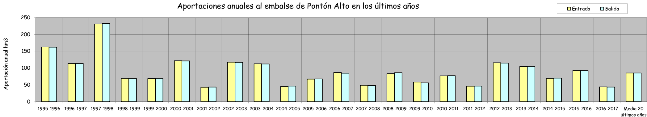
Régimen medio de aportaciones mensuales al embalse de Pontón Alto
