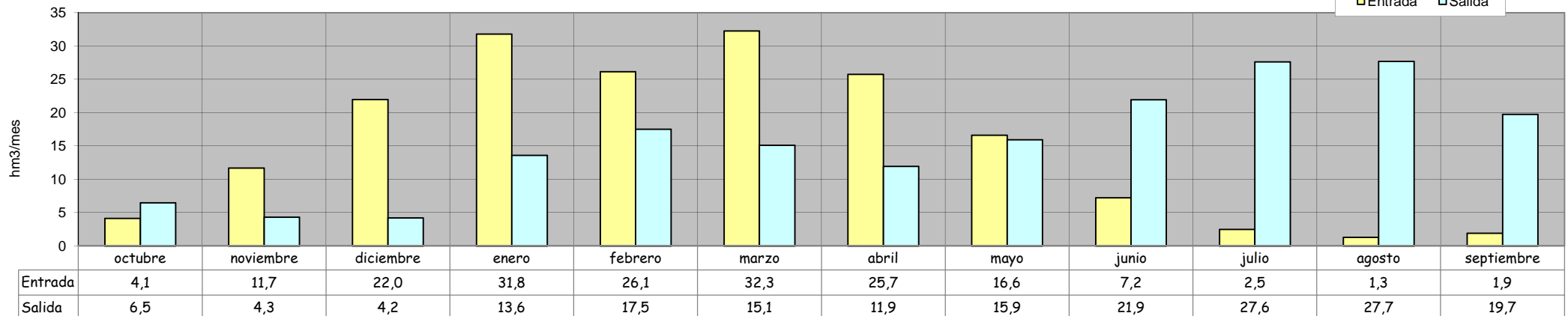
Régimen medio de aportaciones mensuales al embalse de Cuerda del Pozo
