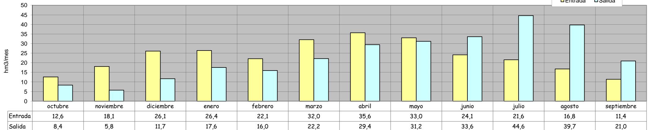
Régimen medio de aportaciones mensuales al embalse de Compuerto
