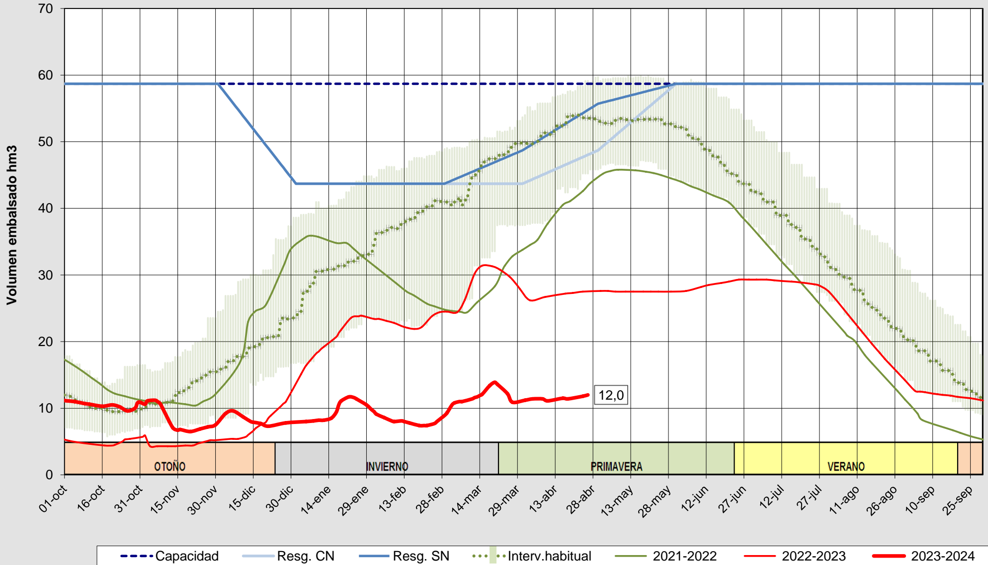
Evolución del volumen almacenado en el embalse de Requejada a fecha 26/04/2024
