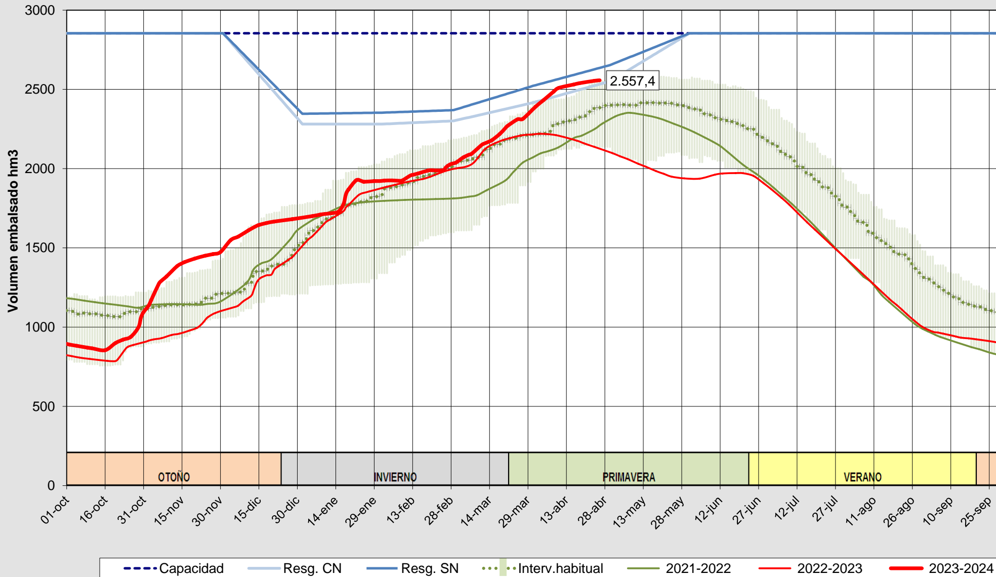
Evolución del volumen almacenado en el sistema del DUERO (ESTADO) a fecha 26/04/2024
