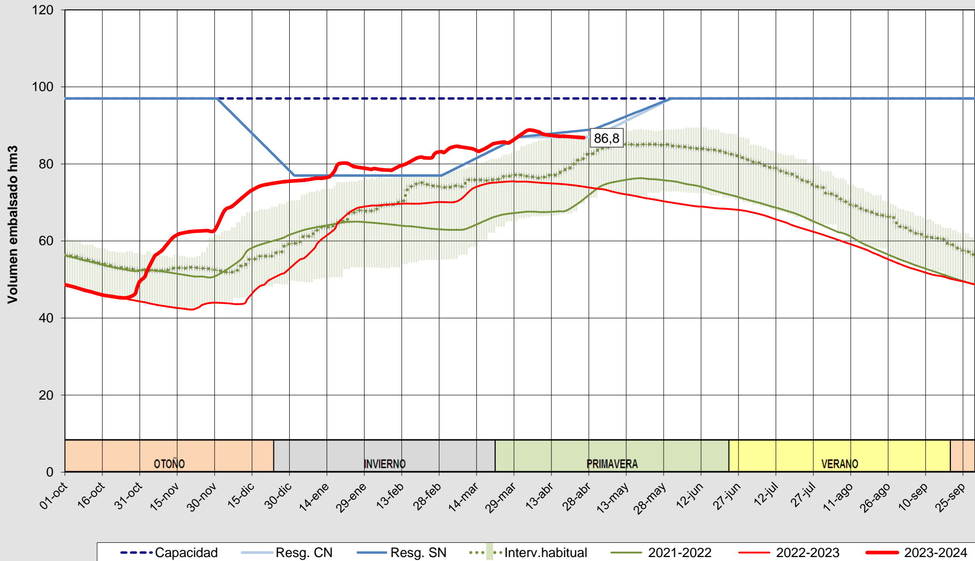
Evolución del volumen almacenado en el sistema del ARLANZÓN a fecha 26/04/2024
