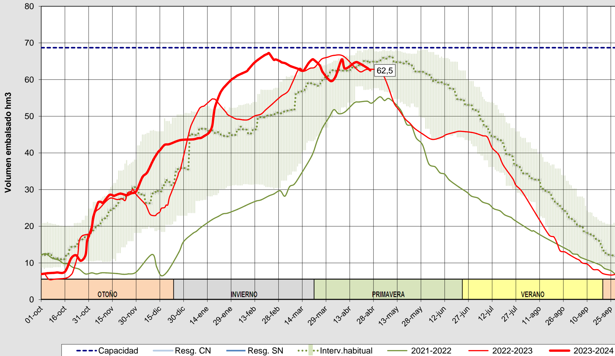
Evolución del volumen almacenado en el embalse de Camporredondo a fecha 26/04/2024
