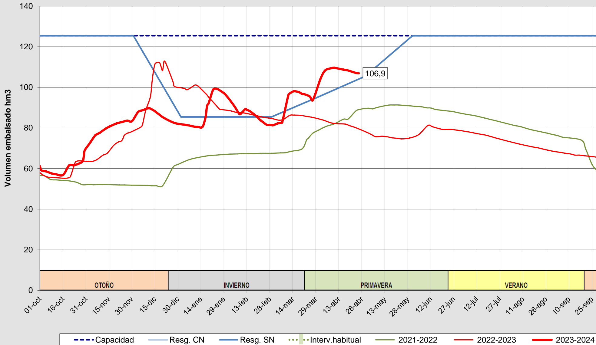
Evolución del volumen almacenado en el sistema del ÁGUEDA a fecha 26/04/2024
