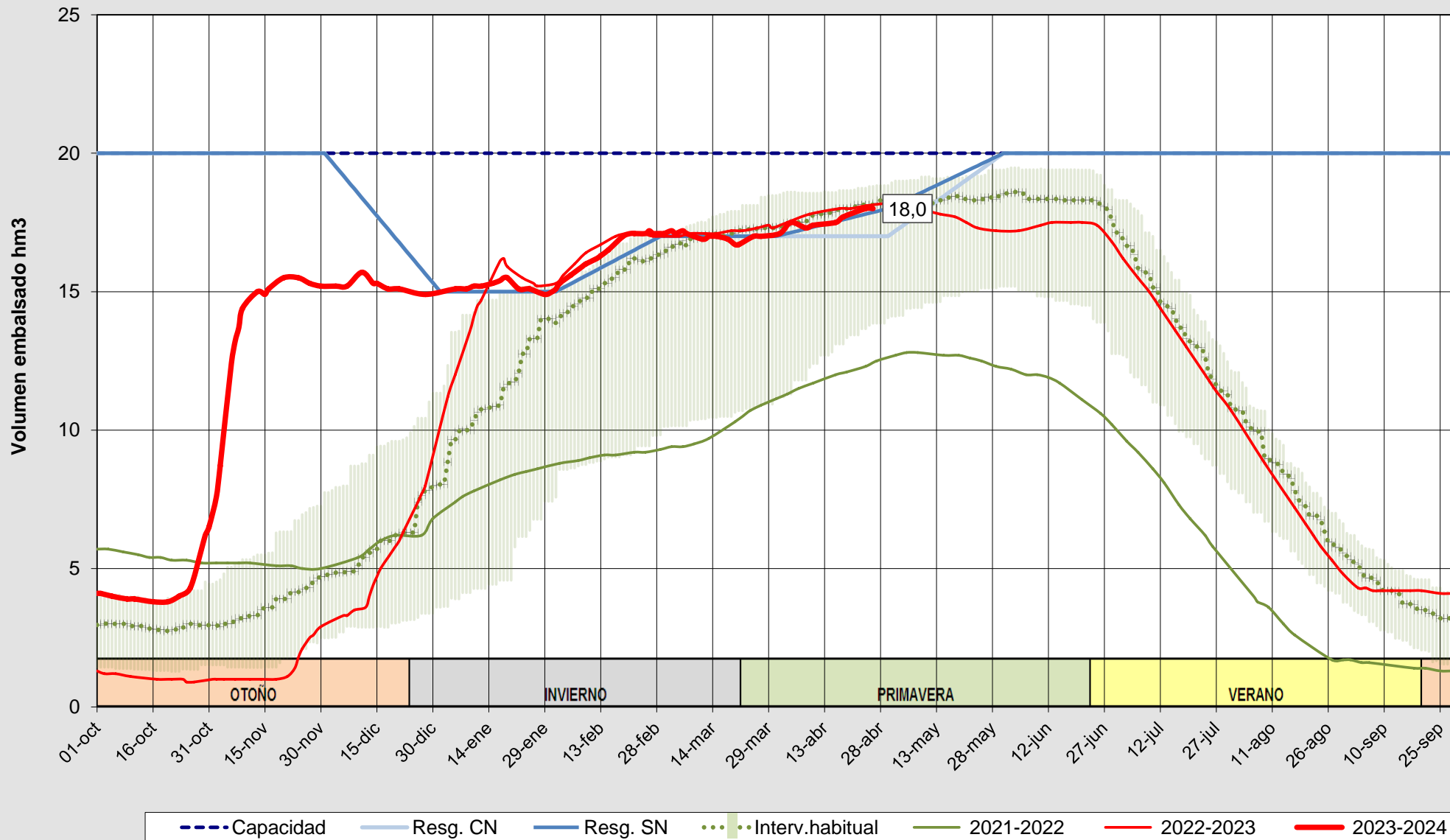
Evolución del volumen almacenado en el embalse de Villameca a fecha 26/04/2024
