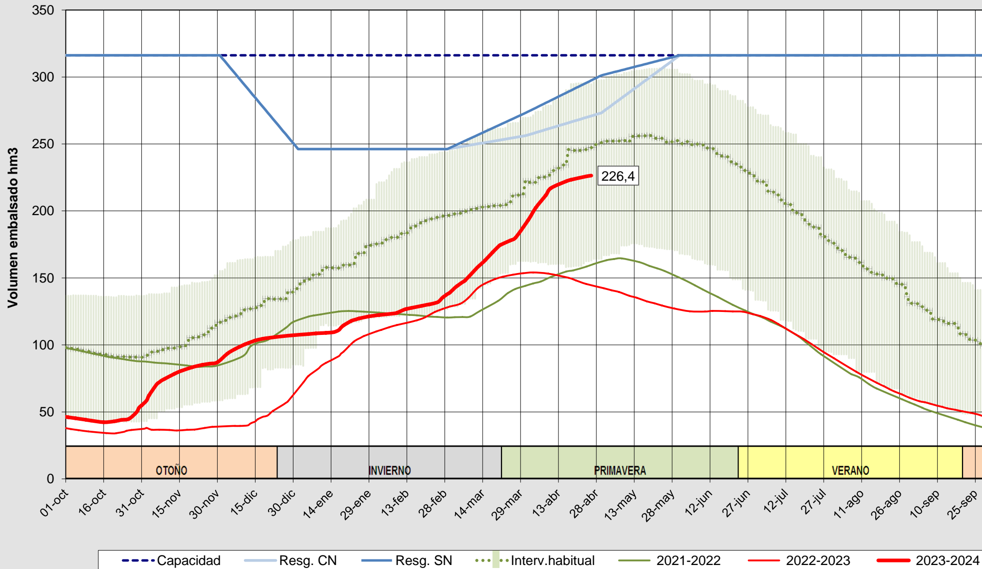
Evolución del volumen almacenado en el sistema del PISUERGA a fecha 26/04/2024
