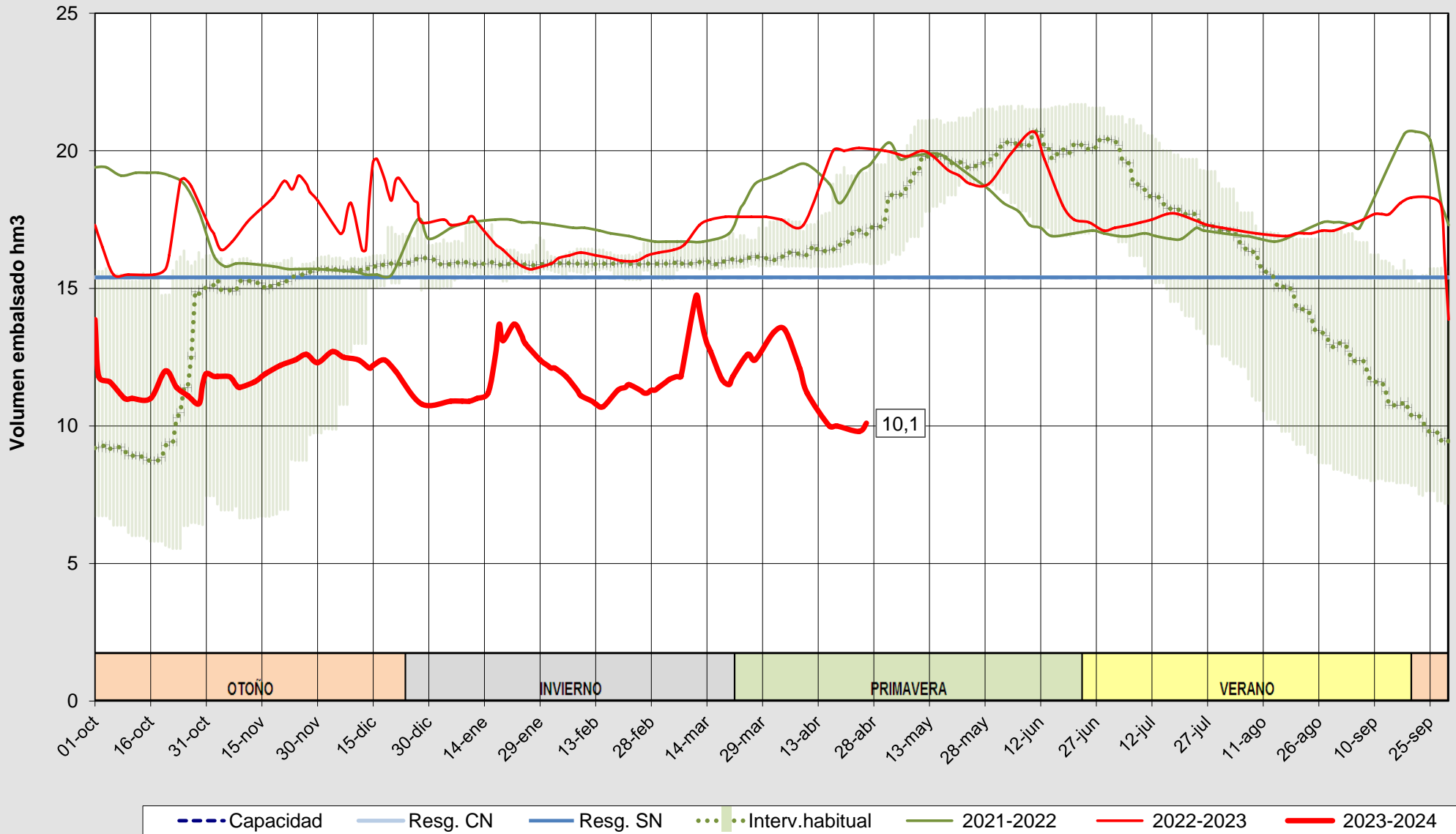
Evolución del volumen almacenado en el embalse de Águeda a fecha 26/04/2024
