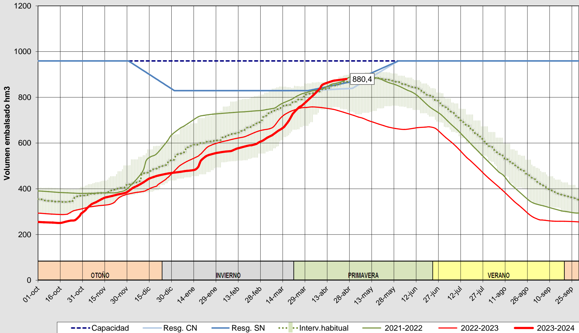
Evolución del volumen almacenado en el sistema del PORMA-ESLA a fecha 26/04/2024
