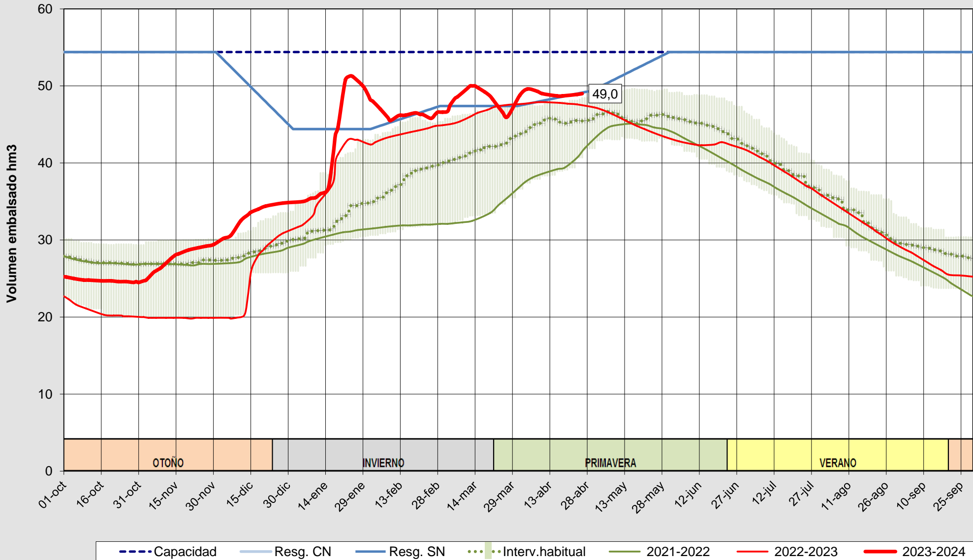
Evolución del volumen almacenado en el embalse de Linares del Arroyo a fecha 26/04/2024
