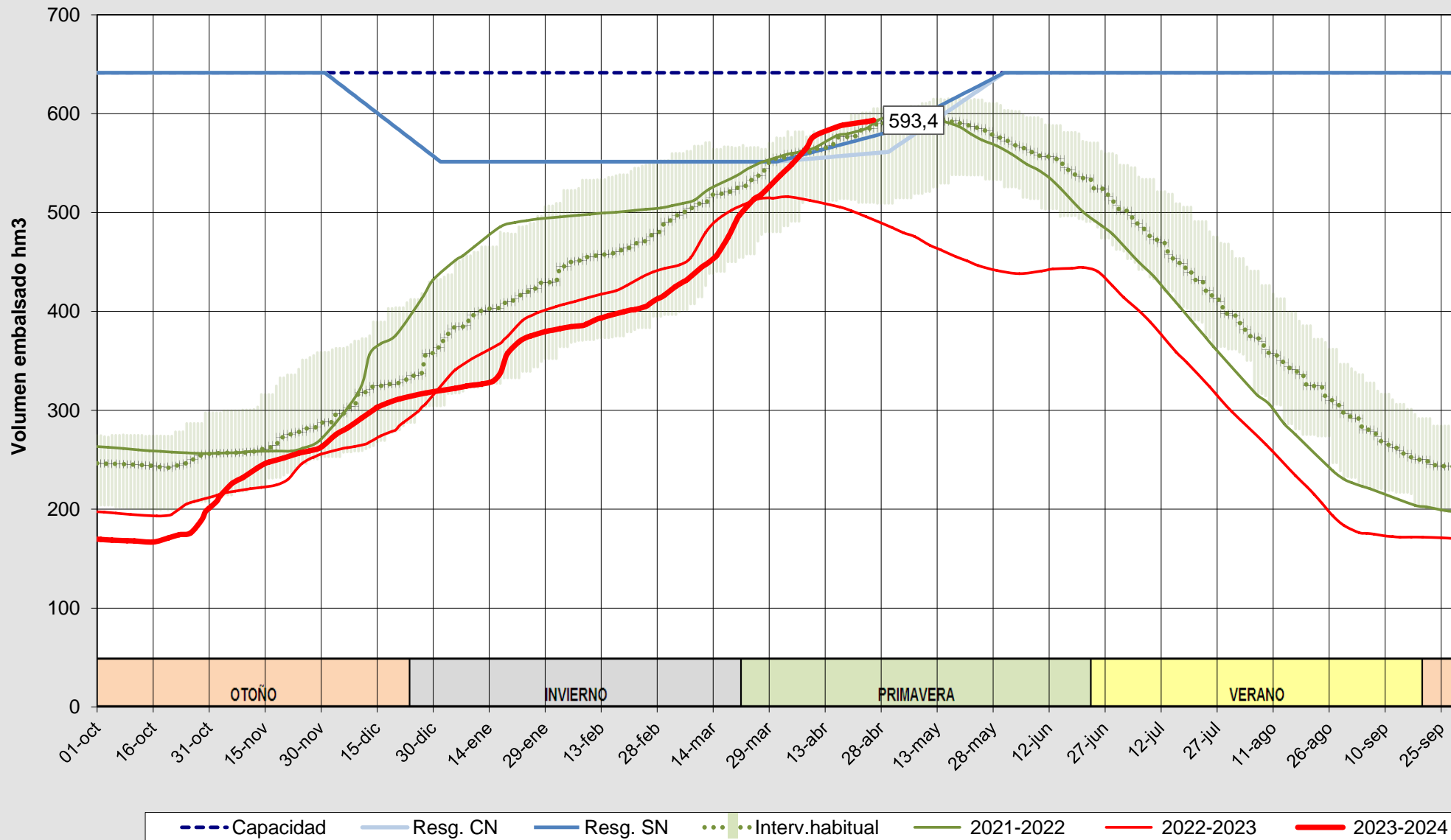
Evolución del volumen almacenado en el embalse de Riaño a fecha 26/04/2024
