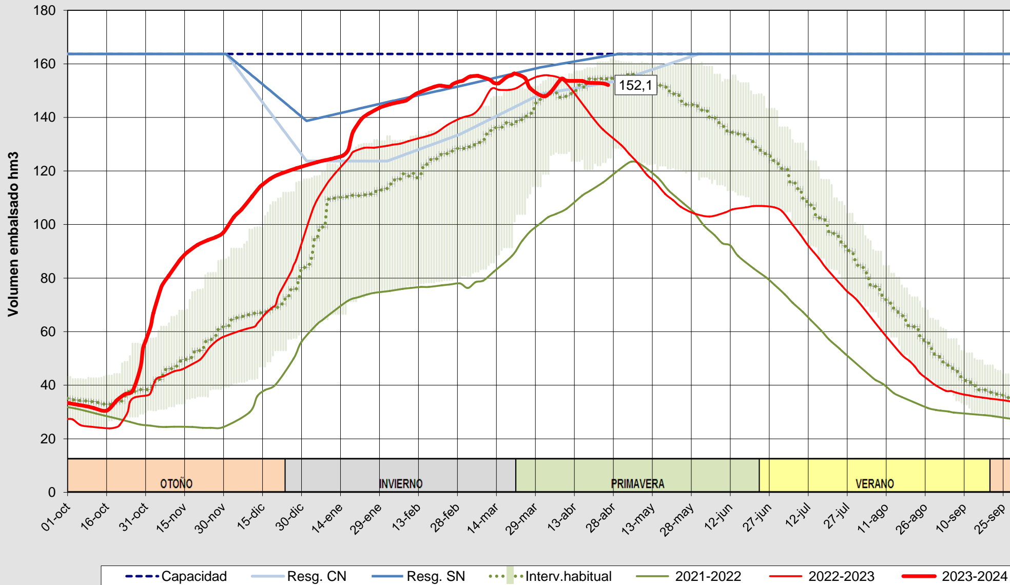
Evolución del volumen almacenado en el sistema del CARRIÓN a fecha 26/04/2024
