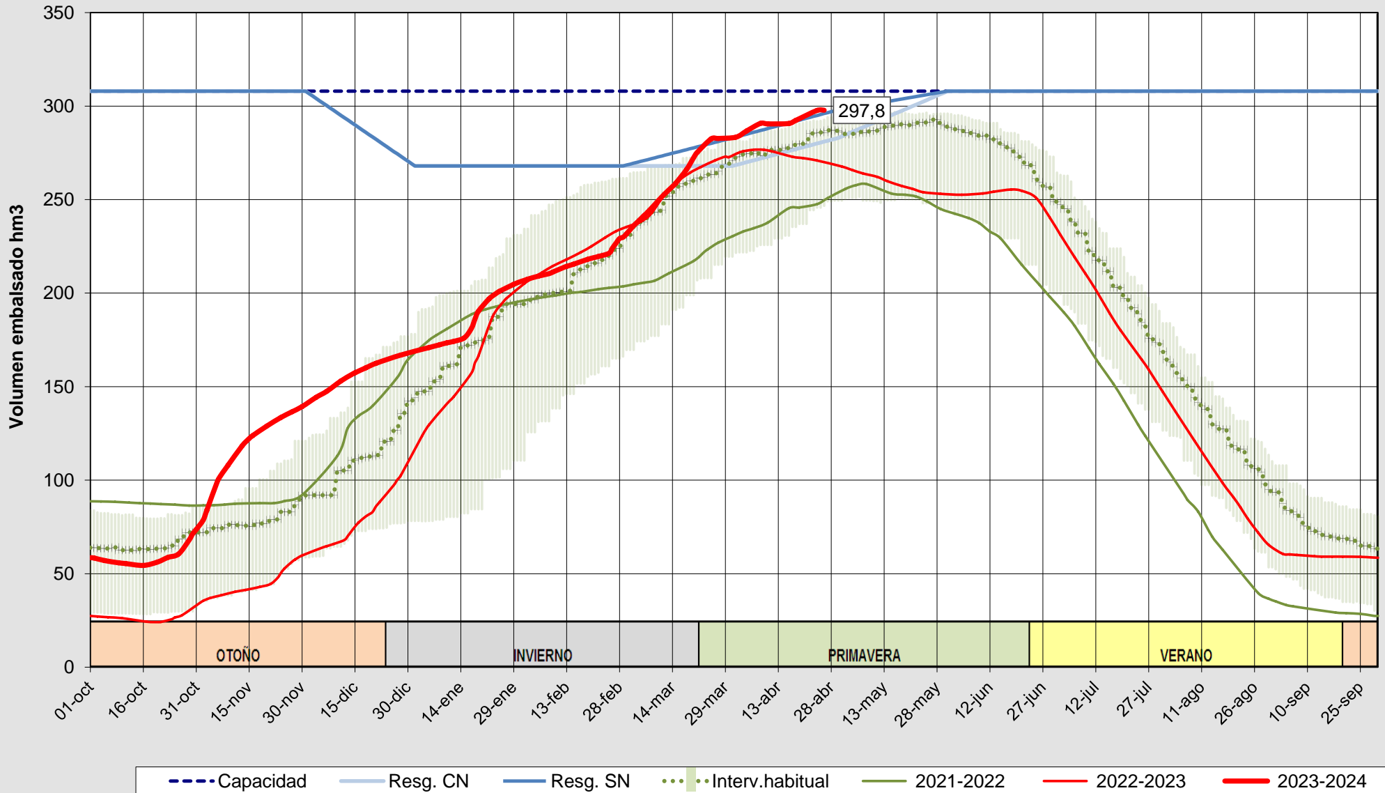
Evolución del volumen almacenado en el embalse de Barrios de Luna a fecha 26/04/2024
