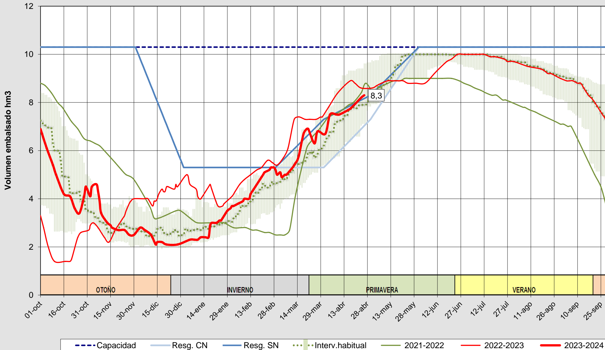
Evolución del volumen almacenado en el embalse de Cervera a fecha 26/04/2024
