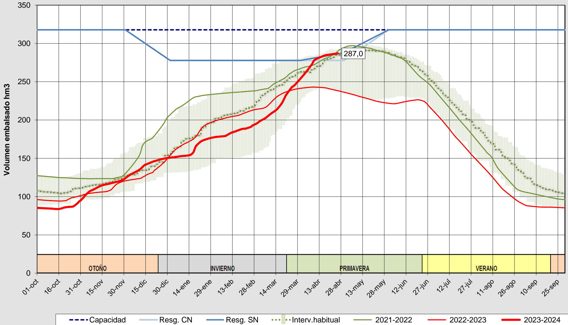
Evolución del volumen almacenado en el embalse de Porma a fecha 26/04/2024
