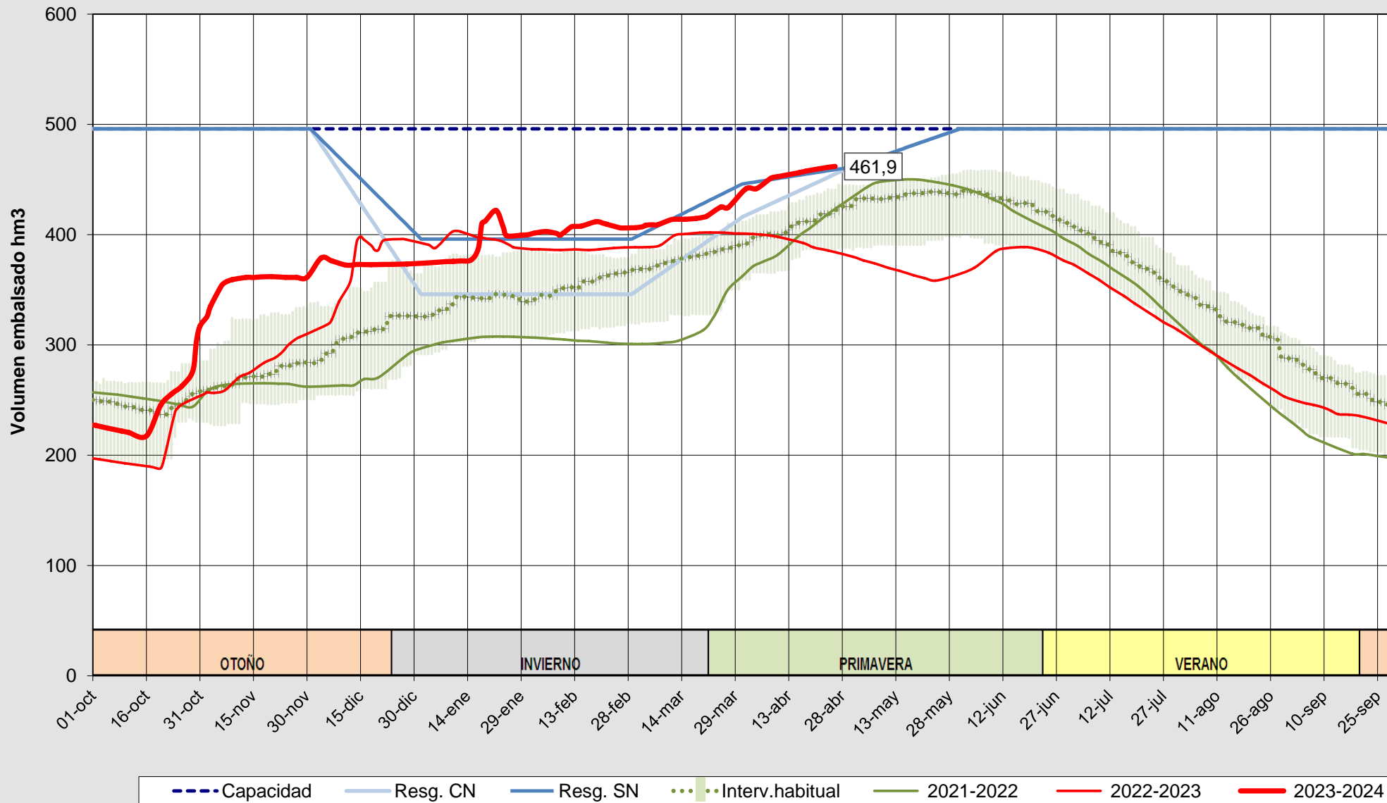
Evolución del volumen almacenado en el embalse de Santa Teresa a fecha 26/04/2024
