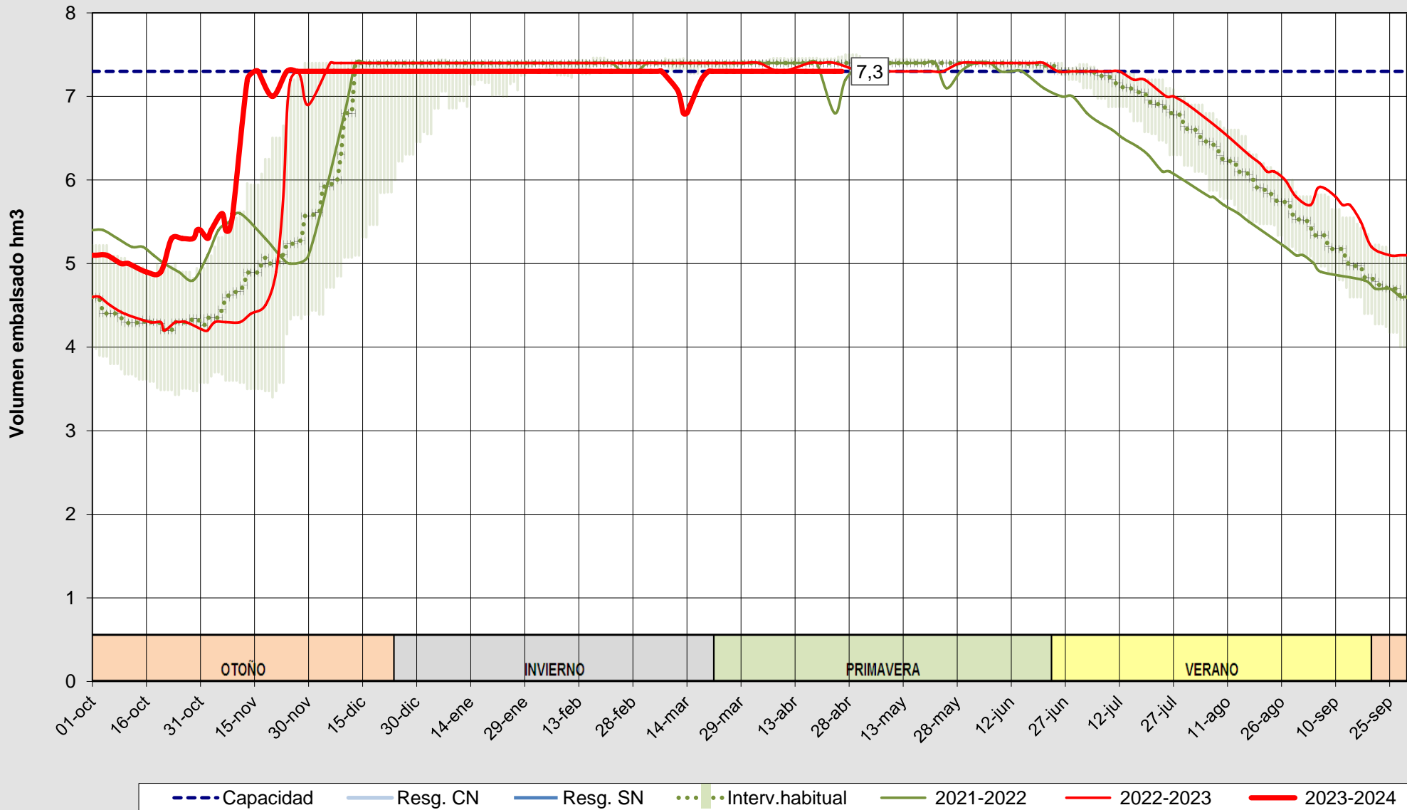
Evolución del volumen almacenado en el embalse de Pontón Alto a fecha 26/04/2024
