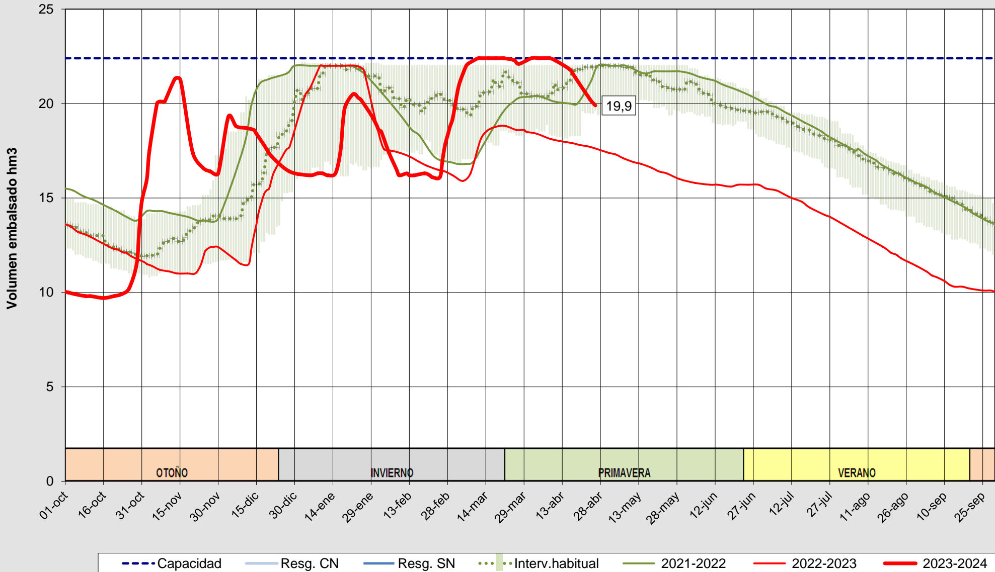
Evolución del volumen almacenado en el embalse de Arlanzón a fecha 26/04/2024
