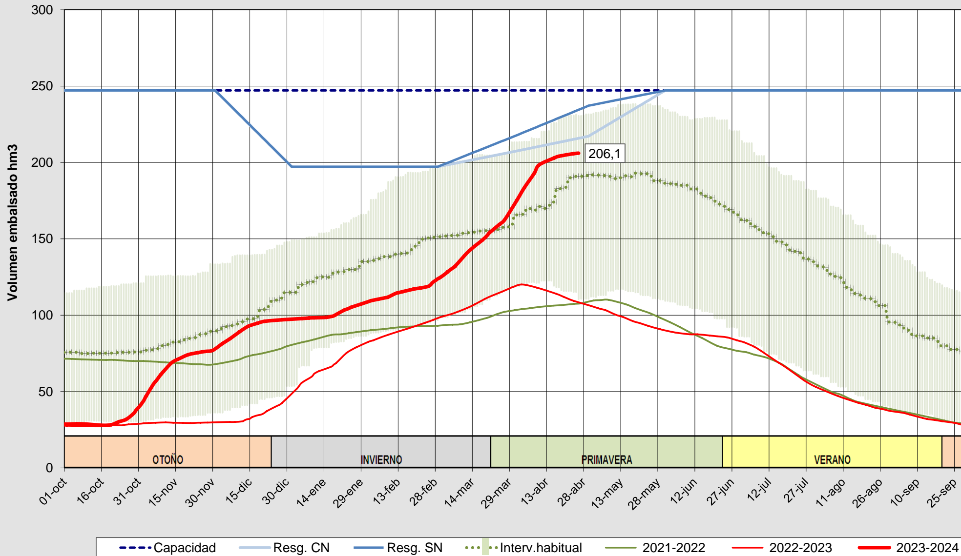
Evolución del volumen almacenado en el embalse de Aguilar a fecha 26/04/2024
