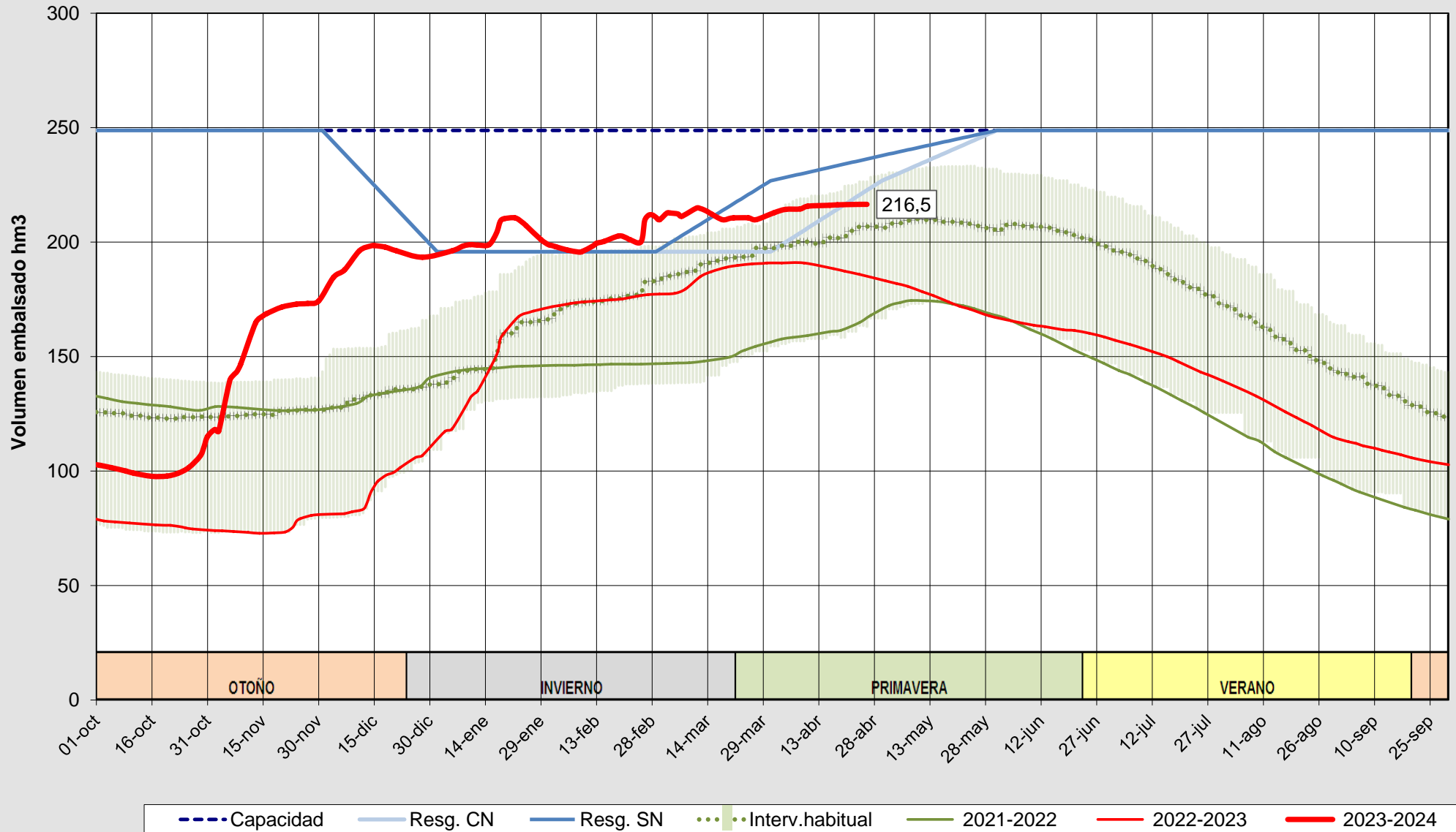
Evolución del volumen almacenado en el embalse de Cuerda del Pozo a fecha 26/04/2024
