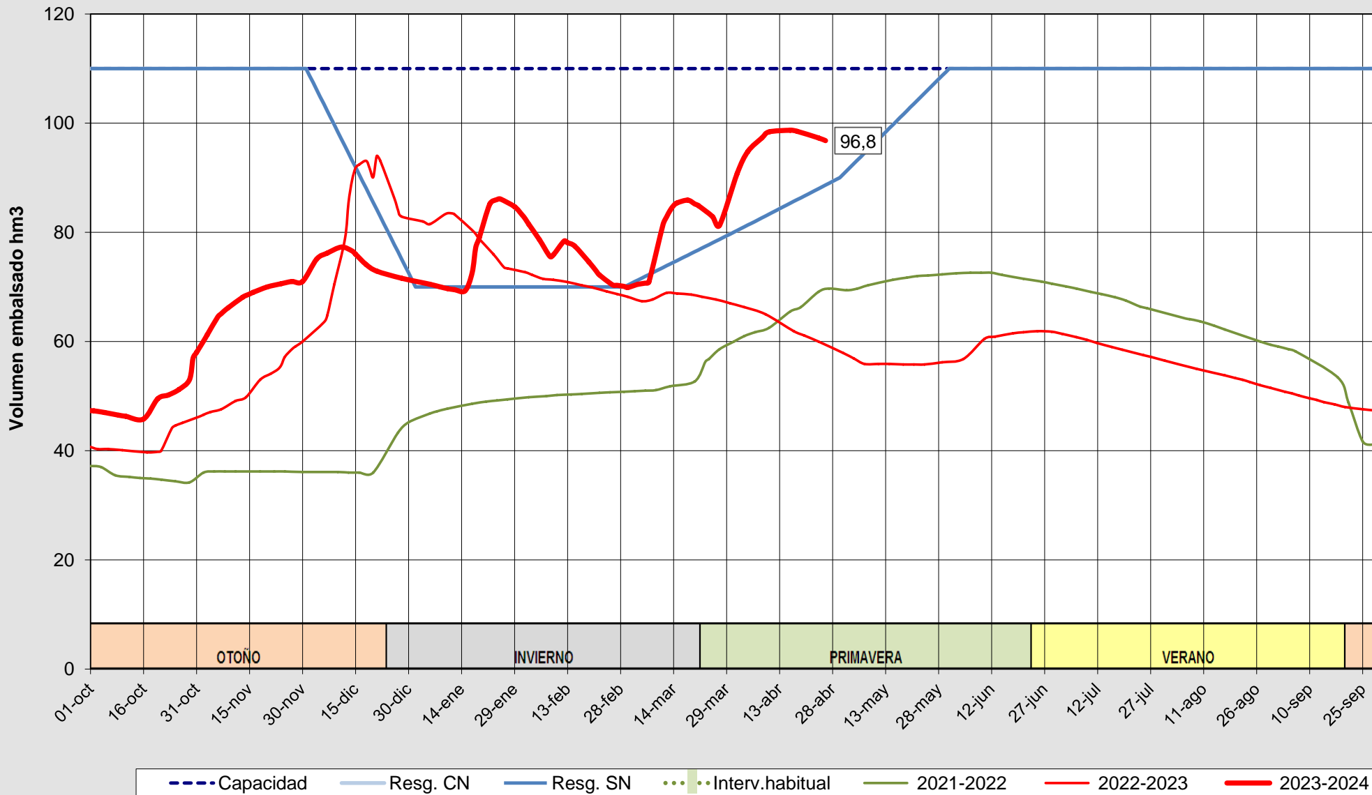
Evolución del volumen almacenado en el embalse de Iruña a fecha 26/04/2024
