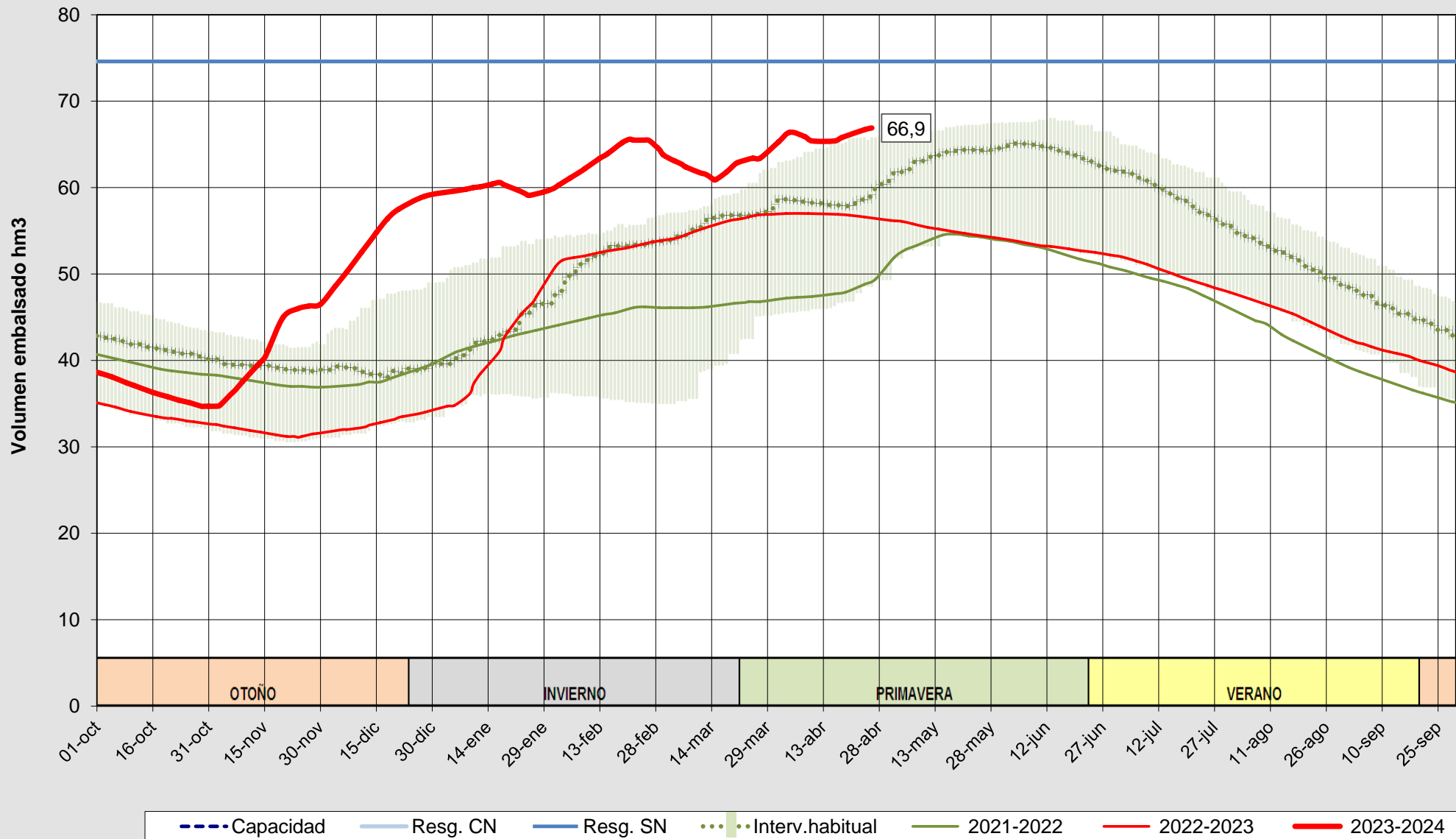
Evolución del volumen almacenado en el embalse de Úzquiza a fecha 26/04/2024
