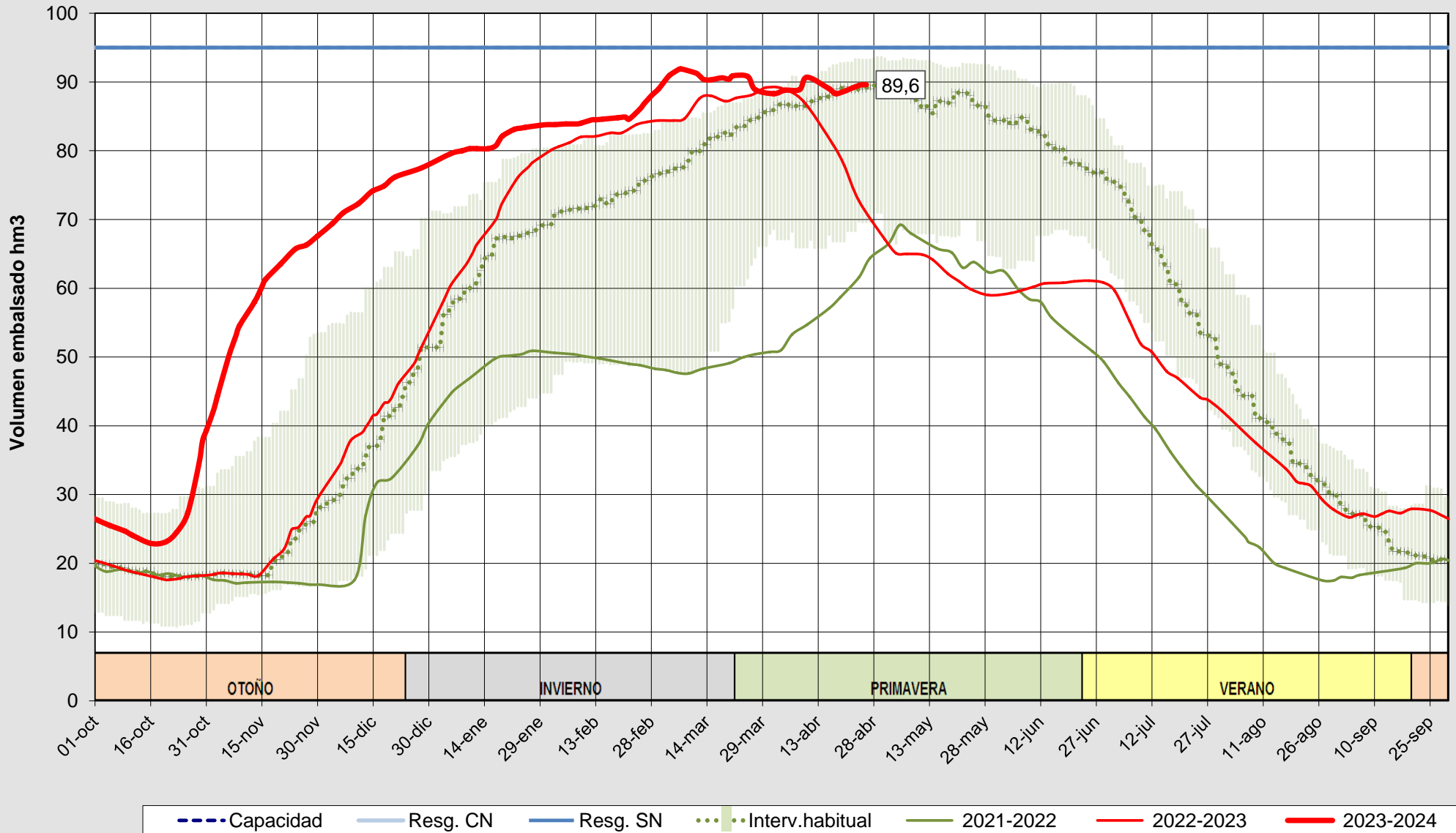
Evolución del volumen almacenado en el embalse de Compuerto a fecha 26/04/2024
