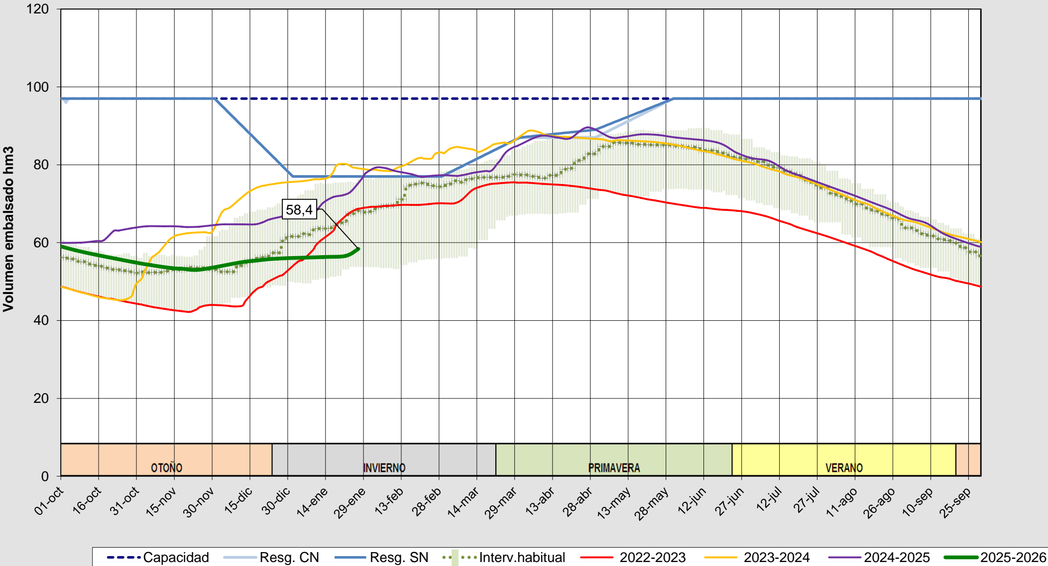
Evolución del volumen almacenado en el sistema del ARLANZÓN a fecha 27/01/2026
