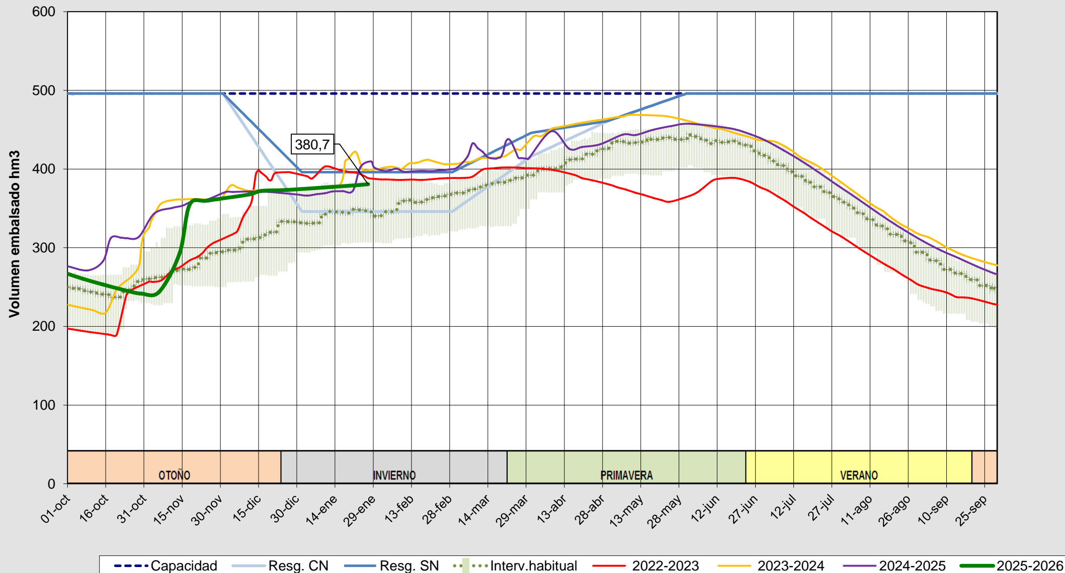
Evolución del volumen almacenado en el embalse de Santa Teresa a fecha 27/01/2026
