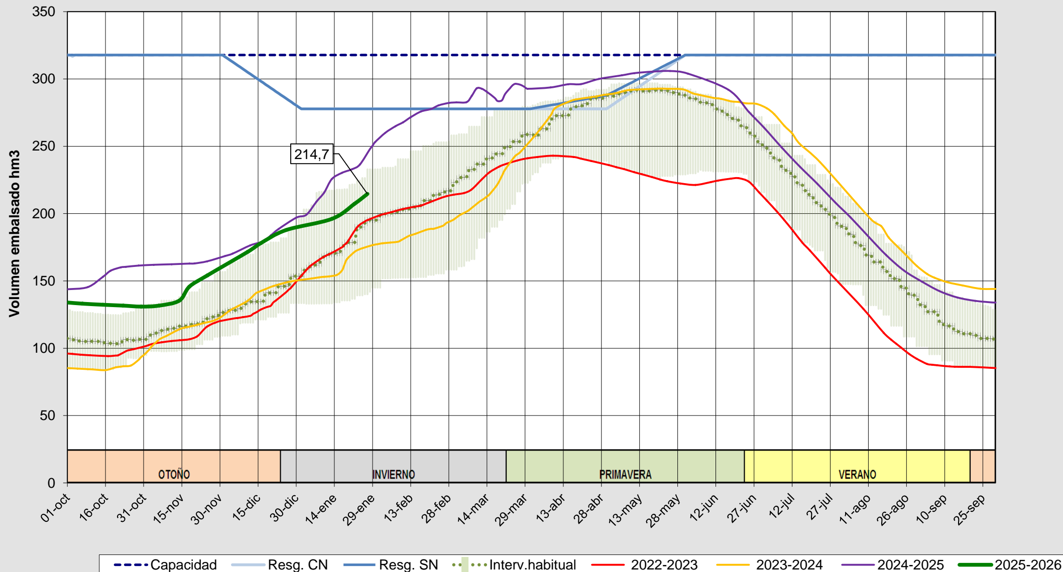
Evolución del volumen almacenado en el embalse de Porma a fecha 27/01/2026
