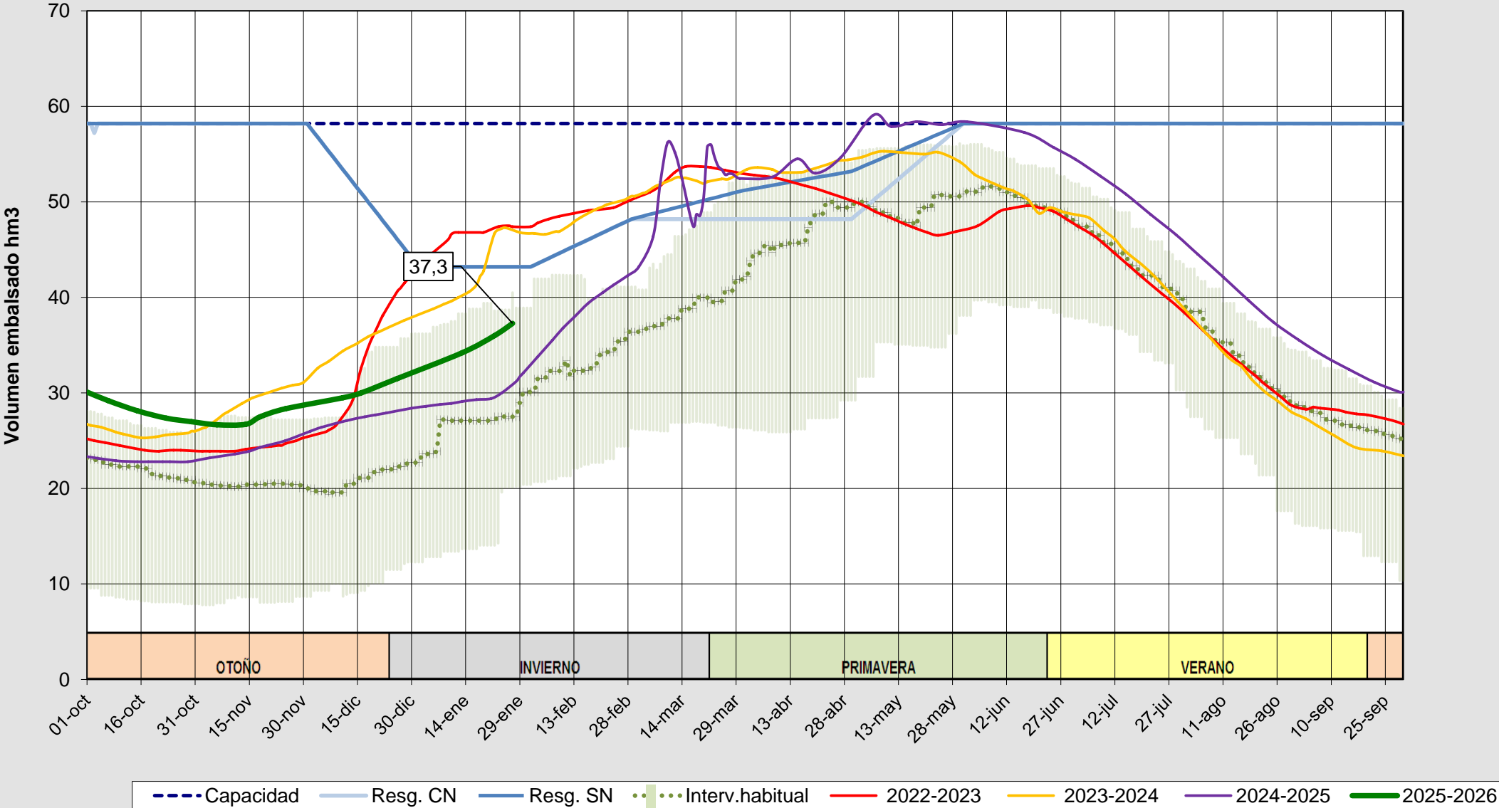
Evolución del volumen almacenado en el embalse de Las Cogotas a fecha 27/01/2026
