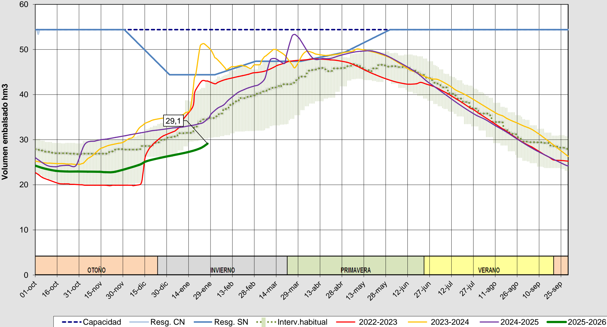
Evolución del volumen almacenado en el embalse de Linares del Arroyo a fecha 27/01/2026
