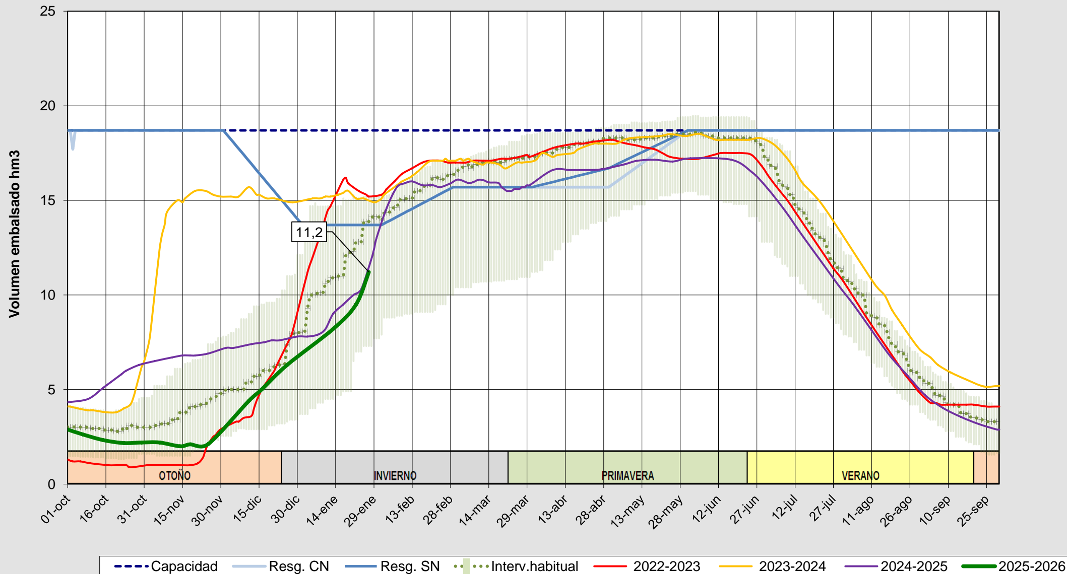
Evolución del volumen almacenado en el embalse de Villameca a fecha 27/01/2026
