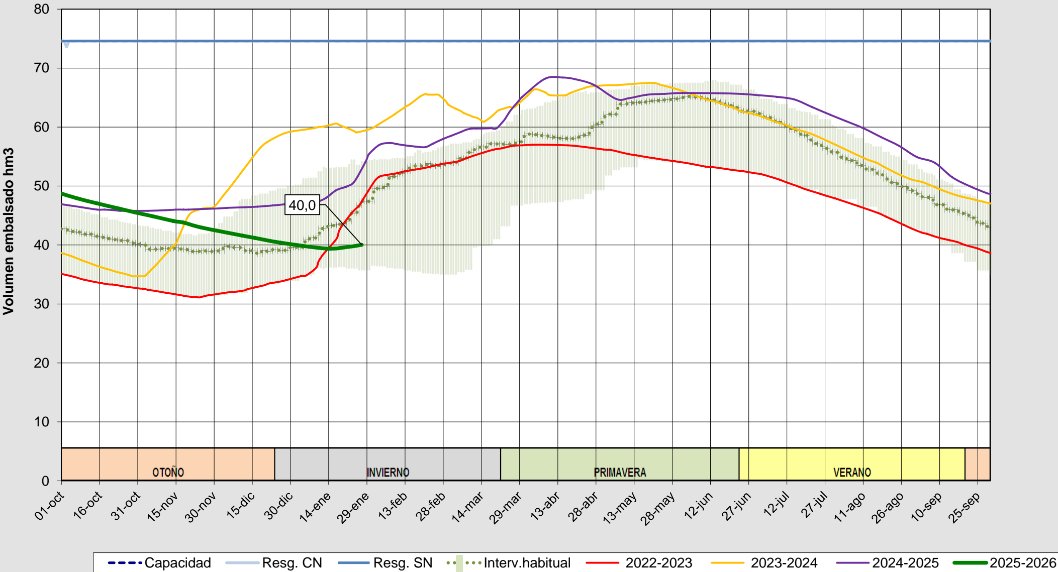
Evolución del volumen almacenado en el embalse de Úzquiza a fecha 27/01/2026
