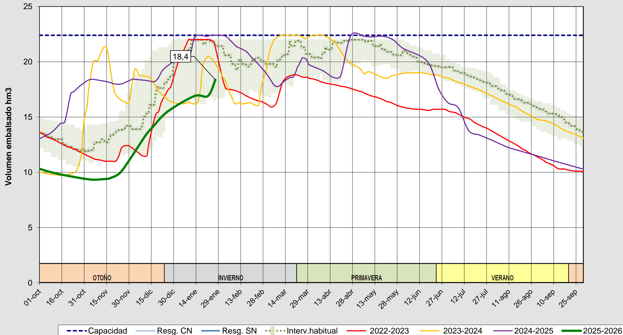
Evolución del volumen almacenado en el embalse de Arlanzón a fecha 27/01/2026
