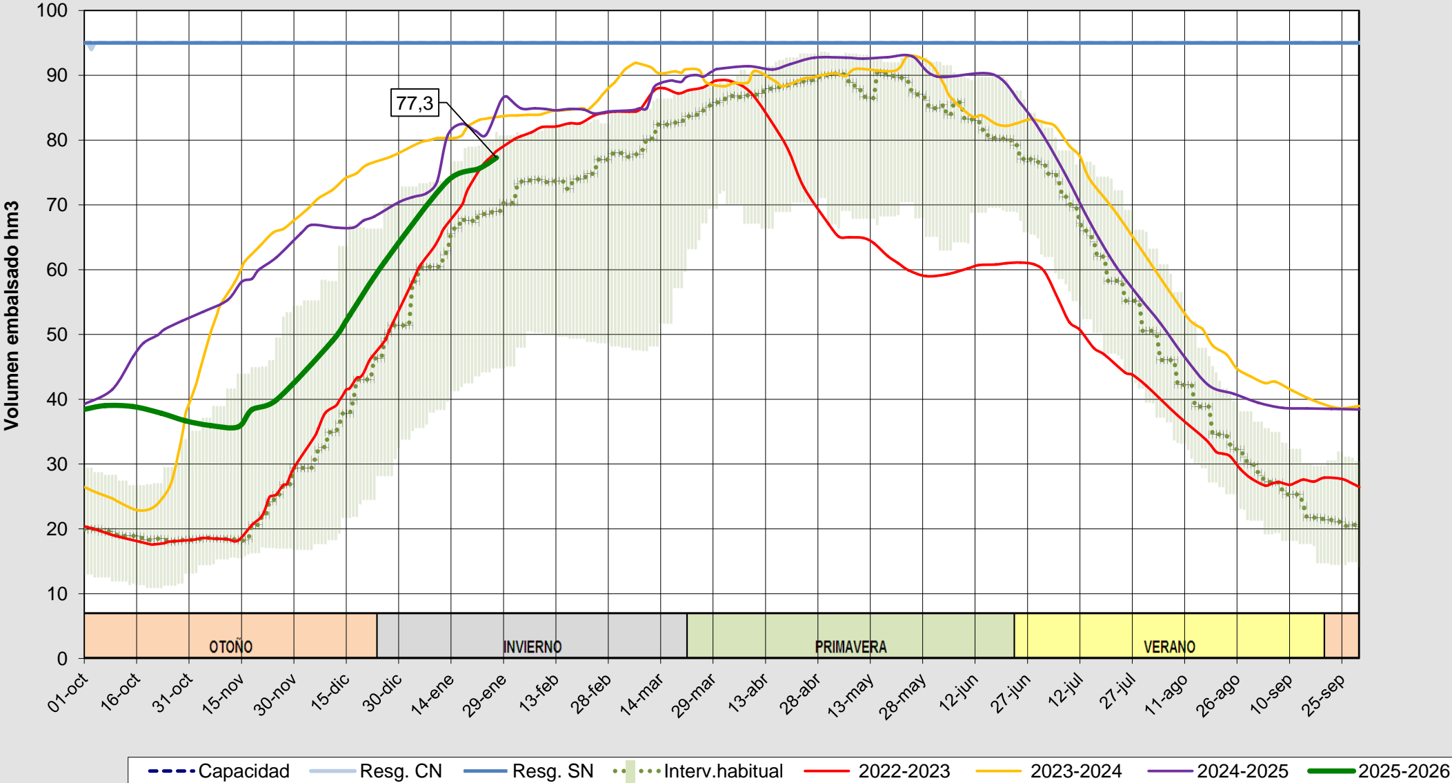
Evolución del volumen almacenado en el embalse de Compuerto a fecha 27/01/2026
