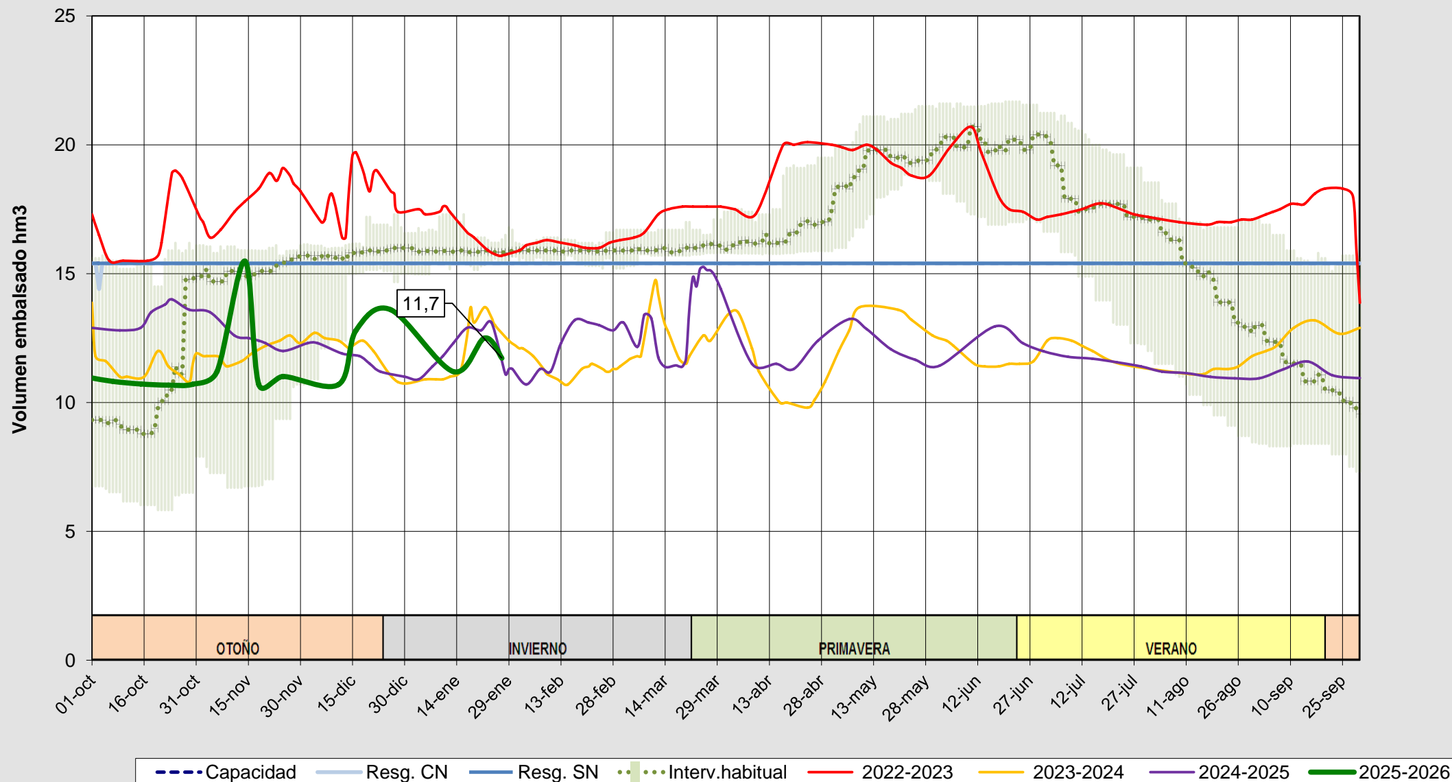
Evolución del volumen almacenado en el embalse de Águeda a fecha 27/01/2026
