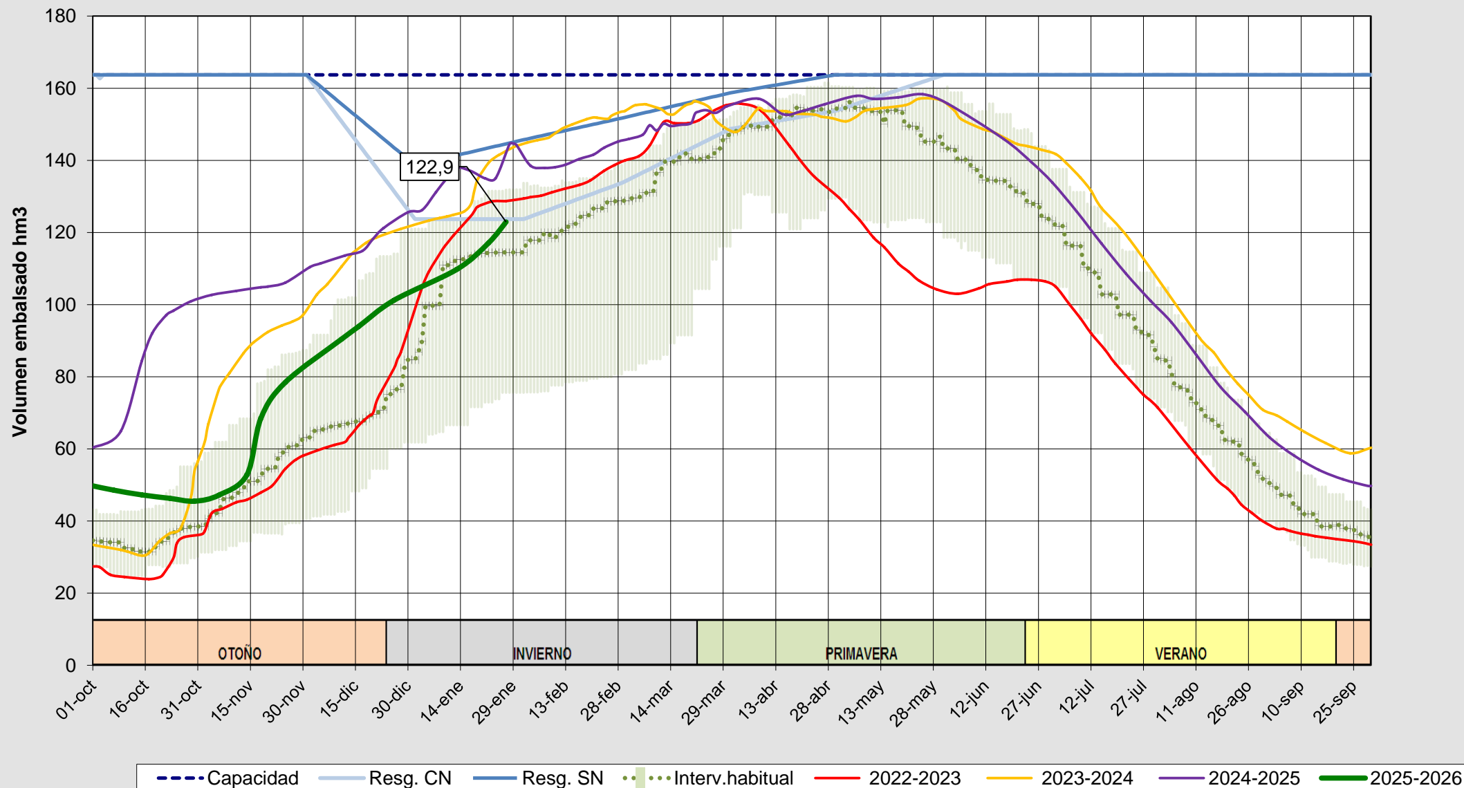
Evolución del volumen almacenado en el sistema del CARRIÓN a fecha 27/01/2026
