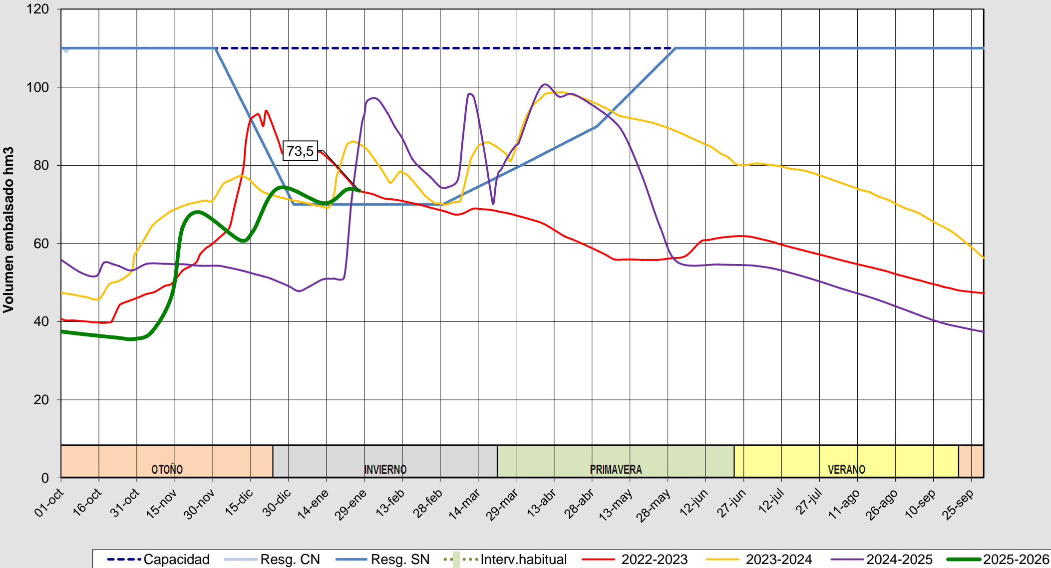
Evolución del volumen almacenado en el embalse de Irueña a fecha 27/01/2026
