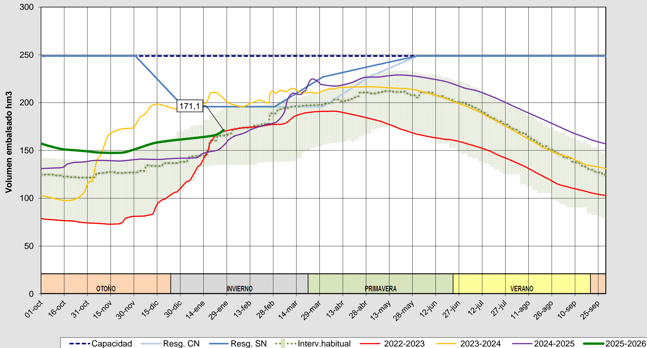
Evolución del volumen almacenado en el embalse de Cuerda del Pozo a fecha 27/01/2026
