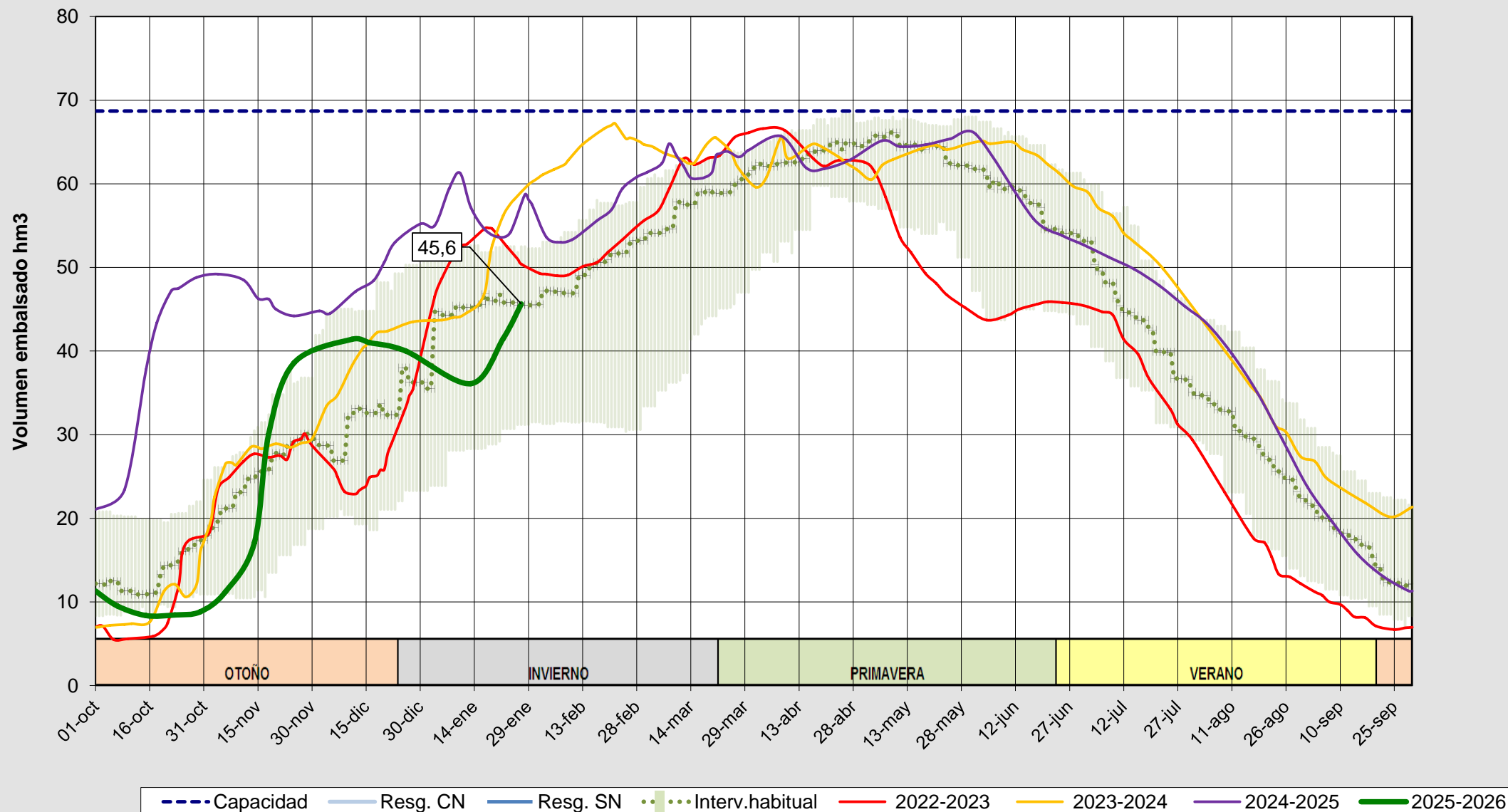
Evolución del volumen almacenado en el embalse de Camporredondo a fecha 27/01/2026
