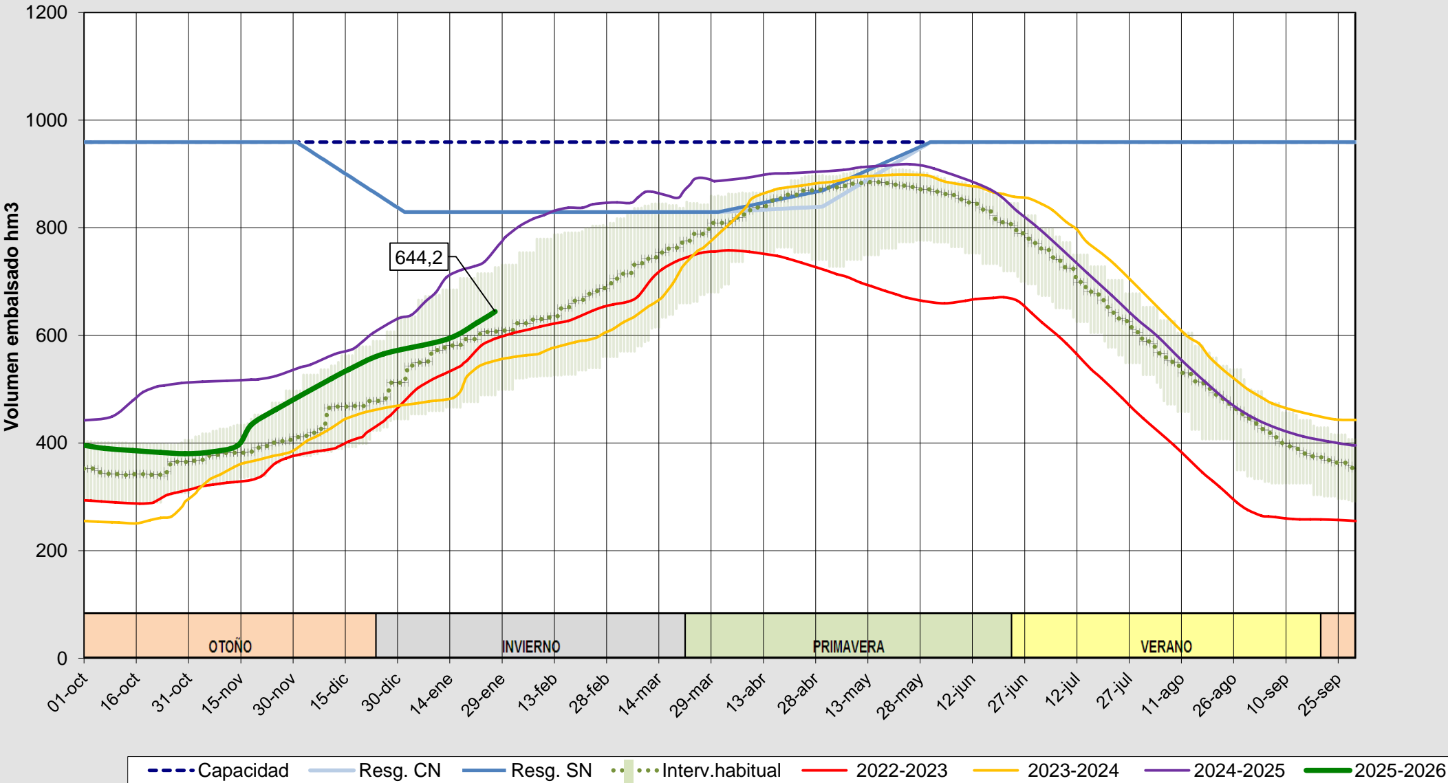
Evolución del volumen almacenado en el sistema del PORMA-ESLA a fecha 27/01/2026
