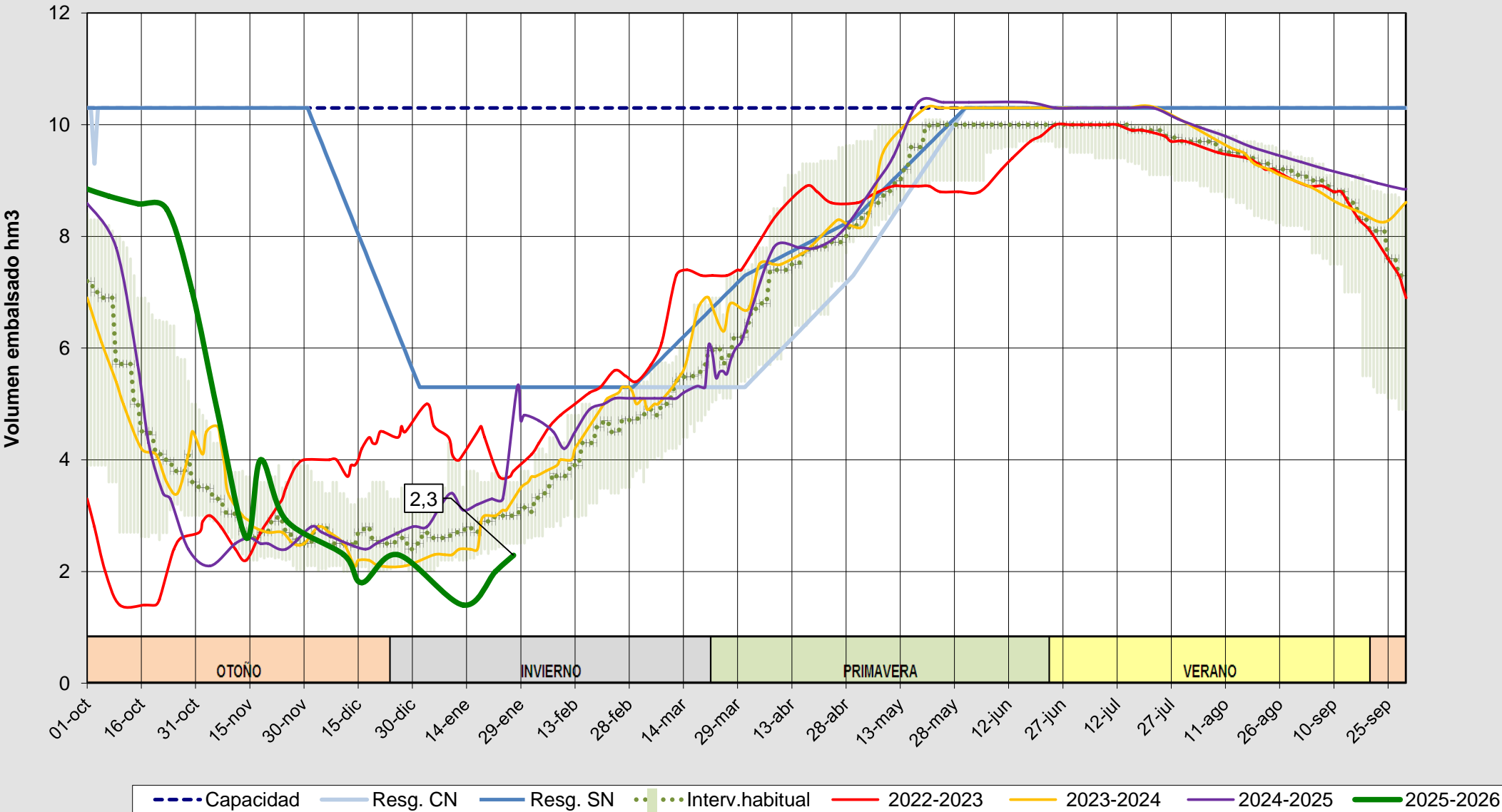
Evolución del volumen almacenado en el embalse de Cervera a fecha 27/01/2026
