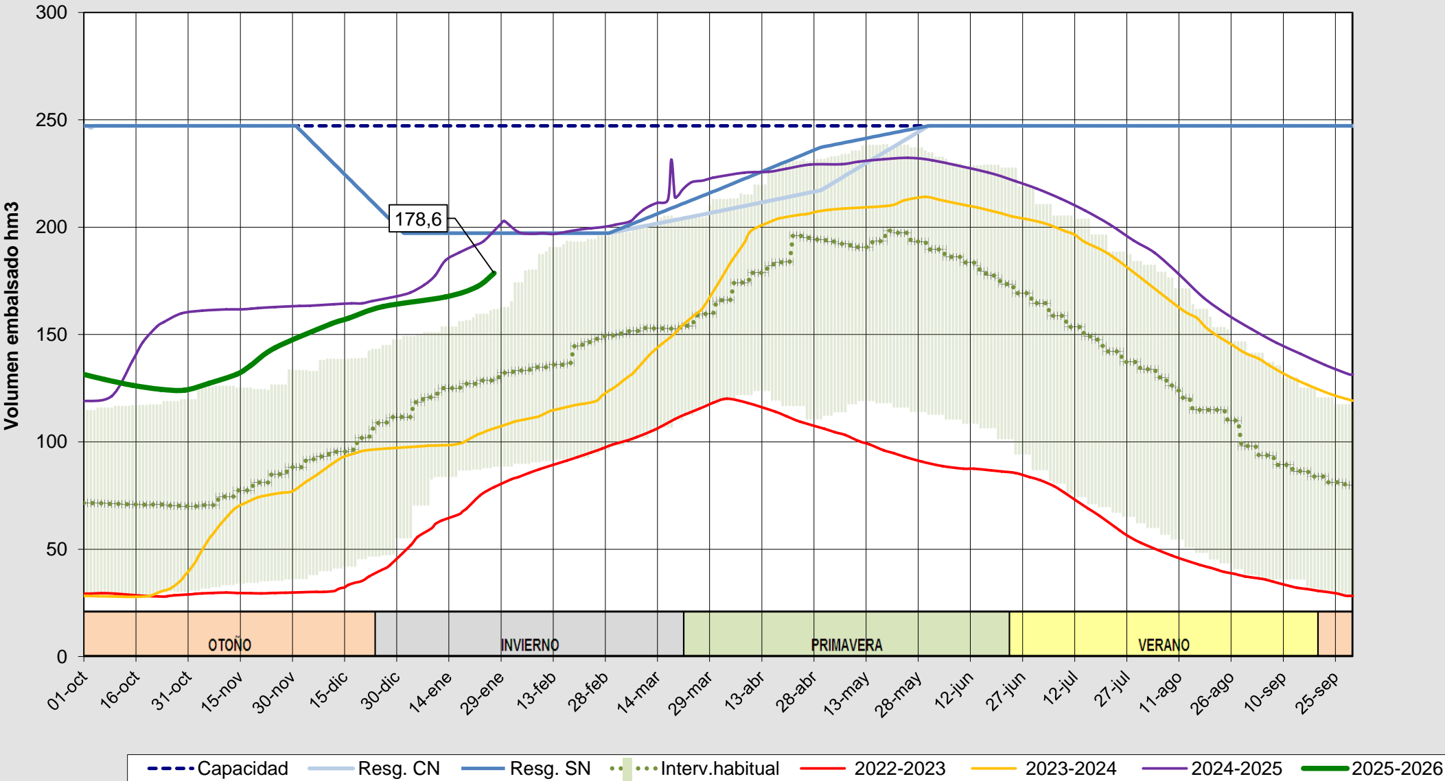
Evolución del volumen almacenado en el embalse de Aguilar a fecha 27/01/2026
