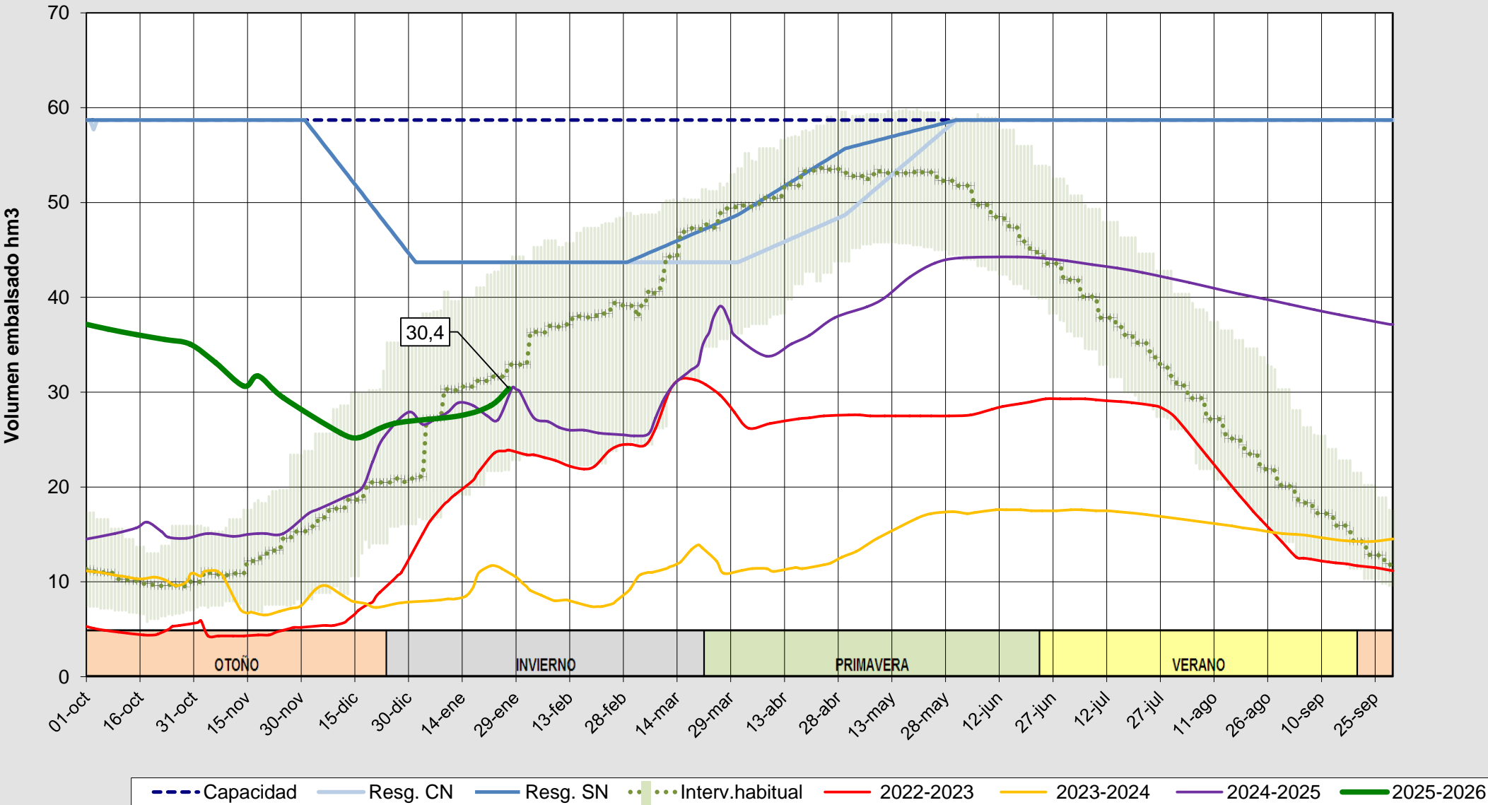
Evolución del volumen almacenado en el embalse de Requejada a fecha 27/01/2026
