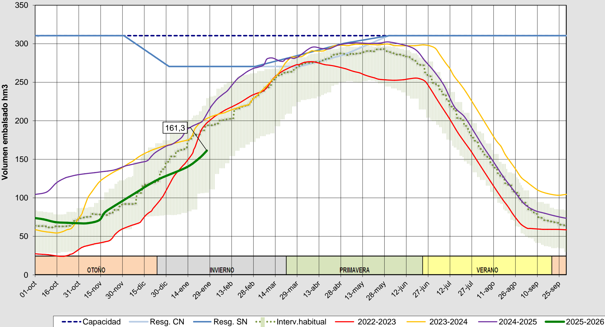
Evolución del volumen almacenado en el embalse de Barrios de Luna a fecha 27/01/2026
