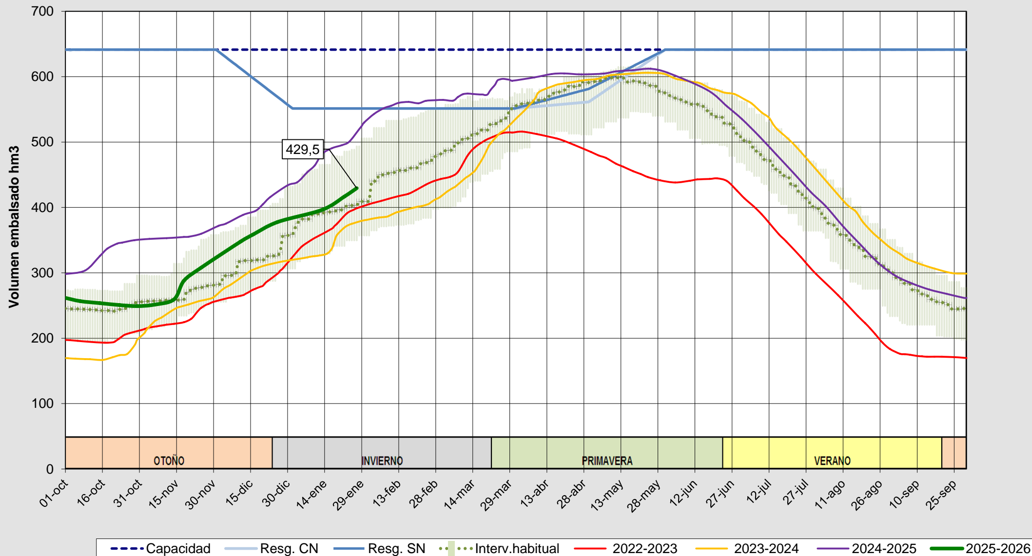
Evolución del volumen almacenado en el embalse de Riaño a fecha 27/01/2026
