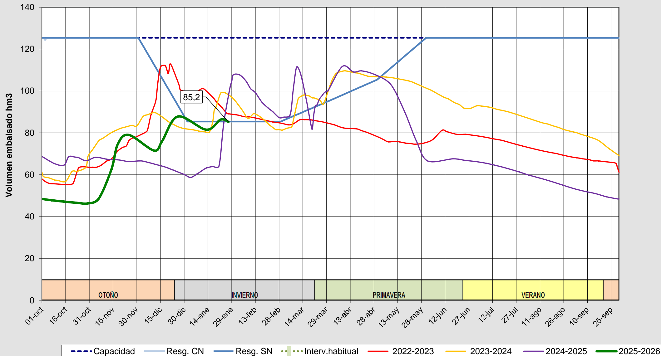
Evolución del volumen almacenado en el sistema del ÁGUEDA a fecha 27/01/2026
