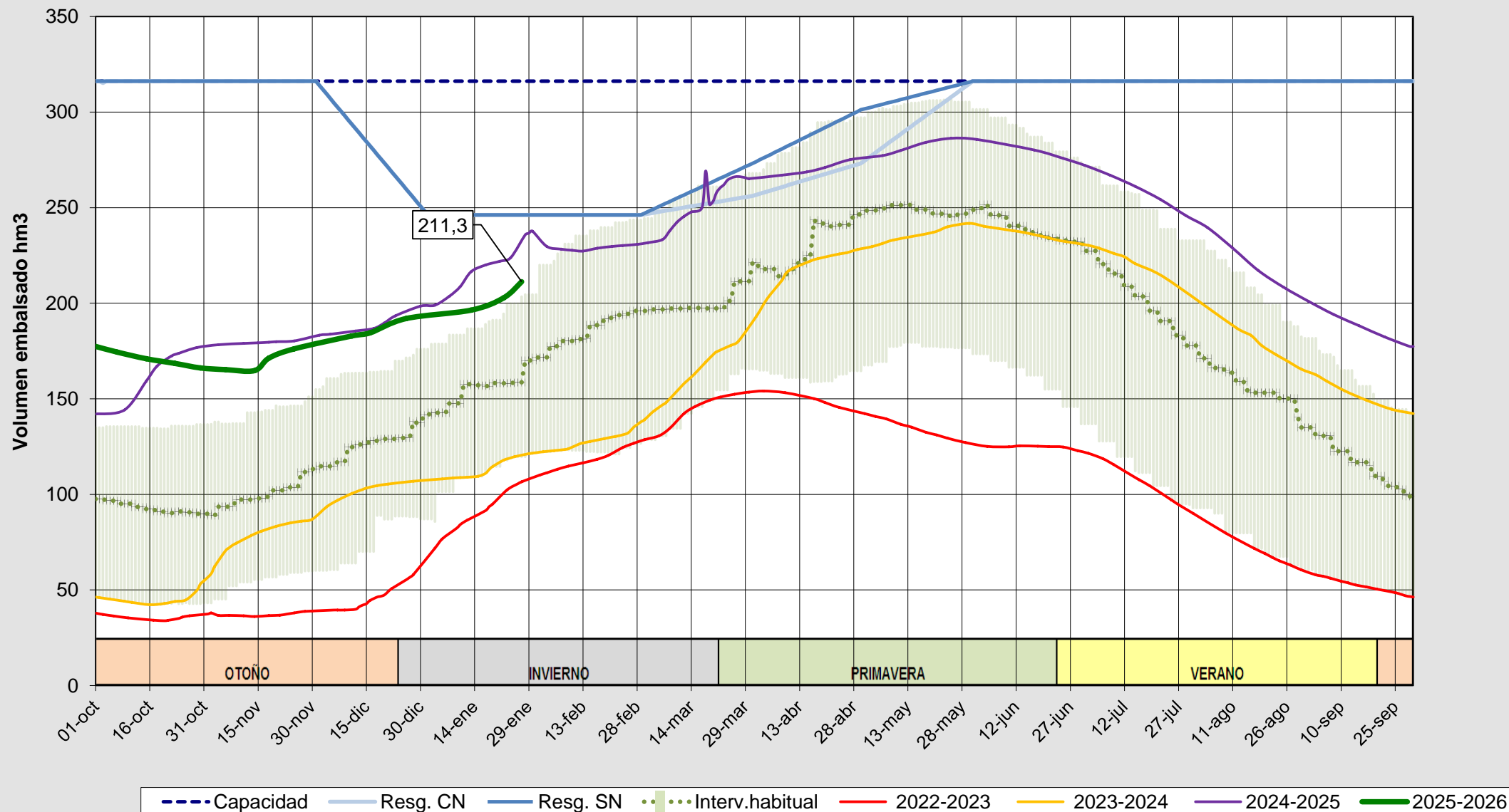
Evolución del volumen almacenado en el sistema del PISUERGA a fecha 27/01/2026
