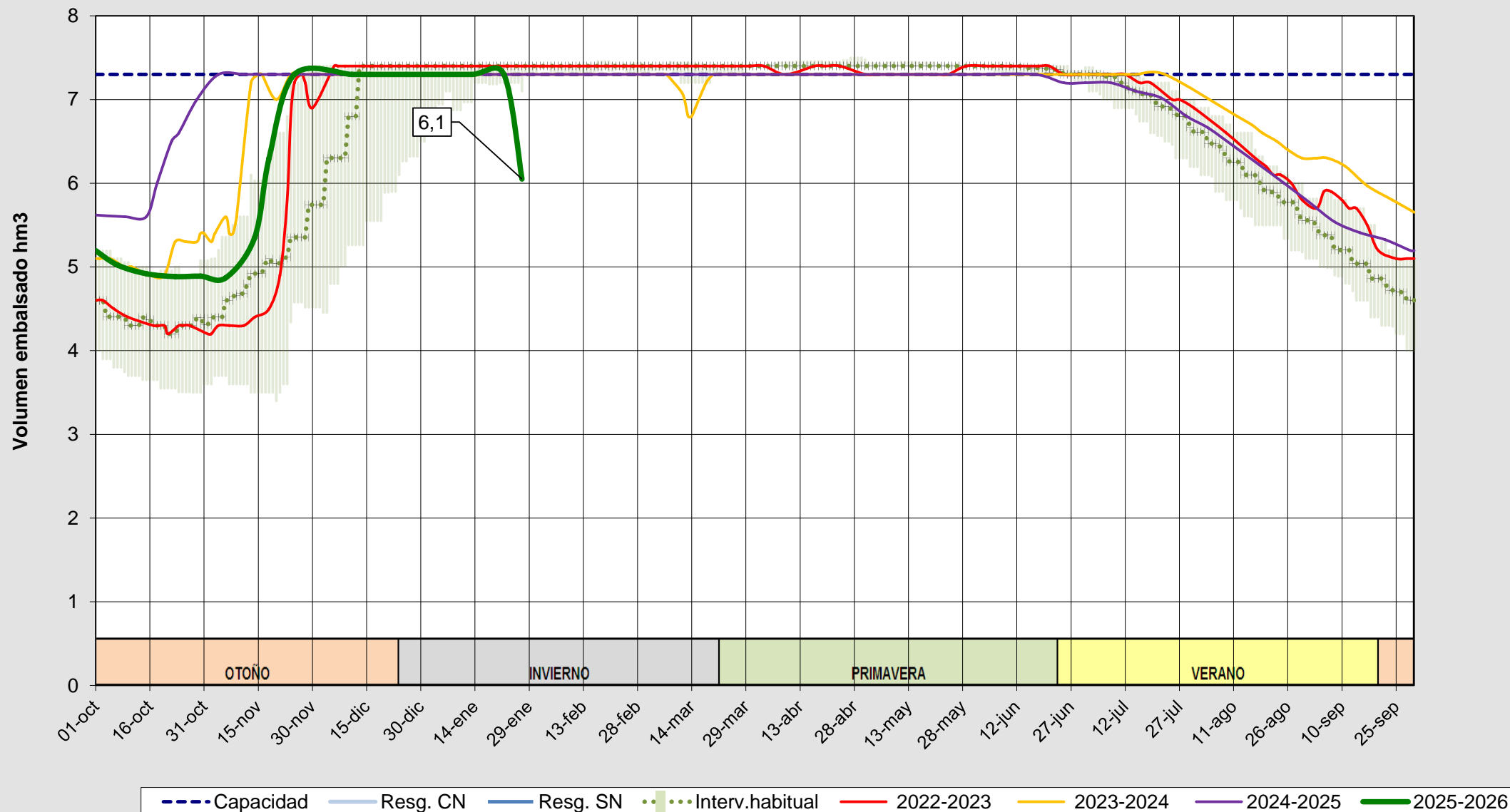
Evolución del volumen almacenado en el embalse de Pontón Alto a fecha 27/01/2026
