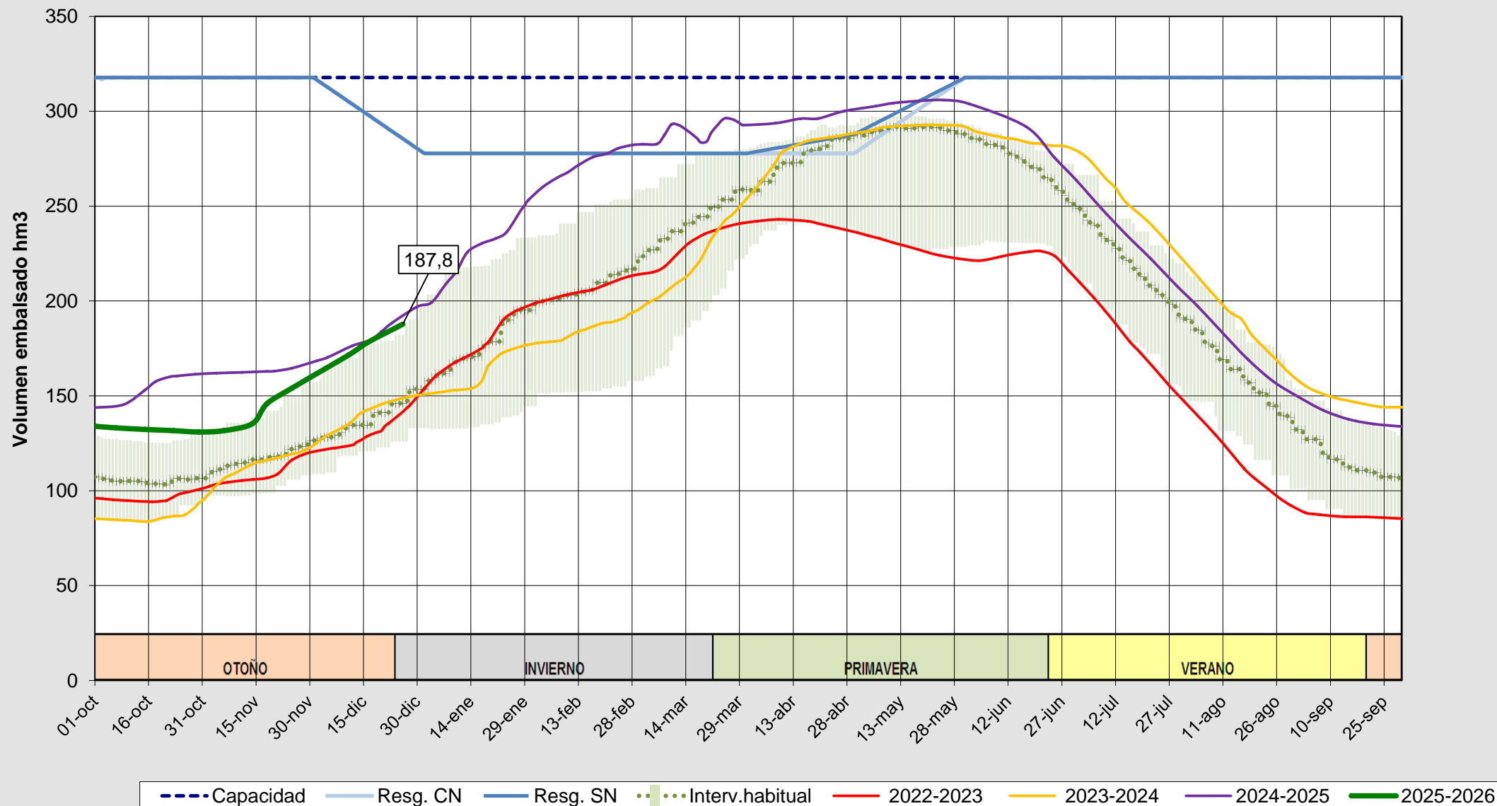
Evolución del volumen almacenado en el embalse de Porma a fecha 26/12/2025
