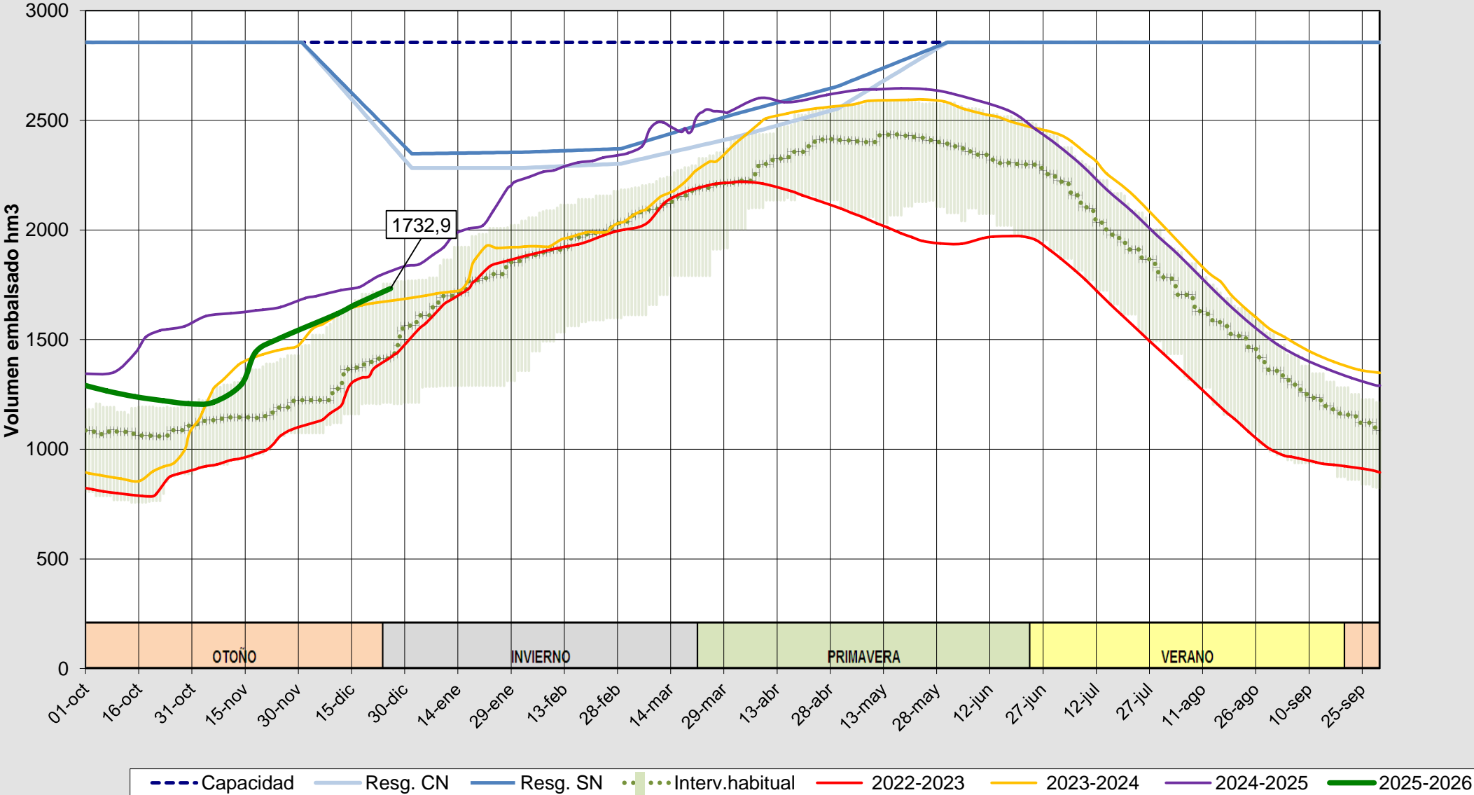
Evolución del volumen almacenado en el sistema del DUERO (ESTADO) a fecha 26/12/2025
