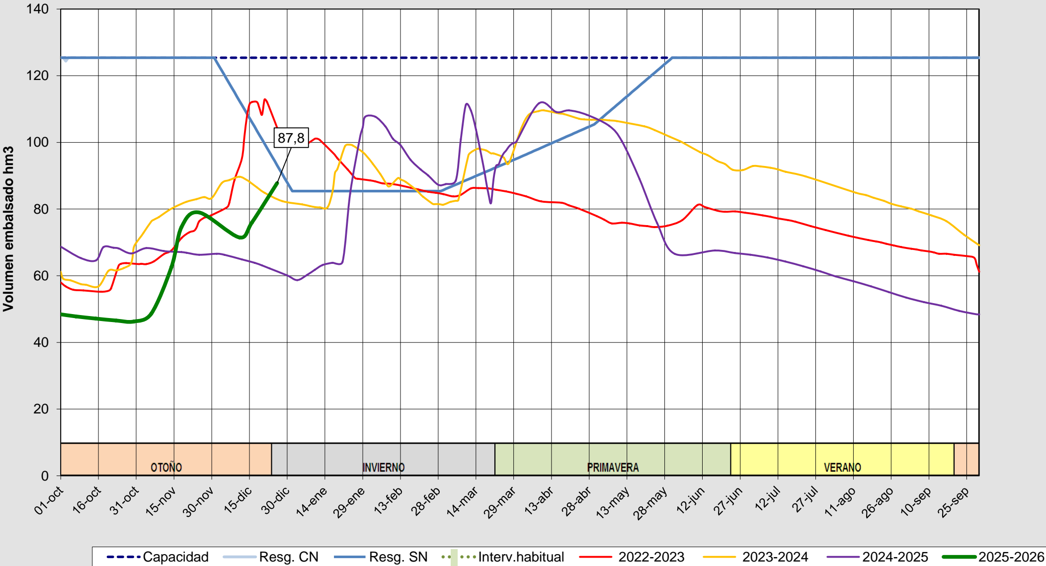
Evolución del volumen almacenado en el sistema del ÁGUEDA a fecha 26/12/2025
