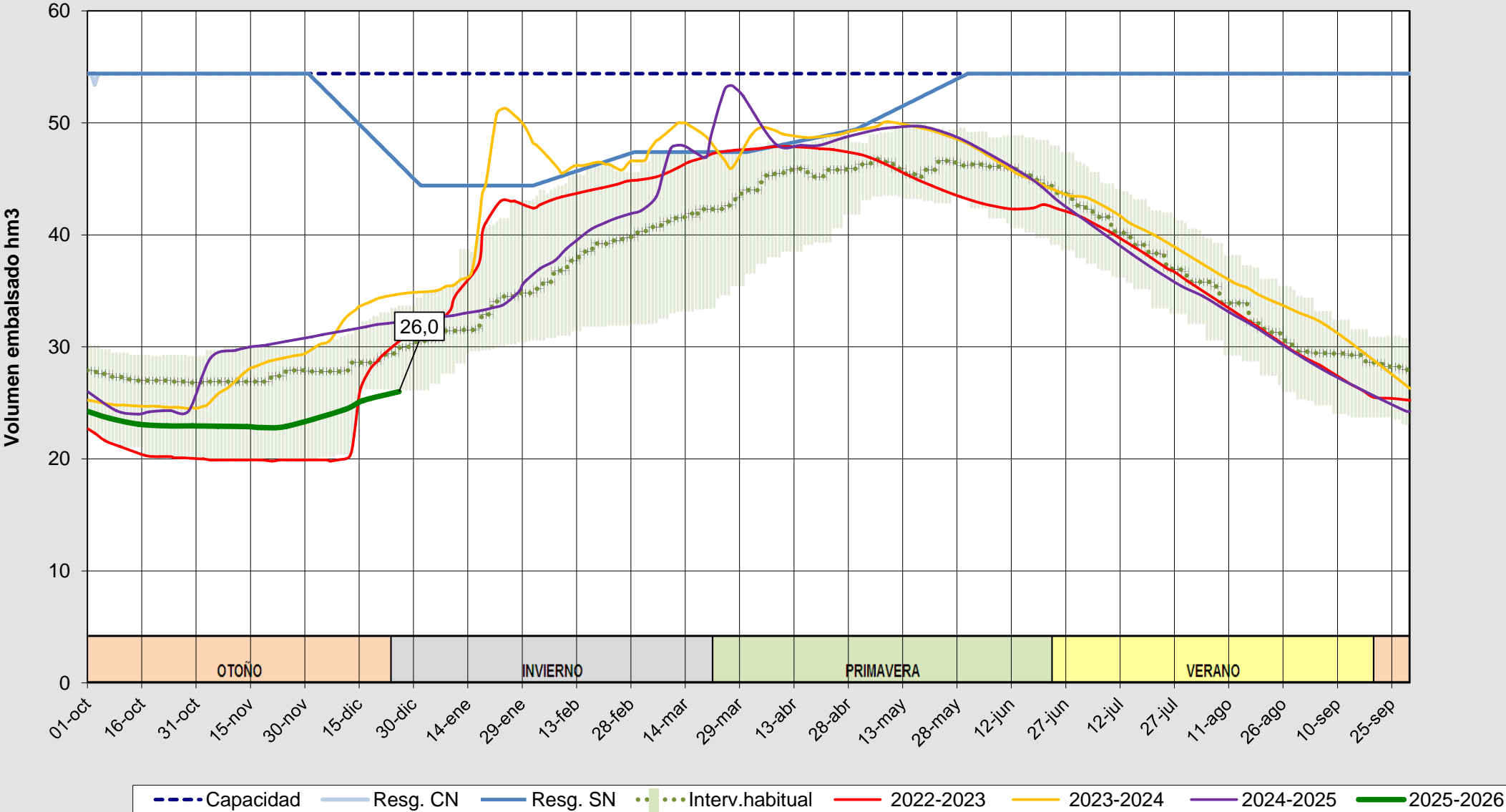
Evolución del volumen almacenado en el embalse de Linares del Arroyo a fecha 26/12/2025
