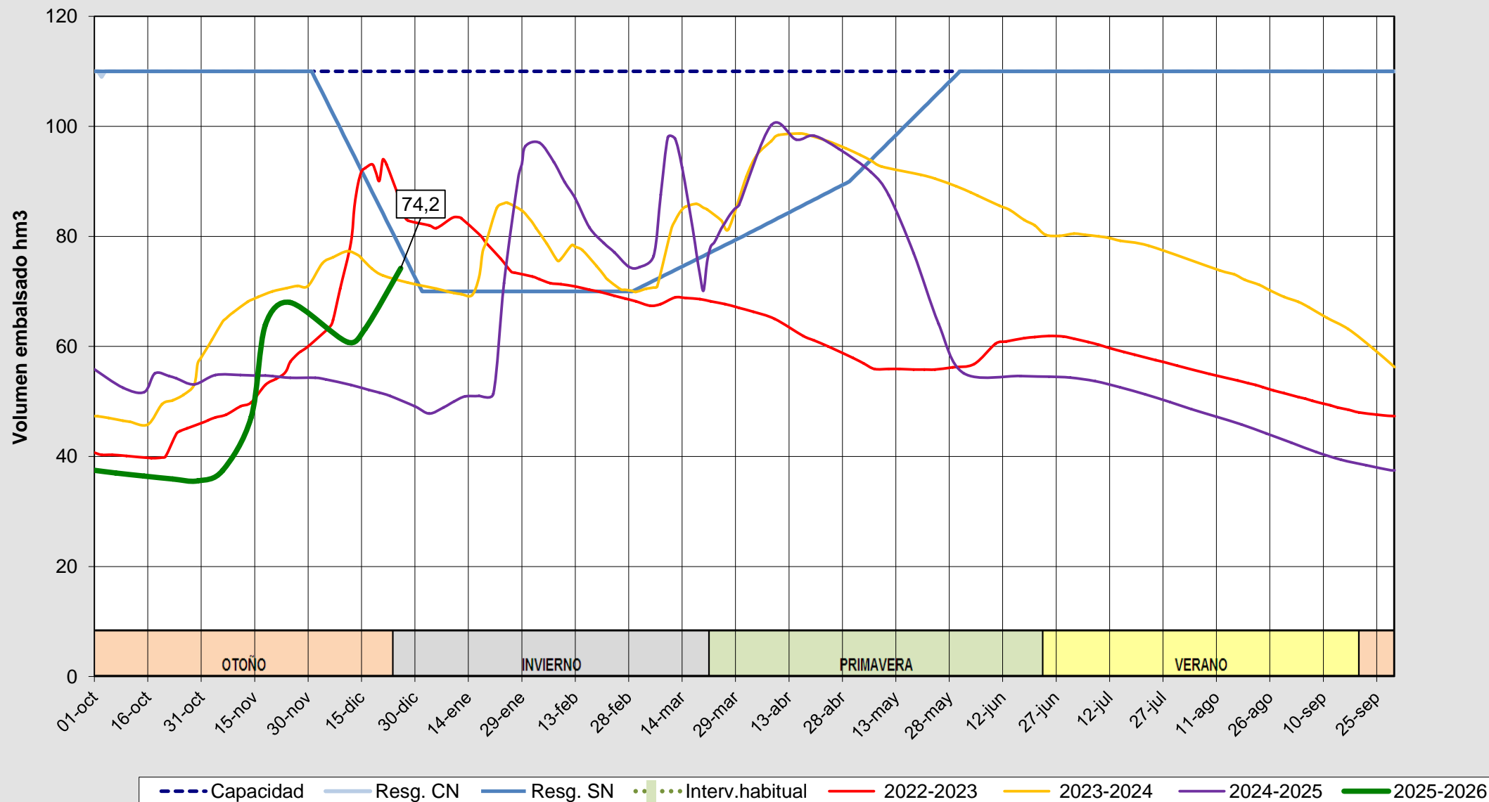
Evolución del volumen almacenado en el embalse de Irueña a fecha 26/12/2025
