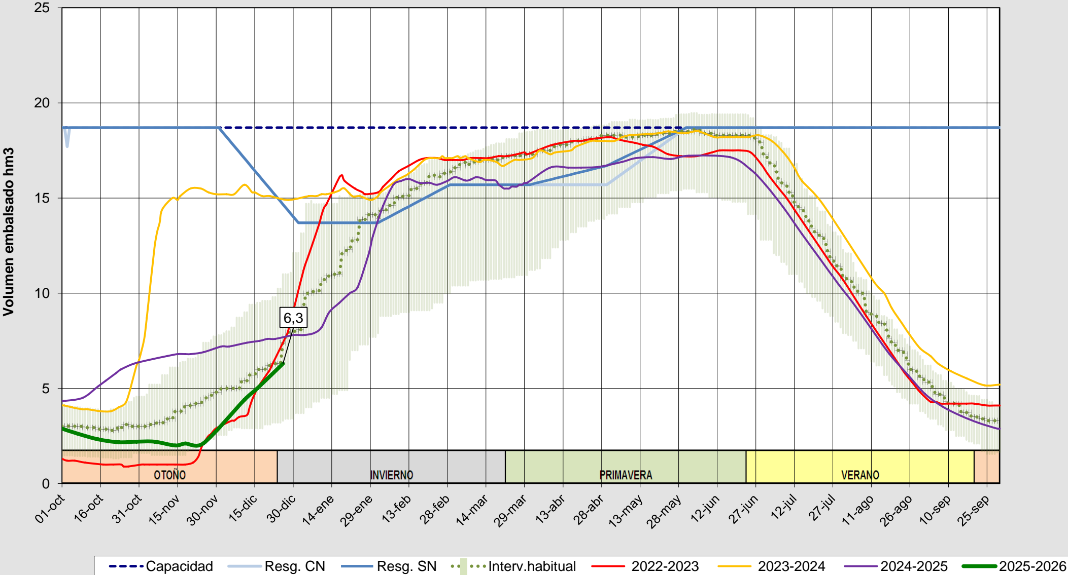
Evolución del volumen almacenado en el embalse de Villameca a fecha 26/12/2025
