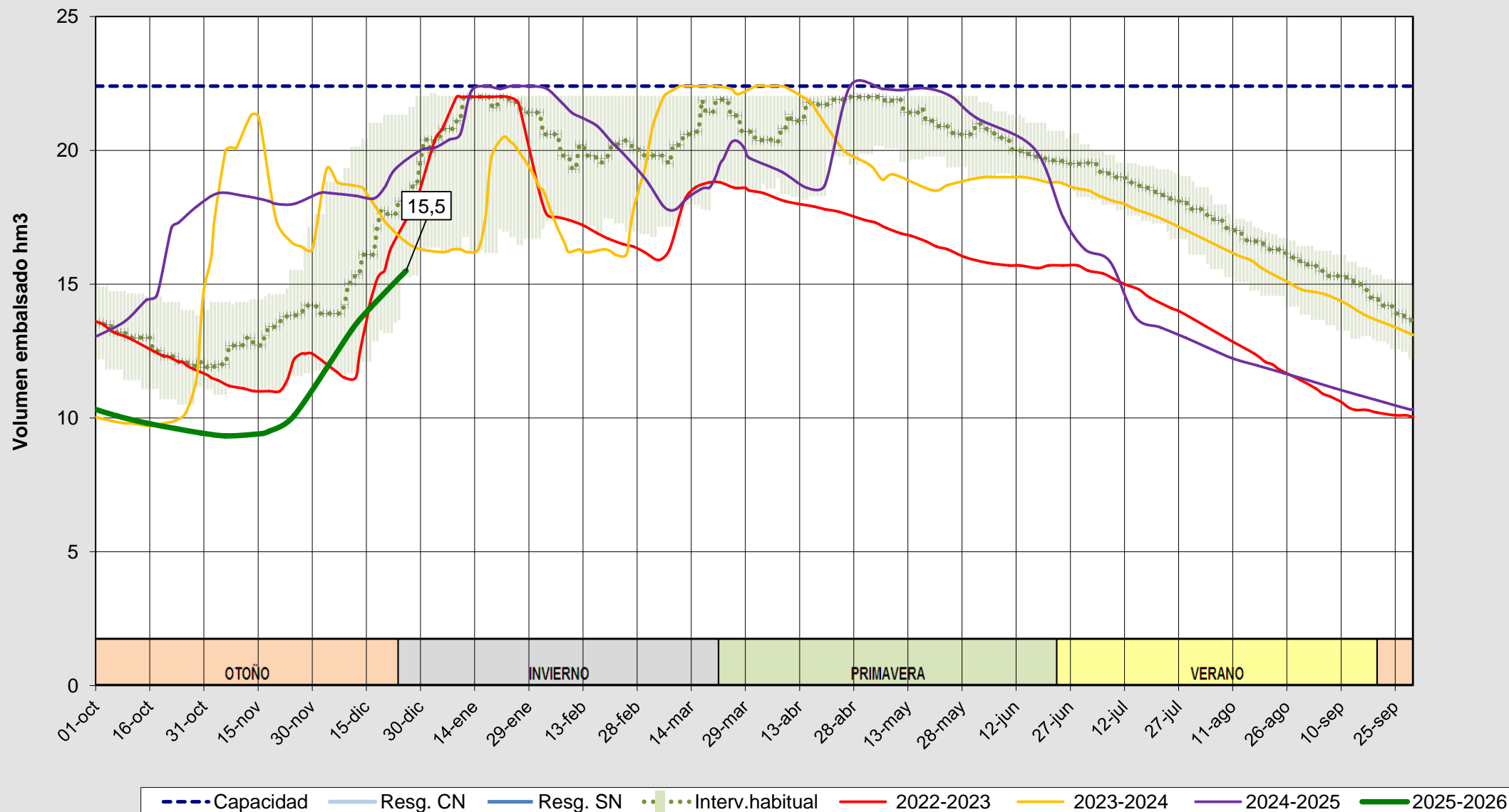
Evolución del volumen almacenado en el embalse de Arlanzón a fecha 26/12/2025
