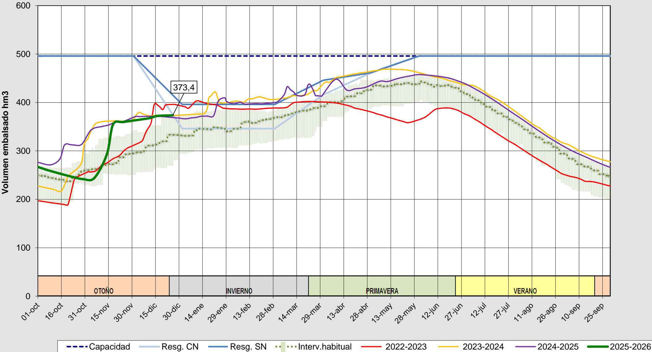
Evolución del volumen almacenado en el embalse de Santa Teresa a fecha 26/12/2025
