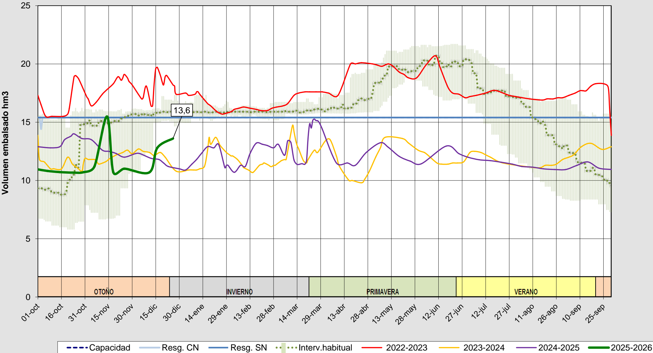
Evolución del volumen almacenado en el embalse de Águeda a fecha 26/12/2025
