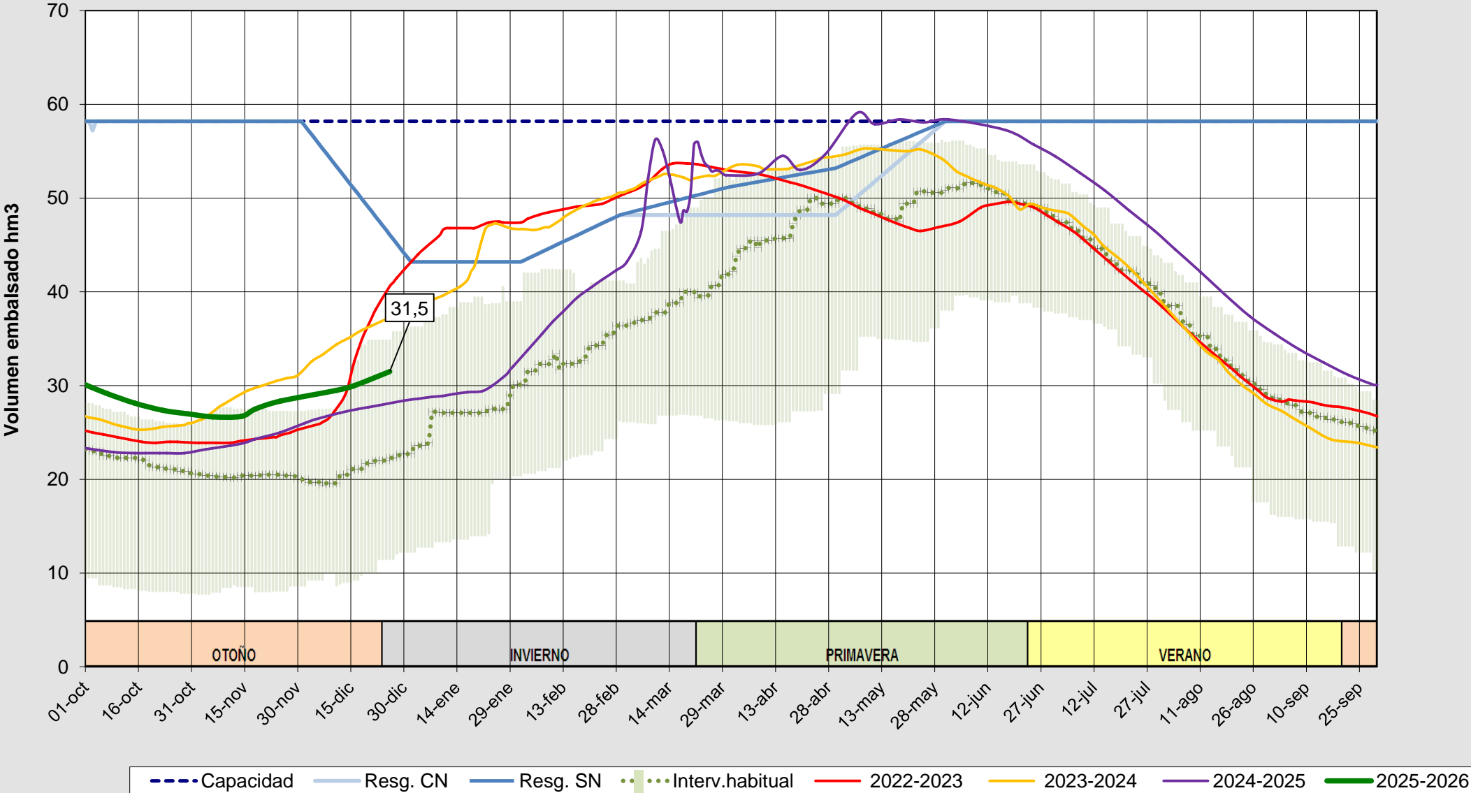
Evolución del volumen almacenado en el embalse de Las Cogotas a fecha 26/12/2025
