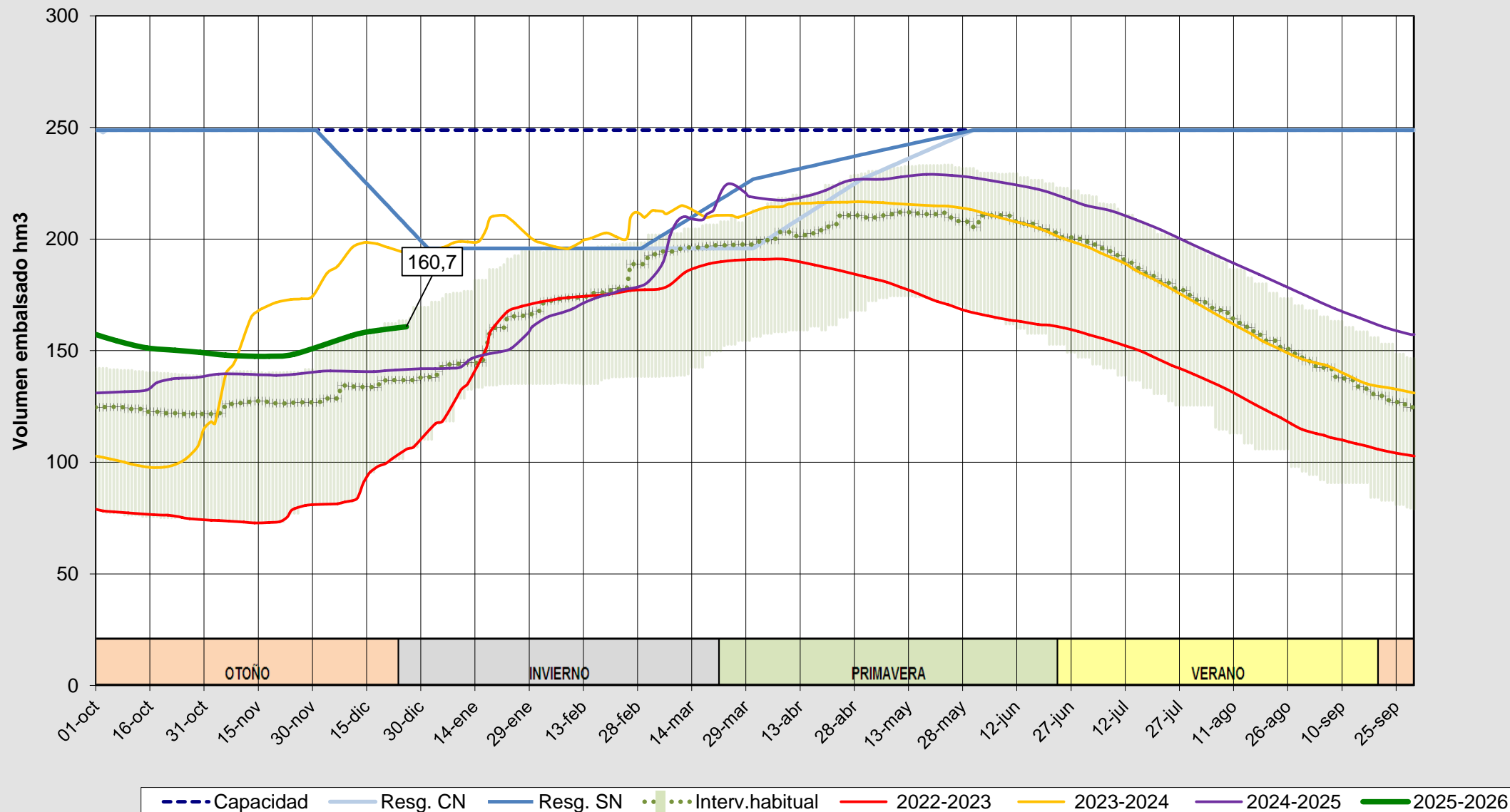
Evolución del volumen almacenado en el embalse de Cuerda del Pozo a fecha 26/12/2025
