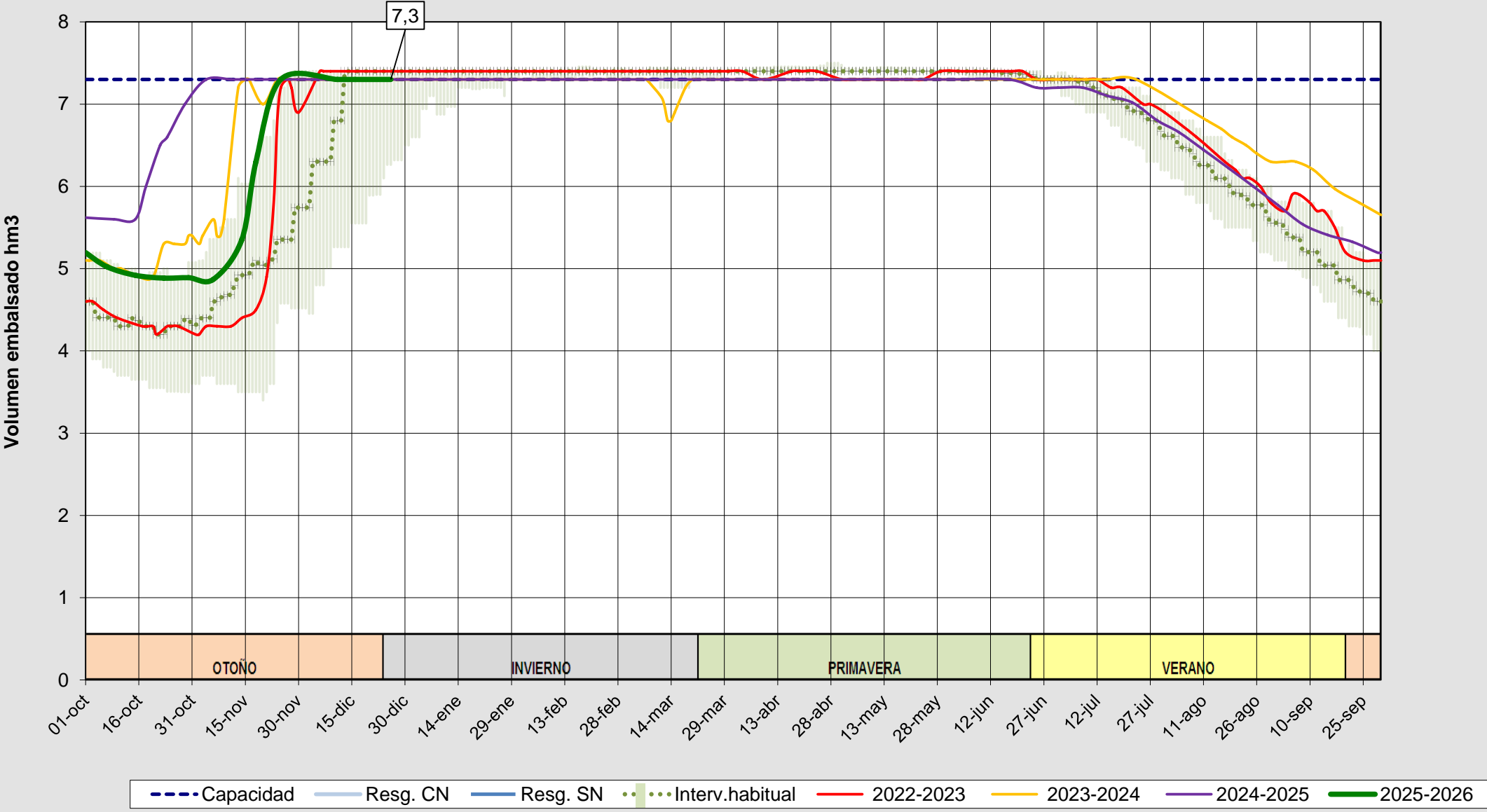
Evolución del volumen almacenado en el embalse de Pontón Alto a fecha 26/12/2025
