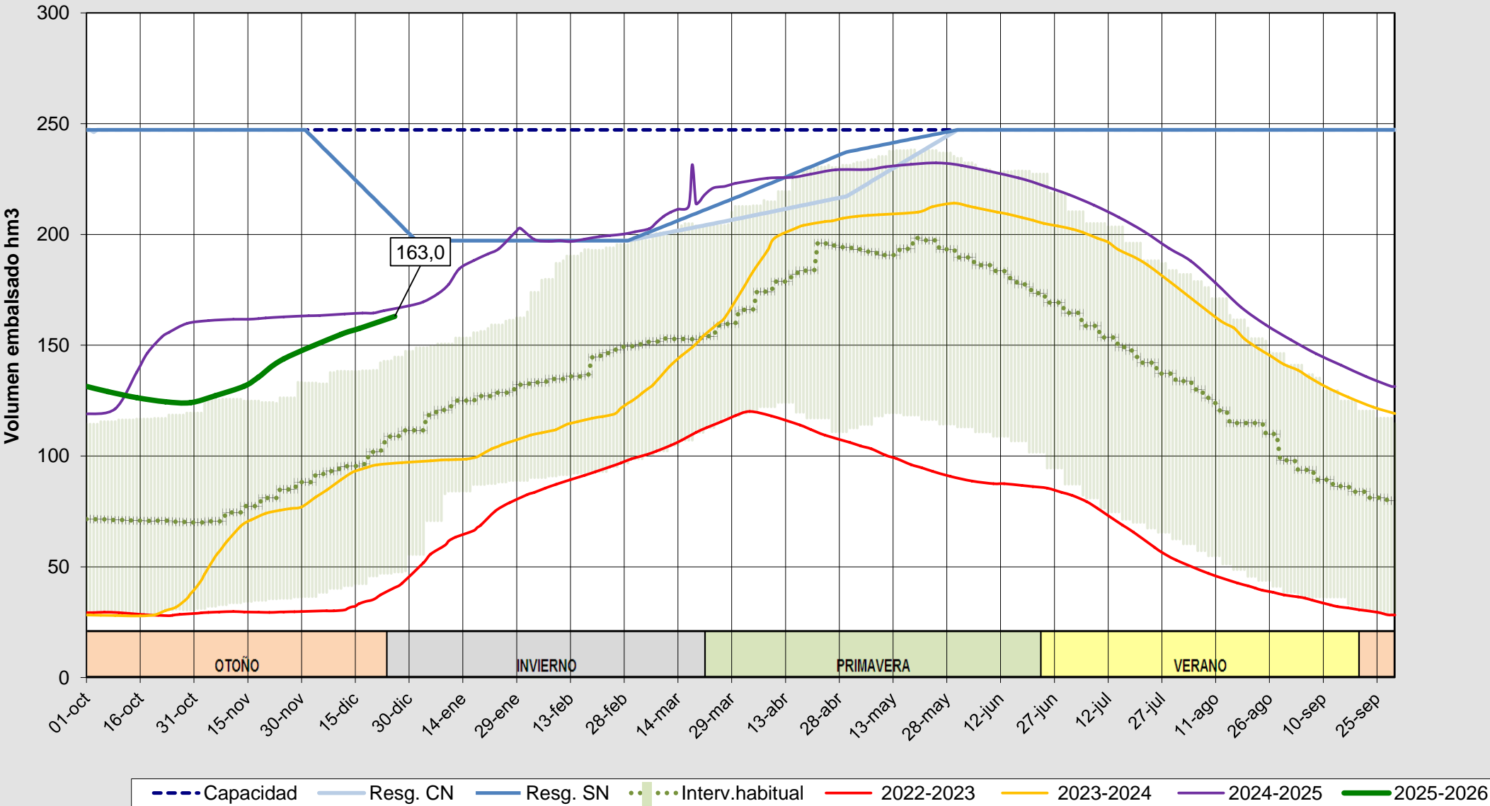
Evolución del volumen almacenado en el embalse de Aguilar a fecha 26/12/2025
