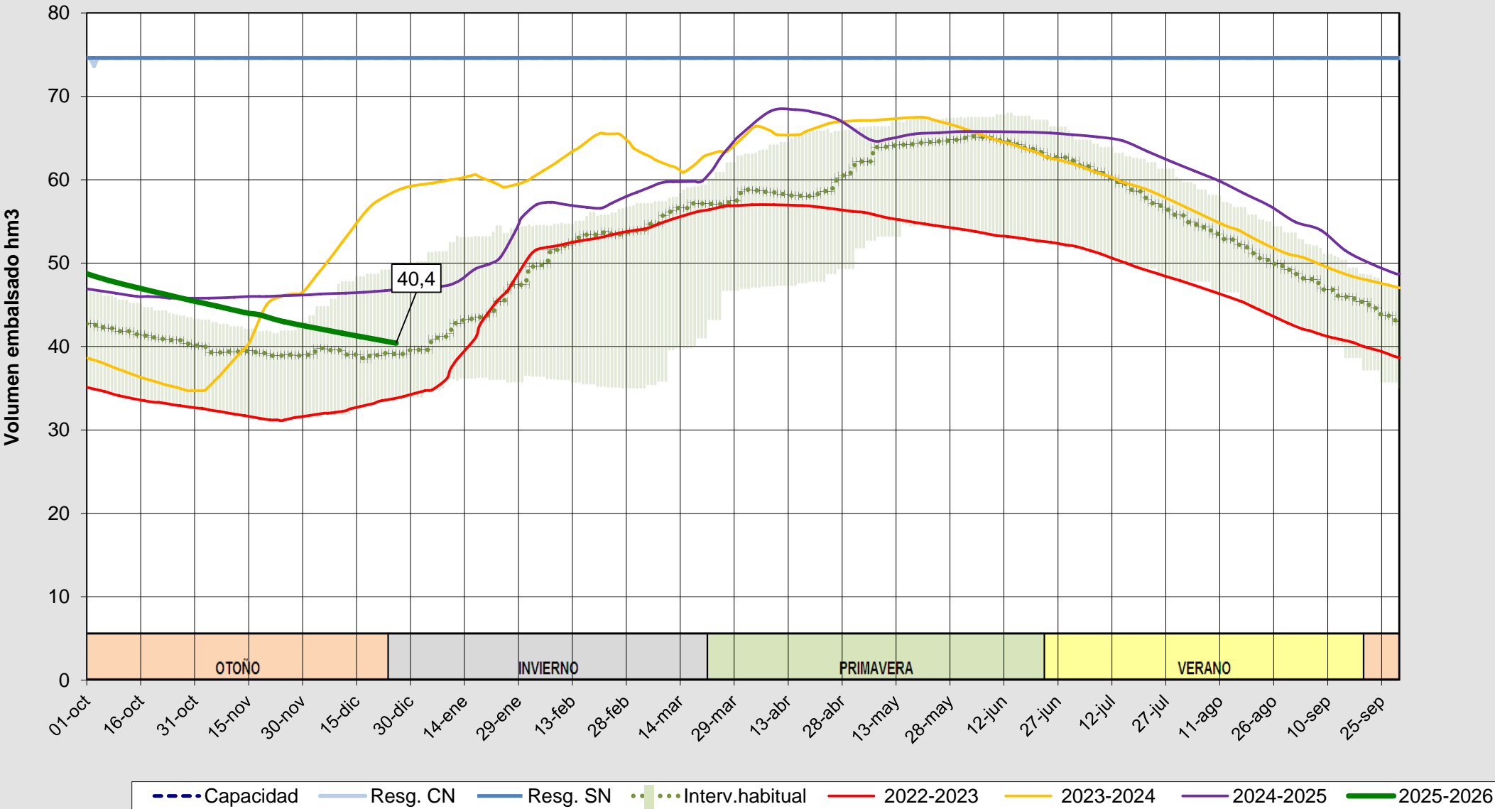
Evolución del volumen almacenado en el embalse de Úzquiza a fecha 26/12/2025
