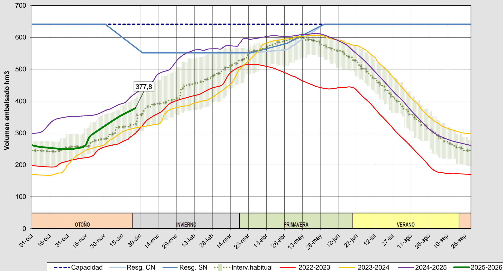
Evolución del volumen almacenado en el embalse de Riaño a fecha 26/12/2025
