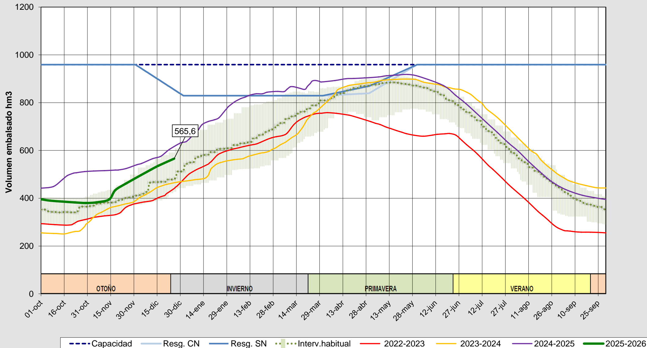
Evolución del volumen almacenado en el sistema del PORMA-ESLA a fecha 26/12/2025
