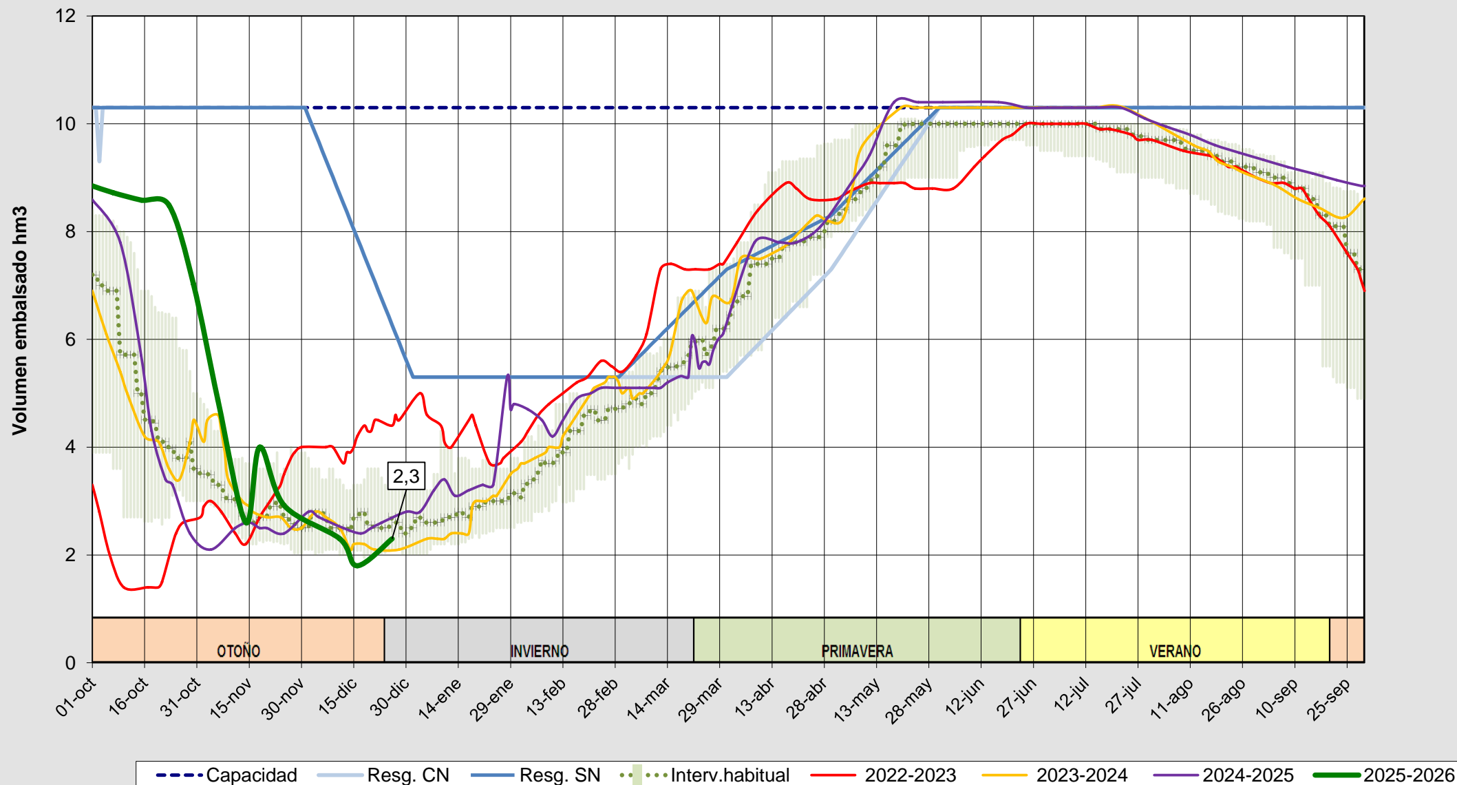
Evolución del volumen almacenado en el embalse de Cervera a fecha 26/12/2025
