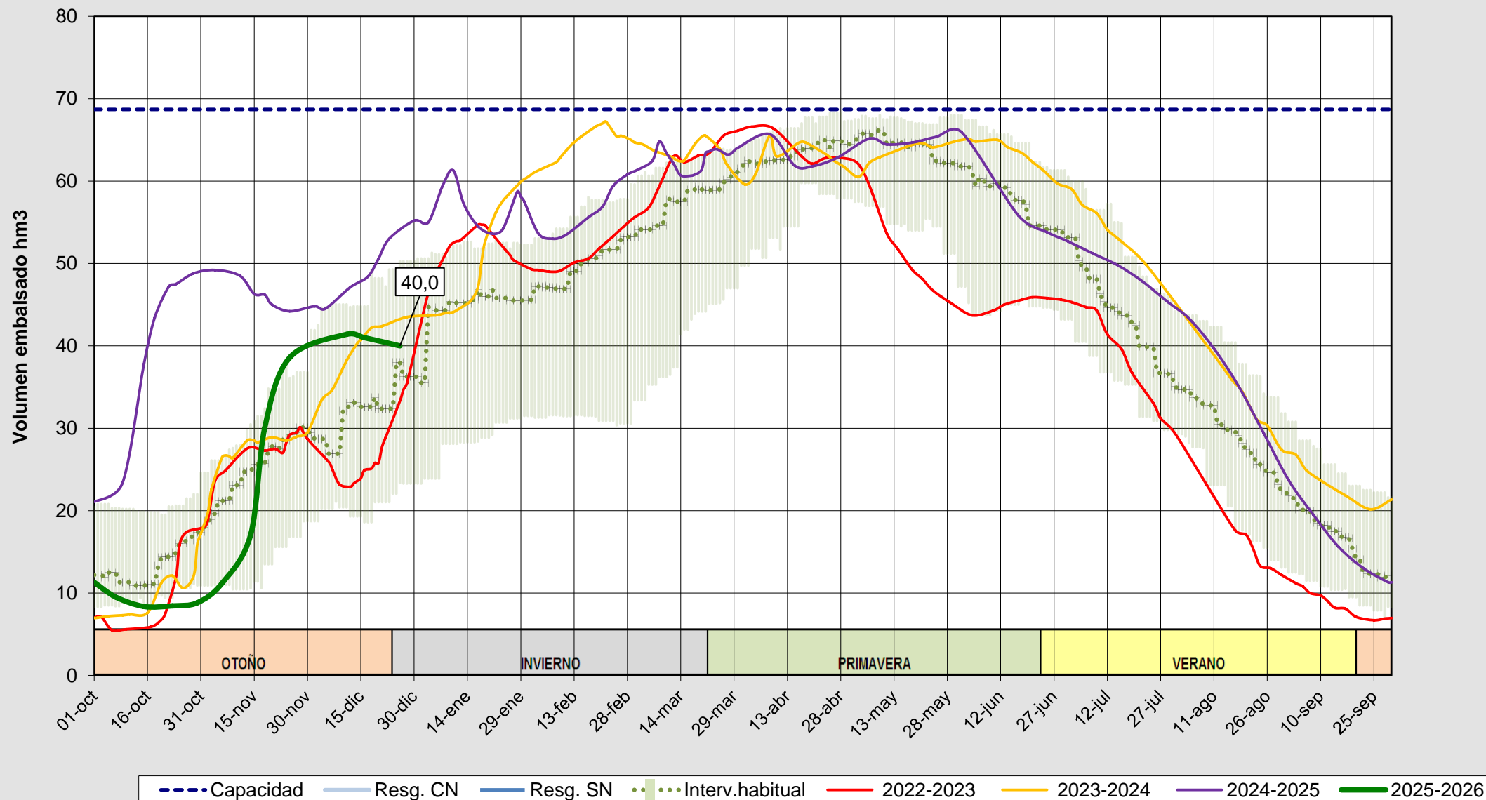
Evolución del volumen almacenado en el embalse de Camporredondo a fecha 26/12/2025
