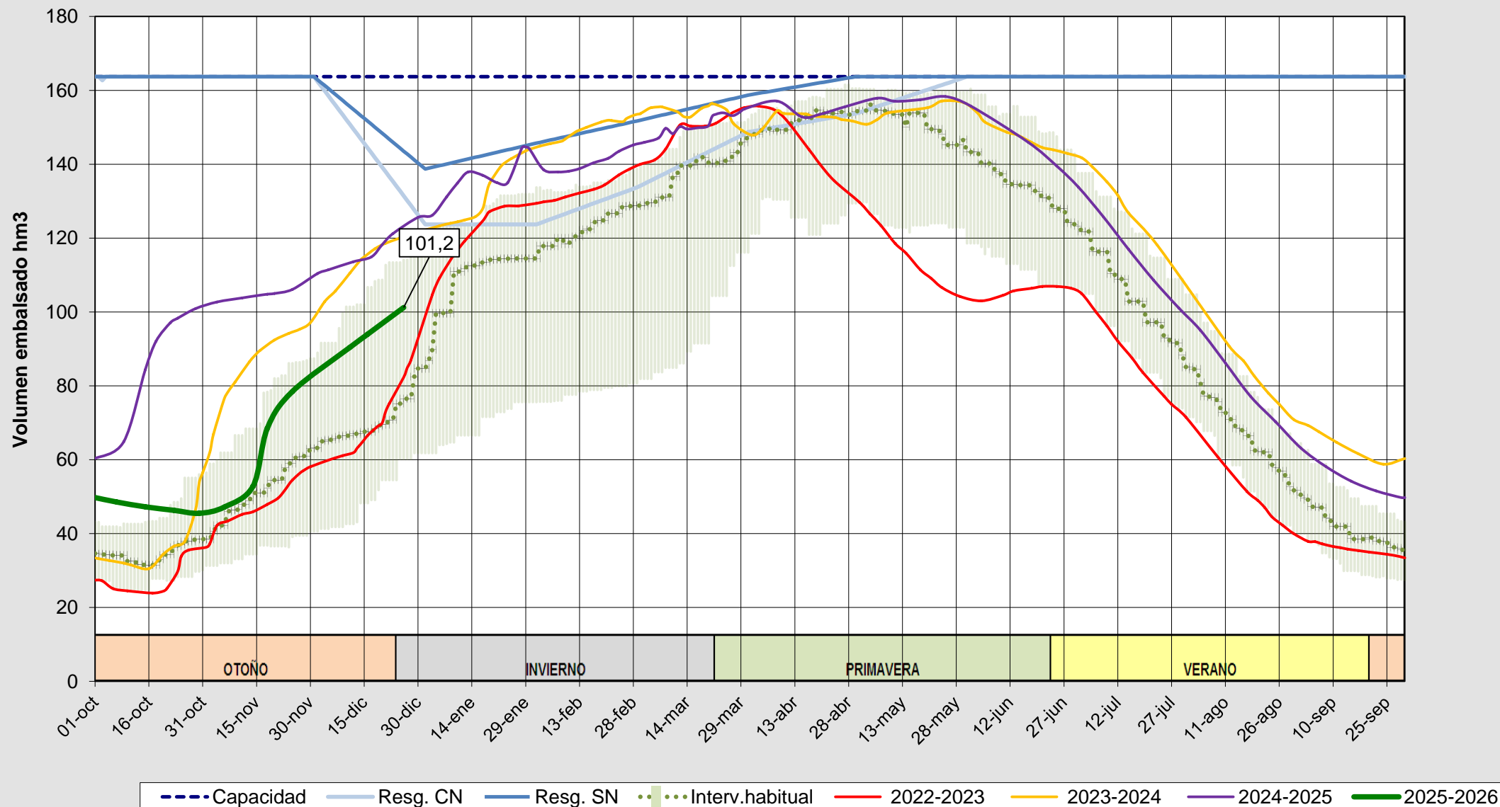
Evolución del volumen almacenado en el sistema del CARRIÓN a fecha 26/12/2025
