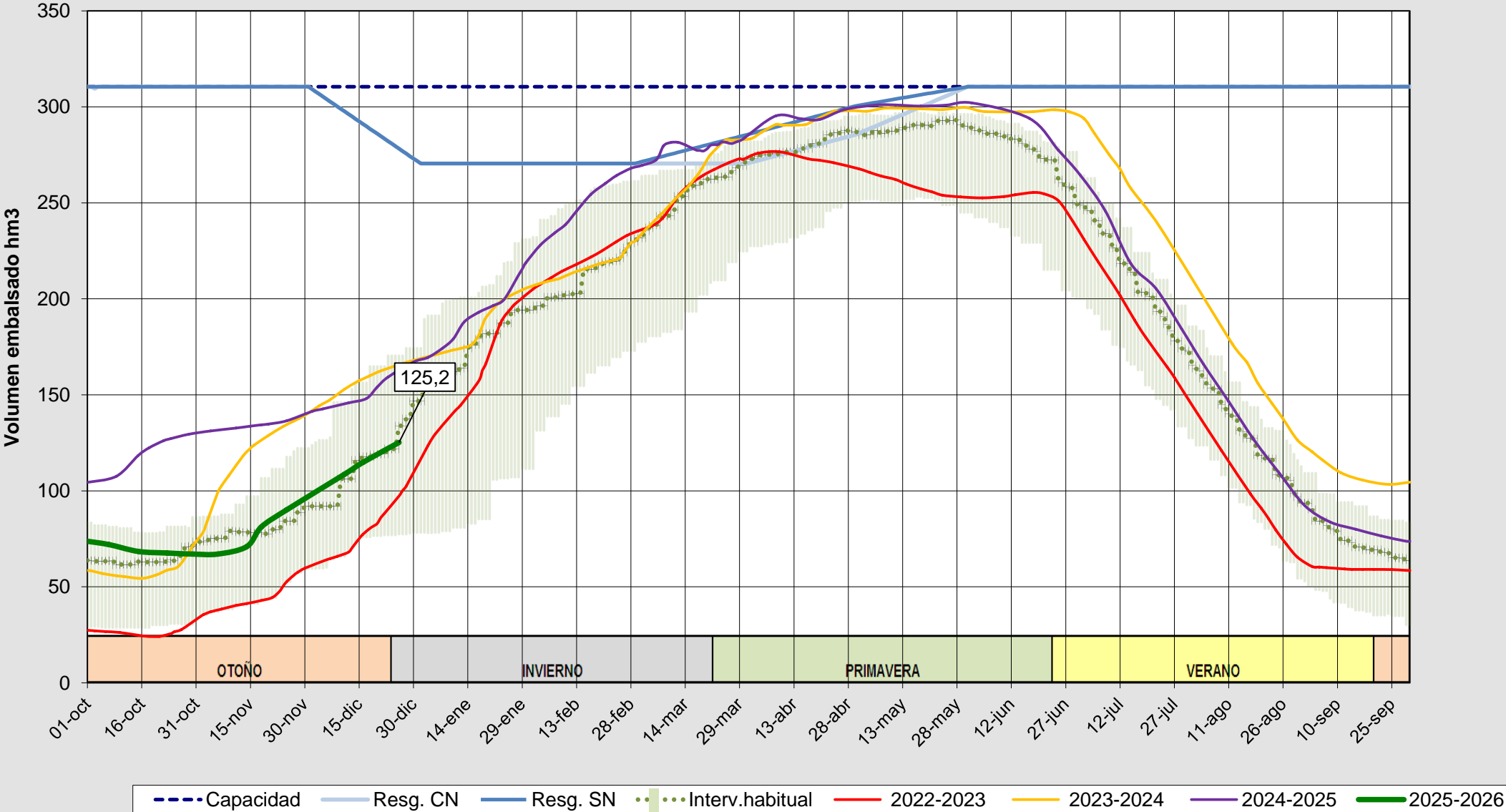
Evolución del volumen almacenado en el embalse de Barrios de Luna a fecha 26/12/2025
