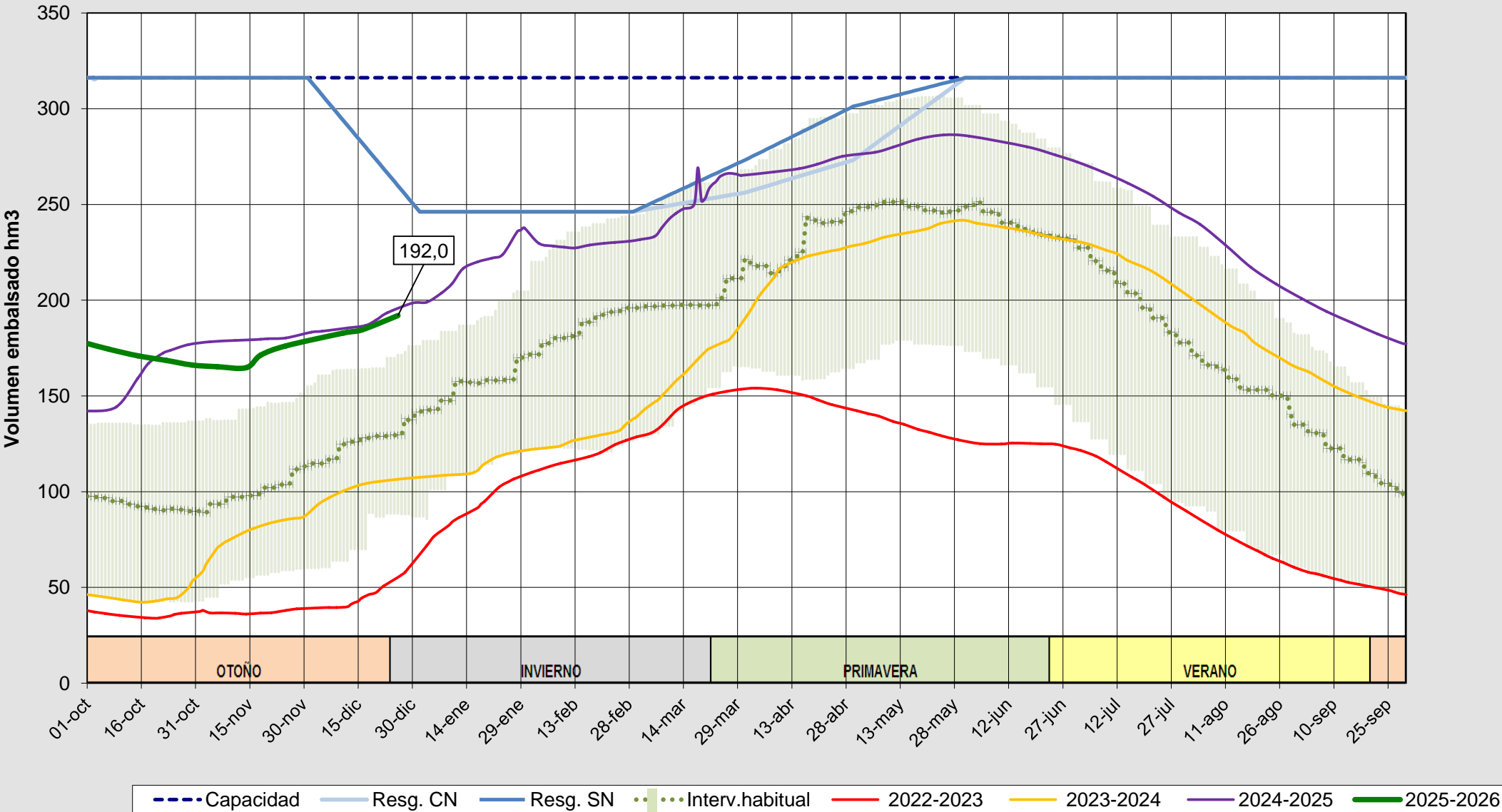
Evolución del volumen almacenado en el sistema del PISUERGA a fecha 26/12/2025
