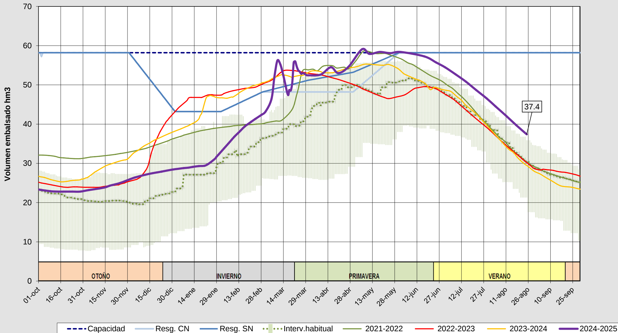
Evolución del volumen almacenado en el embalse de Las Cogotas a fecha 26/08/2025
