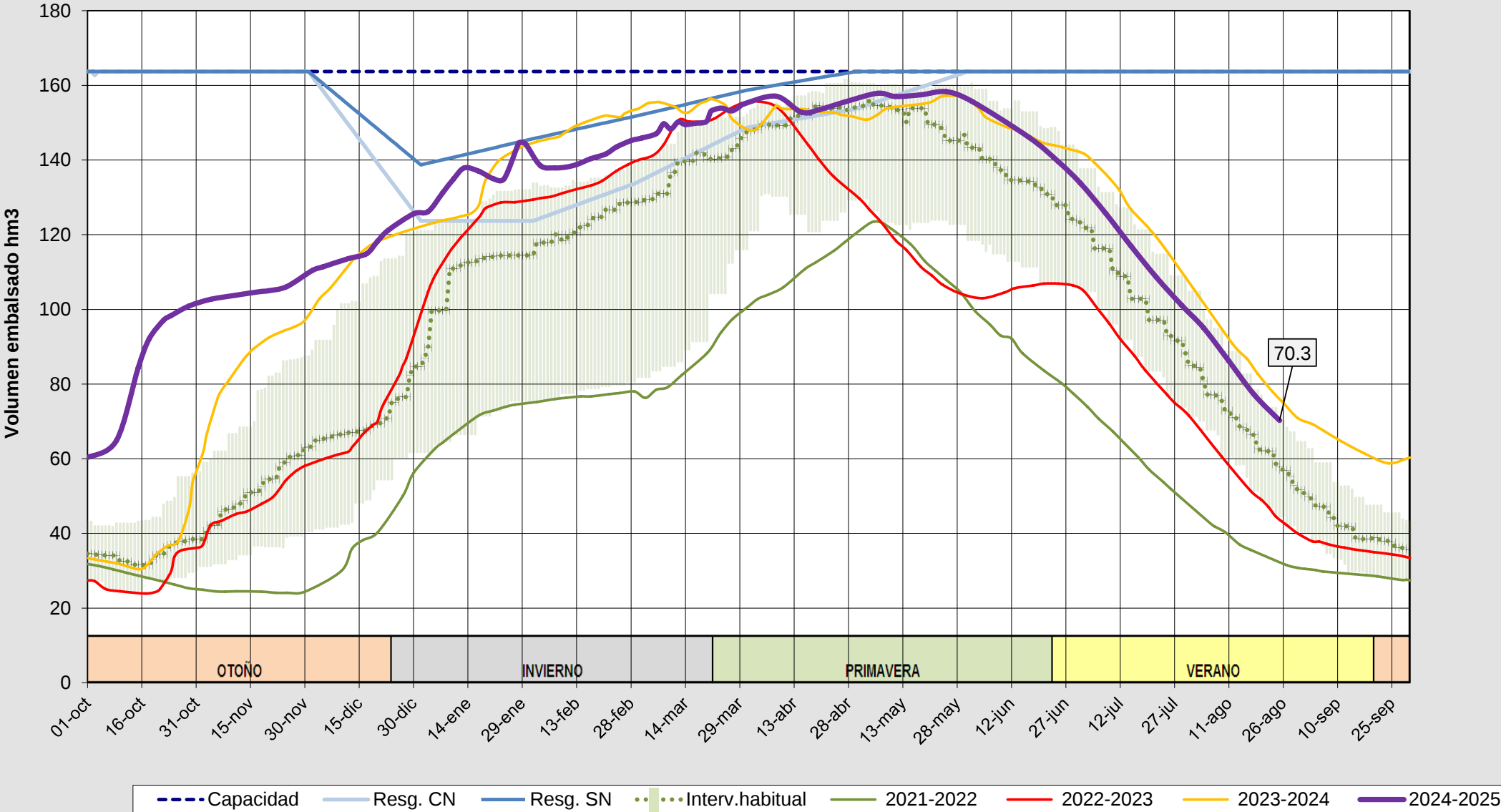
Evolución del volumen almacenado en el sistema del CARRIÓN a fecha 26/08/2025
