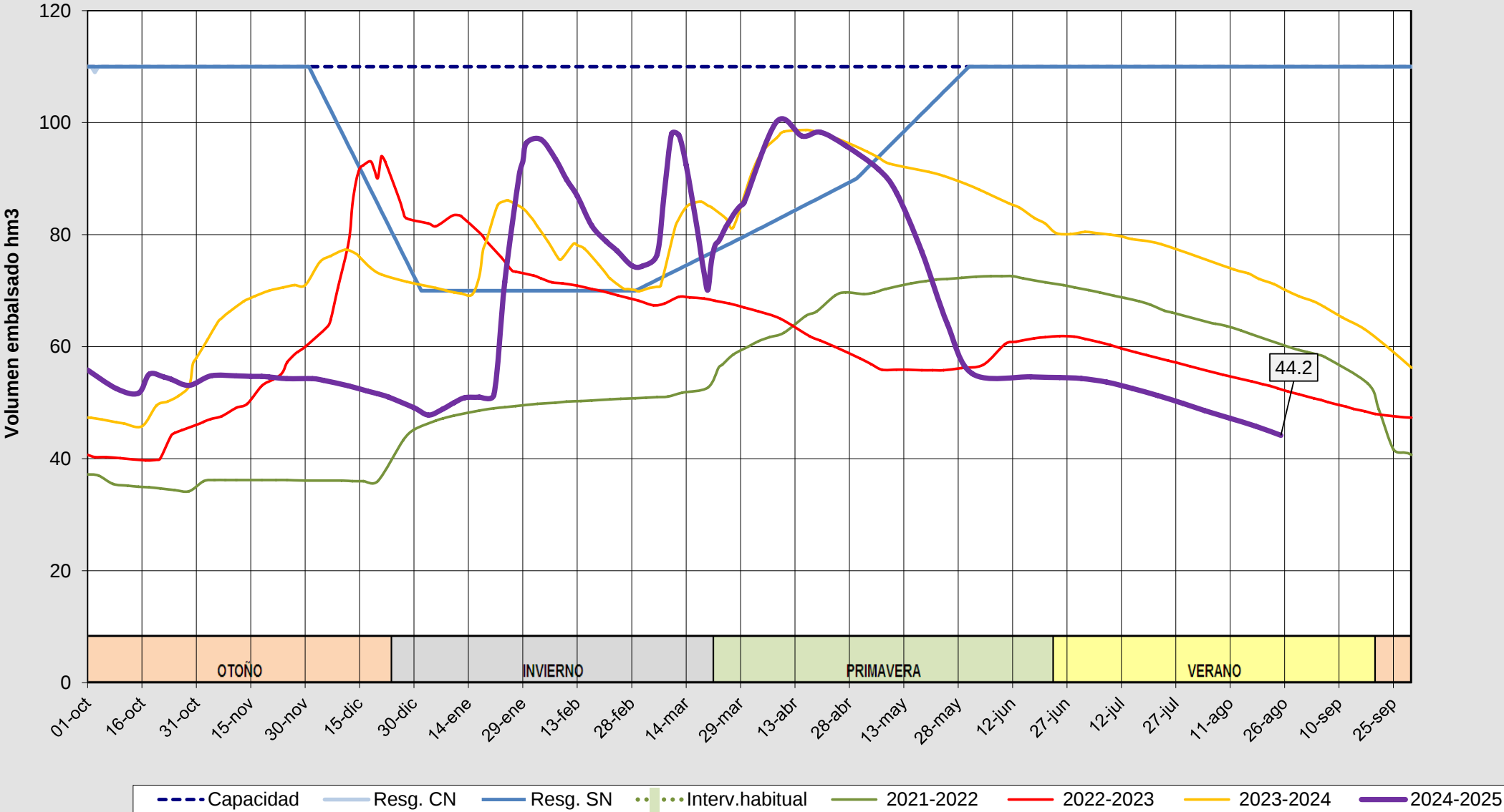
Evolución del volumen almacenado en el embalse de Irueña a fecha 26/08/2025
