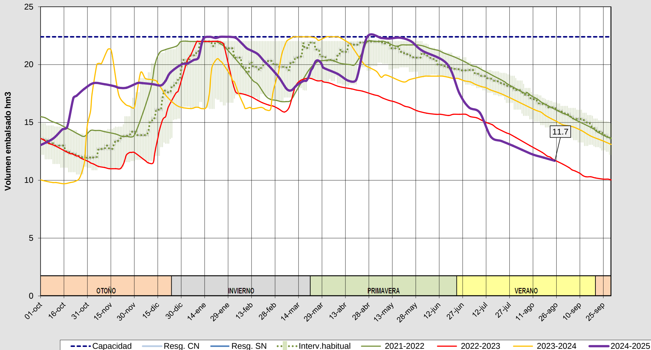
Evolución del volumen almacenado en el embalse de Arlanzón a fecha 26/08/2025
