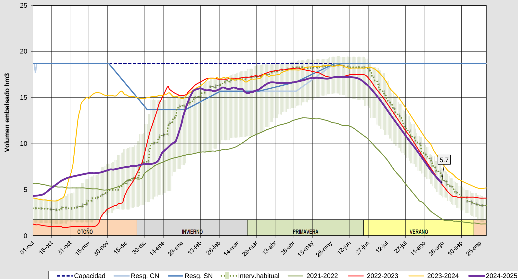
Evolución del volumen almacenado en el embalse de Villameca a fecha 26/08/2025
