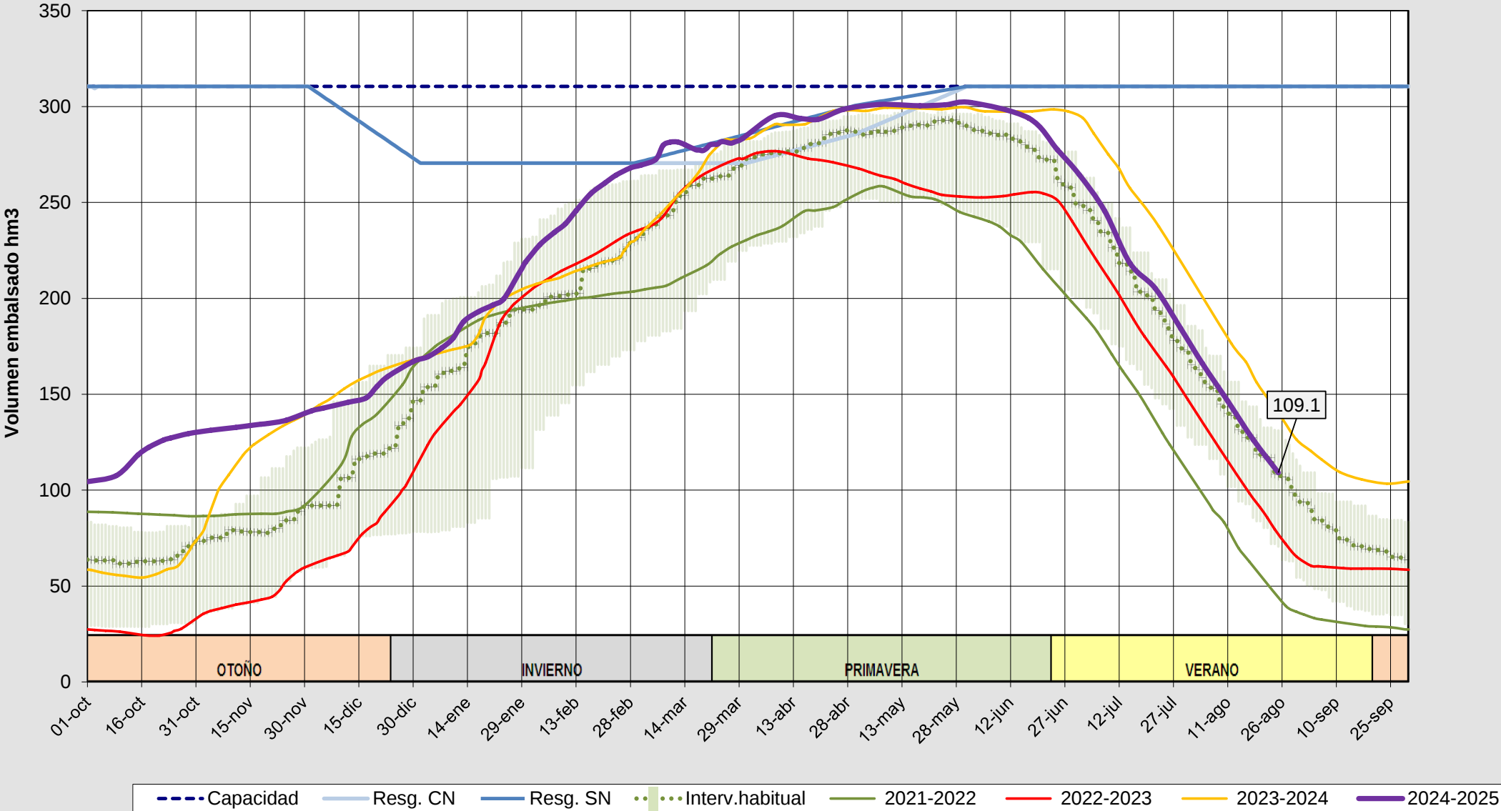
Evolución del volumen almacenado en el embalse de Barrios de Luna a fecha 26/08/2025
