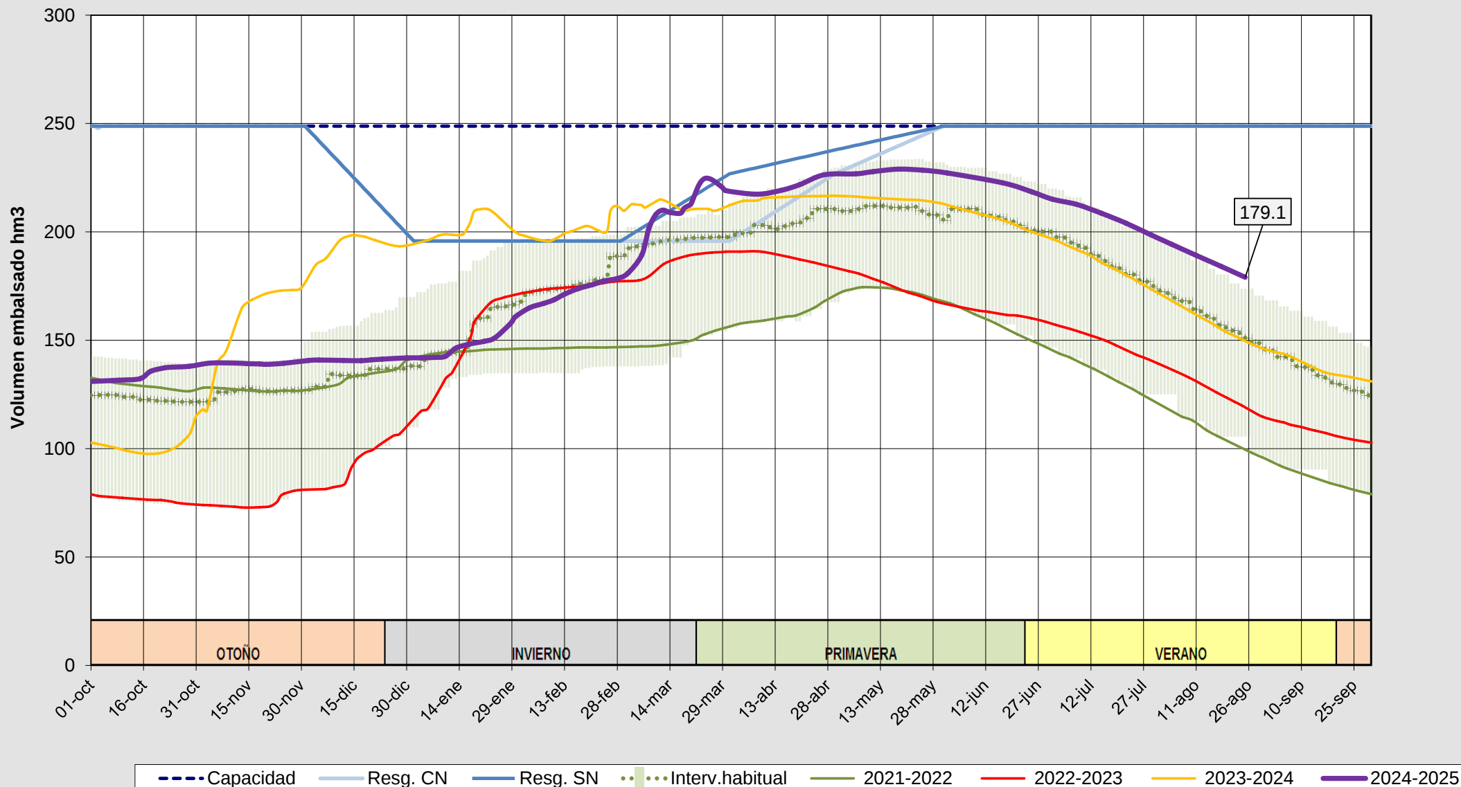
Evolución del volumen almacenado en el embalse de Cuerda del Pozo a fecha 26/08/2025
