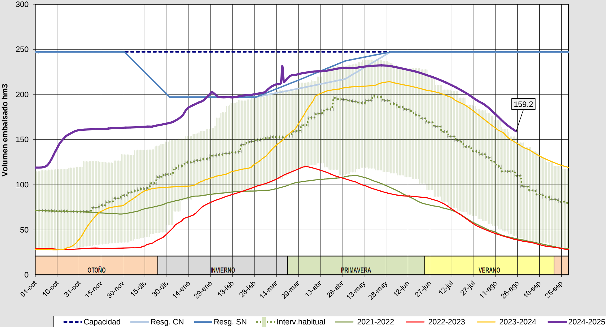
Evolución del volumen almacenado en el embalse de Aguilar a fecha 26/08/2025
