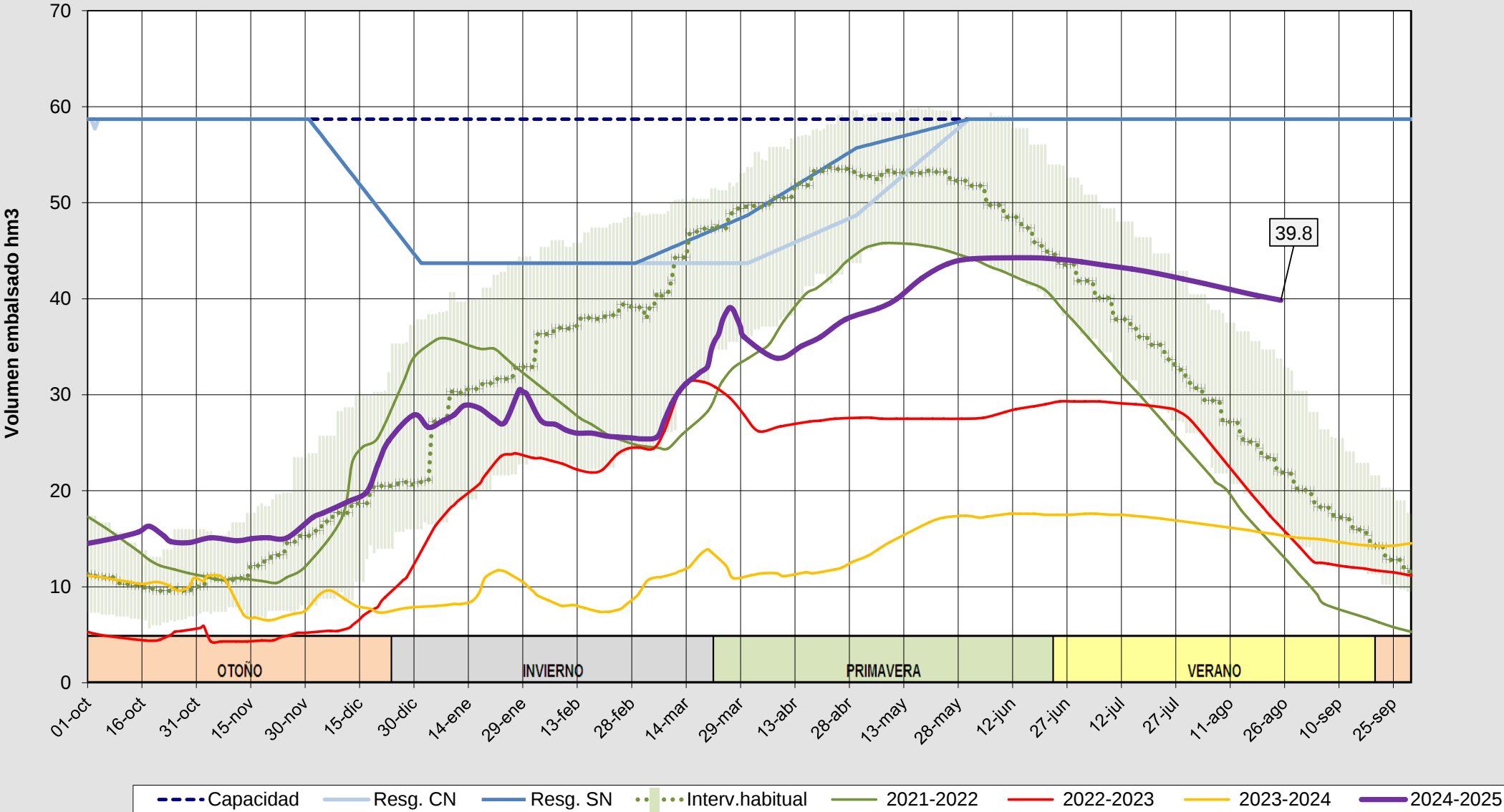
Evolución del volumen almacenado en el embalse de Requejada a fecha 26/08/2025
