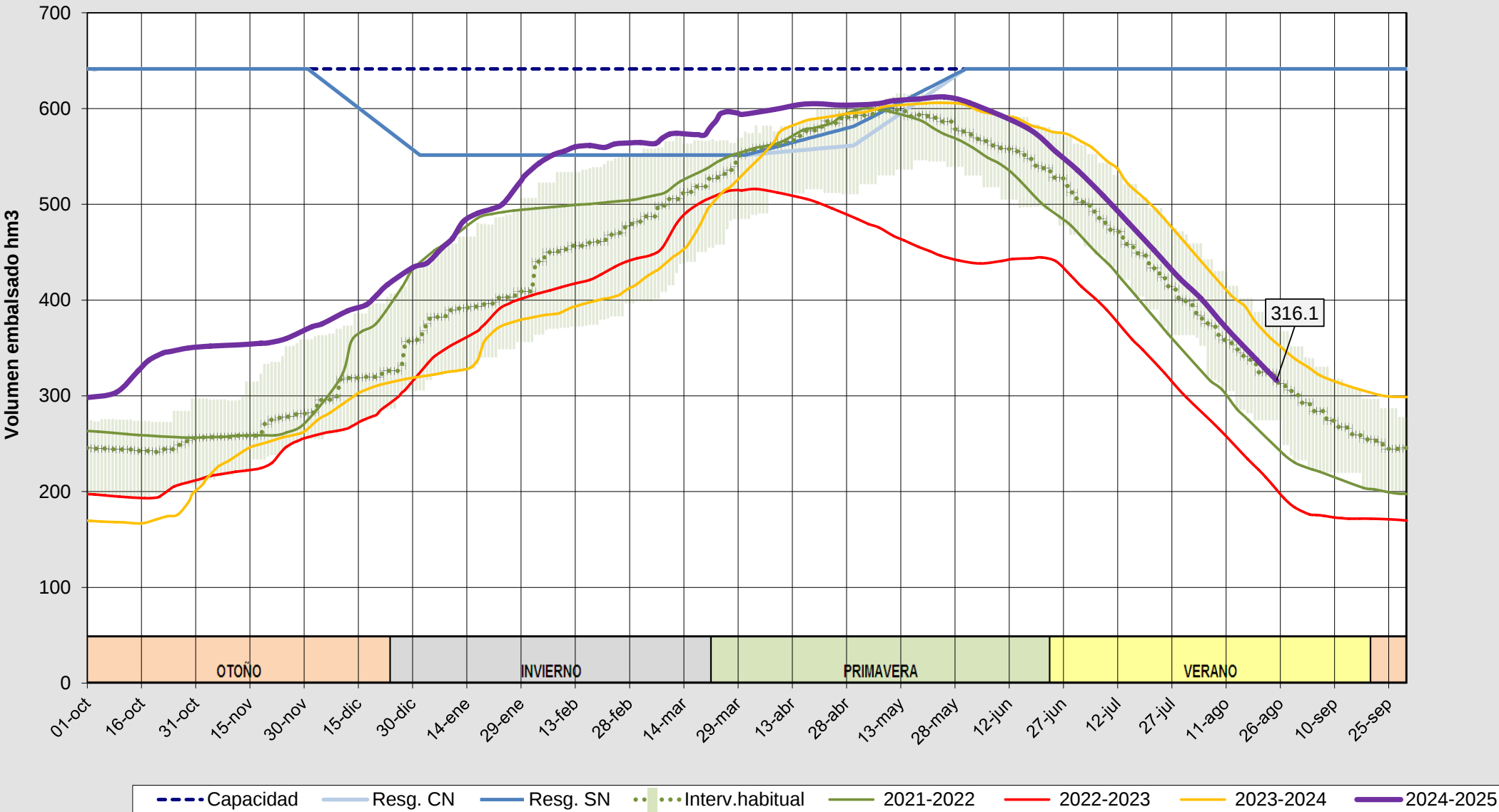
Evolución del volumen almacenado en el embalse de Riaño a fecha 26/08/2025
