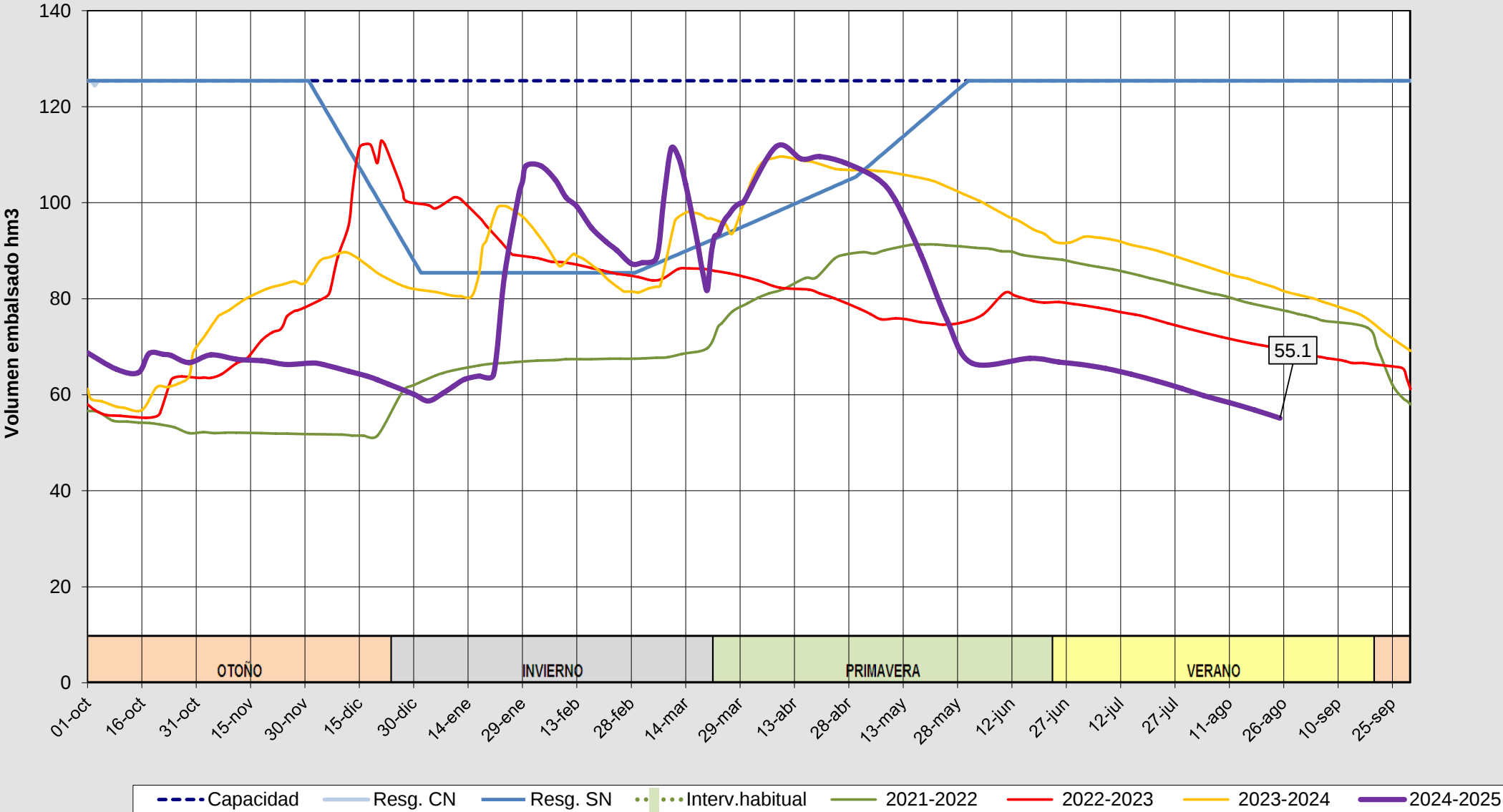
Evolución del volumen almacenado en el sistema del ÁGUEDA a fecha 26/08/2025
