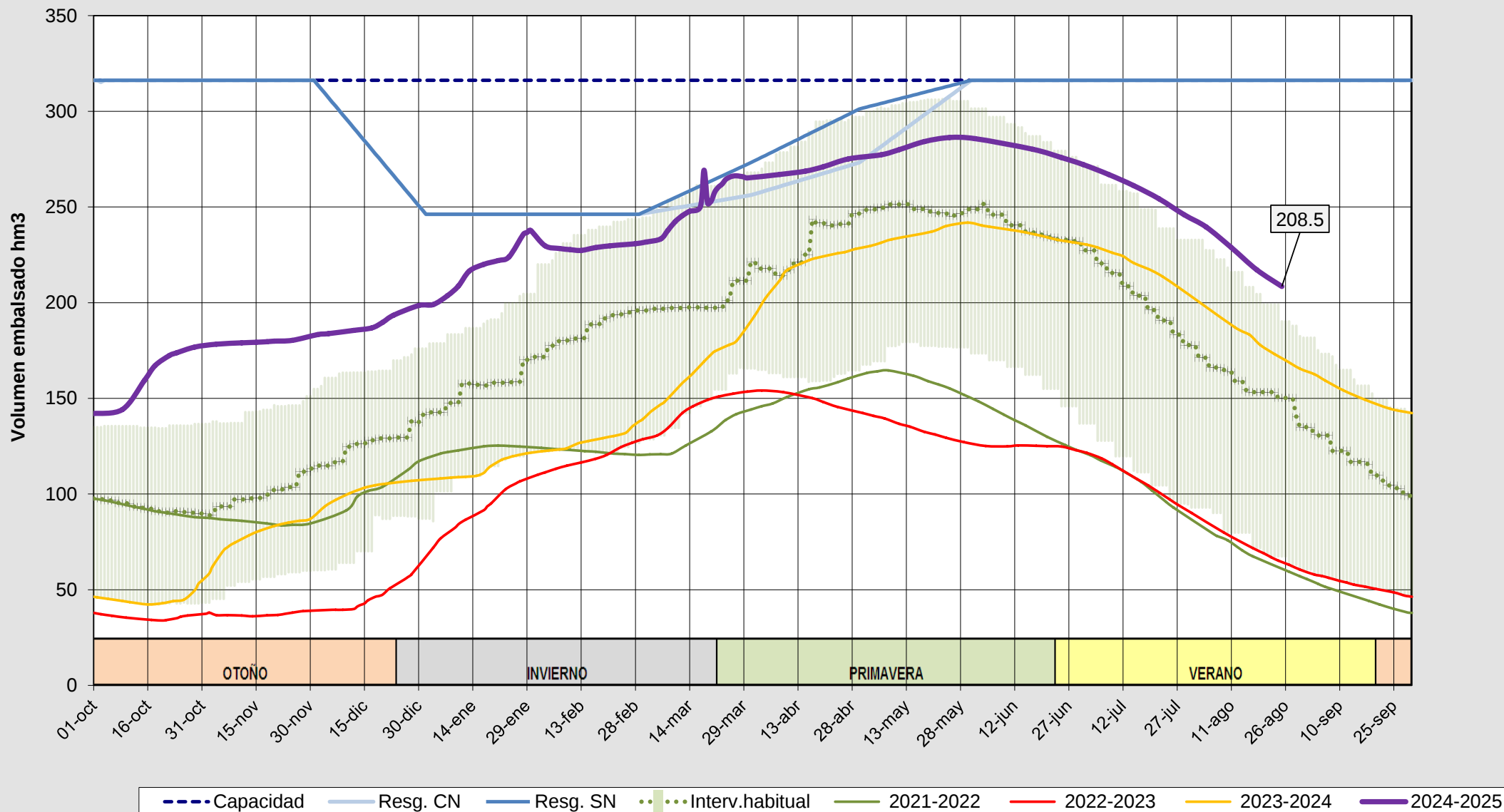
Evolución del volumen almacenado en el sistema del PISUERGA a fecha 26/08/2025
