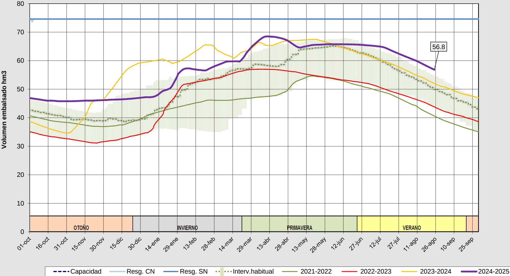
Evolución del volumen almacenado en el embalse de Úzquiza a fecha 26/08/2025
