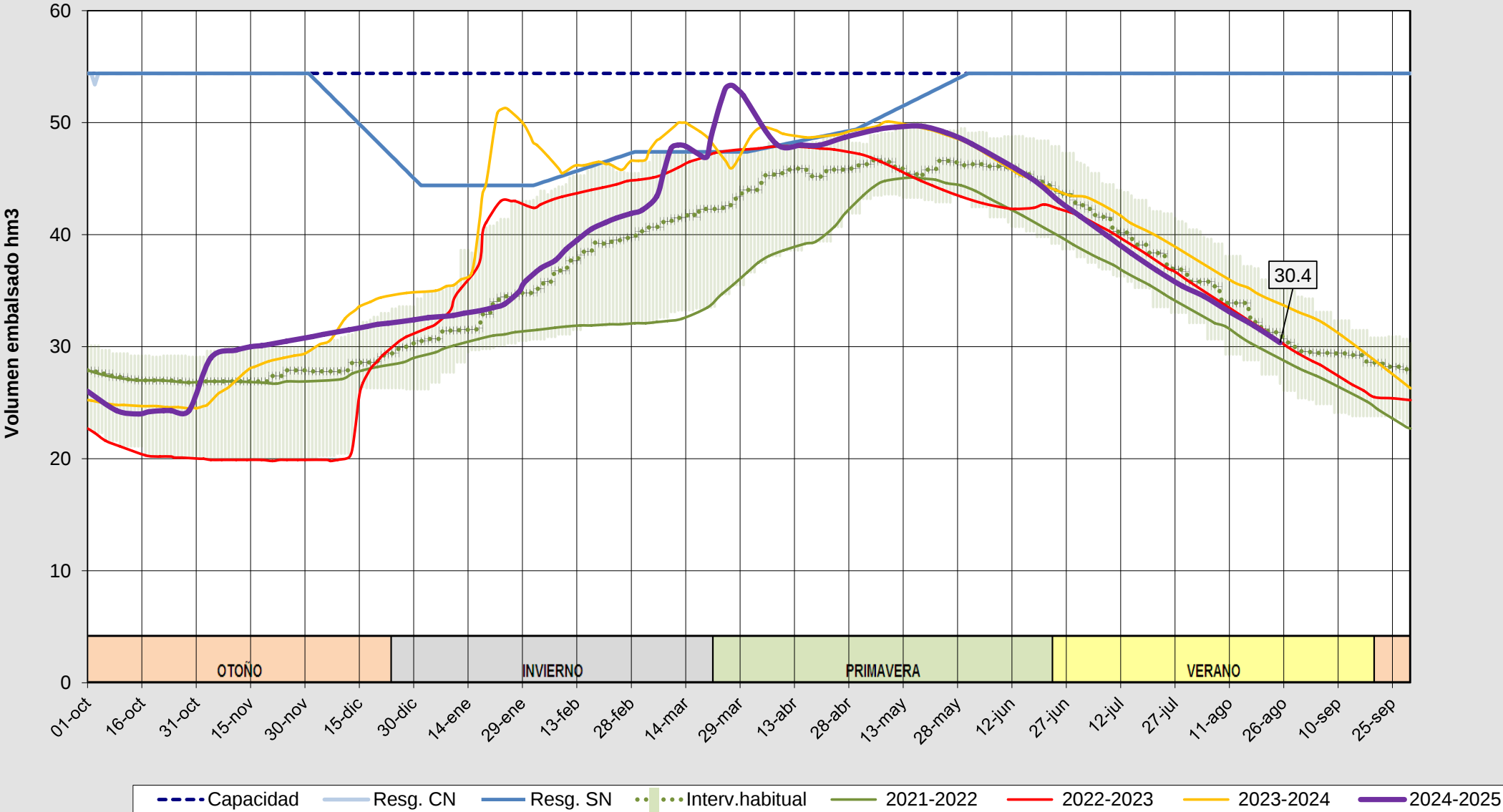
Evolución del volumen almacenado en el embalse de Linares del Arroyo a fecha 26/08/2025
