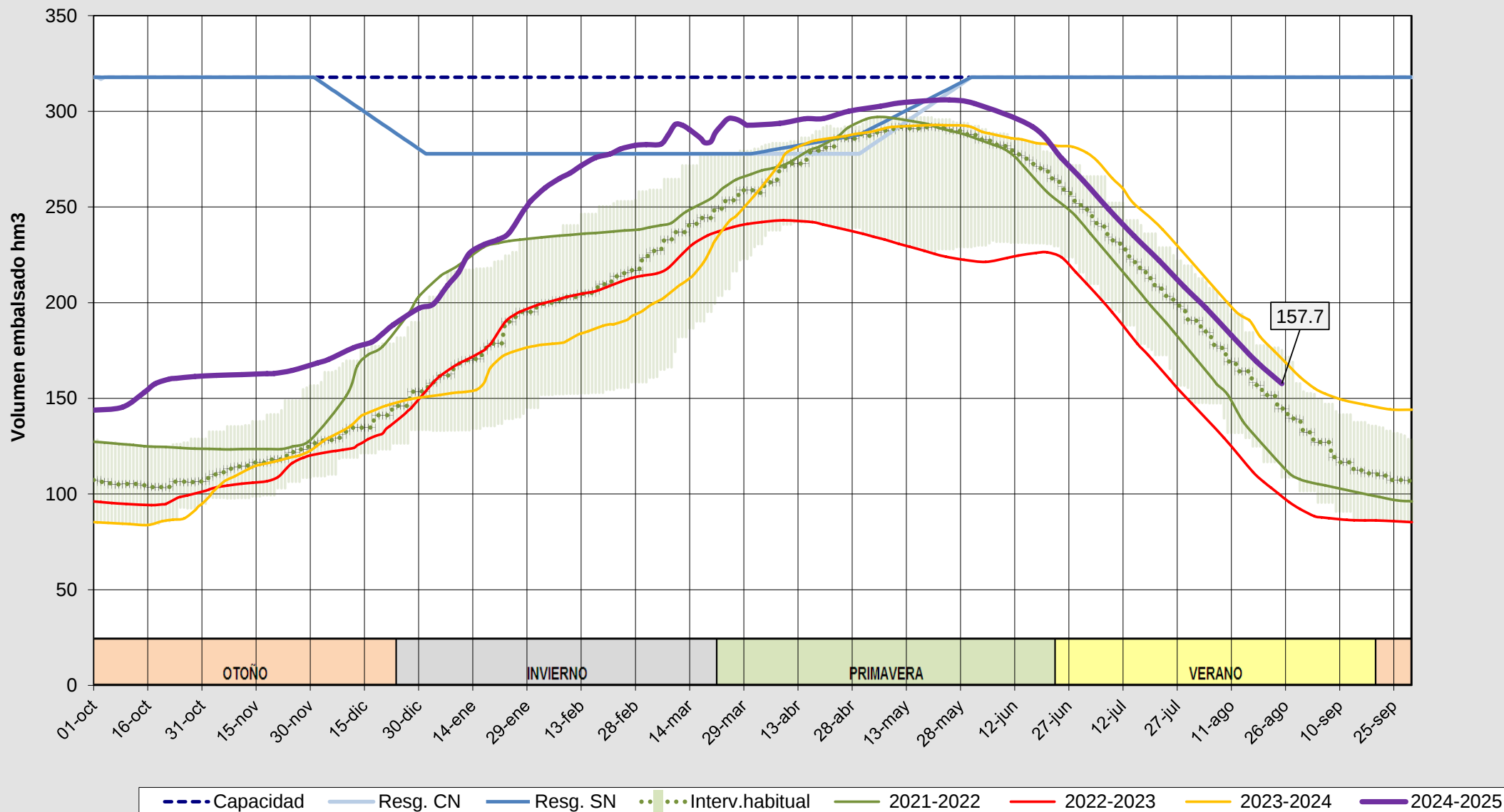
Evolución del volumen almacenado en el embalse de Porma a fecha 26/08/2025
