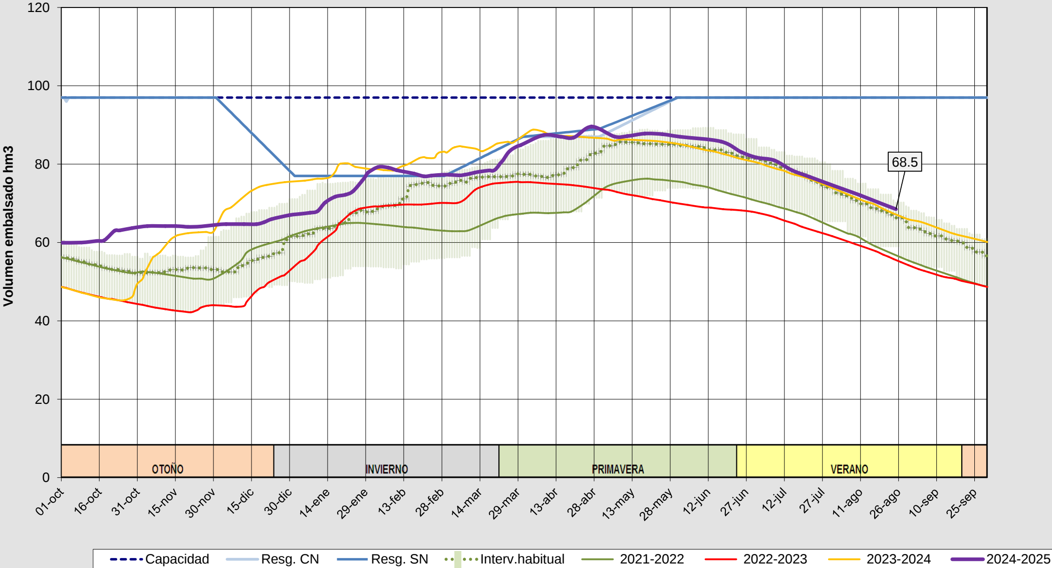
Evolución del volumen almacenado en el sistema del ARLANZÓN a fecha 26/08/2025
