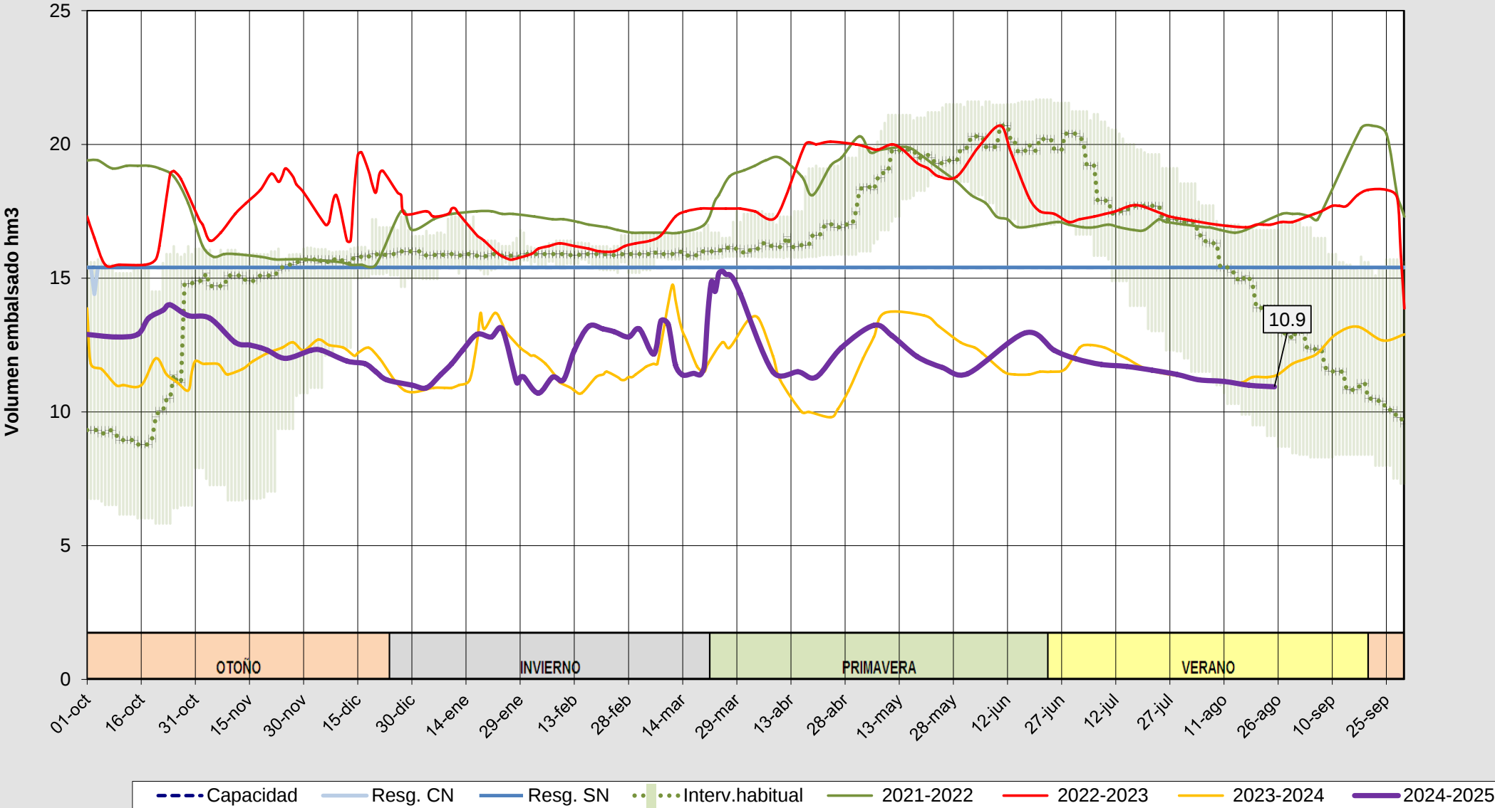
Evolución del volumen almacenado en el embalse de Águeda a fecha 26/08/2025
