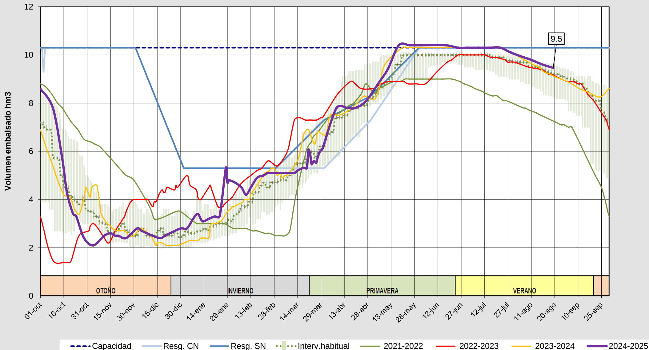
Evolución del volumen almacenado en el embalse de Cervera a fecha 26/08/2025
