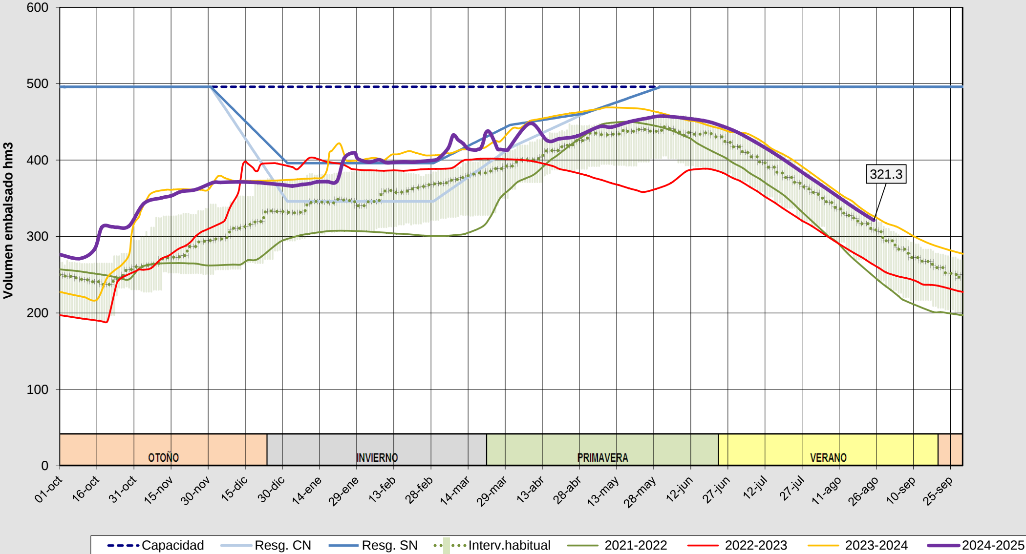
Evolución del volumen almacenado en el embalse de Santa Teresa a fecha 26/08/2025
