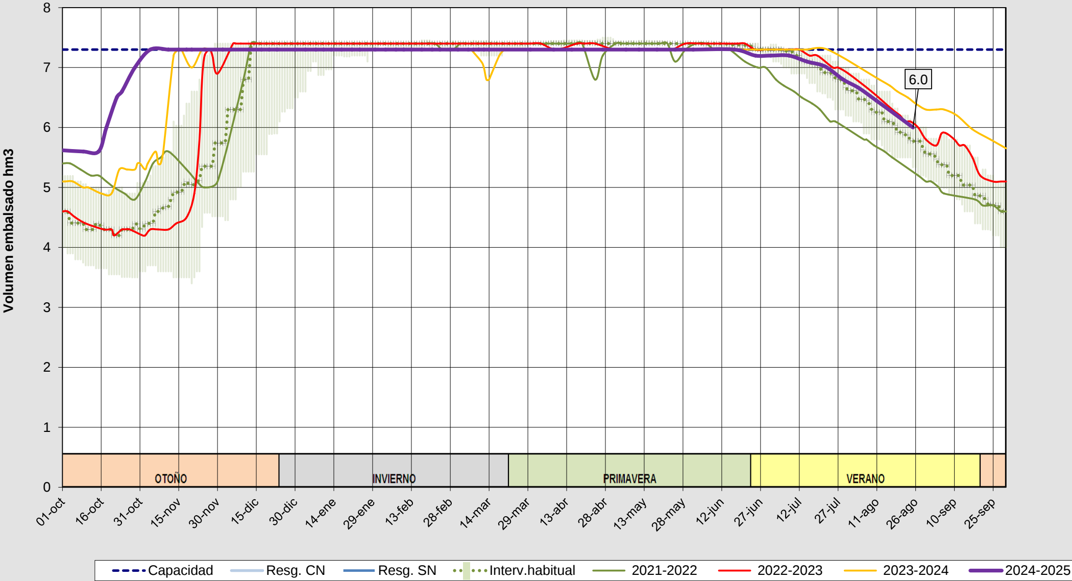
Evolución del volumen almacenado en el embalse de Pontón Alto a fecha 26/08/2025
