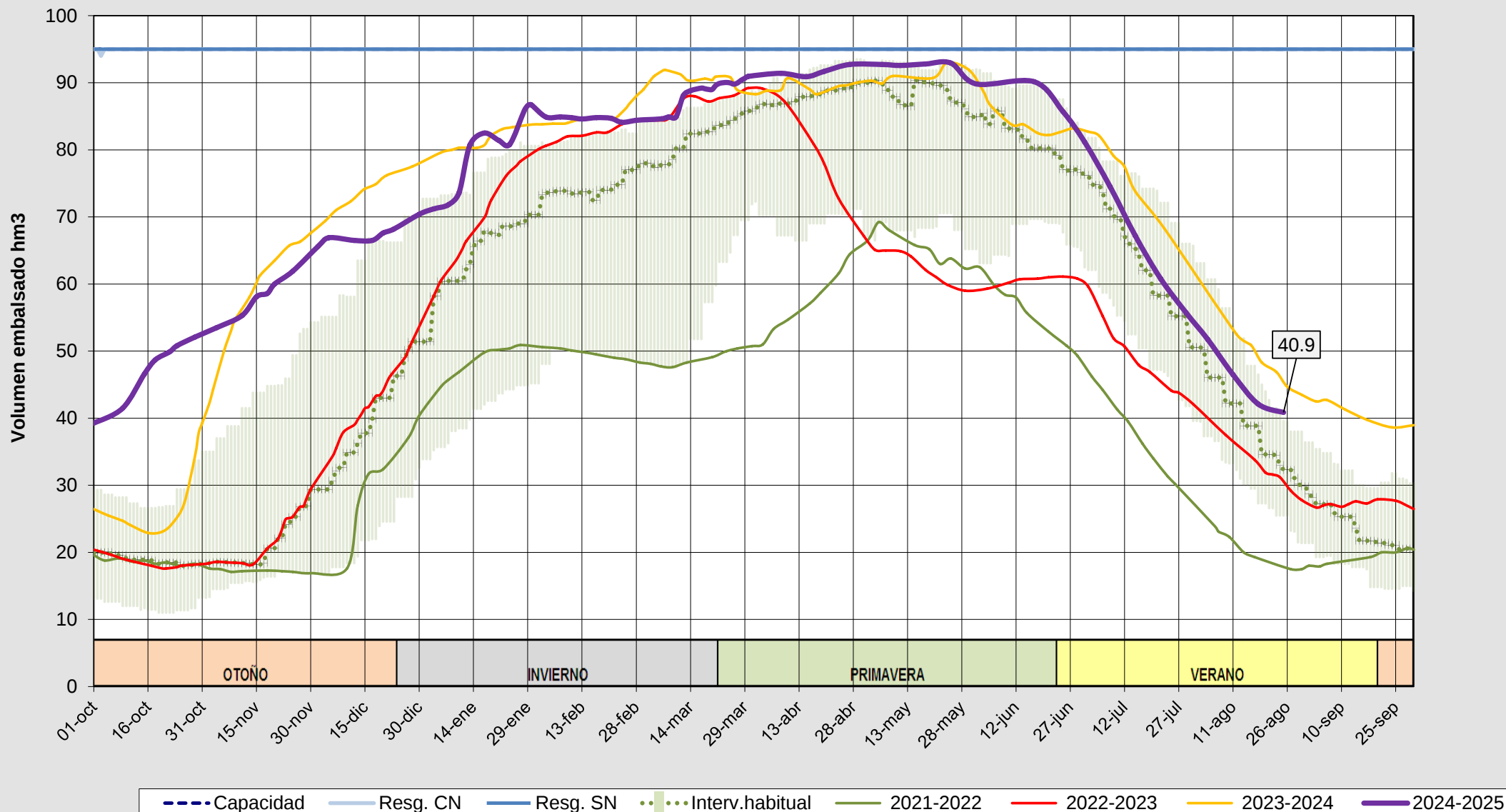
Evolución del volumen almacenado en el embalse de Compuerto a fecha 26/08/2025
