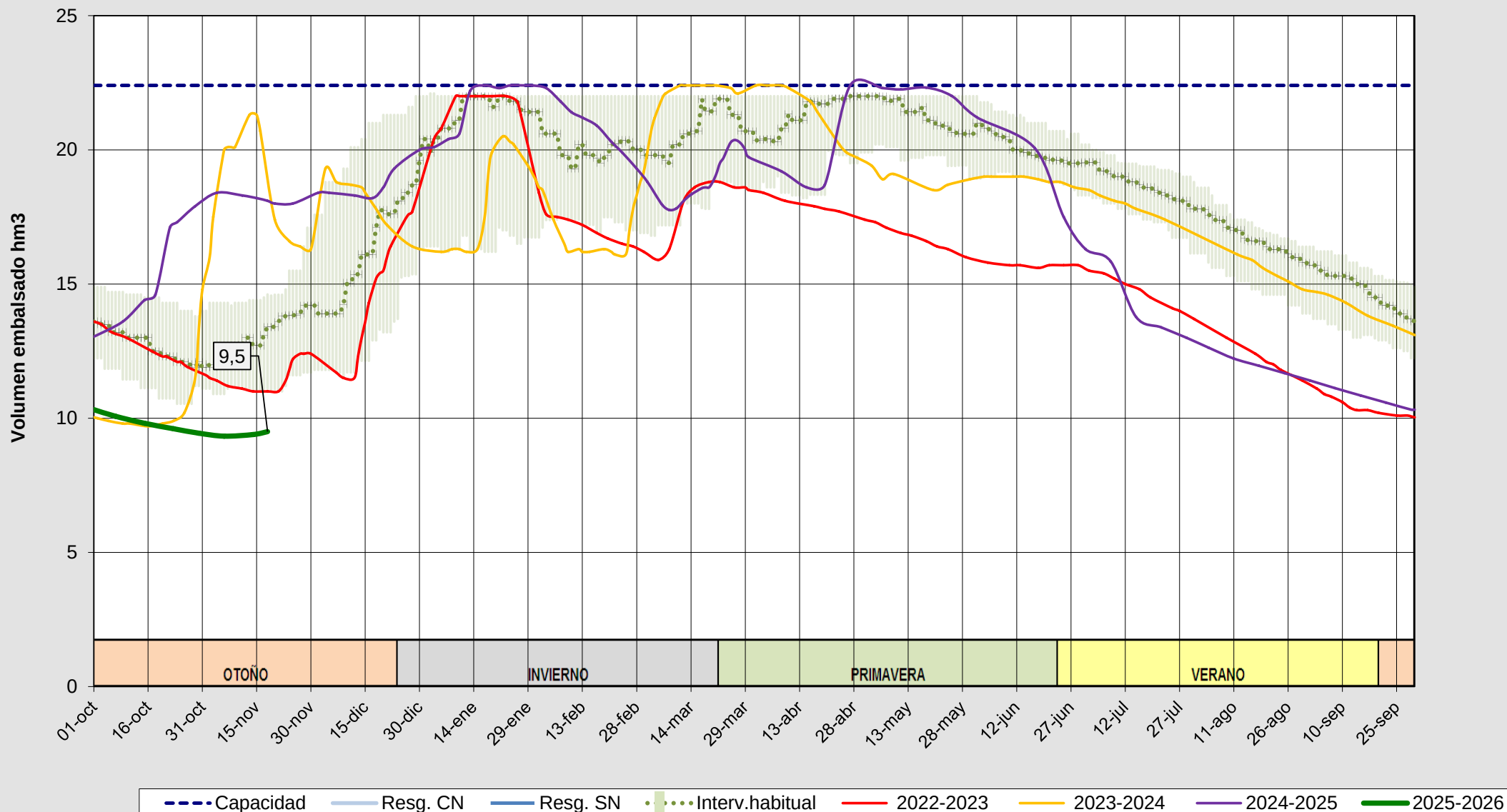
Evolución del volumen almacenado en el embalse de Arlanzón a fecha 18/11/2025
