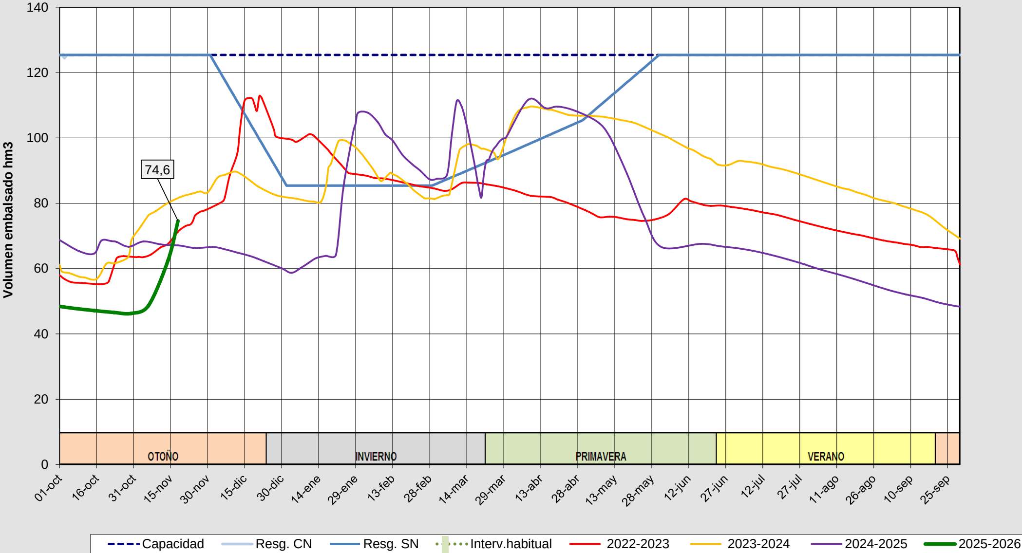
Evolución del volumen almacenado en el sistema del ÁGUEDA a fecha 18/11/2025
