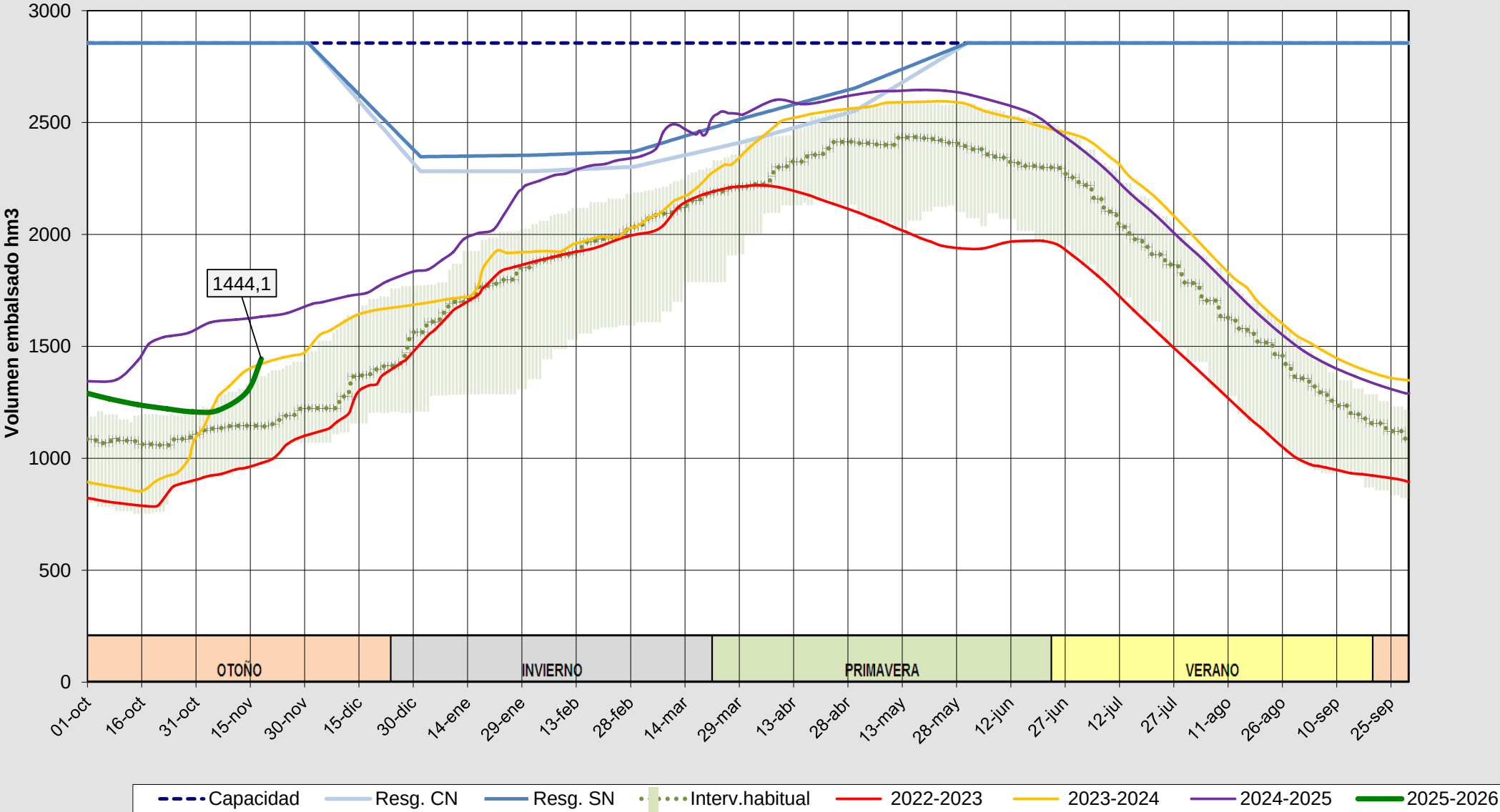
Evolución del volumen almacenado en el sistema del DUERO (ESTADO) a fecha 18/11/2025
