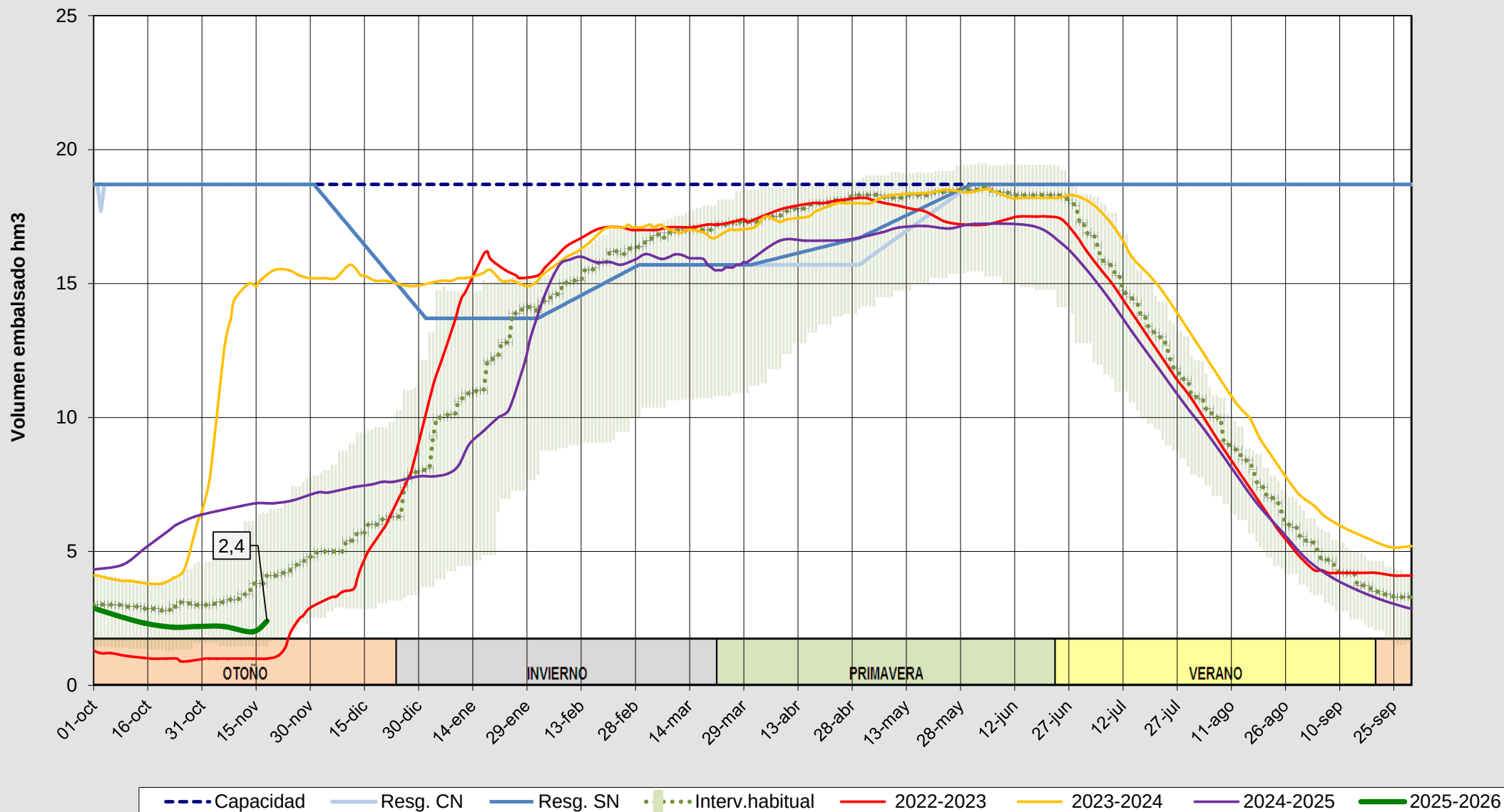
Evolución del volumen almacenado en el embalse de Villameca a fecha 18/11/2025
