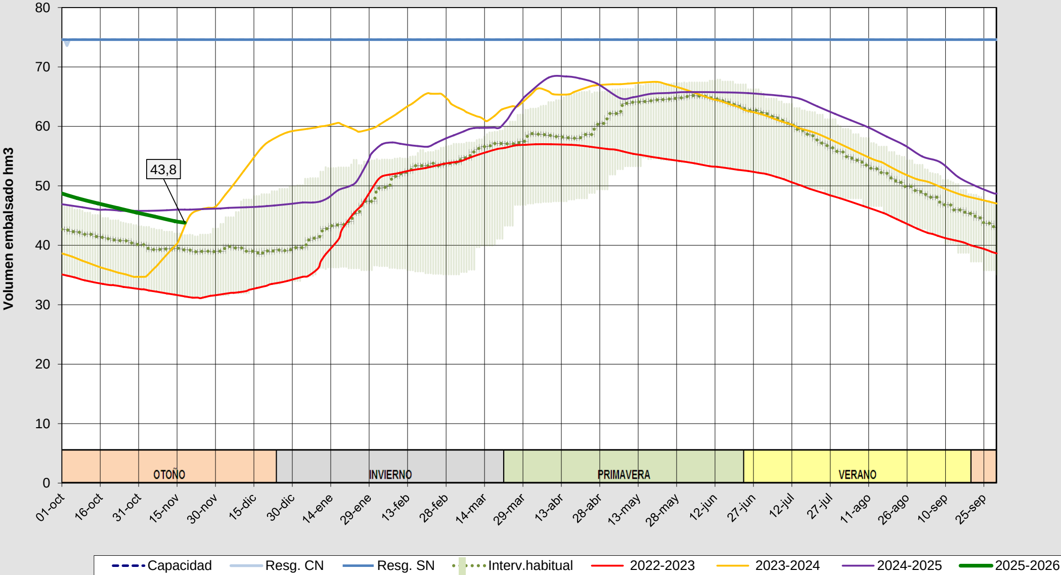
Evolución del volumen almacenado en el embalse de Úzquiza a fecha 18/11/2025
