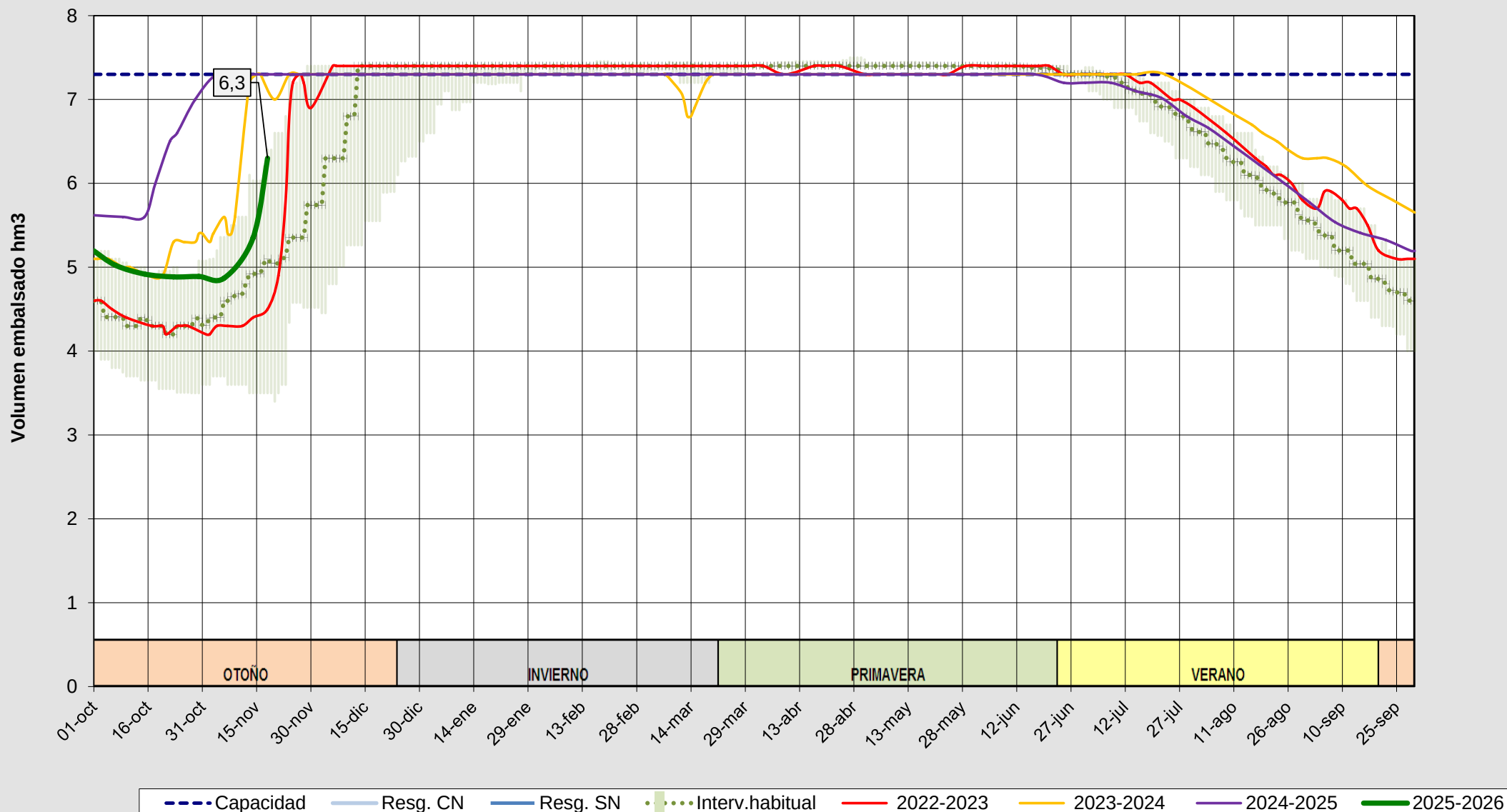
Evolución del volumen almacenado en el embalse de Pontón Alto a fecha 18/11/2025
