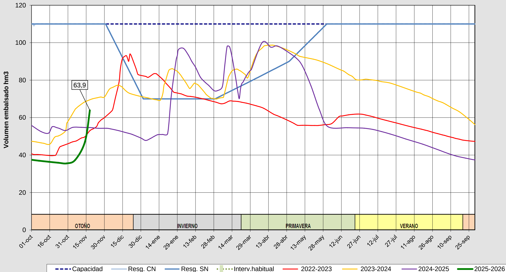
Evolución del volumen almacenado en el embalse de Iruña a fecha 18/11/2025
