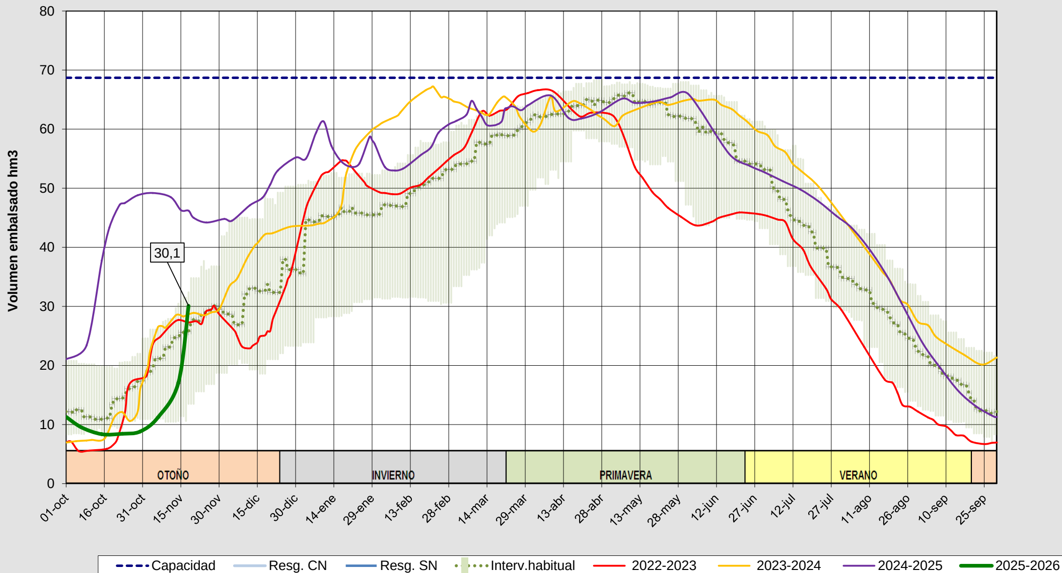
Evolución del volumen almacenado en el embalse de Camporredondo a fecha 18/11/2025
