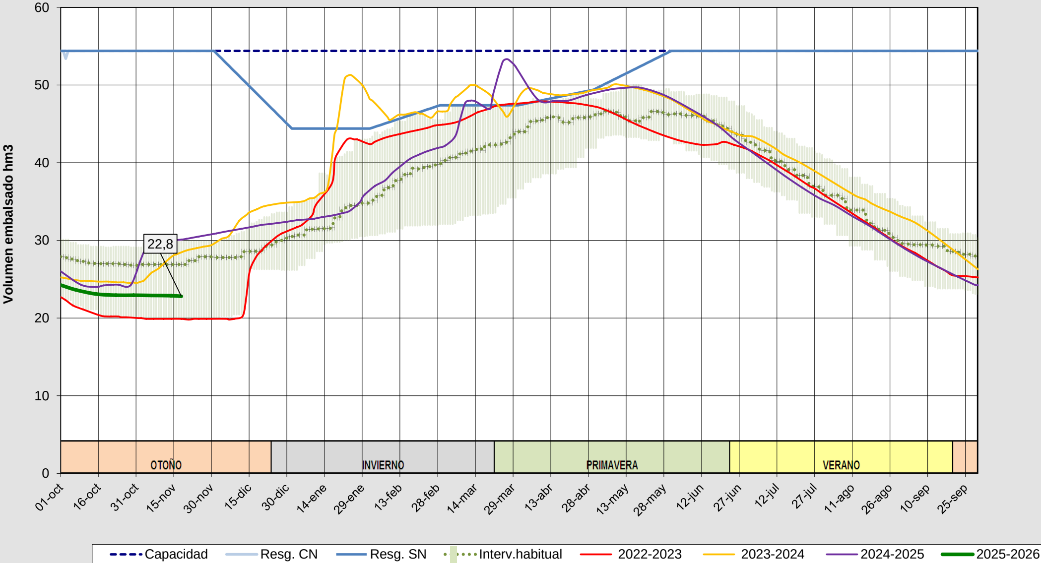
Evolución del volumen almacenado en el embalse de Linares del Arroyo a fecha 18/11/2025
