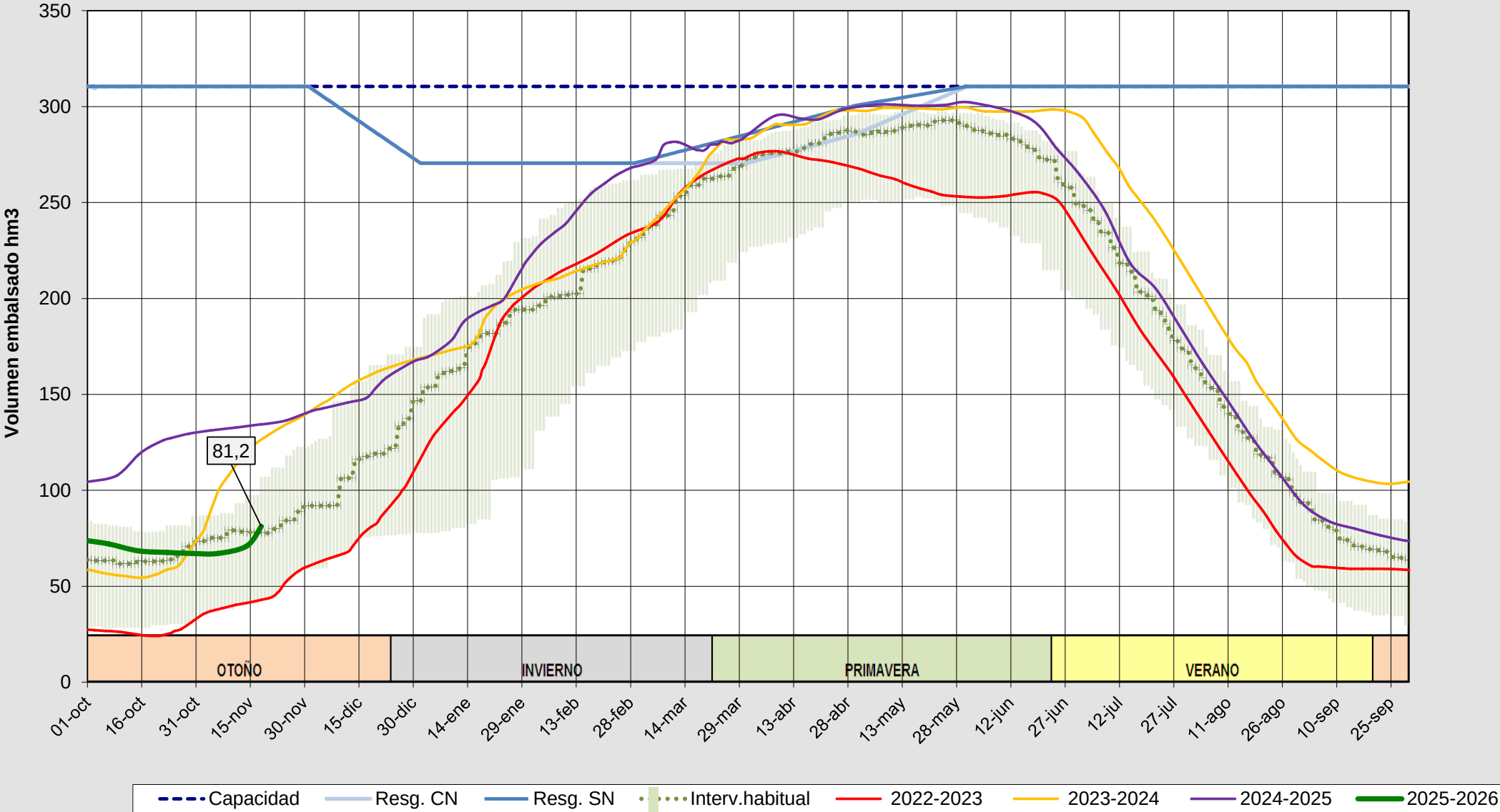
Evolución del volumen almacenado en el embalse de Barrios de Luna a fecha 18/11/2025
