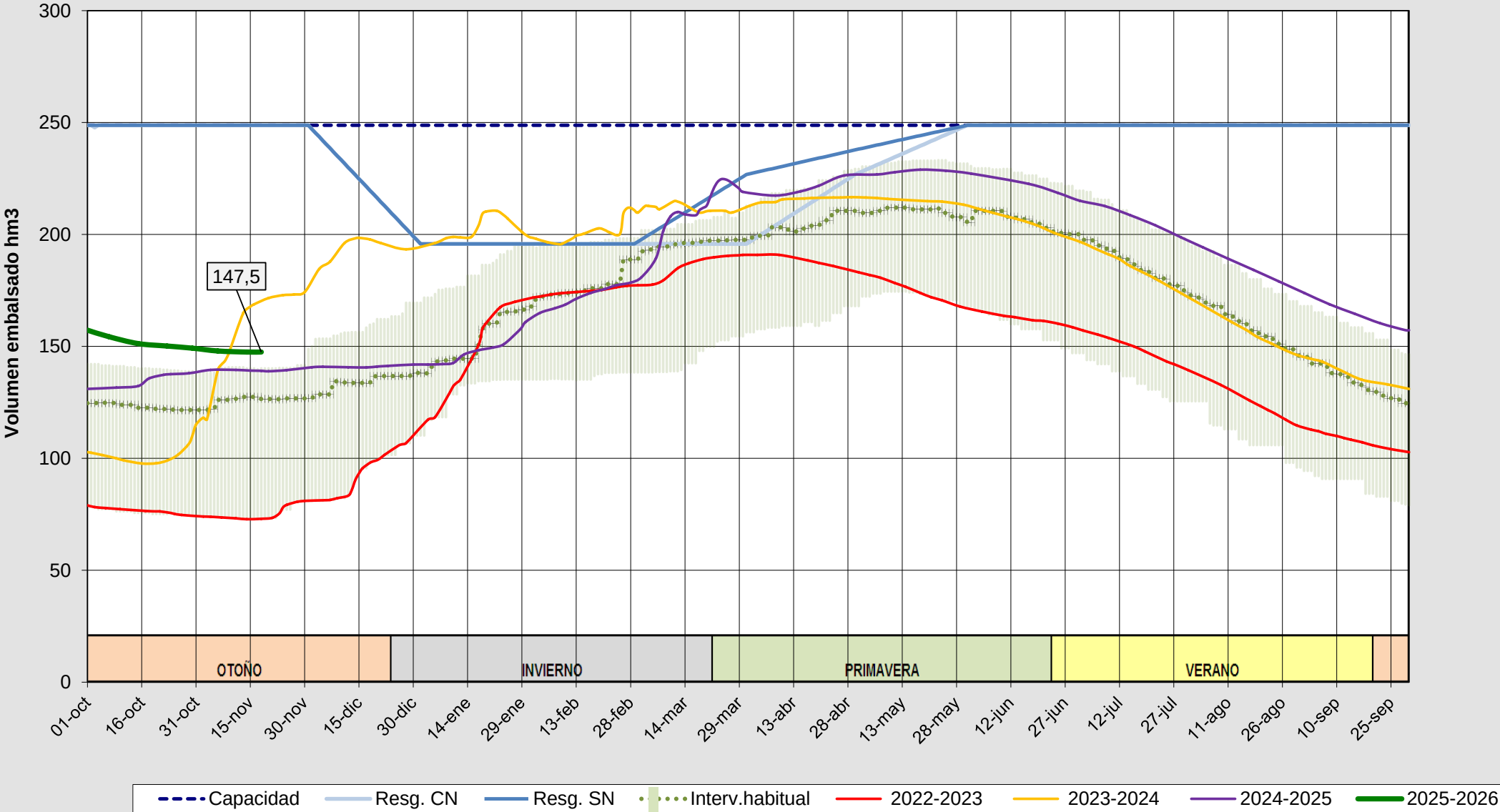
Evolución del volumen almacenado en el embalse de Cuerda del Pozo a fecha 18/11/2025
