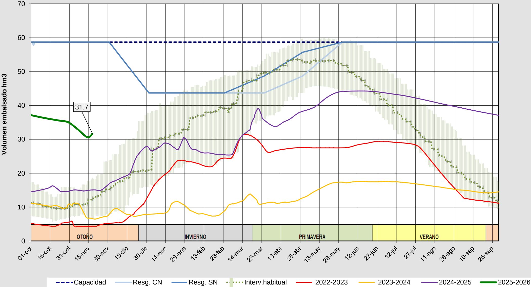
Evolución del volumen almacenado en el embalse de Requejada a fecha 18/11/2025
