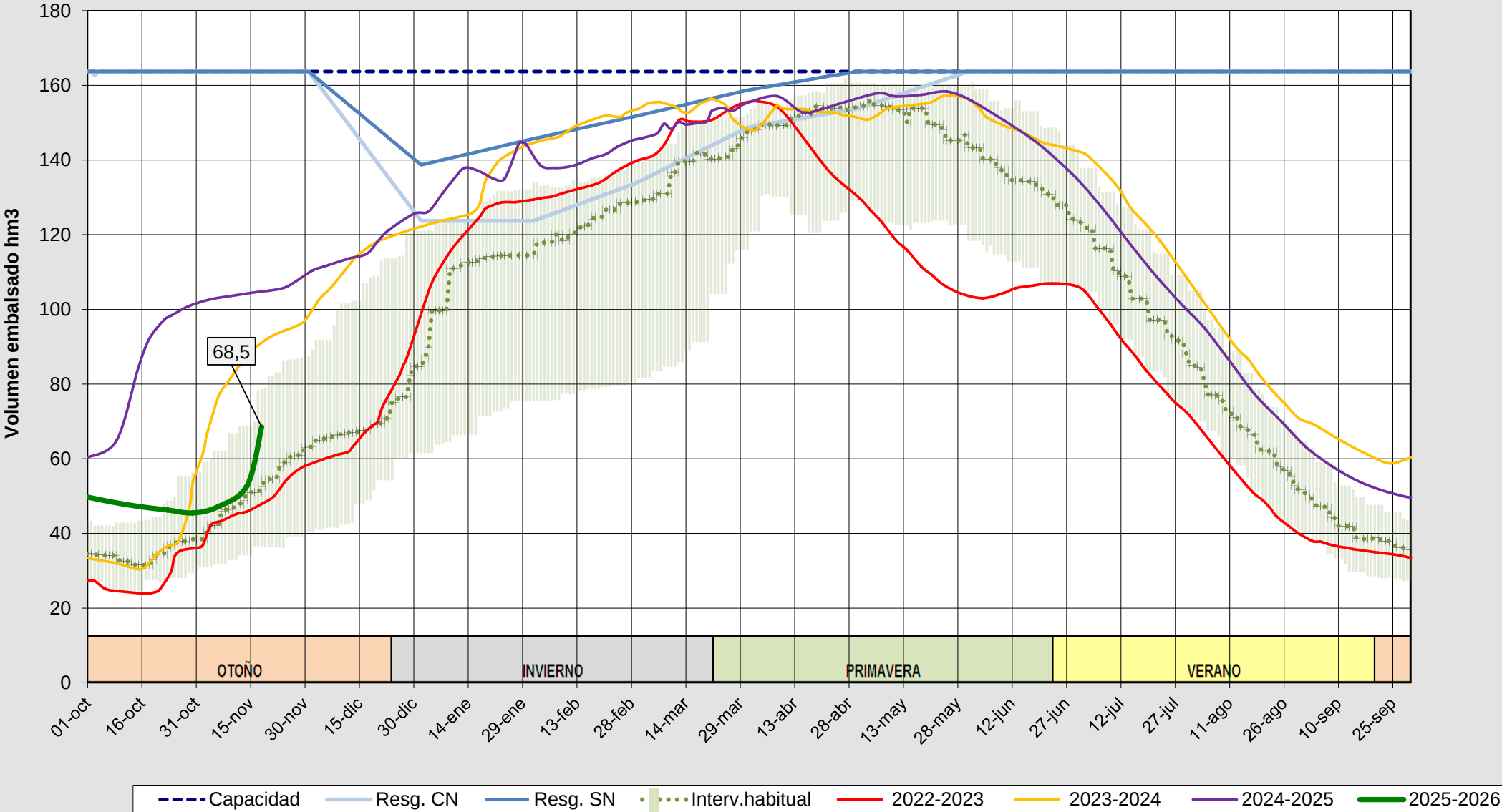
Evolución del volumen almacenado en el sistema del CARRIÓN a fecha 18/11/2025
