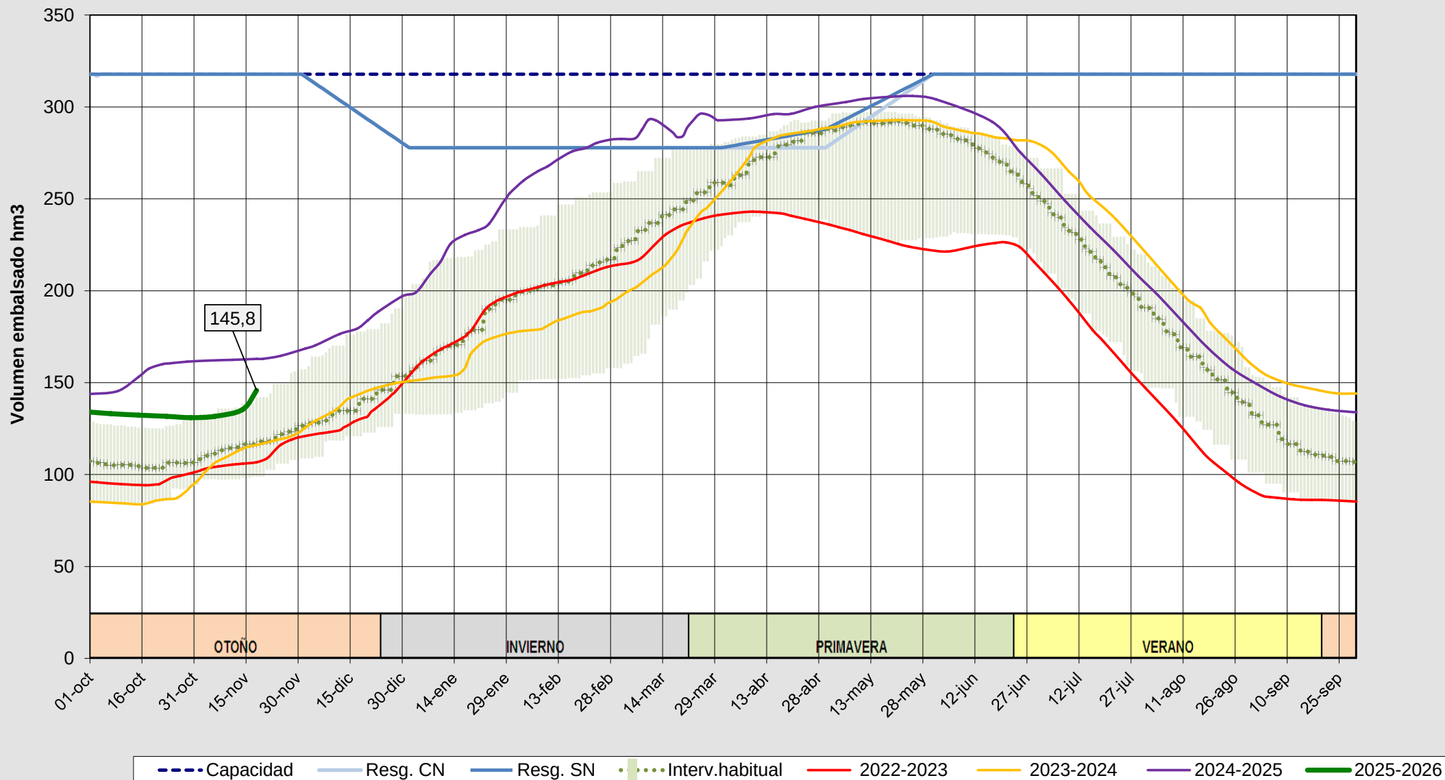
Evolución del volumen almacenado en el embalse de Porma a fecha 18/11/2025
