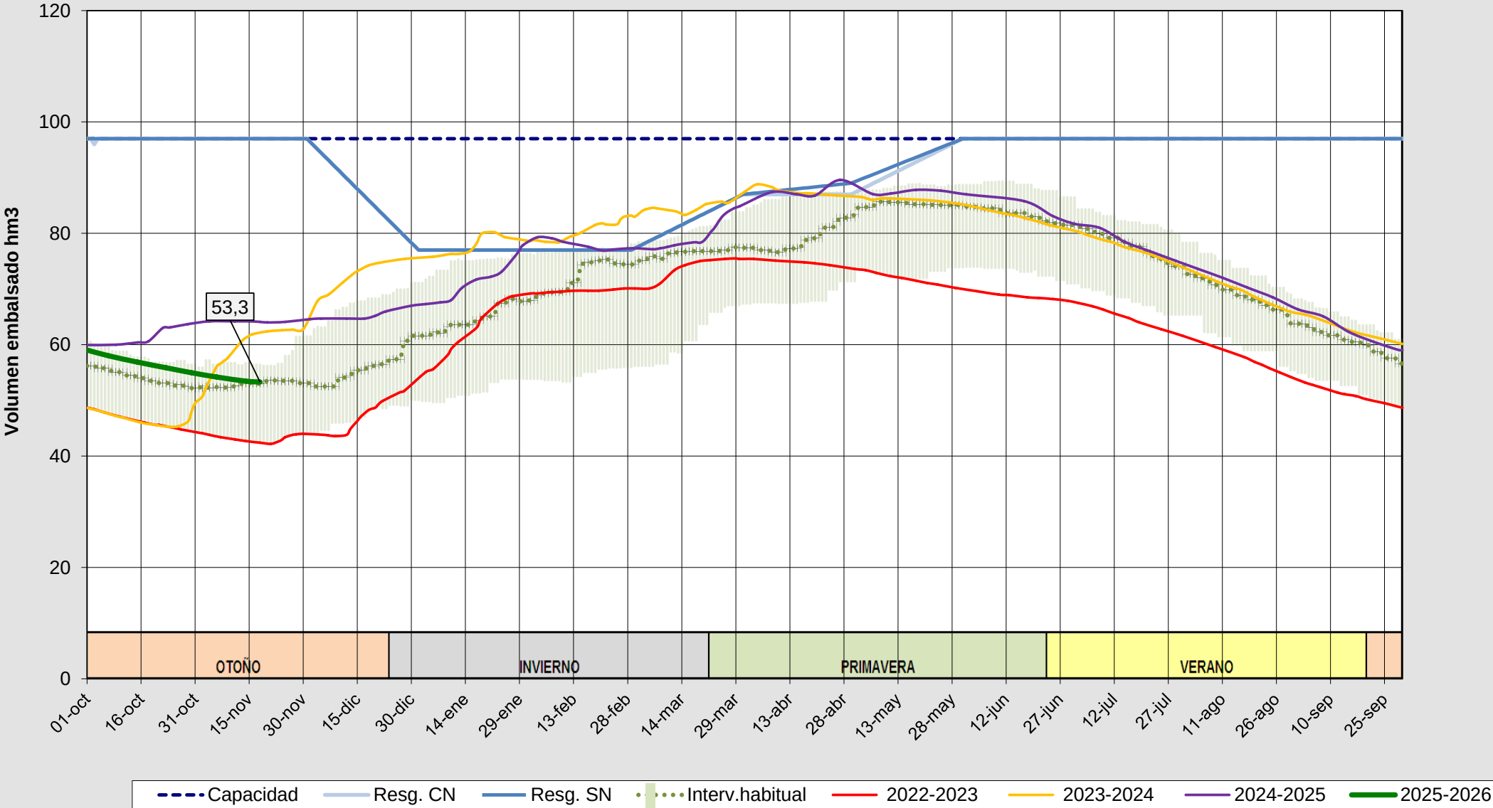
Evolución del volumen almacenado en el sistema del ARLANZÓN a fecha 18/11/2025
