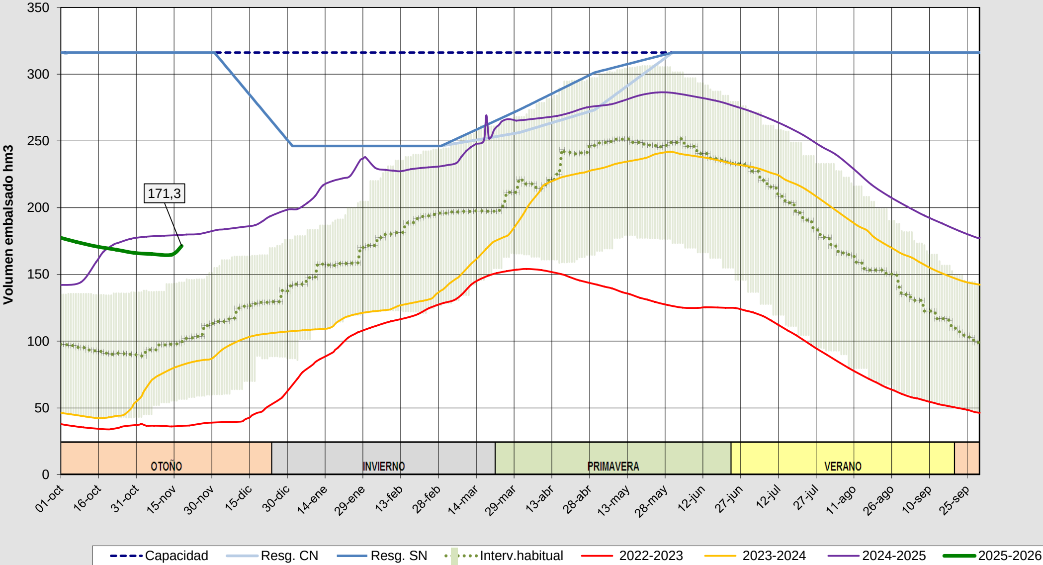
Evolución del volumen almacenado en el sistema del PISUERGA a fecha 18/11/2025
