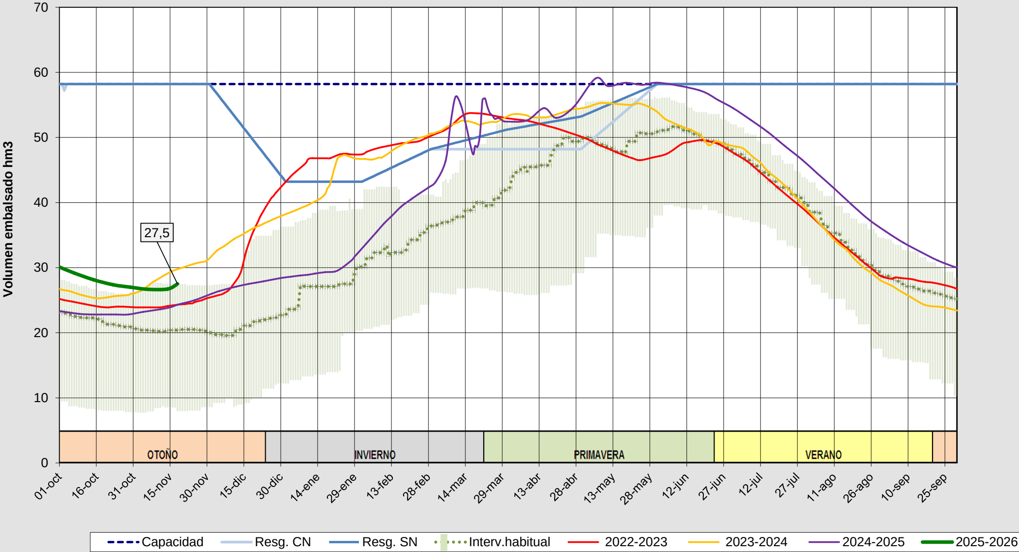
Evolución del volumen almacenado en el embalse de Las Cogotas a fecha 18/11/2025
