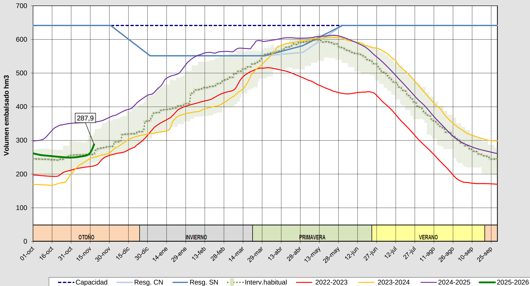
Evolución del volumen almacenado en el embalse de Riaño a fecha 18/11/2025
