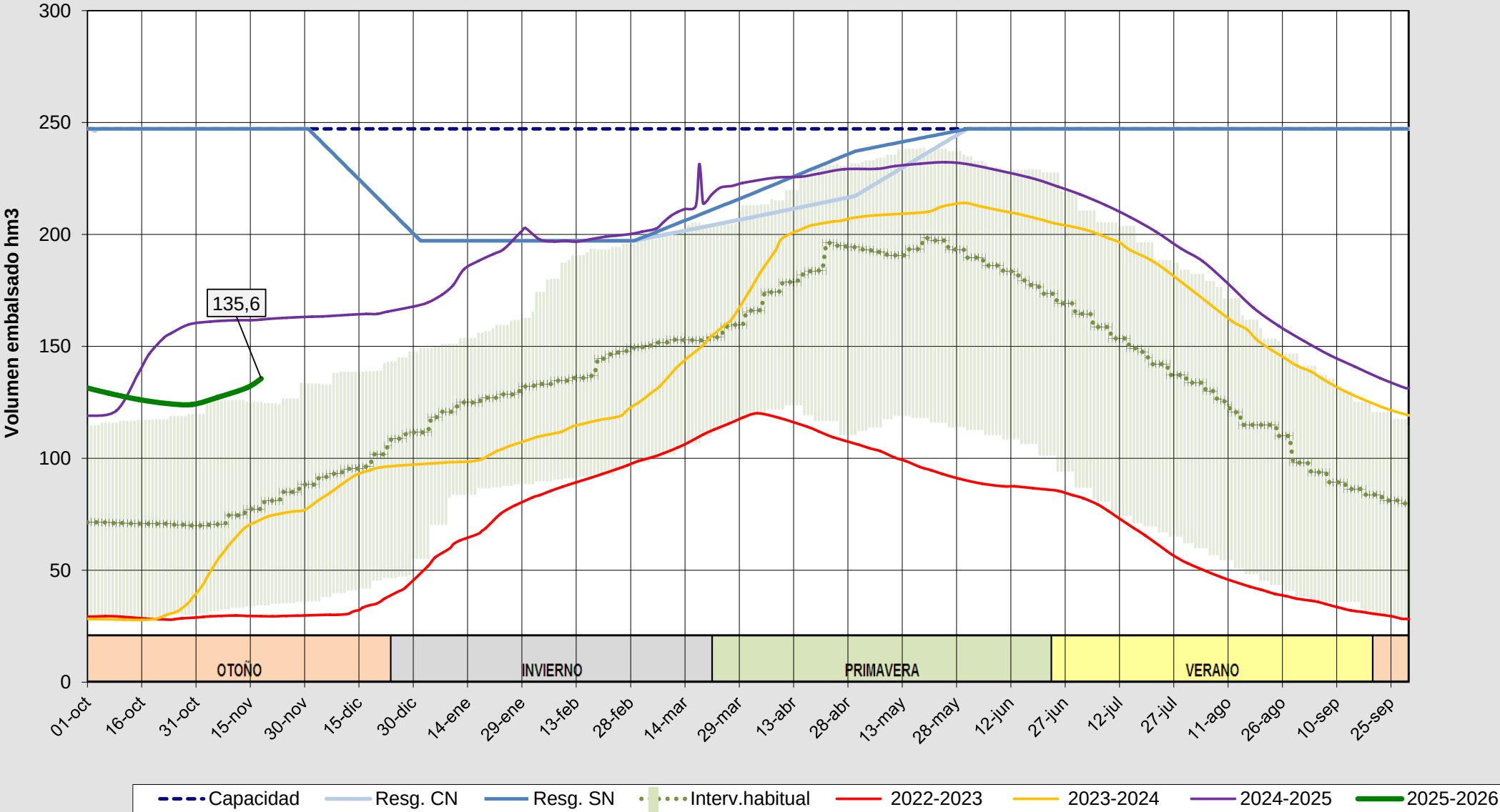
Evolución del volumen almacenado en el embalse de Aguilar a fecha 18/11/2025
