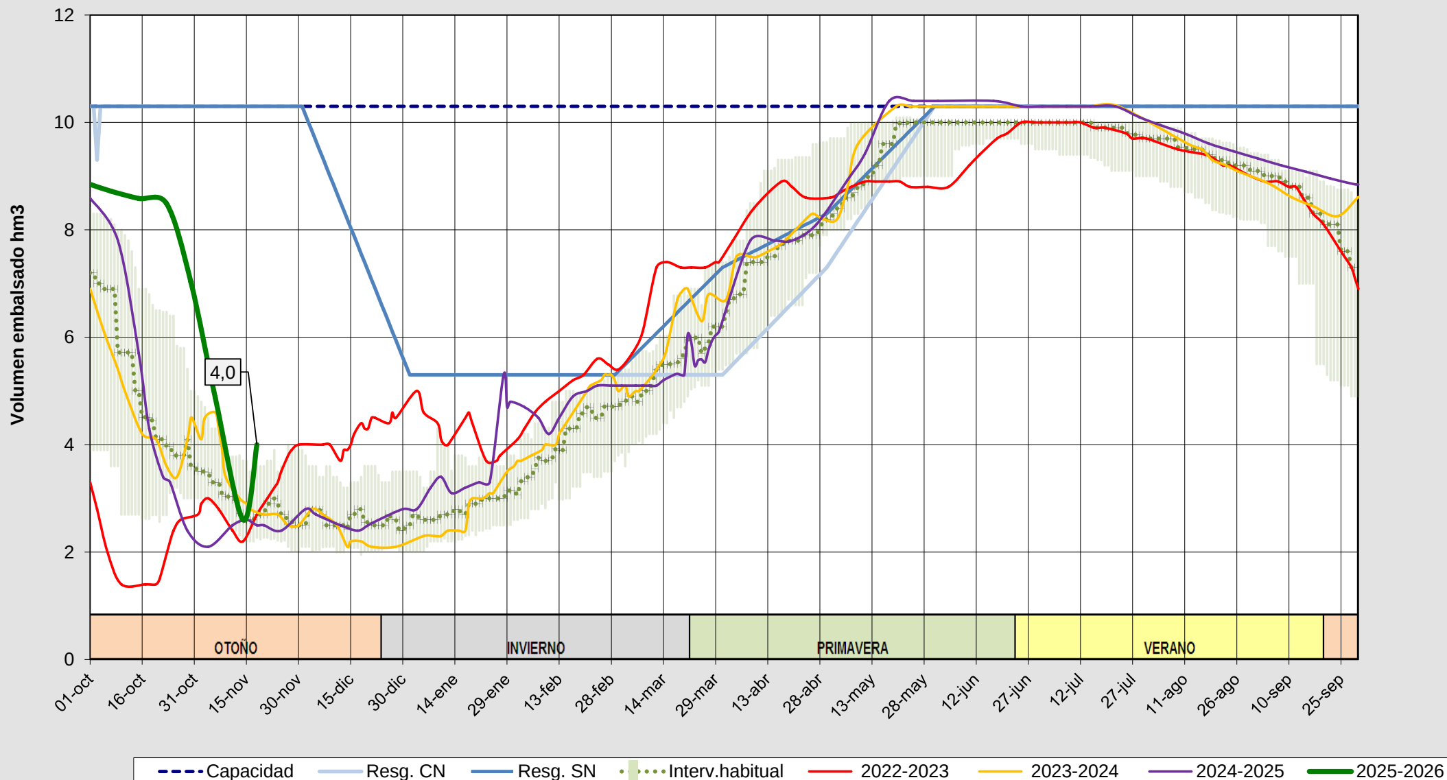
Evolución del volumen almacenado en el embalse de Cervera a fecha 18/11/2025
