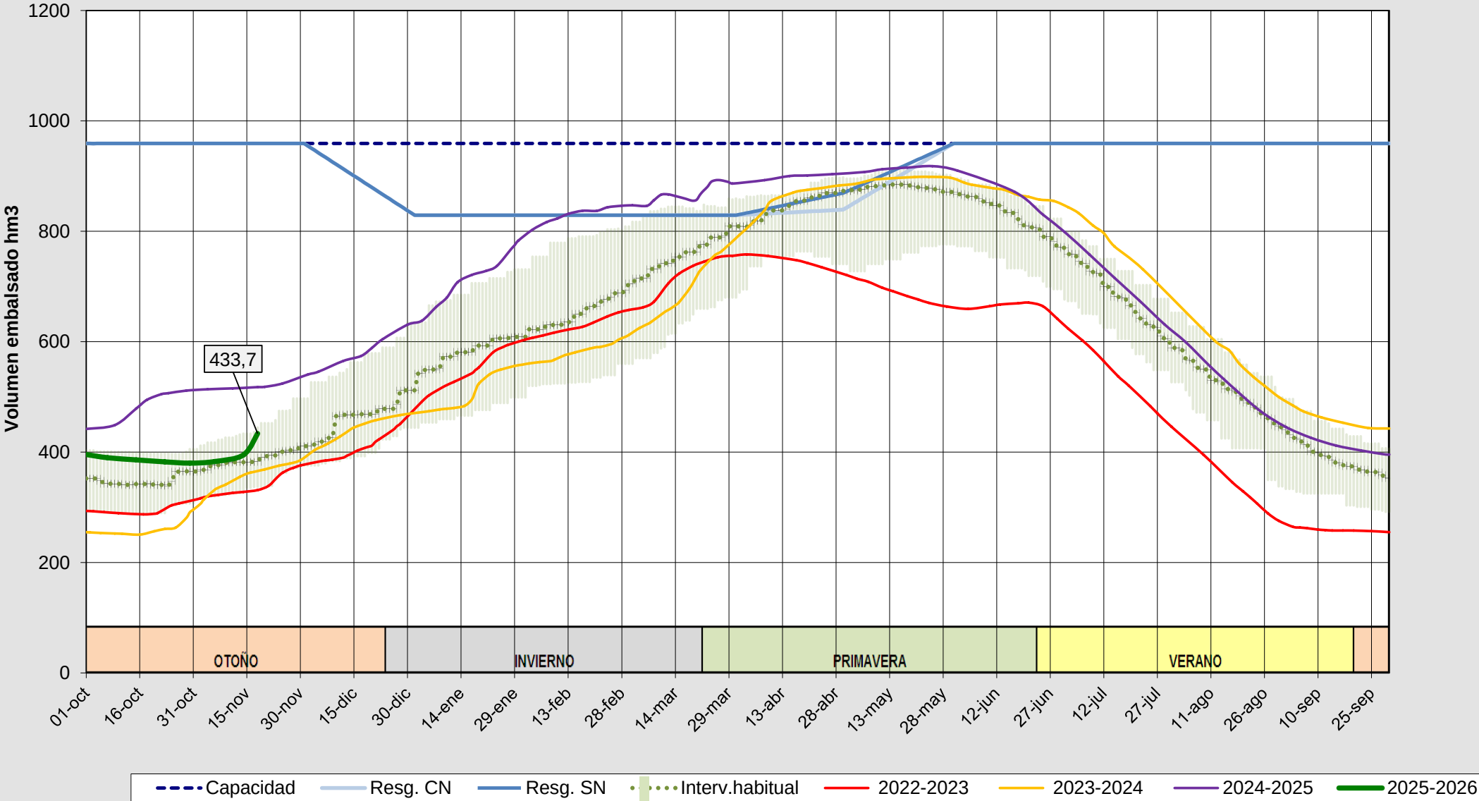
Evolución del volumen almacenado en el sistema del PORMA-ESLA a fecha 18/11/2025
