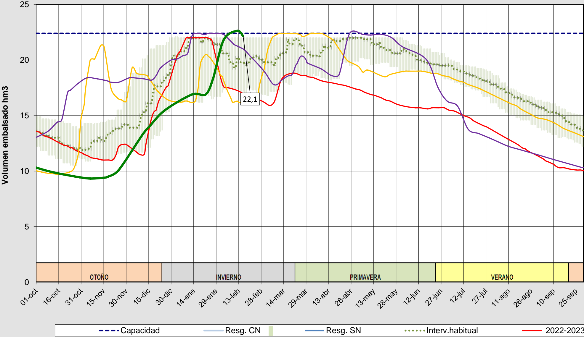
Evolución del volumen almacenado en el embalse de Arlanzón a fecha 16/02/2026
