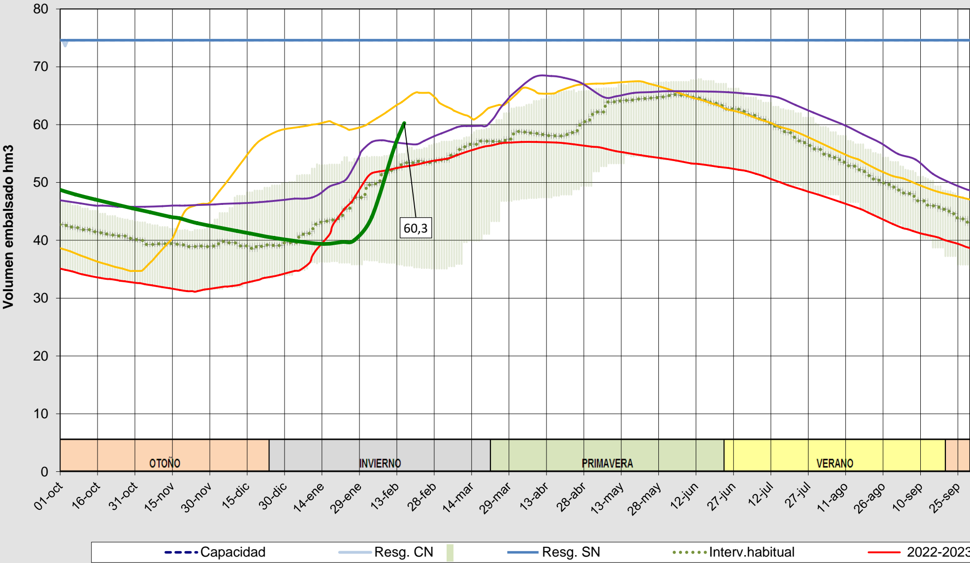
Evolución del volumen almacenado en el embalse de Úzquiza a fecha 16/02/2026
