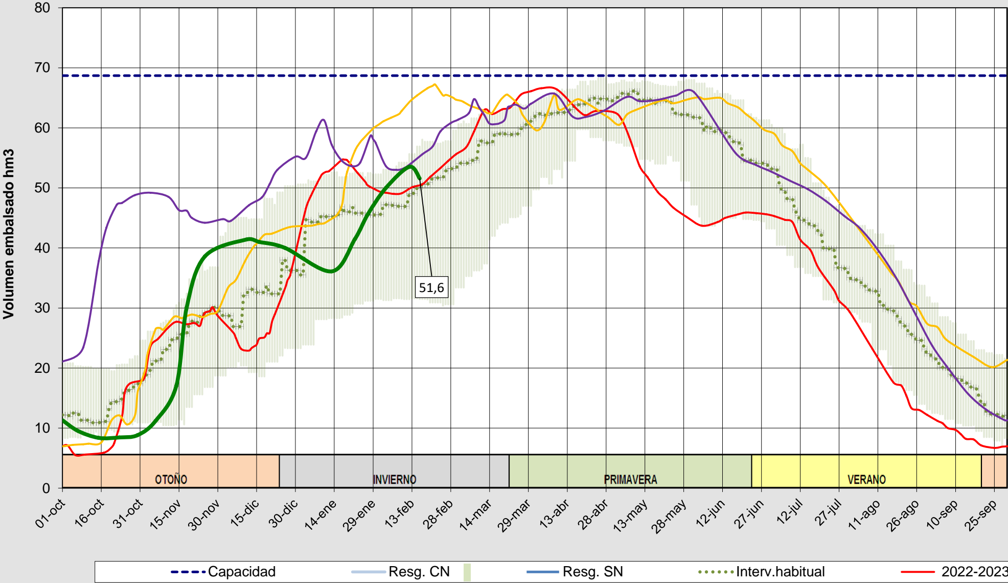
Evolución del volumen almacenado en el embalse de Camporredondo a fecha 16/02/2026
