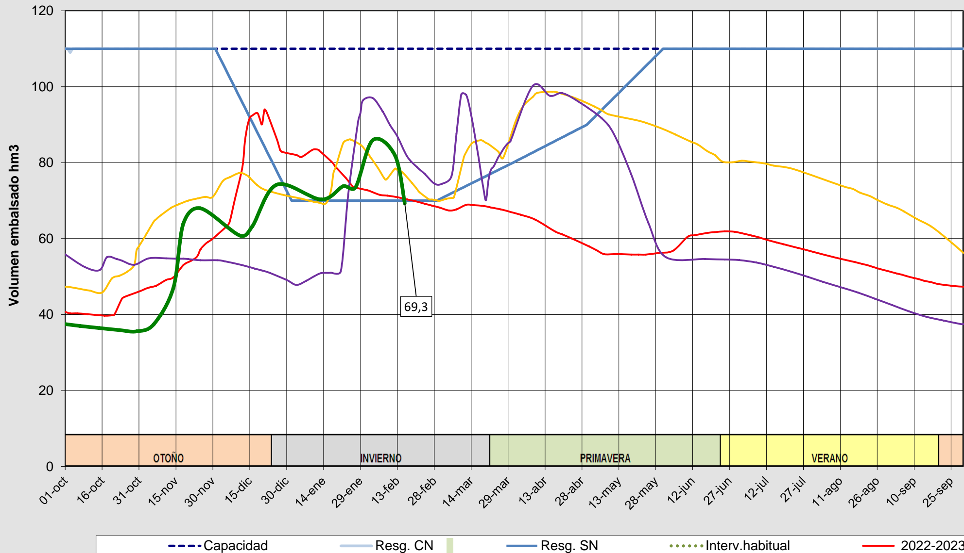
Evolución del volumen almacenado en el embalse de Irueña a fecha 16/02/2026
