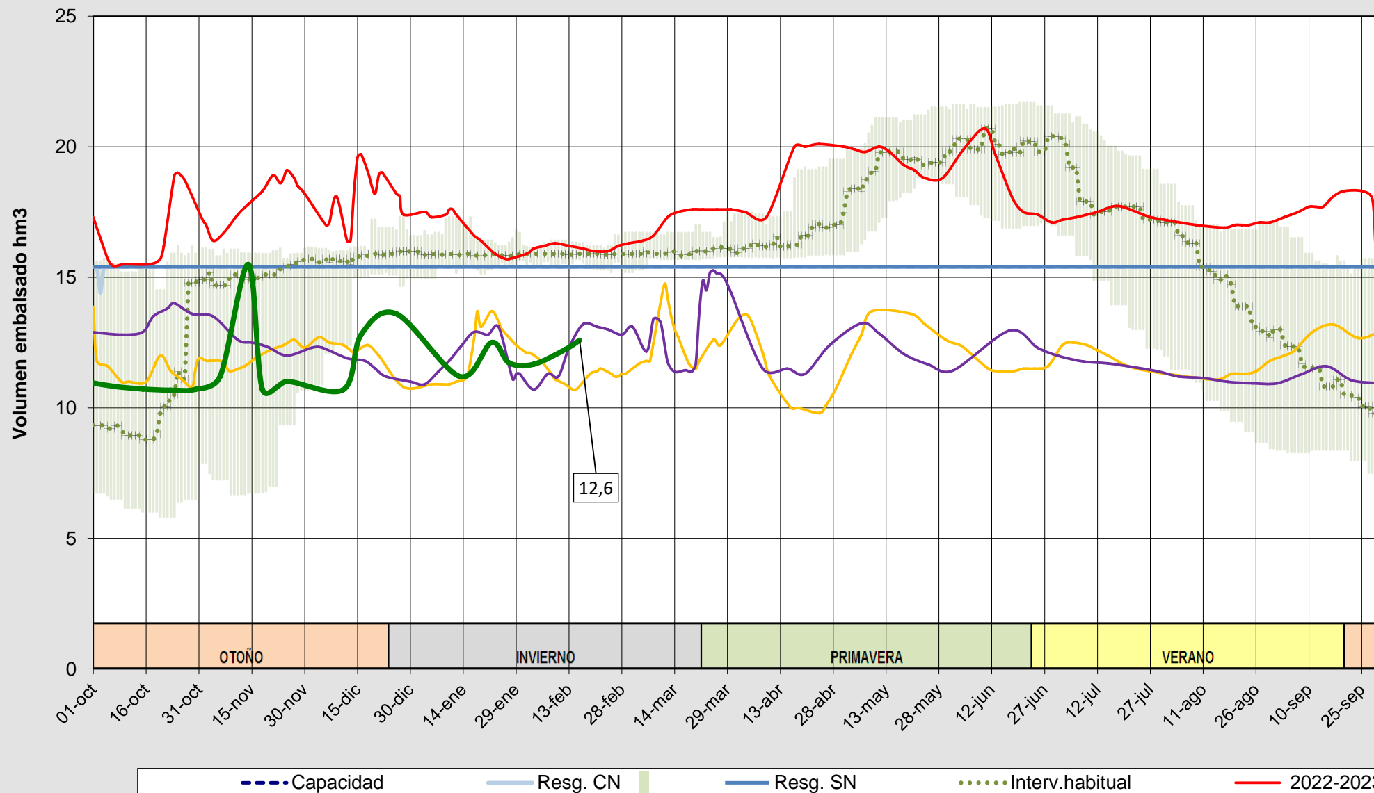
Evolución del volumen almacenado en el embalse de Águeda a fecha 16/02/2026
