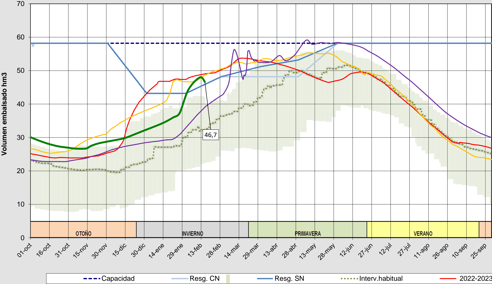
Evolución del volumen almacenado en el embalse de Las Cogotas a fecha 16/02/2026
