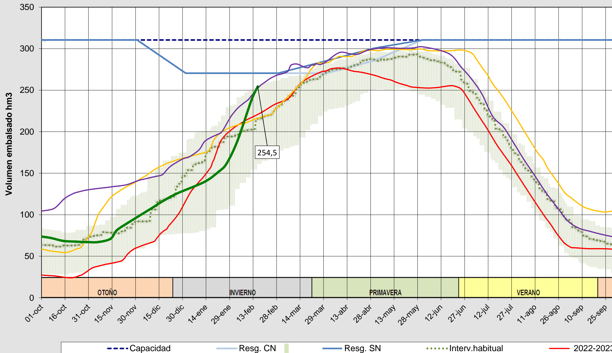
Evolución del volumen almacenado en el embalse de Barrios de Luna a fecha 16/02/2026
