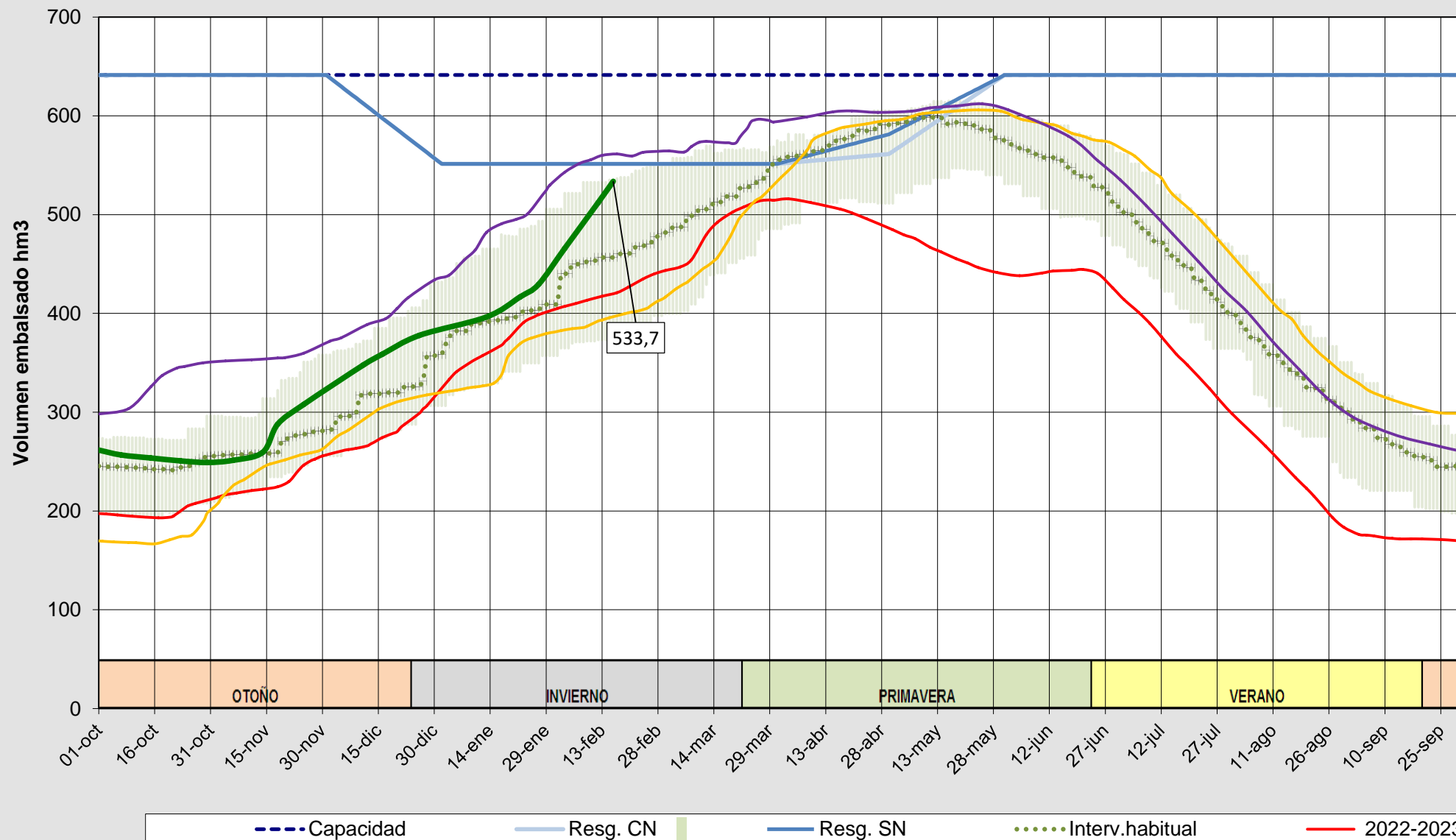
Evolución del volumen almacenado en el embalse de Riaño a fecha 16/02/2026
