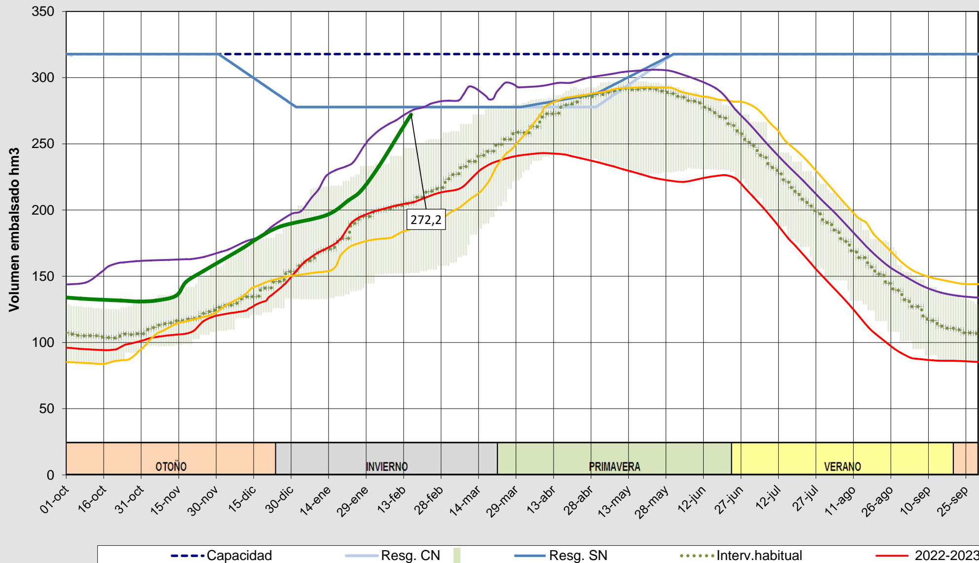
Evolución del volumen almacenado en el embalse de Porma a fecha 16/02/2026
