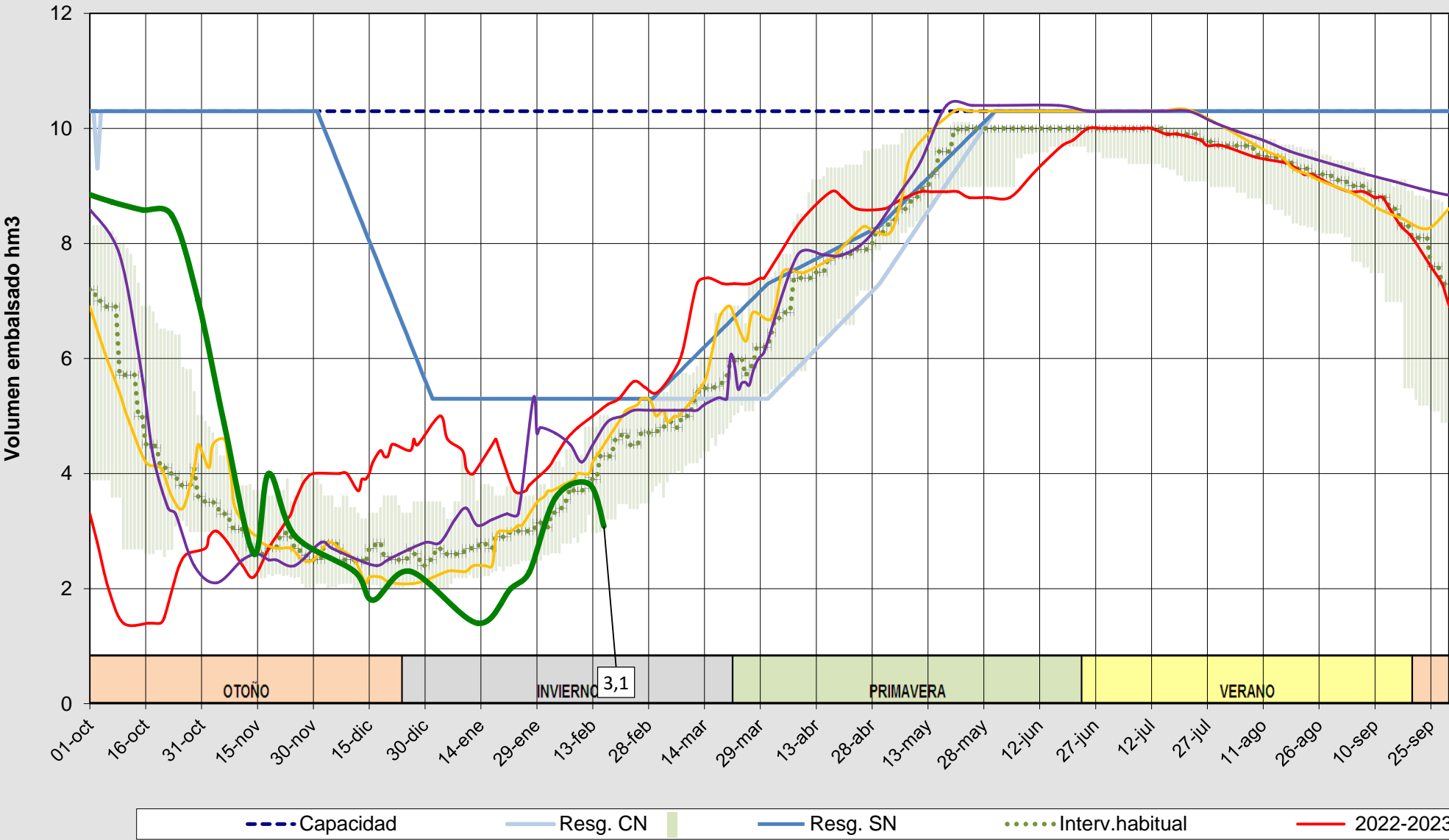
Evolución del volumen almacenado en el embalse de Cervera a fecha 16/02/2026
