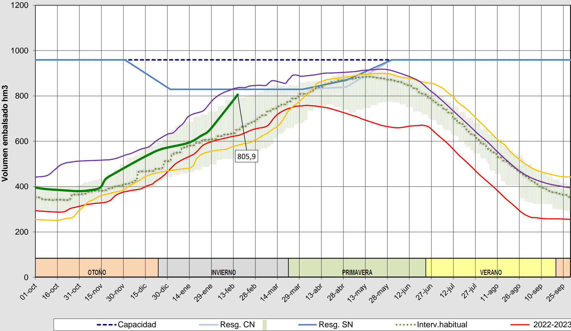
Evolución del volumen almacenado en el sistema del PORMA-ESLA a fecha 16/02/2026
