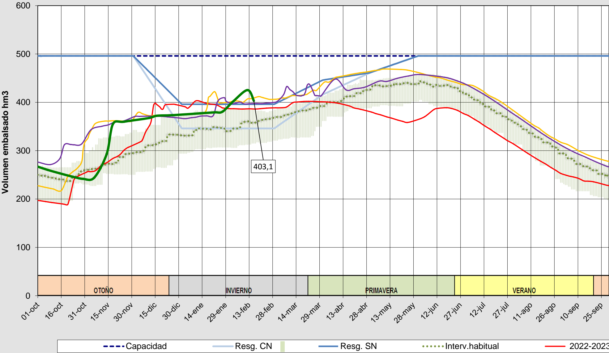
Evolución del volumen almacenado en el embalse de Santa Teresa a fecha 16/02/2026
