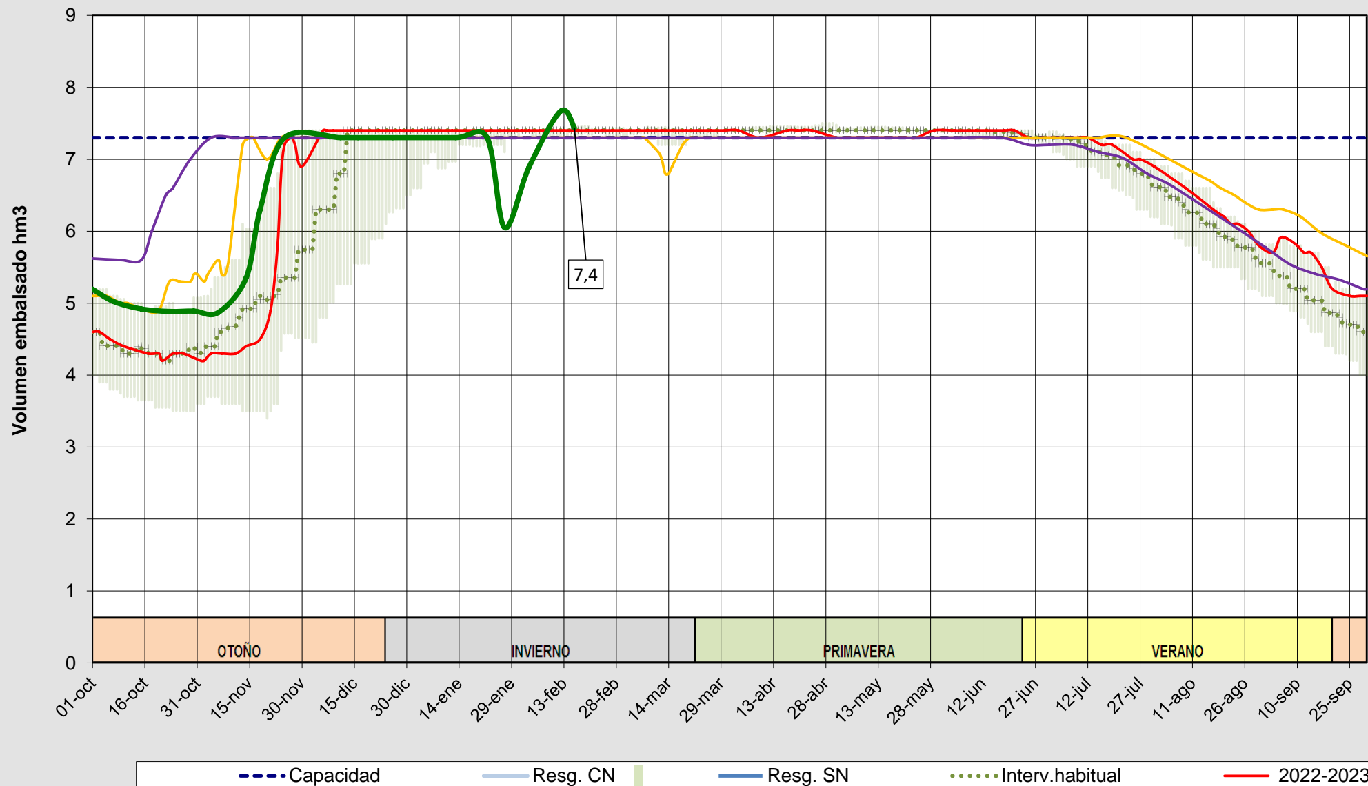
Evolución del volumen almacenado en el embalse de Pontón Alto a fecha 16/02/2026
