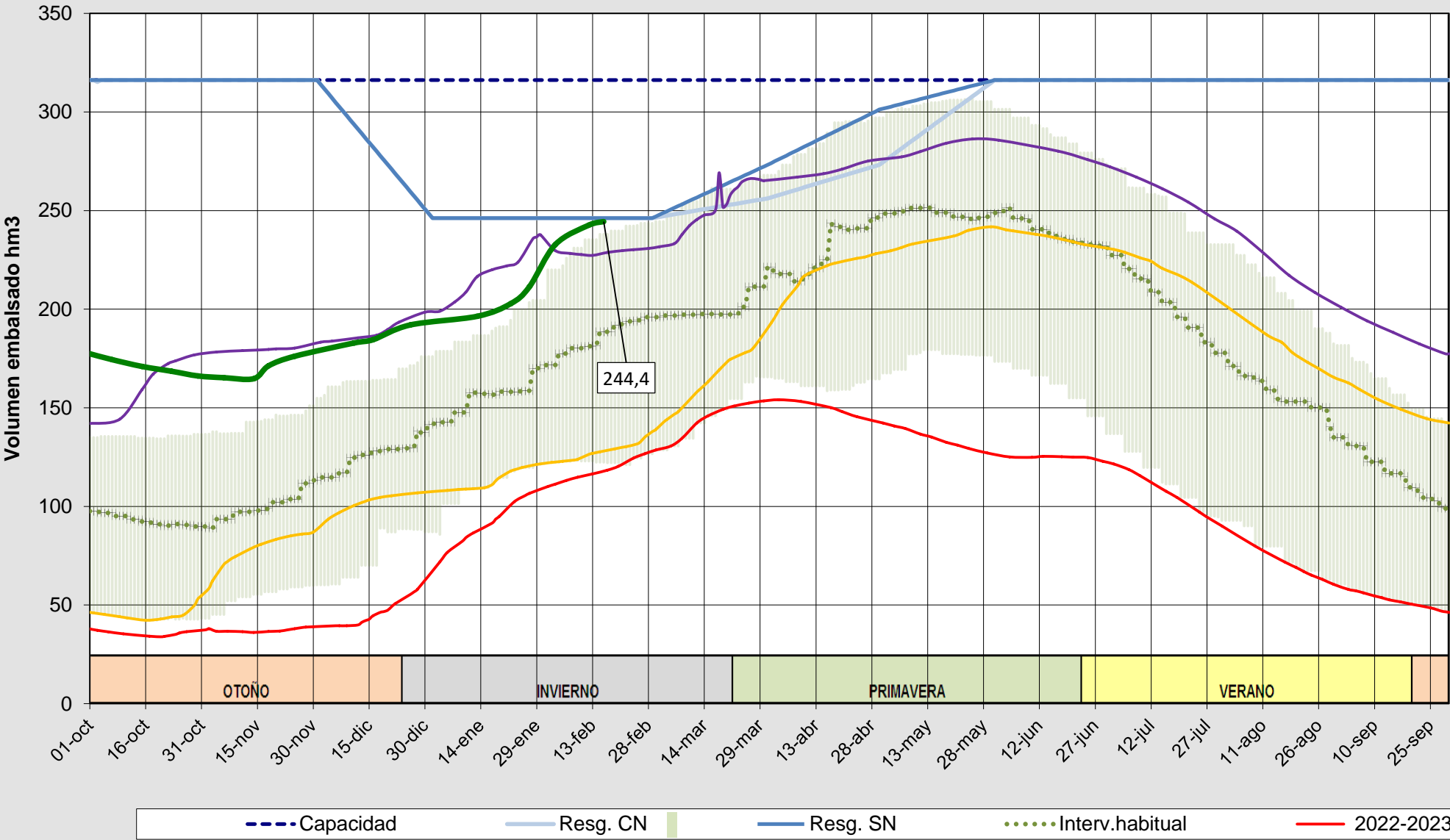
Evolución del volumen almacenado en el sistema del PISUERGA a fecha 16/02/2026
