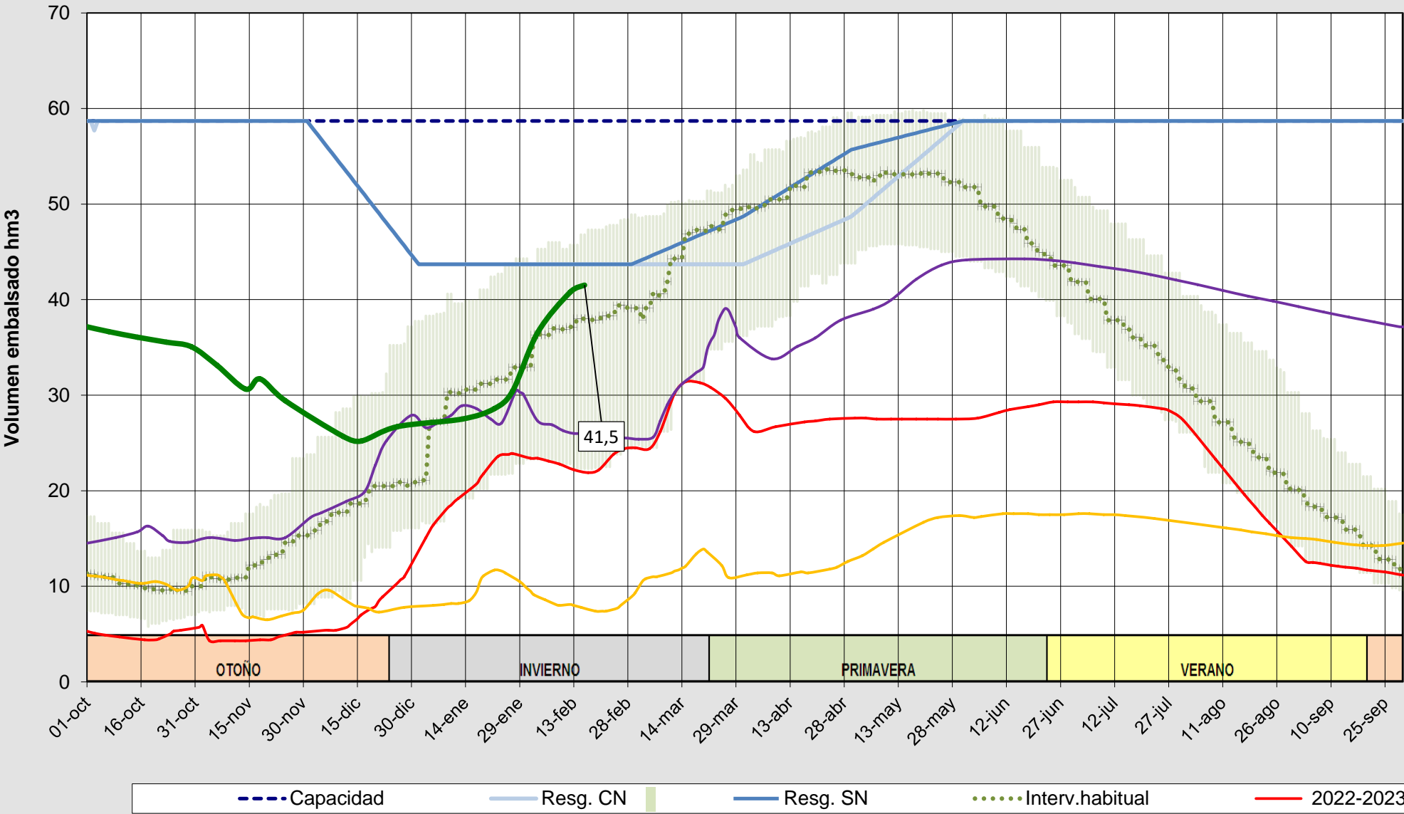
Evolución del volumen almacenado en el embalse de Requejada a fecha 16/02/2026
