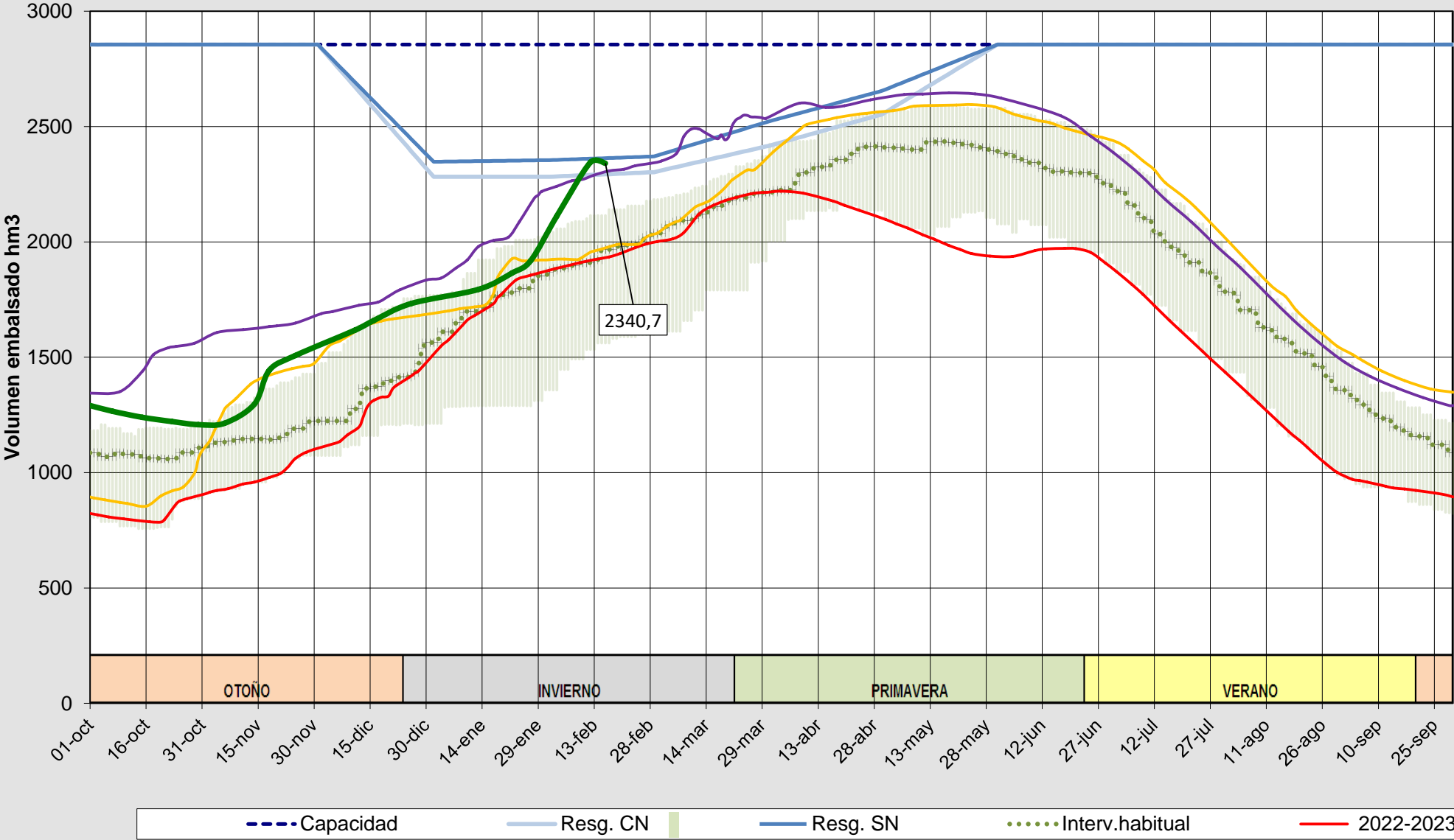
Evolución del volumen almacenado en el sistema del DUERO (ESTADO) a fecha 16/02/2026
