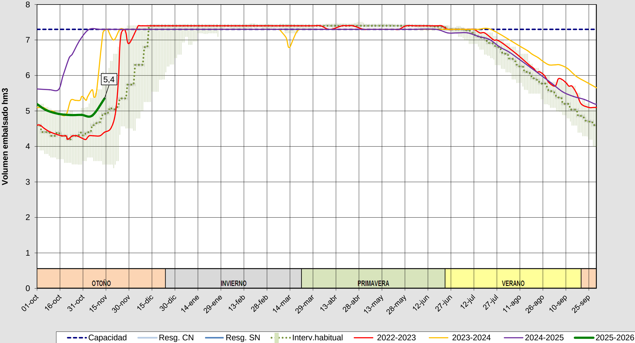
Evolución del volumen almacenado en el embalse de Pontón Alto a fecha 14/11/2025
