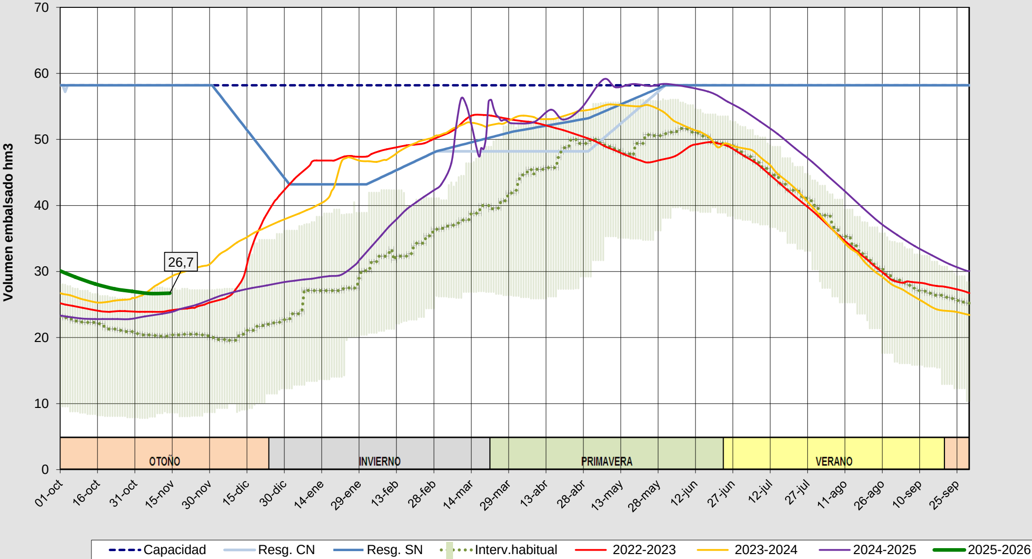
Evolución del volumen almacenado en el embalse de Las Cogotas a fecha 14/11/2025
