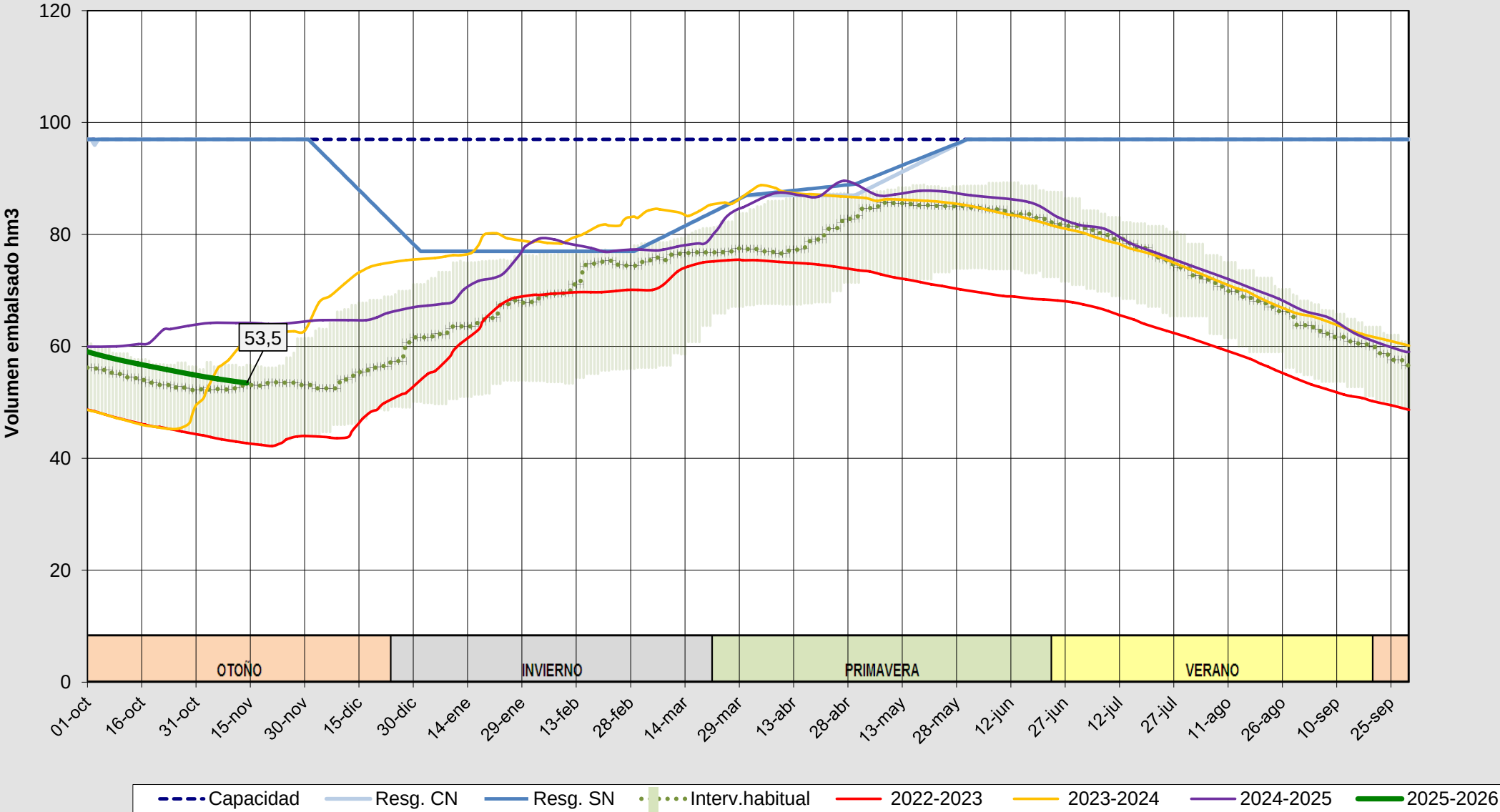
Evolución del volumen almacenado en el sistema del ARLANZÓN a fecha 14/11/2025
