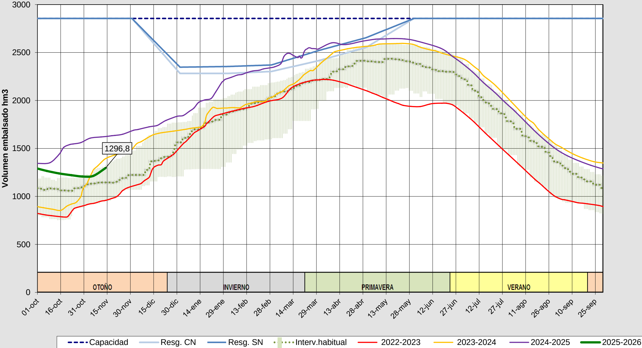
Evolución del volumen almacenado en el sistema del DUERO (ESTADO) a fecha 14/11/2025
