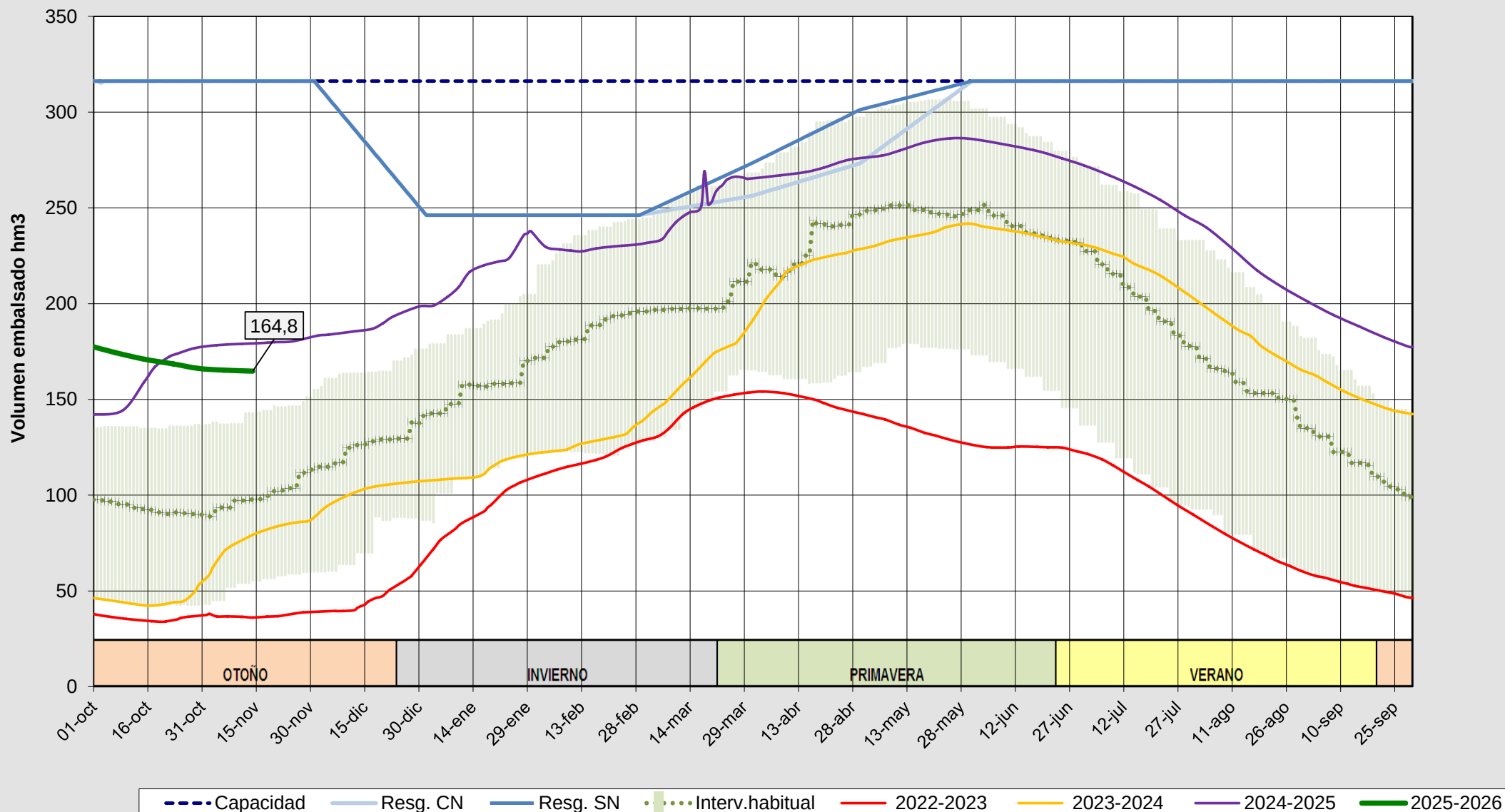
Evolución del volumen almacenado en el sistema del PISUERGA a fecha 14/11/2025
