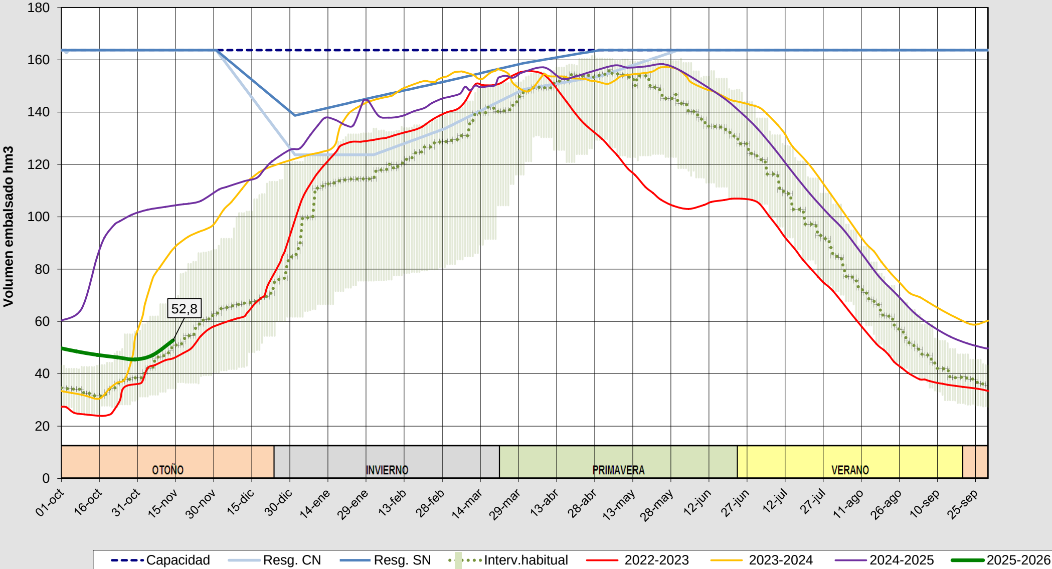
Evolución del volumen almacenado en el sistema del CARRIÓN a fecha 14/11/2025
