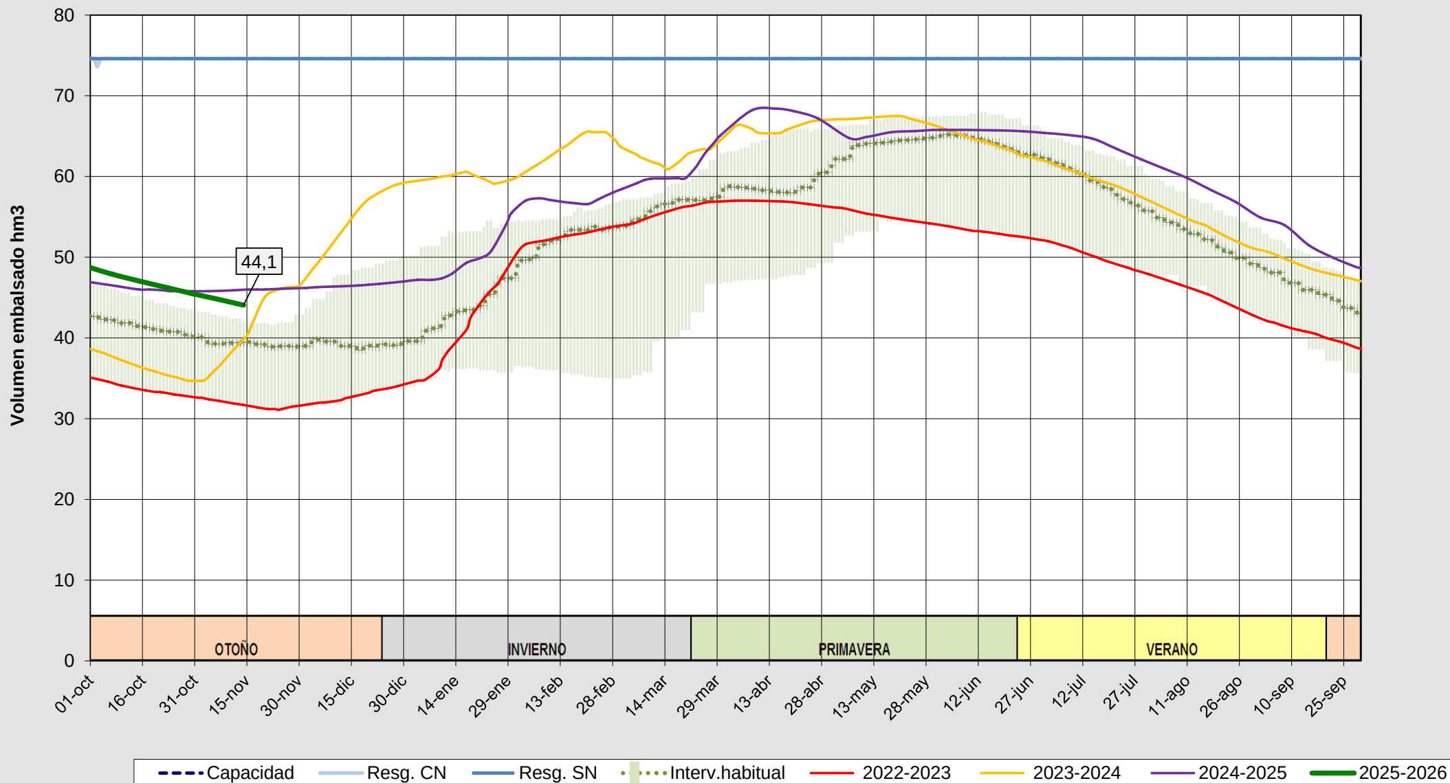
Evolución del volumen almacenado en el embalse de Úzquiza a fecha 14/11/2025
