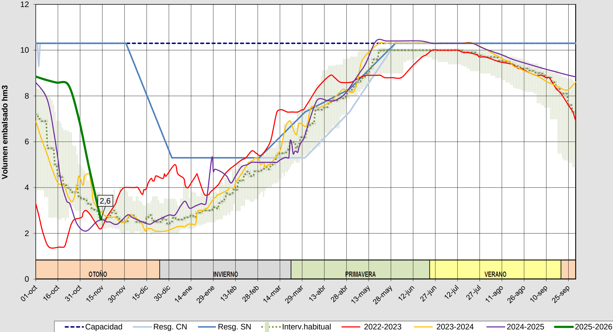
Evolución del volumen almacenado en el embalse de Cervera a fecha 14/11/2025
