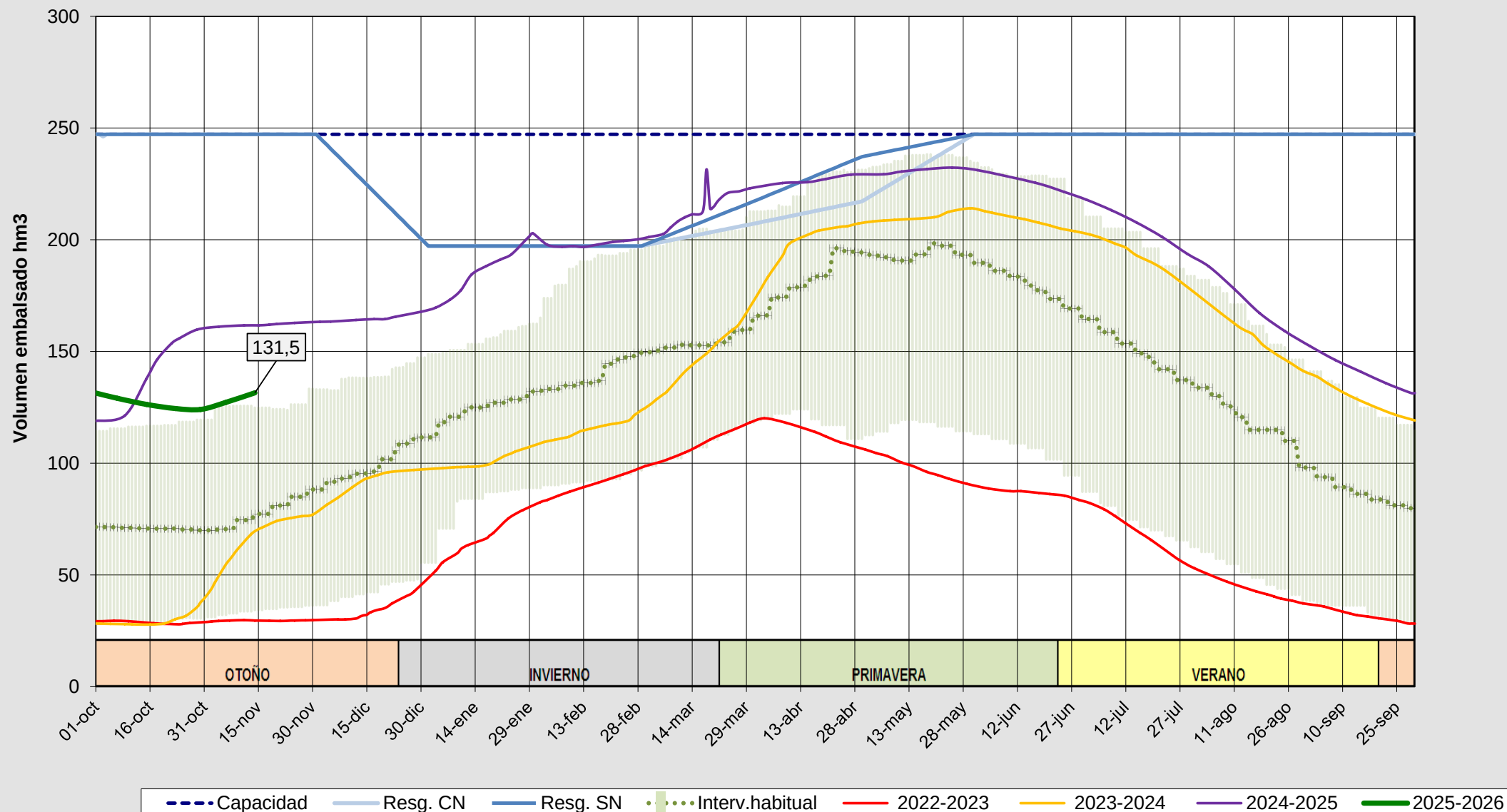
Evolución del volumen almacenado en el embalse de Aguilar a fecha 14/11/2025
