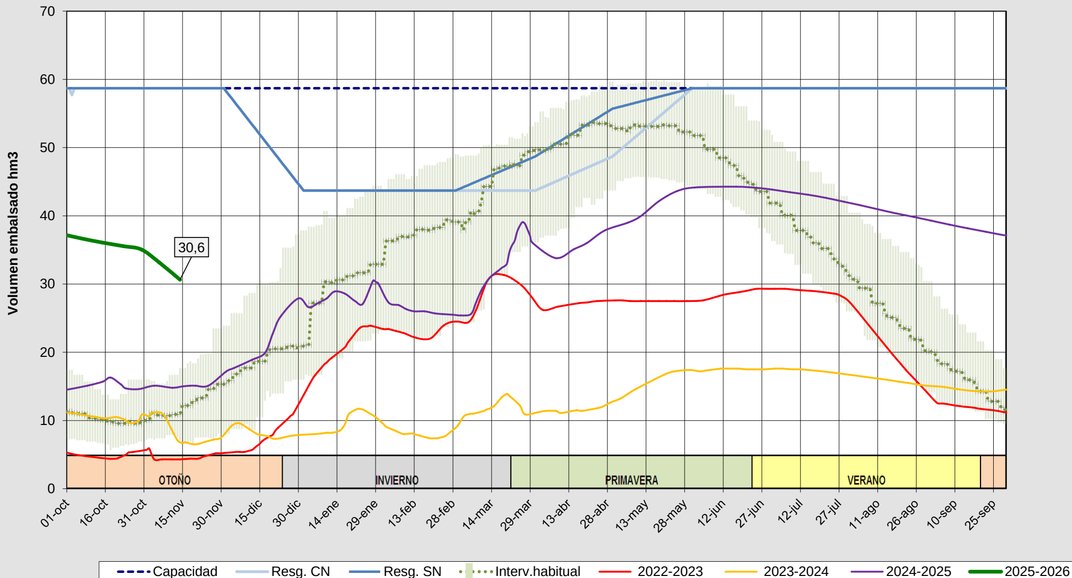
Evolución del volumen almacenado en el embalse de Requejada a fecha 14/11/2025
