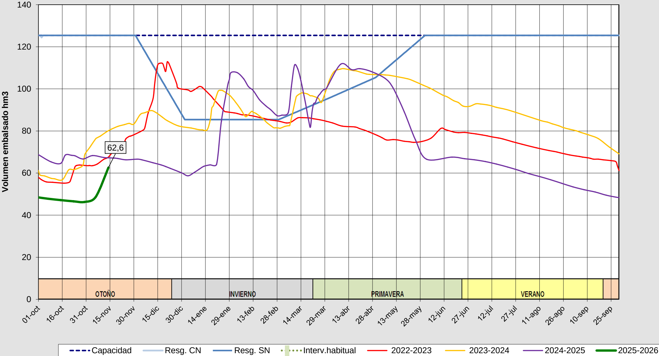
Evolución del volumen almacenado en el sistema del ÁGUEDA a fecha 14/11/2025
