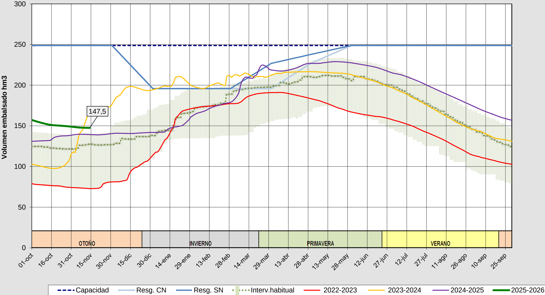
Evolución del volumen almacenado en el embalse de Cuerda del Pozo a fecha 14/11/2025
