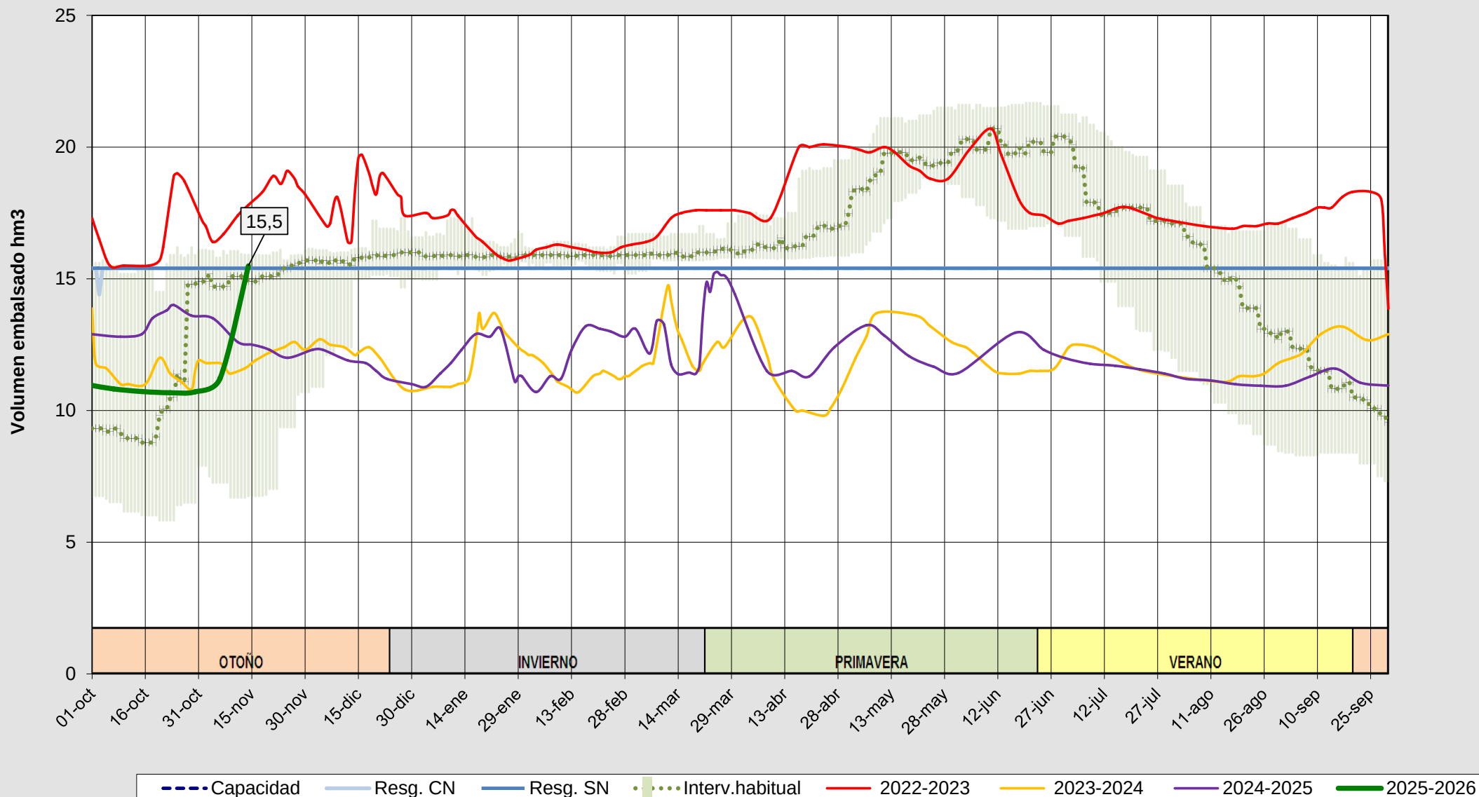
Evolución del volumen almacenado en el embalse de Águeda a fecha 14/11/2025
