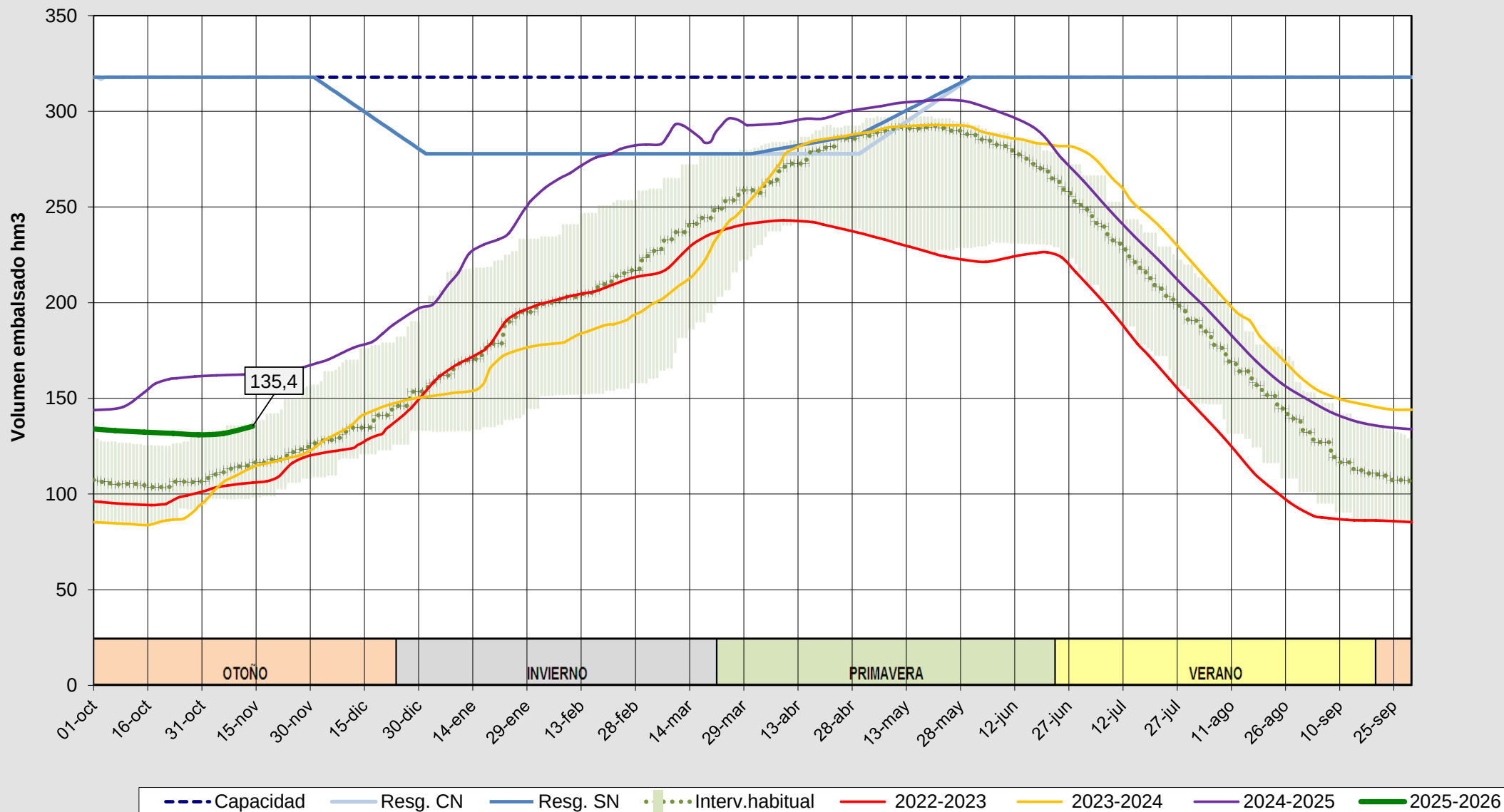
Evolución del volumen almacenado en el embalse de Porma a fecha 14/11/2025
