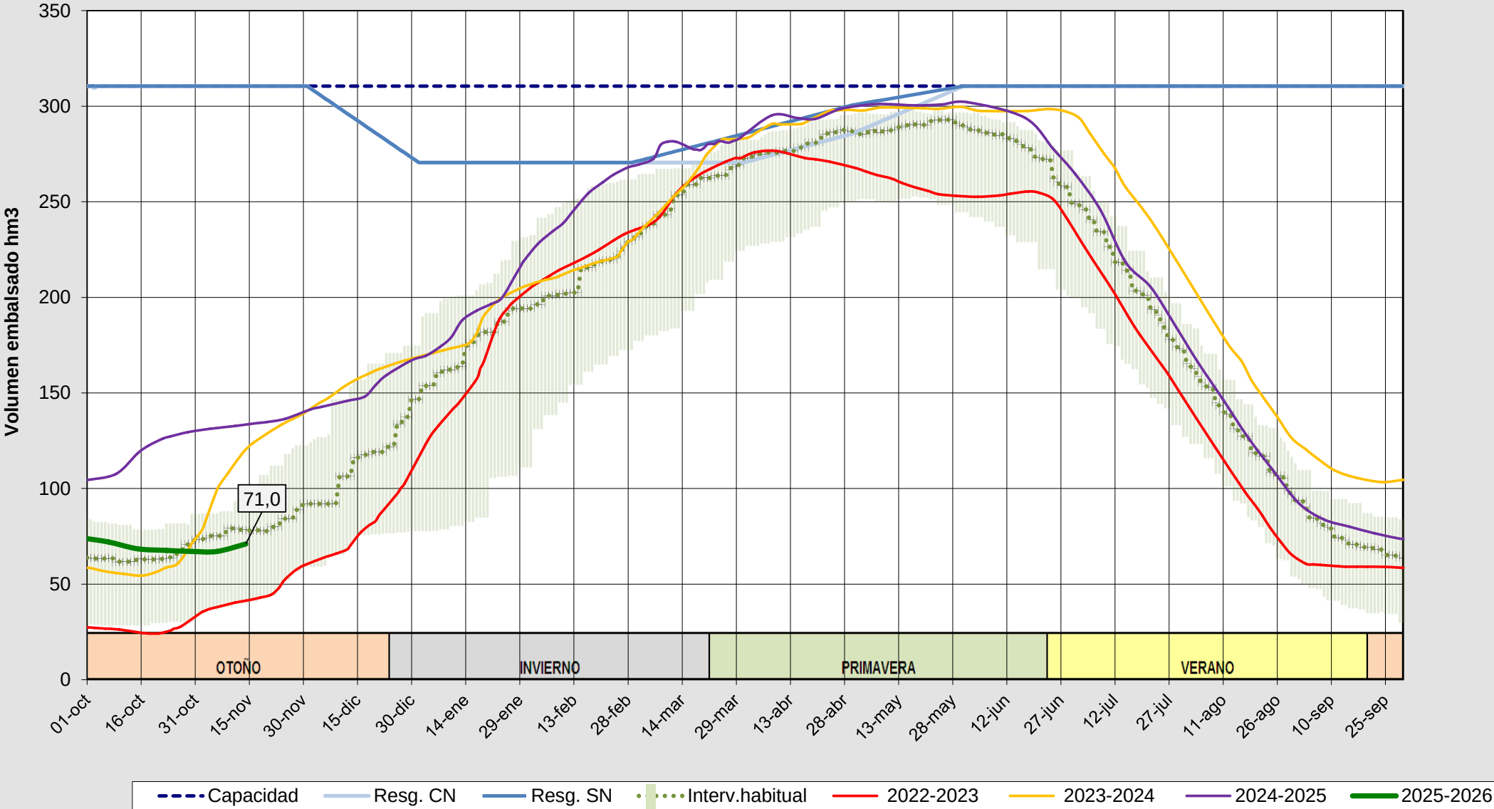
Evolución del volumen almacenado en el embalse de Barrios de Luna a fecha 14/11/2025
