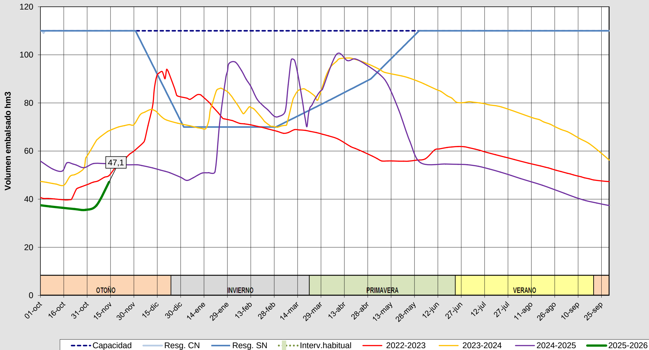
Evolución del volumen almacenado en el embalse de Iruña a fecha 14/11/2025
