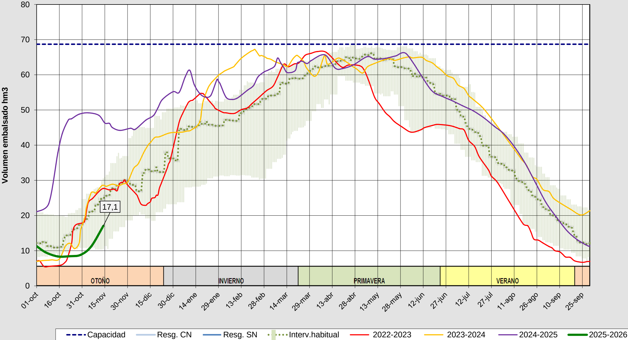
Evolución del volumen almacenado en el embalse de Camporredondo a fecha 14/11/2025
