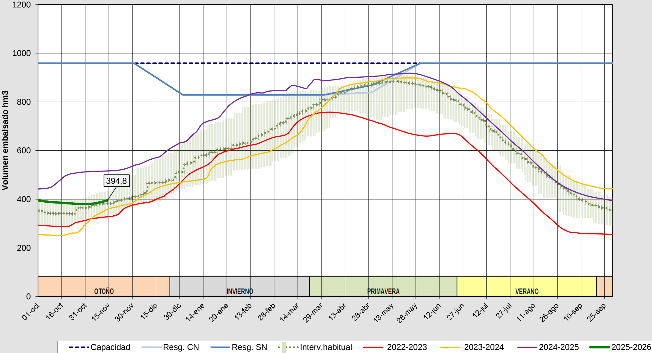
Evolución del volumen almacenado en el sistema del PORMA-ESLA a fecha 14/11/2025
