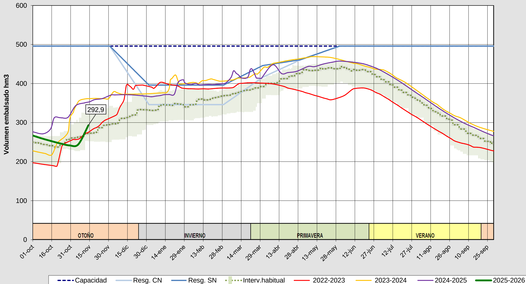
Evolución del volumen almacenado en el embalse de Santa Teresa a fecha 14/11/2025
