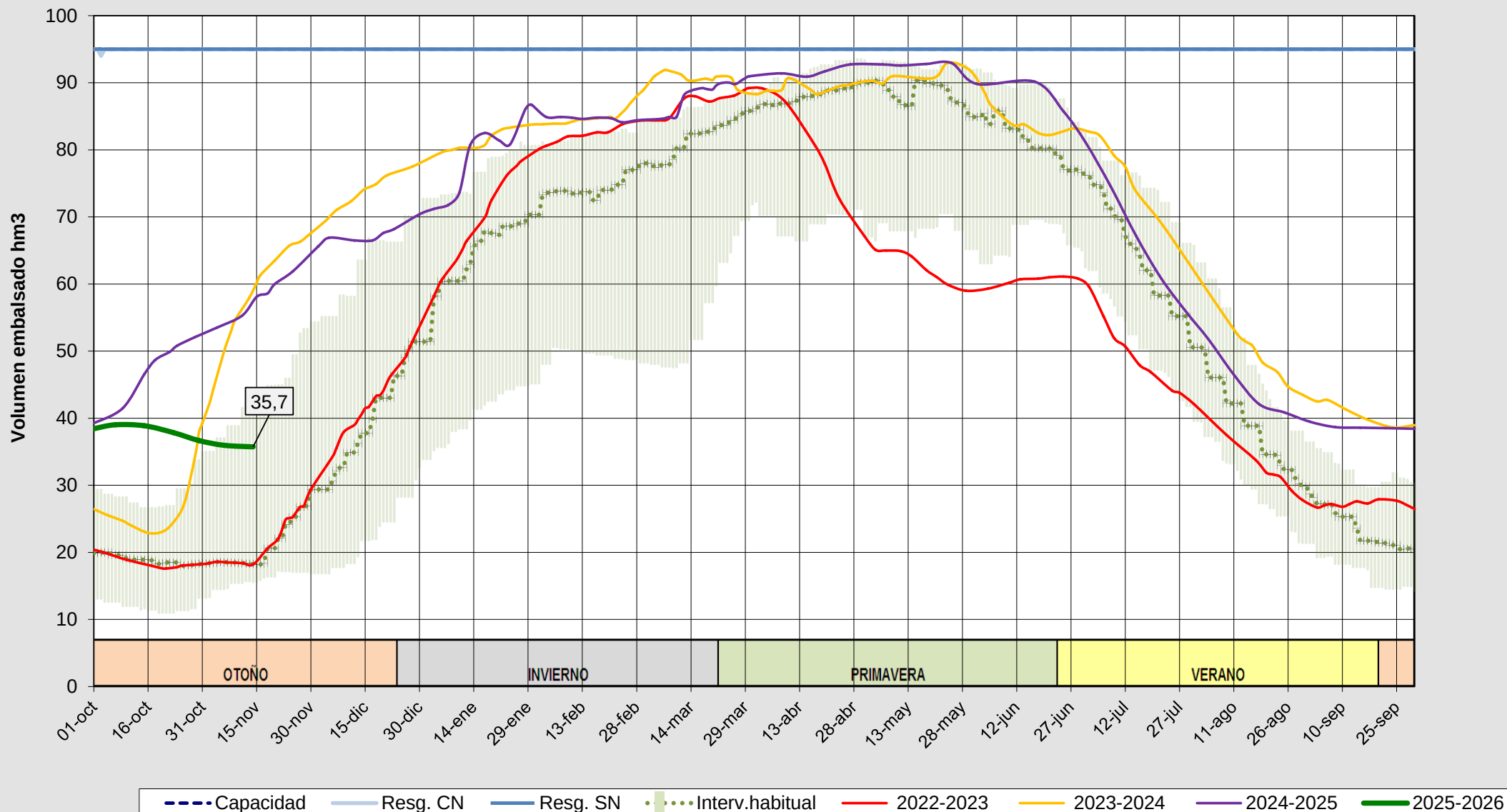
Evolución del volumen almacenado en el embalse de Compuerto a fecha 14/11/2025
