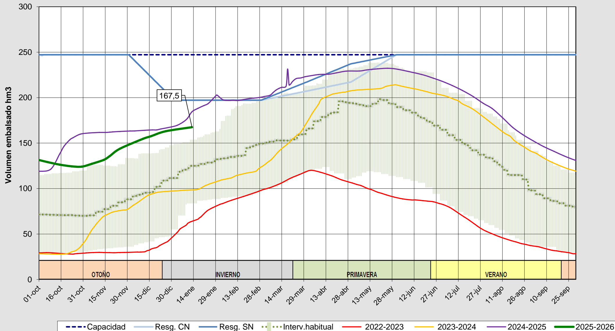
Evolución del volumen almacenado en el embalse de Aguilar a fecha 13/01/2026
