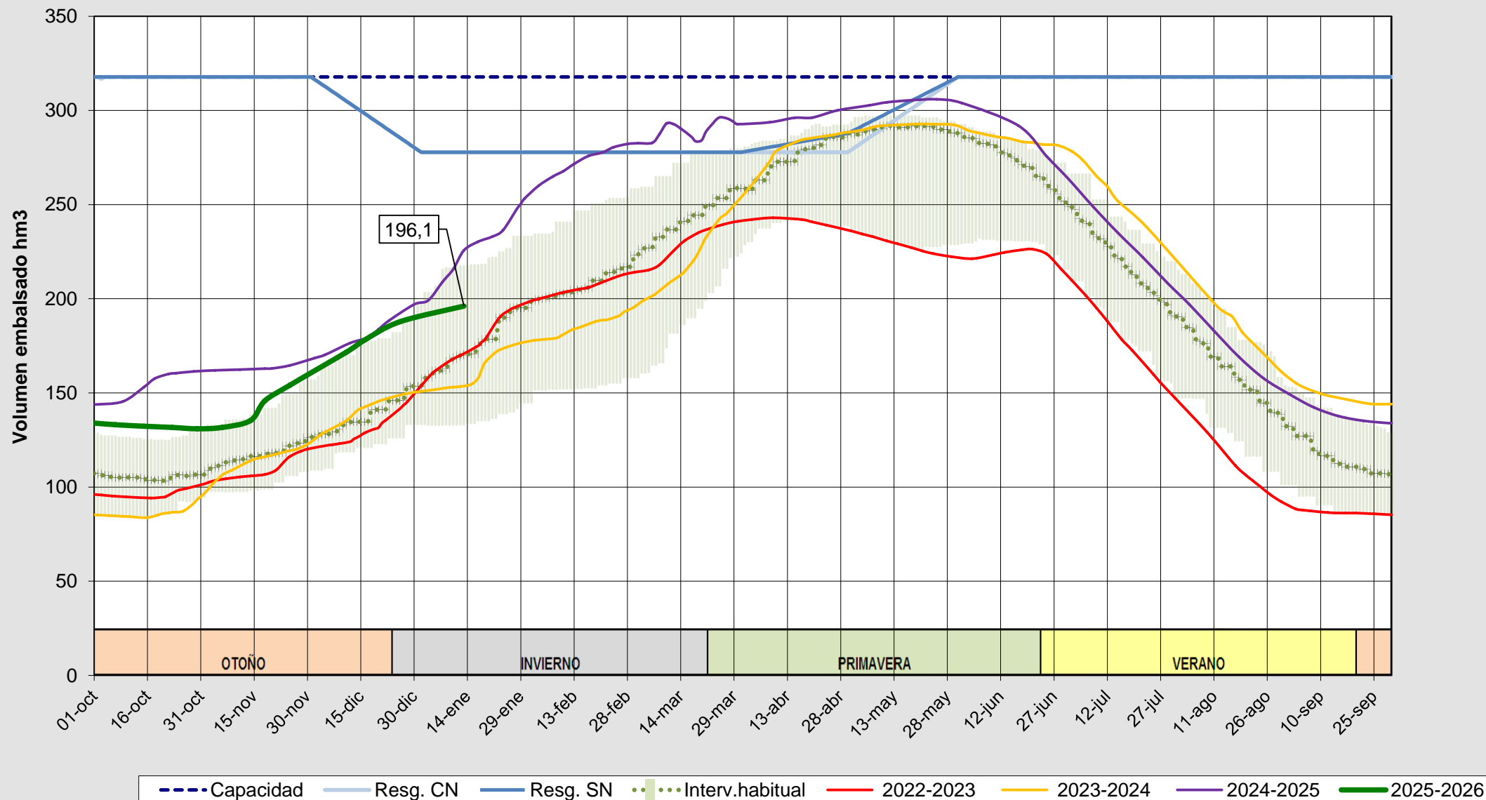
Evolución del volumen almacenado en el embalse de Porma a fecha 13/01/2026
