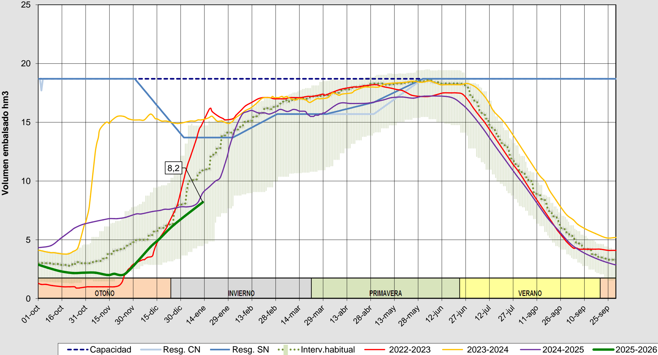
Evolución del volumen almacenado en el embalse de Villameca a fecha 13/01/2026
