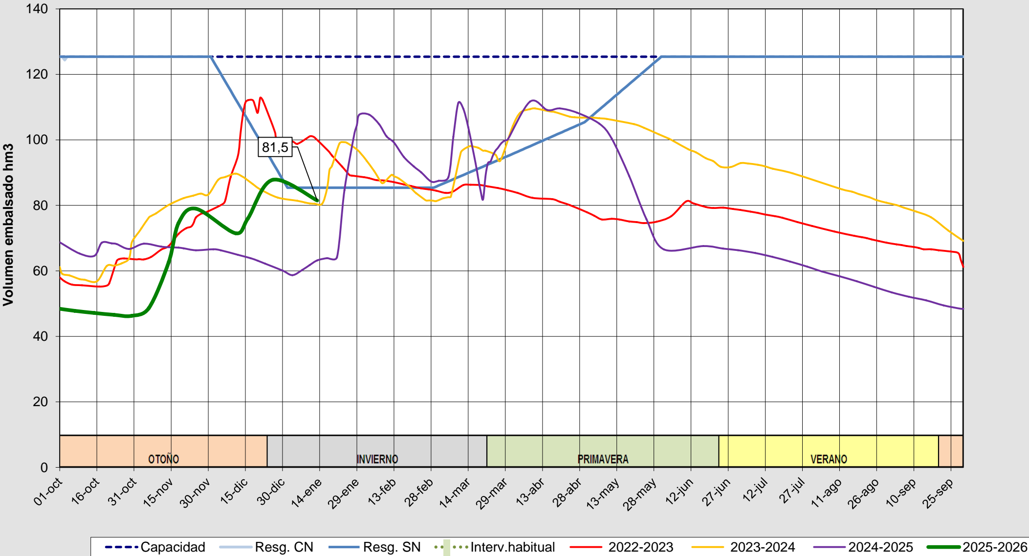
Evolución del volumen almacenado en el sistema del ÁGUEDA a fecha 13/01/2026
