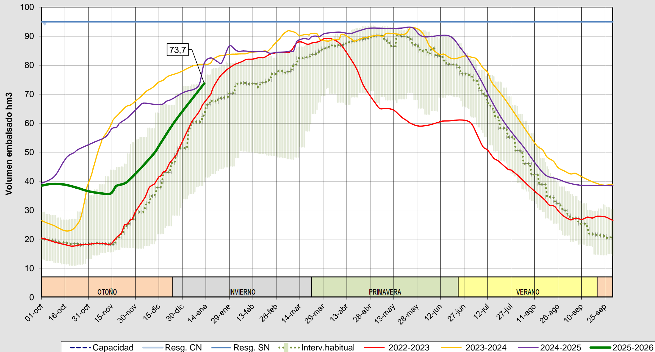
Evolución del volumen almacenado en el embalse de Compuerto a fecha 13/01/2026
