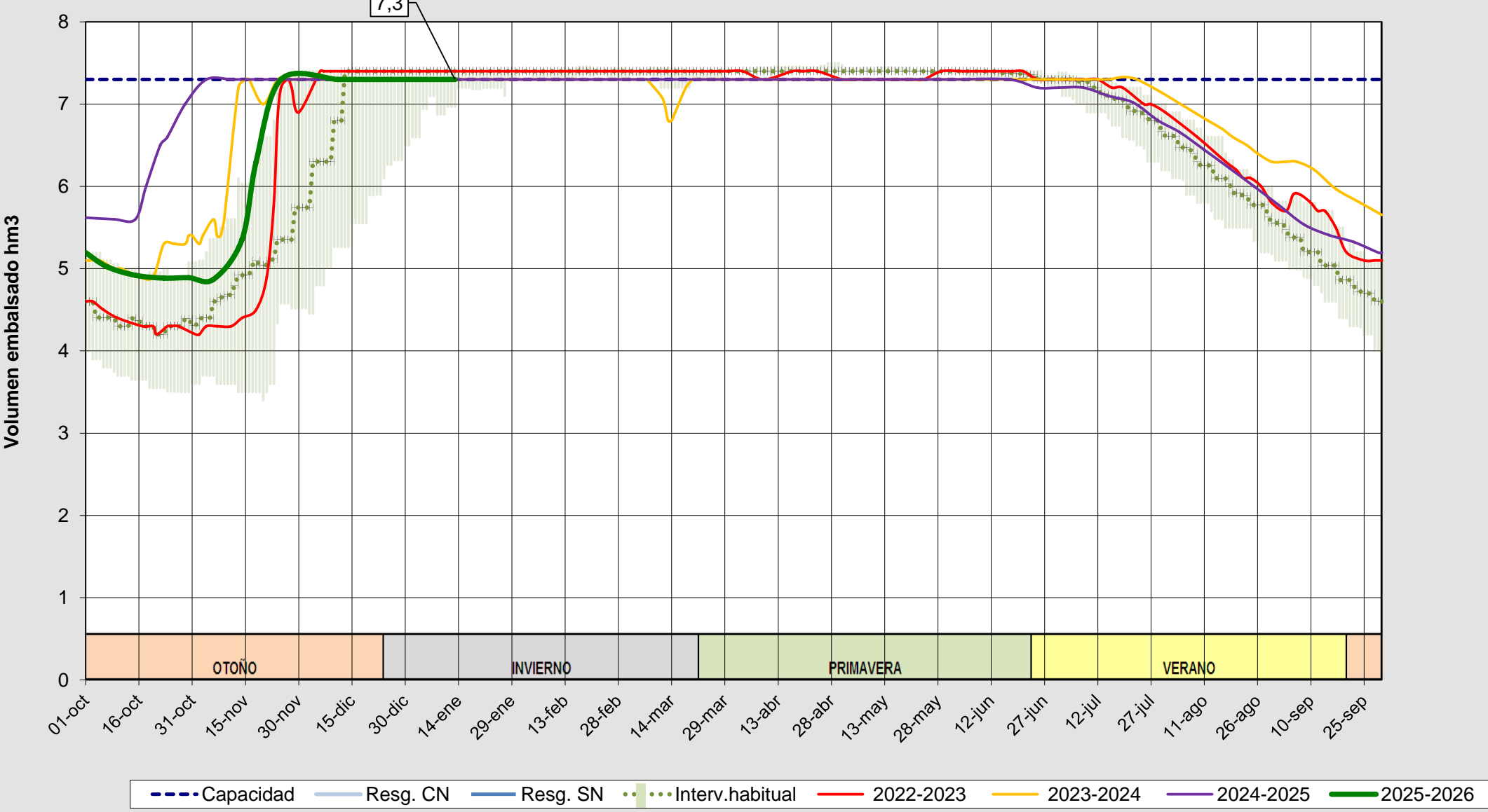
Evolución del volumen almacenado en el embalse de Pontón Alto a fecha 13/01/2026
