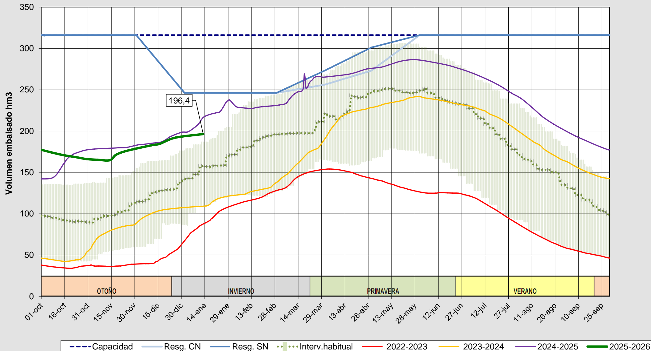
Evolución del volumen almacenado en el sistema del PISUERGA a fecha 13/01/2026
