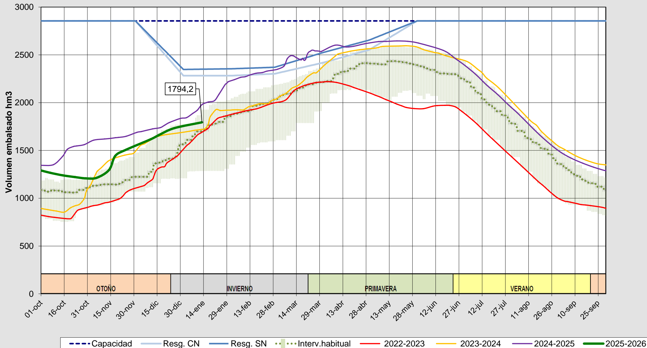
Evolución del volumen almacenado en el sistema del DUERO (ESTADO) a fecha 13/01/2026
