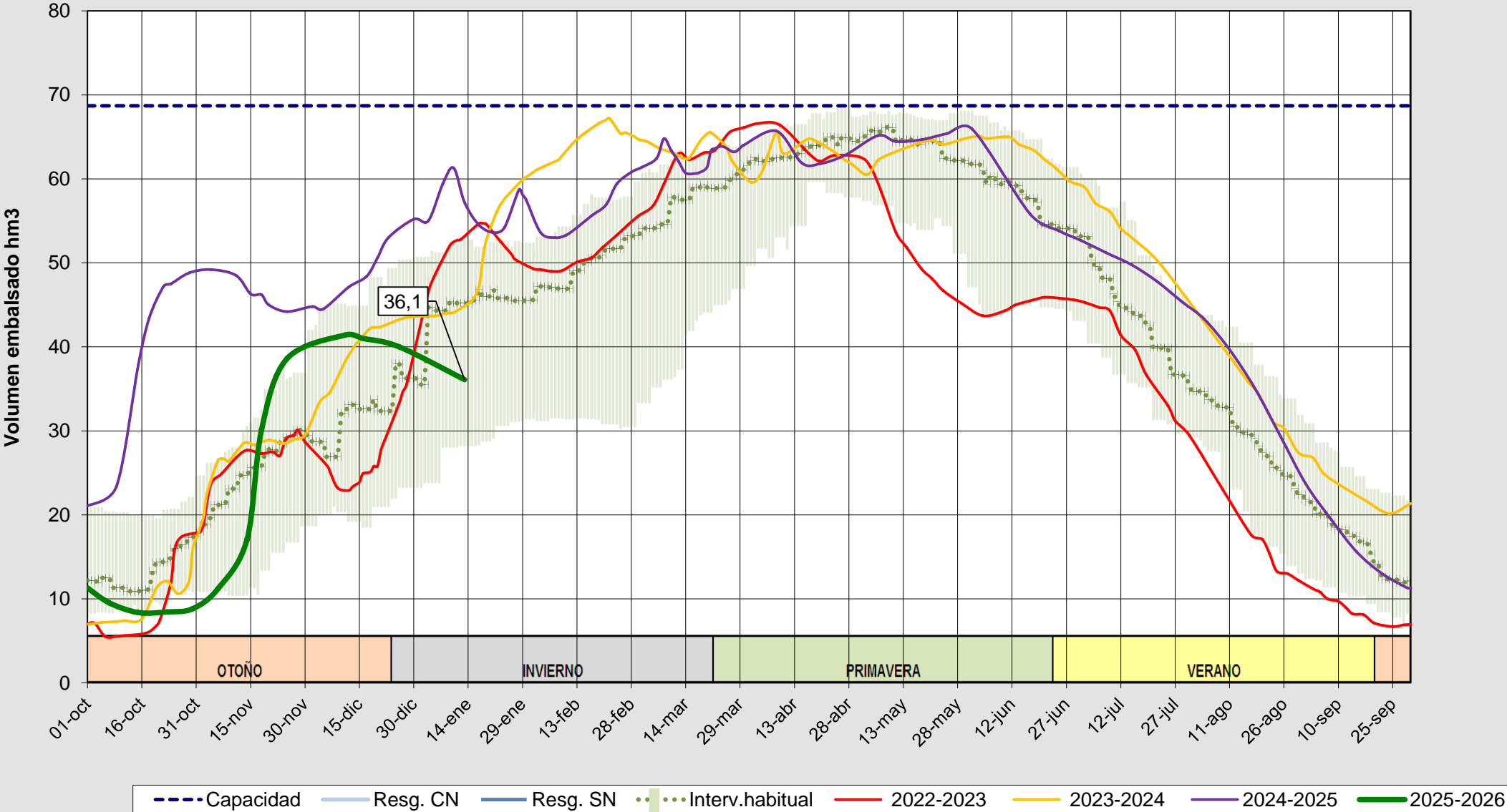
Evolución del volumen almacenado en el embalse de Camporredondo a fecha 13/01/2026
