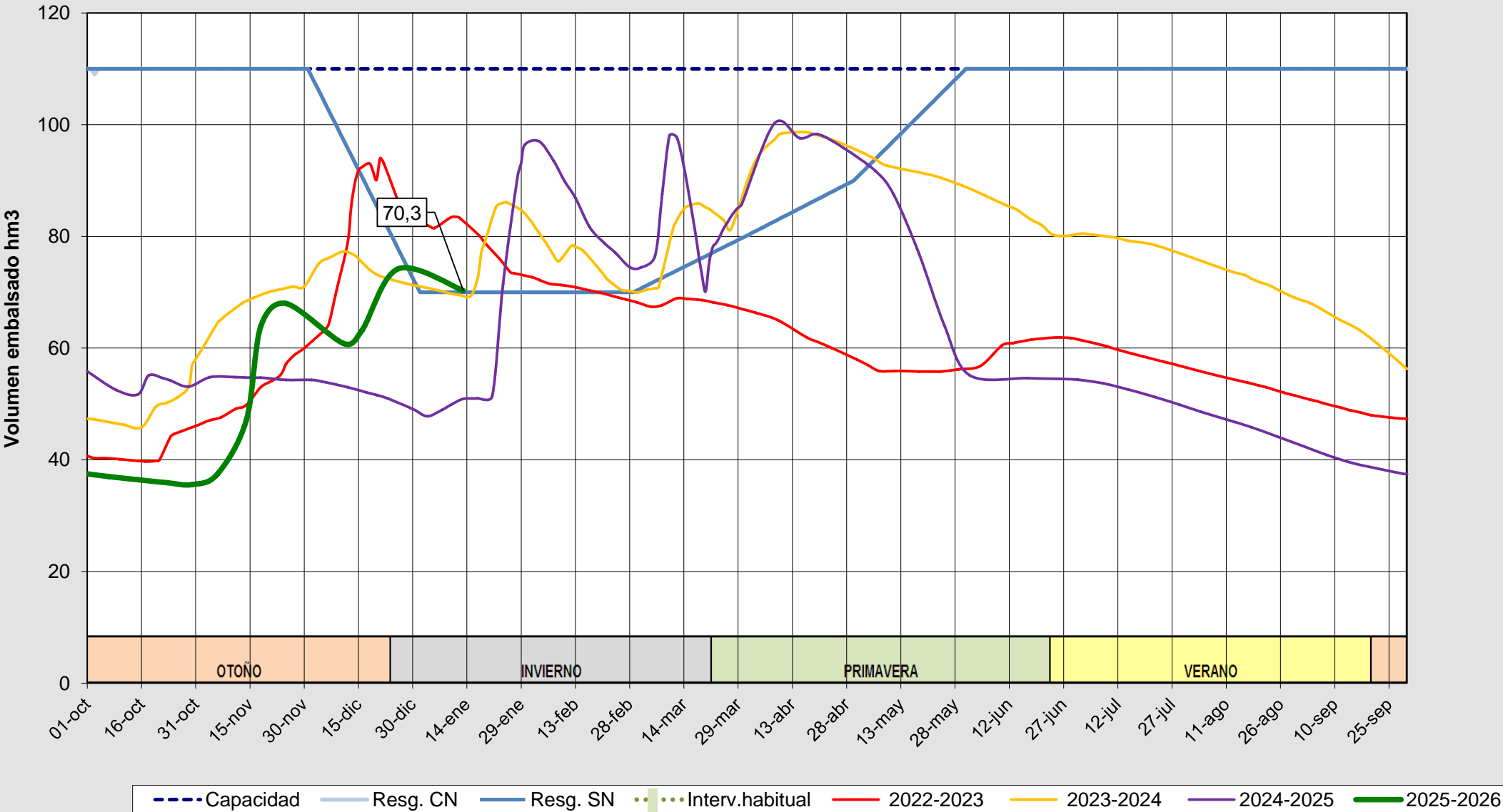
Evolución del volumen almacenado en el embalse de Irueña a fecha 13/01/2026
