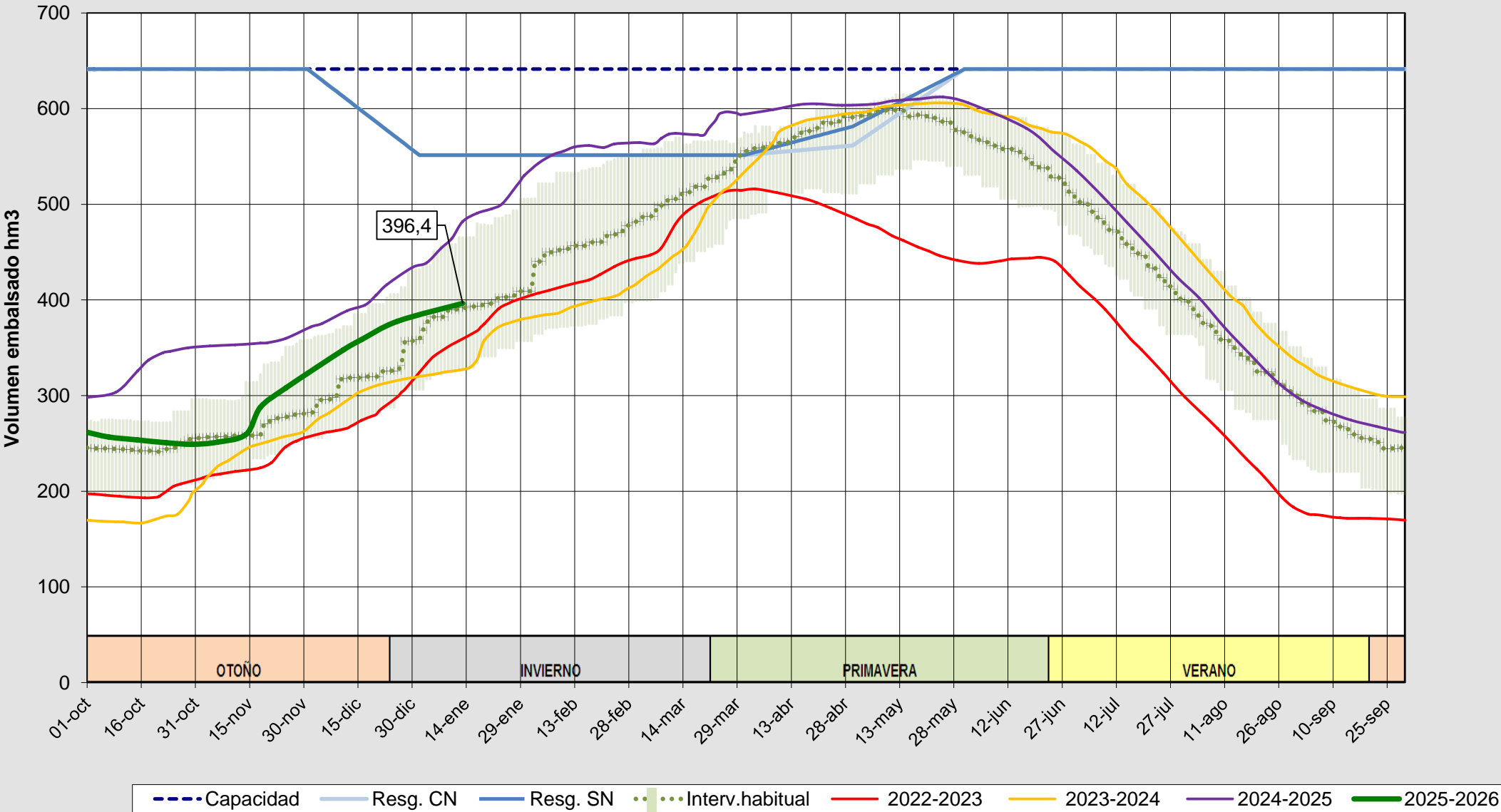
Evolución del volumen almacenado en el embalse de Riaño a fecha 13/01/2026
