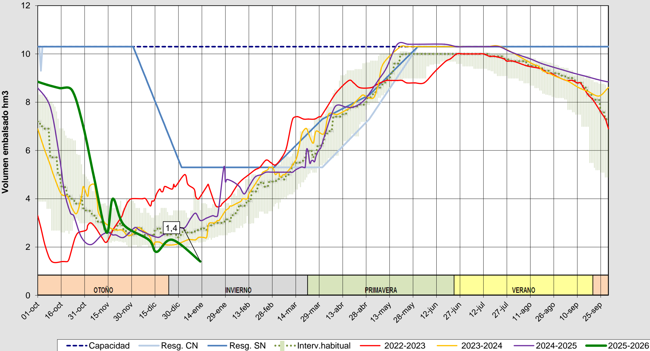
Evolución del volumen almacenado en el embalse de Cervera a fecha 13/01/2026
