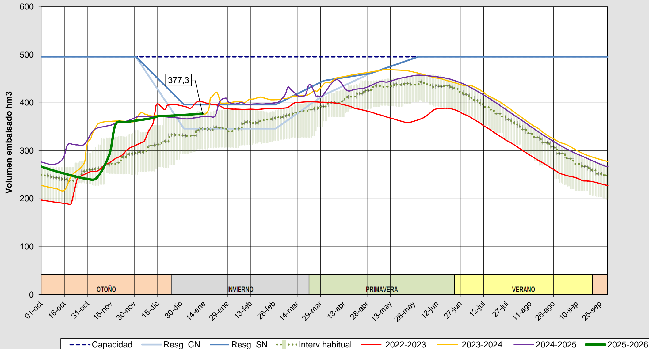
Evolución del volumen almacenado en el embalse de Santa Teresa a fecha 13/01/2026
