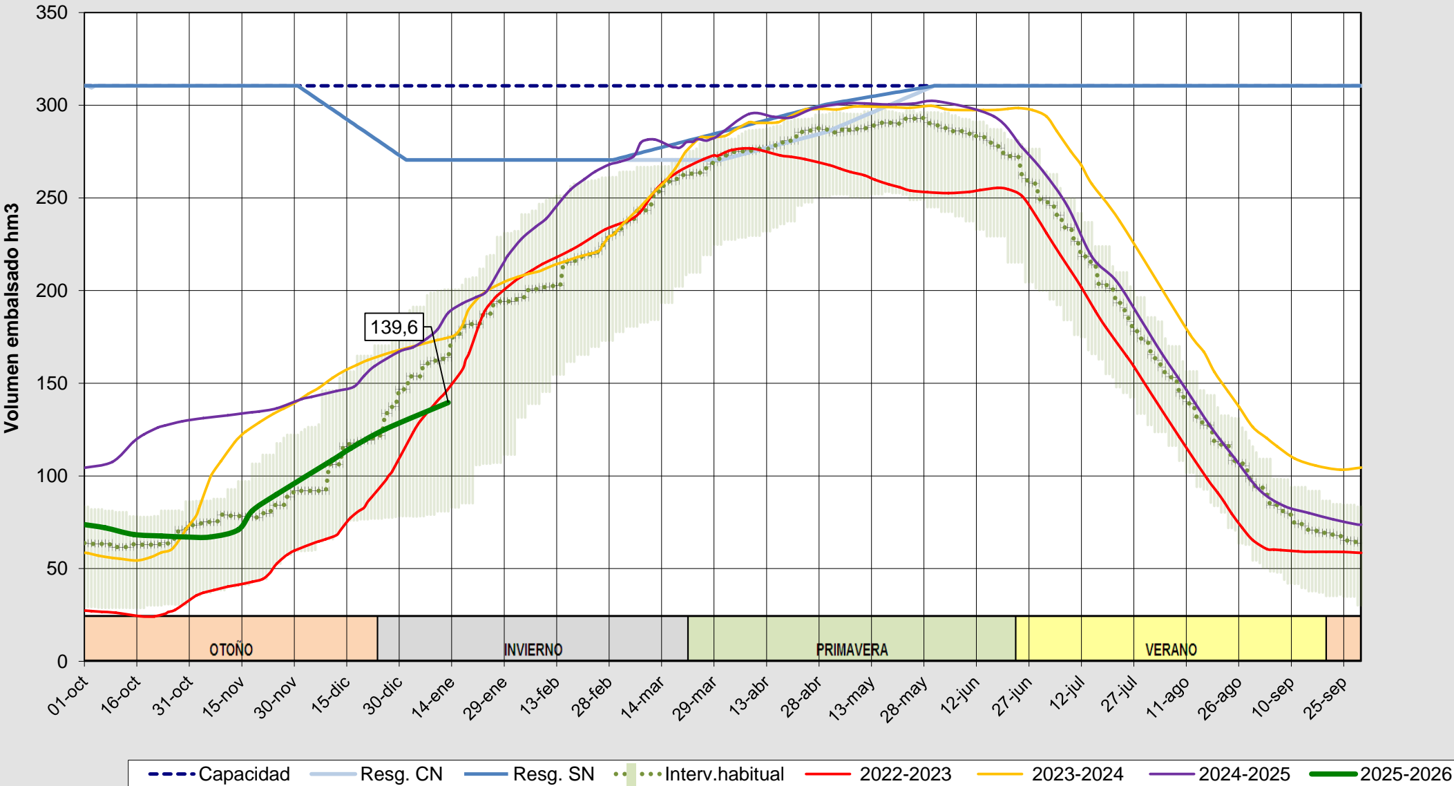
Evolución del volumen almacenado en el embalse de Barrios de Luna a fecha 13/01/2026
