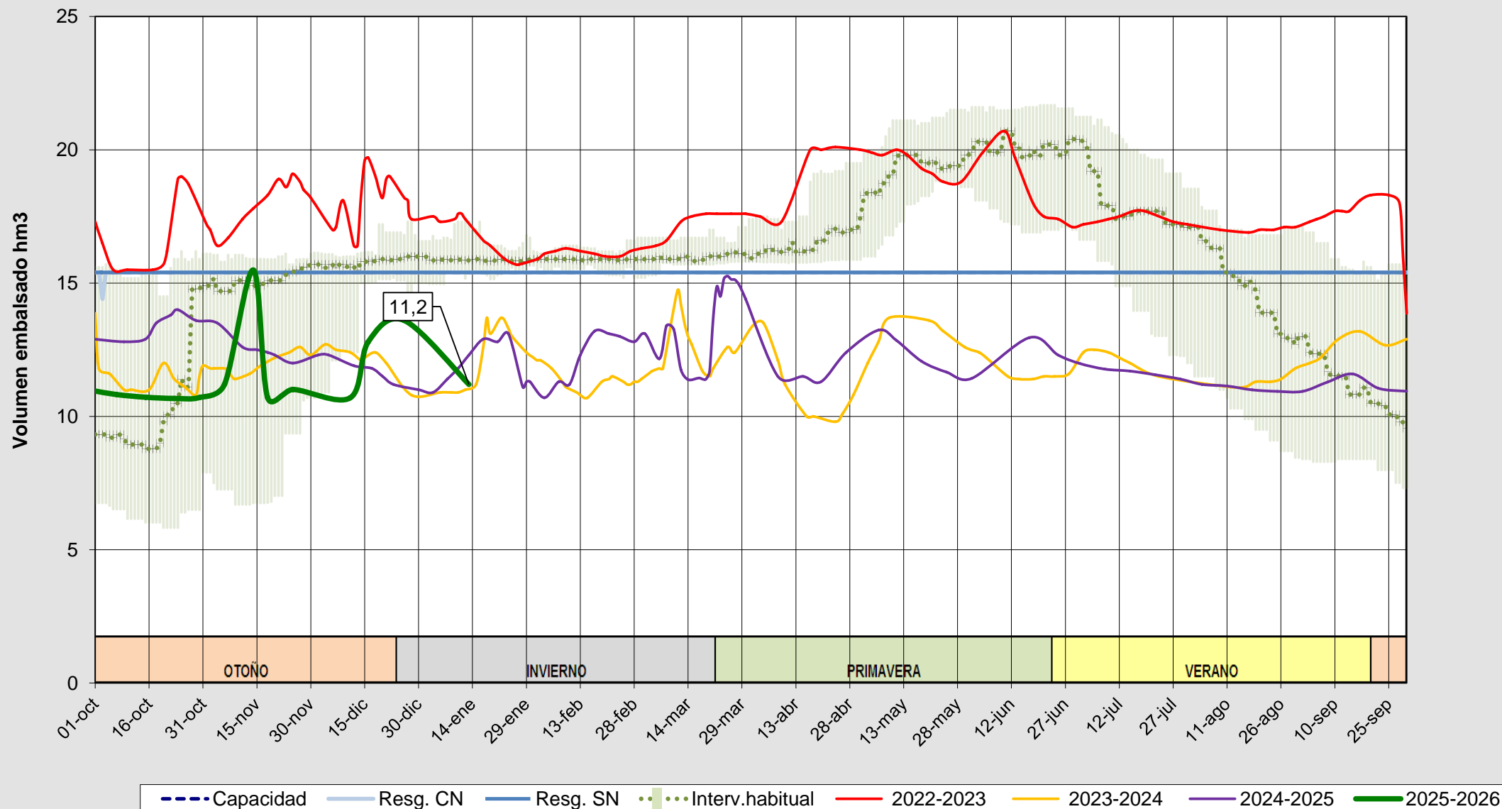
Evolución del volumen almacenado en el embalse de Águeda a fecha 13/01/2026
