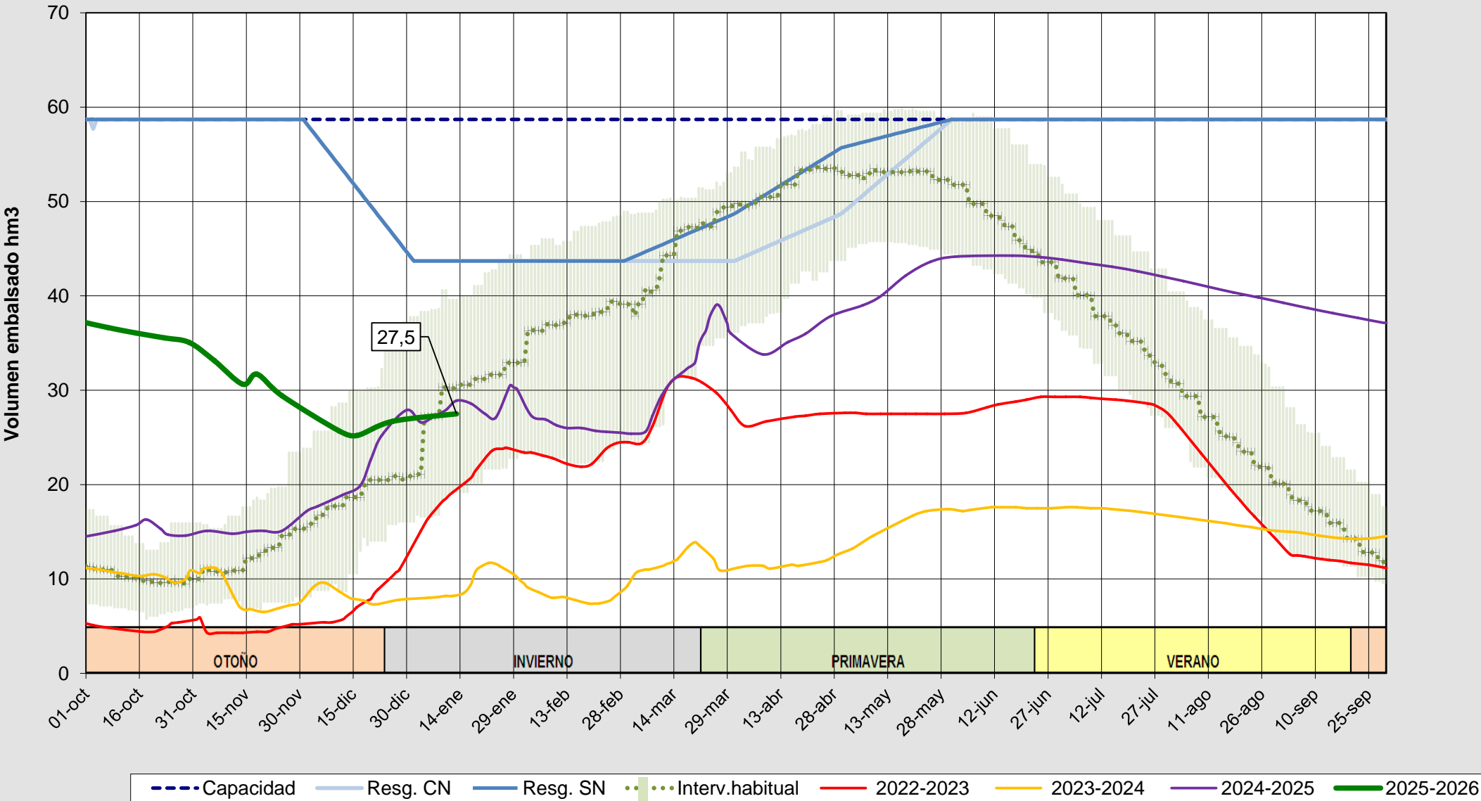
Evolución del volumen almacenado en el embalse de Requejada a fecha 13/01/2026
