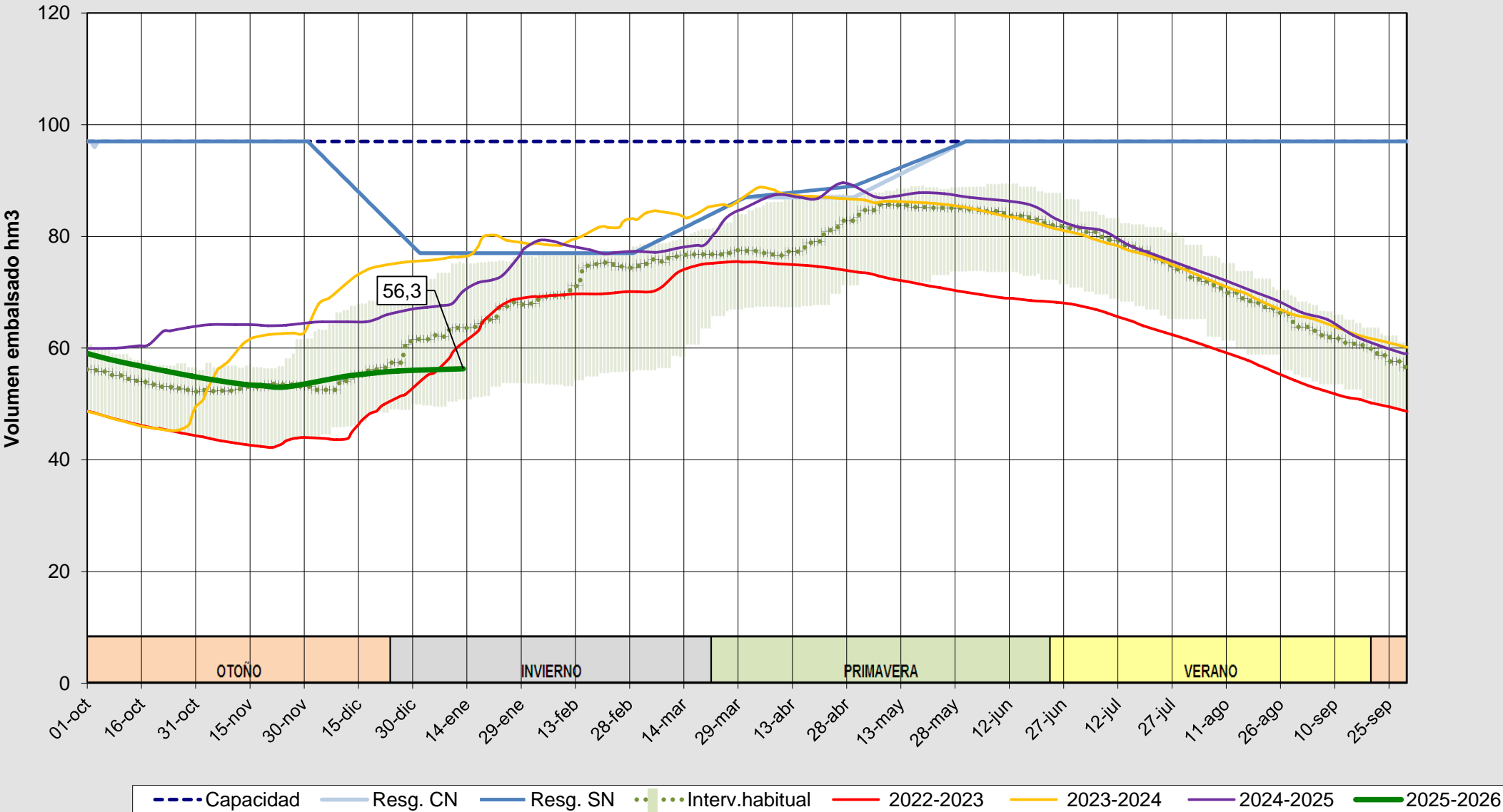
Evolución del volumen almacenado en el sistema del ARLANZÓN a fecha 13/01/2026
