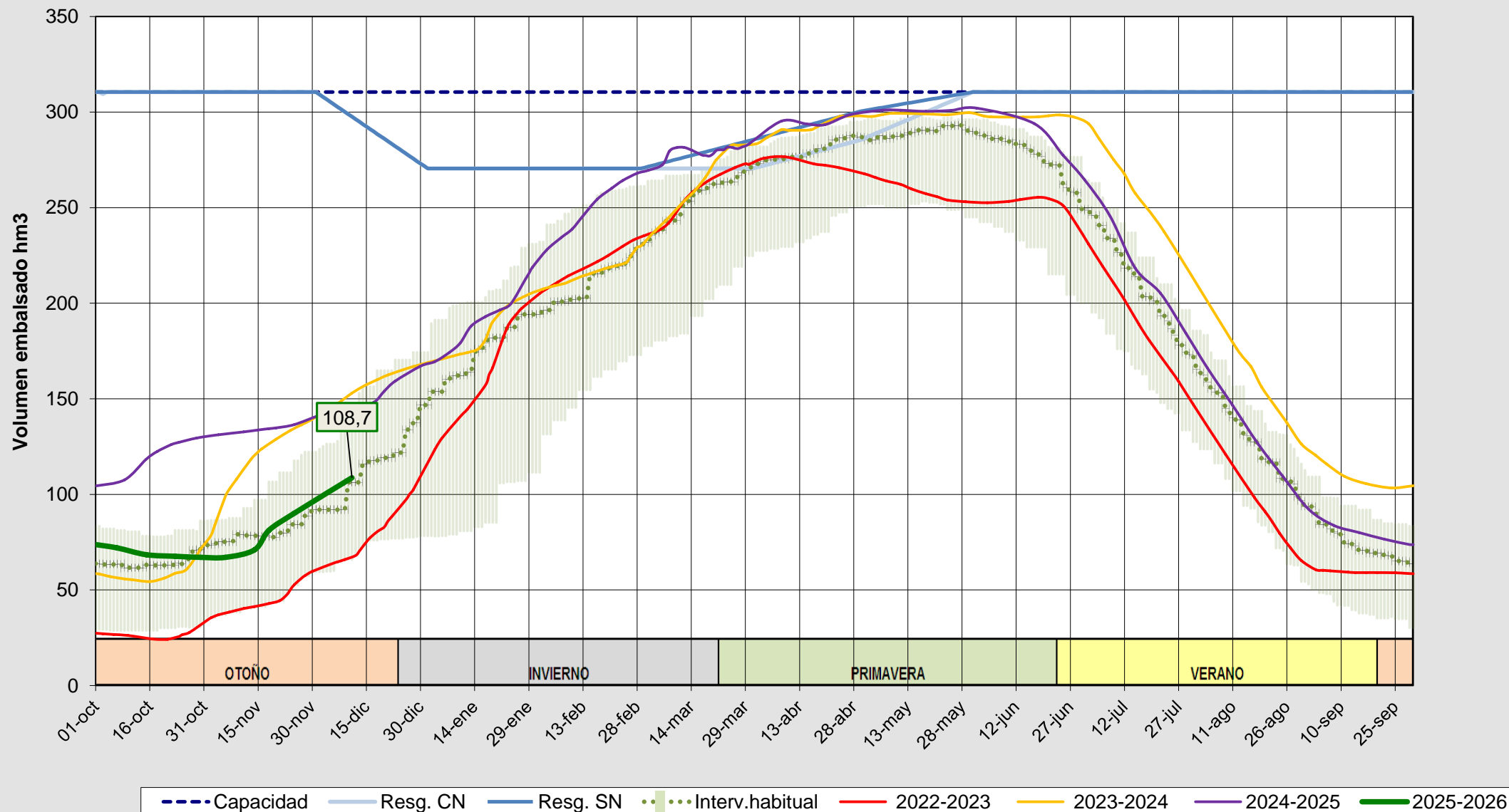
Evolución del volumen almacenado en el embalse de Barrios de Luna a fecha 11/12/2025
