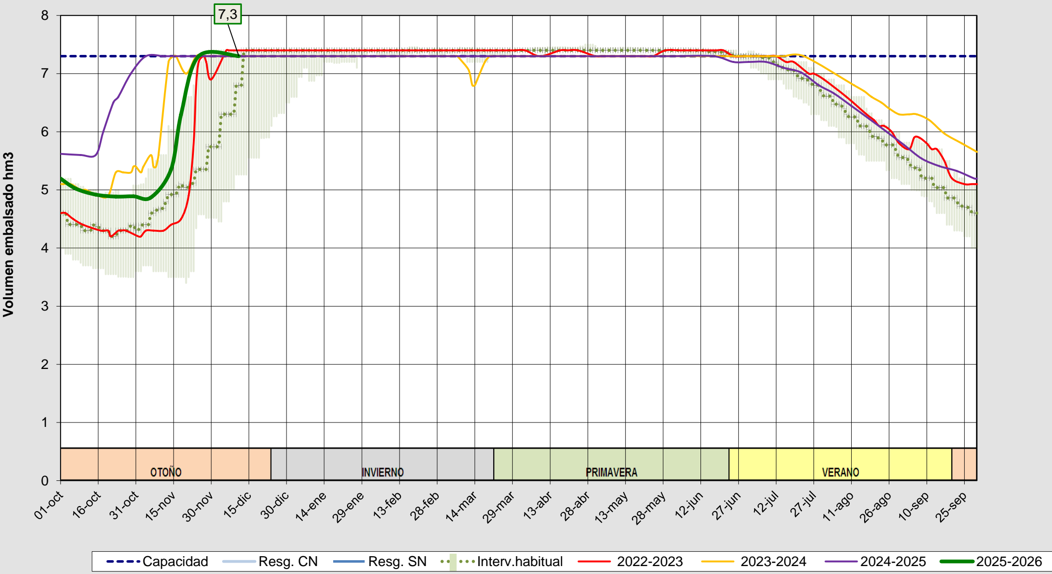
Evolución del volumen almacenado en el embalse de Pontón Alto a fecha 11/12/2025
