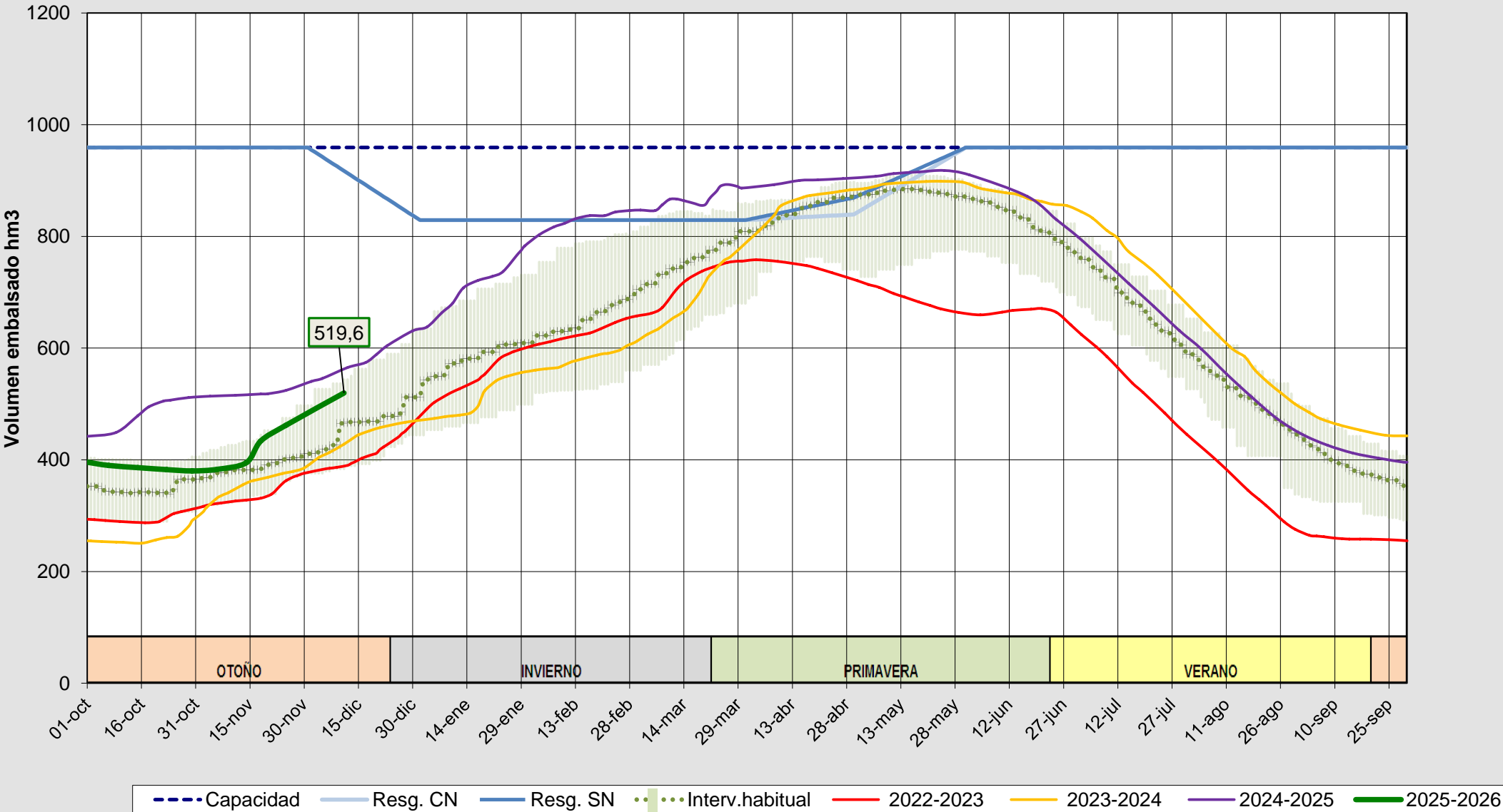
Evolución del volumen almacenado en el sistema del PORMA-ESLA a fecha 11/12/2025
