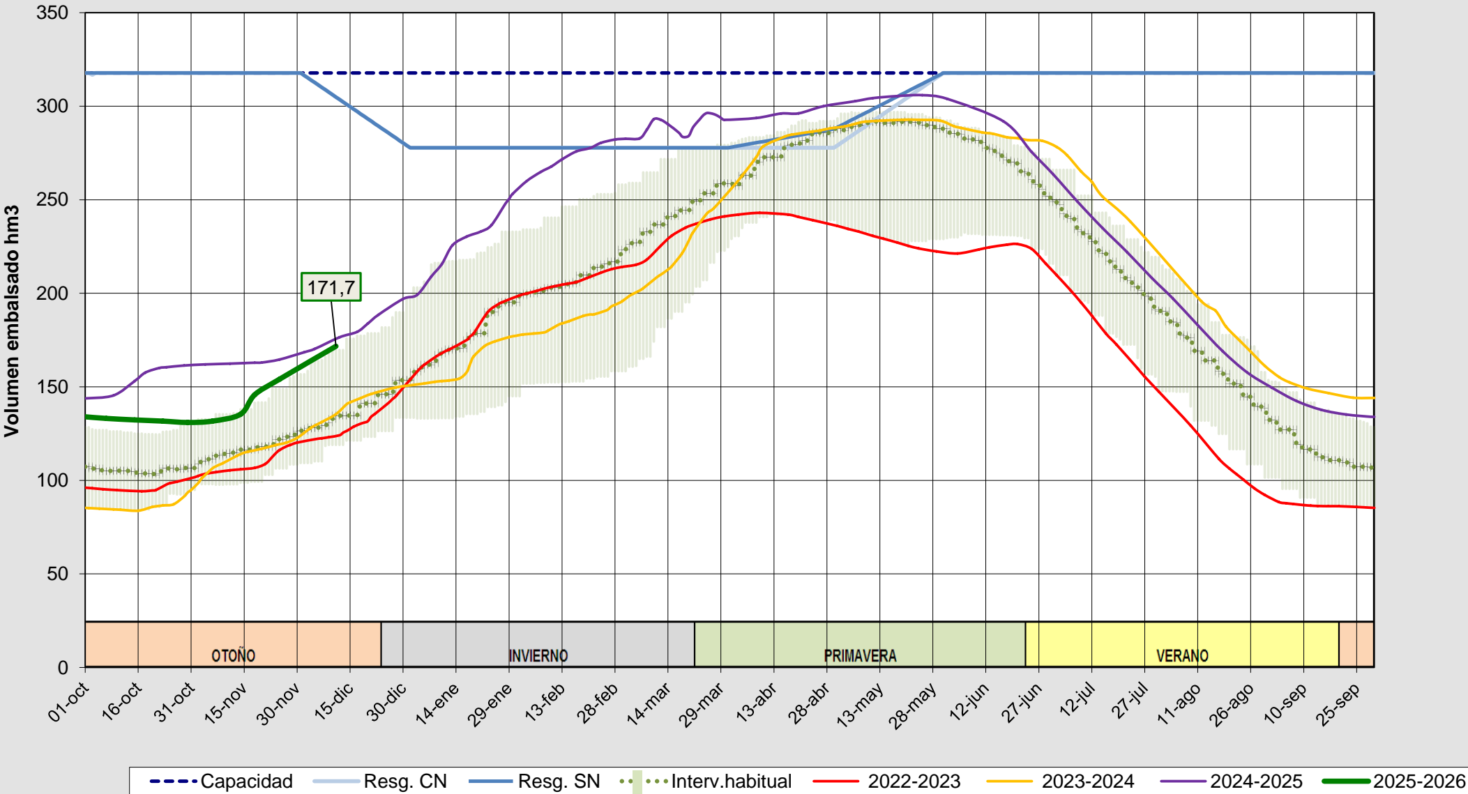
Evolución del volumen almacenado en el embalse de Porma a fecha 11/12/2025
