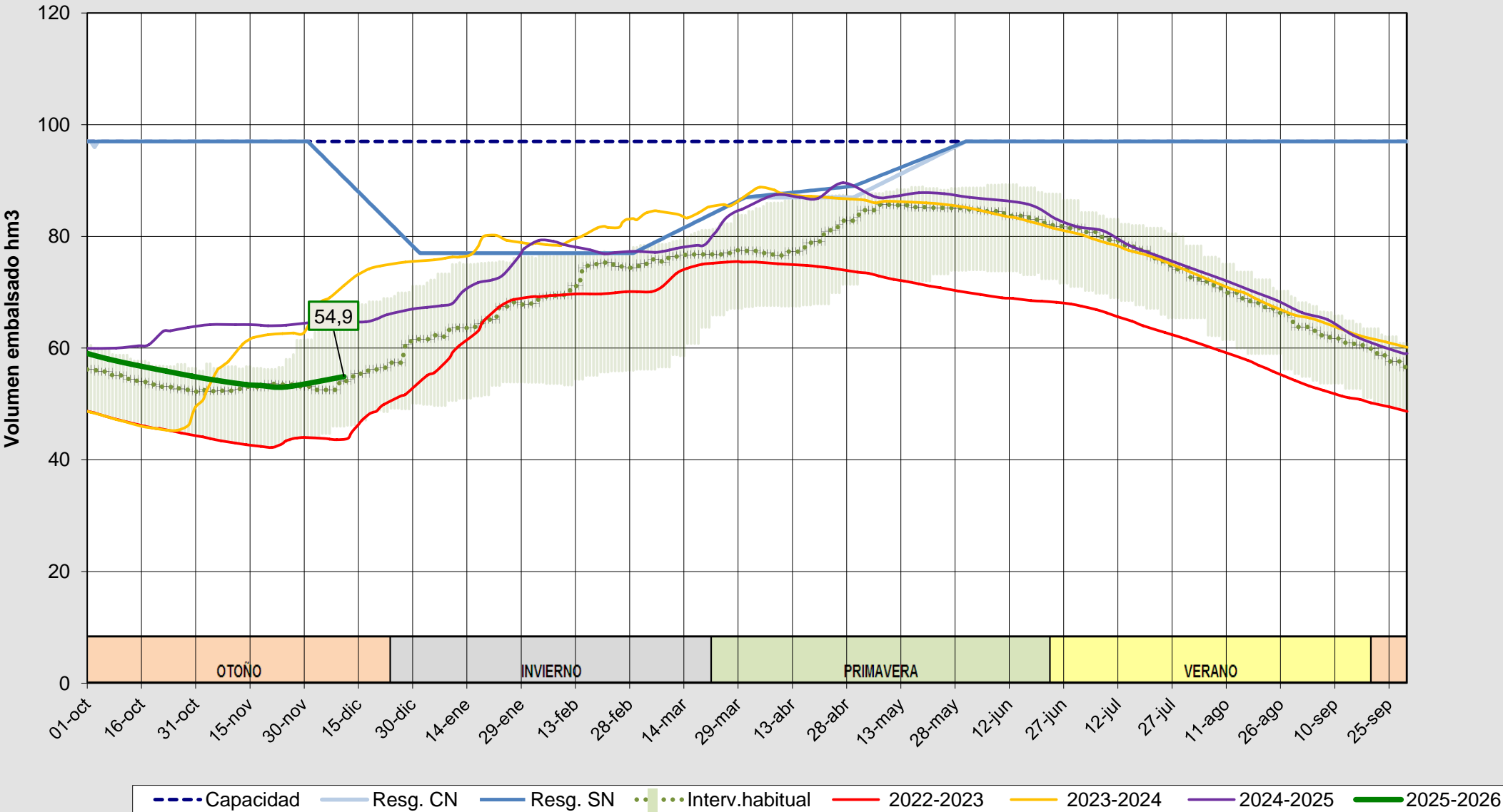
Evolución del volumen almacenado en el sistema del ARLANZÓN a fecha 11/12/2025
