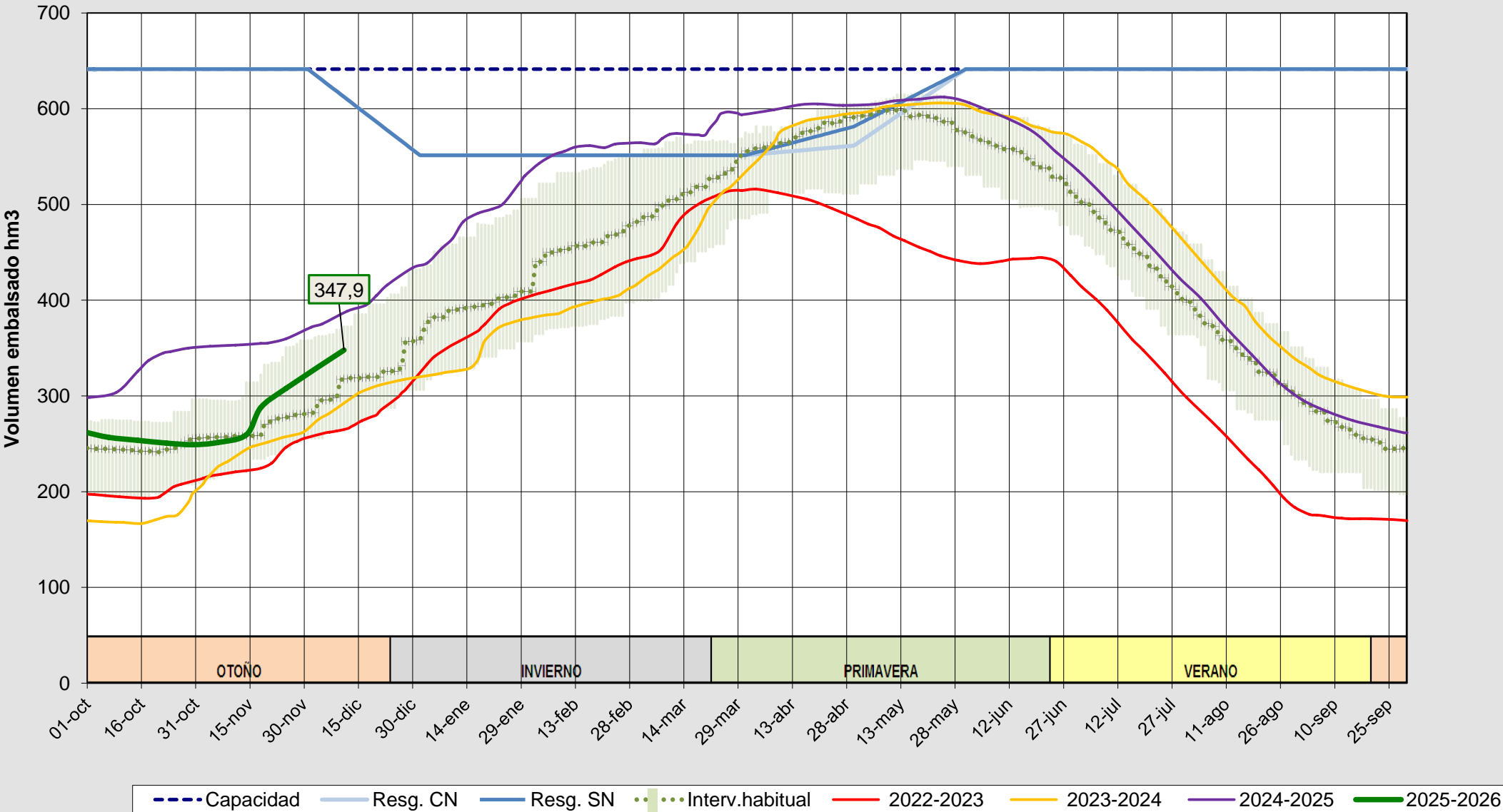
Evolución del volumen almacenado en el embalse de Riaño a fecha 11/12/2025
