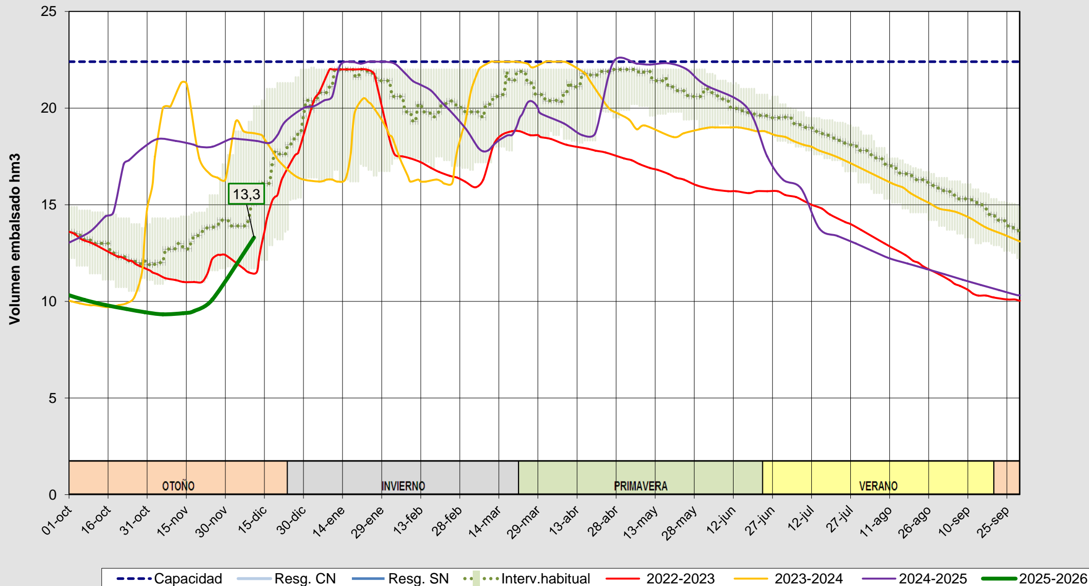
Evolución del volumen almacenado en el embalse de Arlanzón a fecha 11/12/2025
