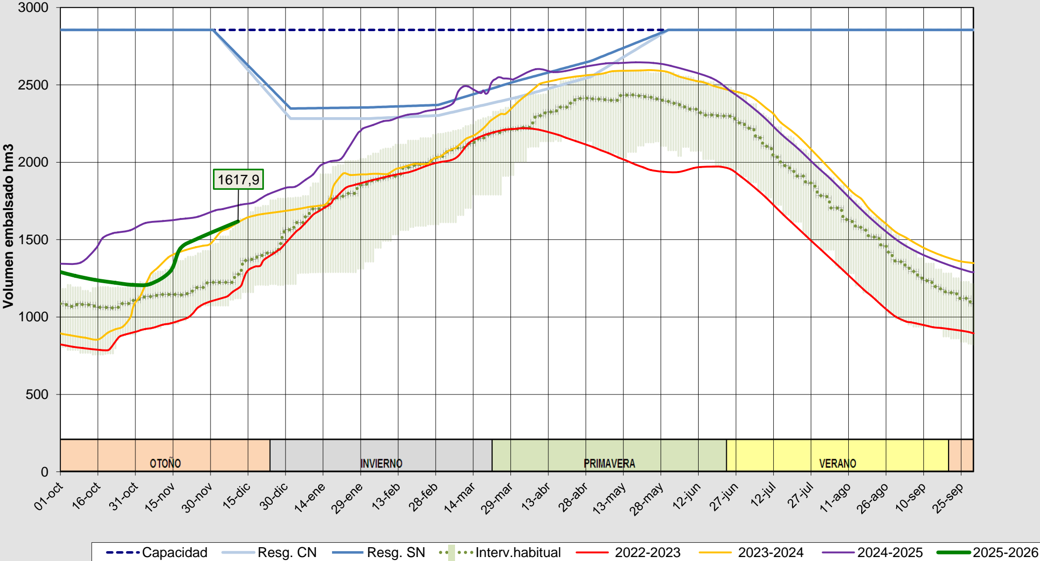
Evolución del volumen almacenado en el sistema del DUERO (ESTADO) a fecha 11/12/2025
