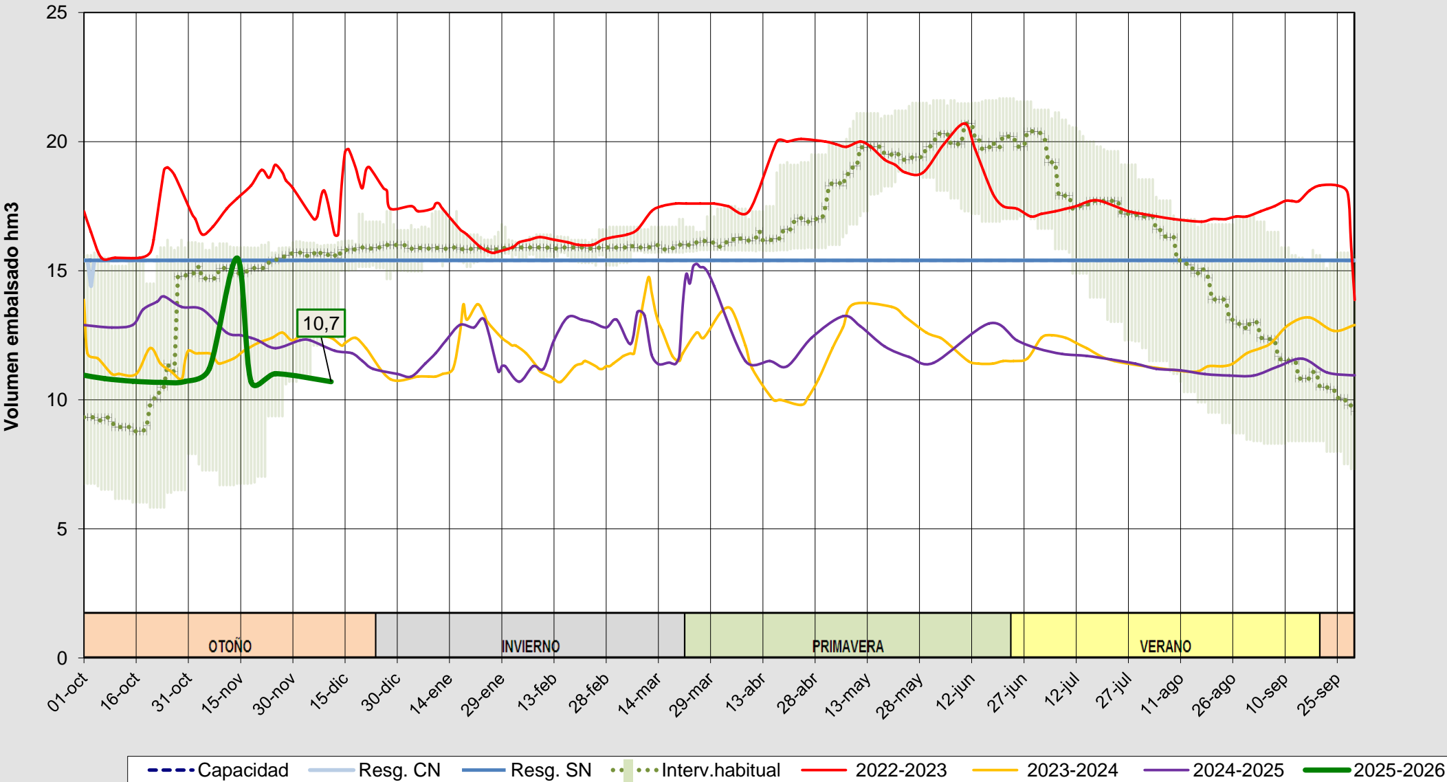
Evolución del volumen almacenado en el embalse de Águeda a fecha 11/12/2025
