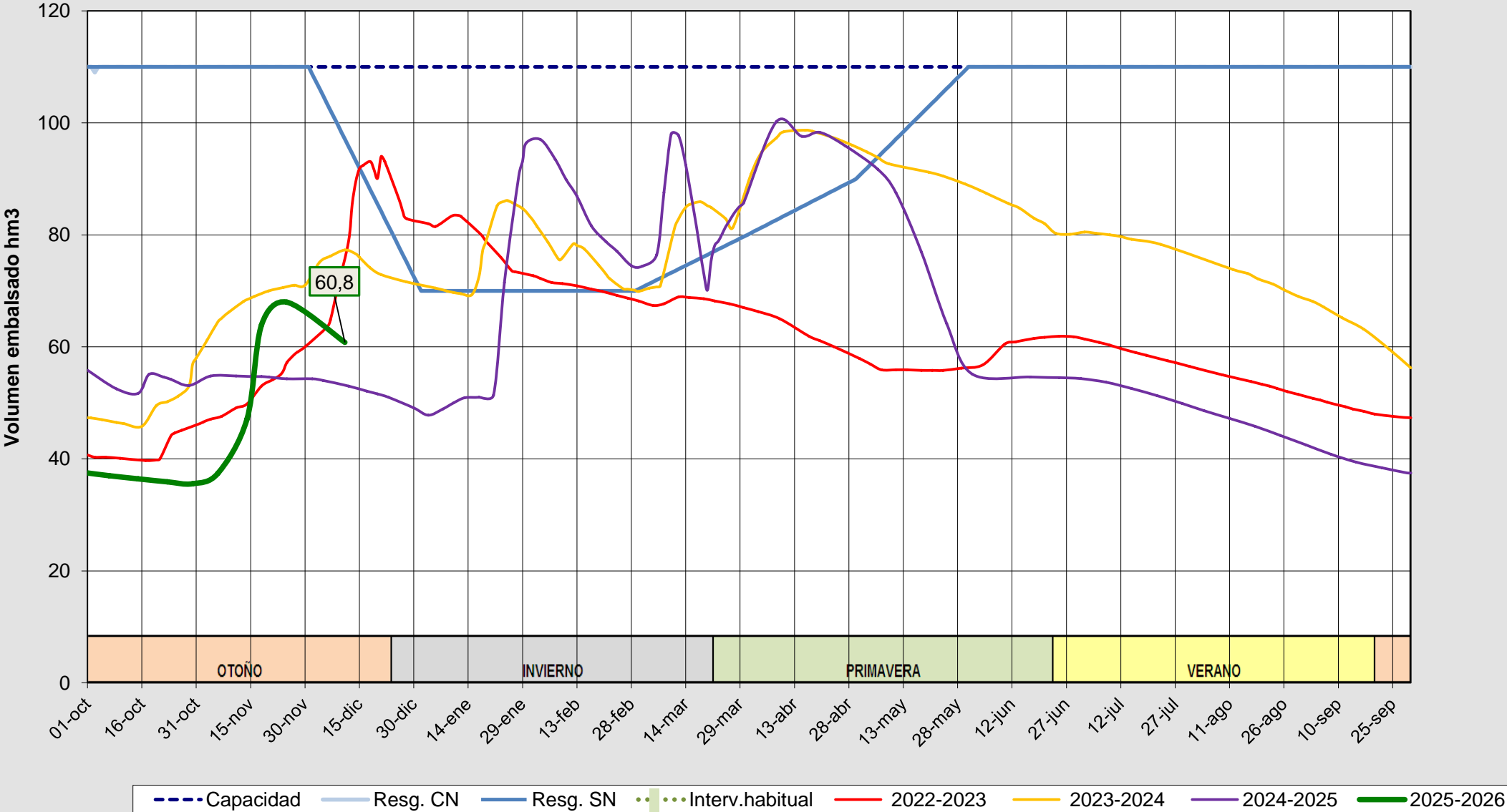
Evolución del volumen almacenado en el embalse de Irueña a fecha 11/12/2025
