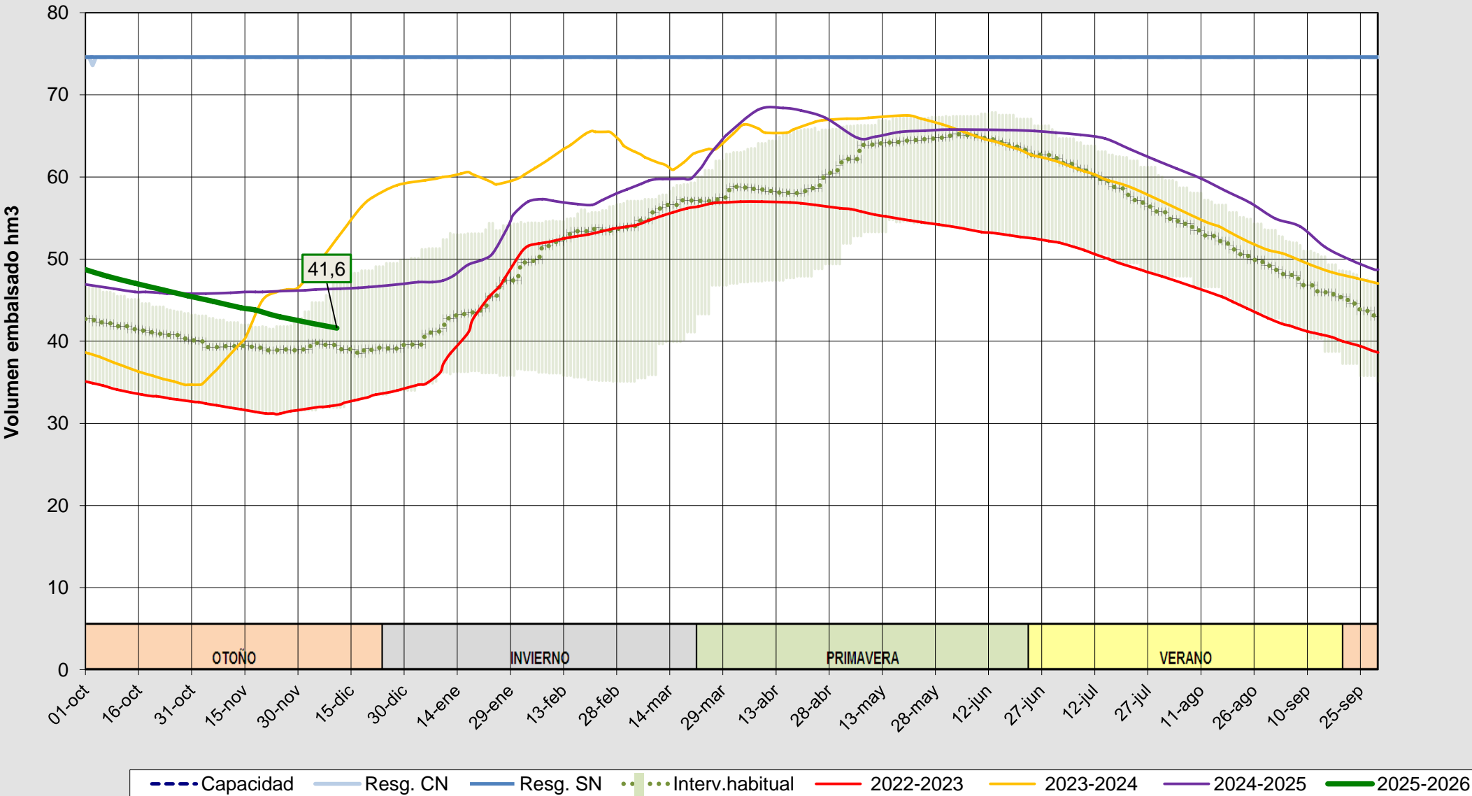
Evolución del volumen almacenado en el embalse de Úzquiza a fecha 11/12/2025
