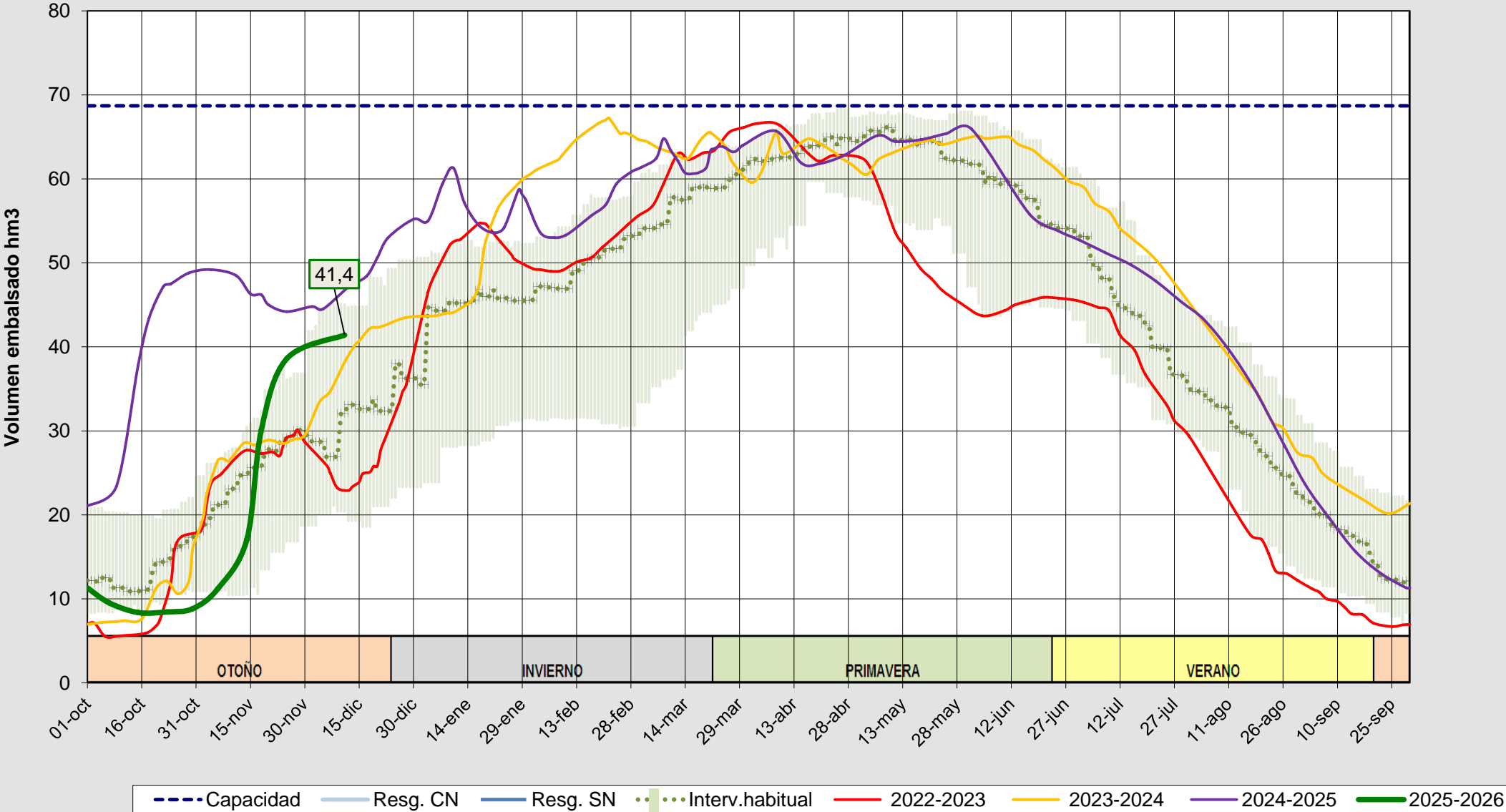
Evolución del volumen almacenado en el embalse de Camporredondo a fecha 11/12/2025
