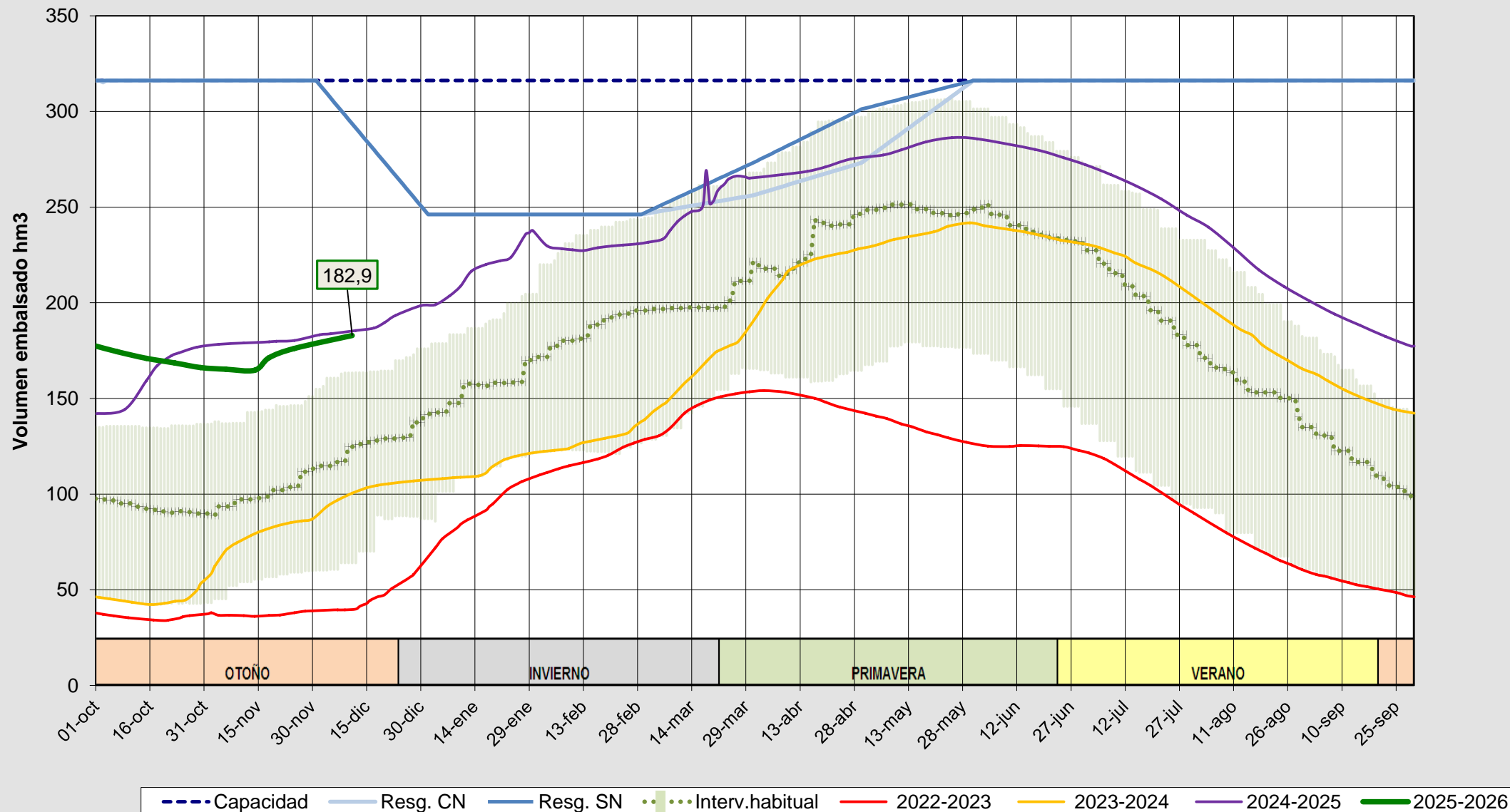
Evolución del volumen almacenado en el sistema del PISUERGA a fecha 11/12/2025
