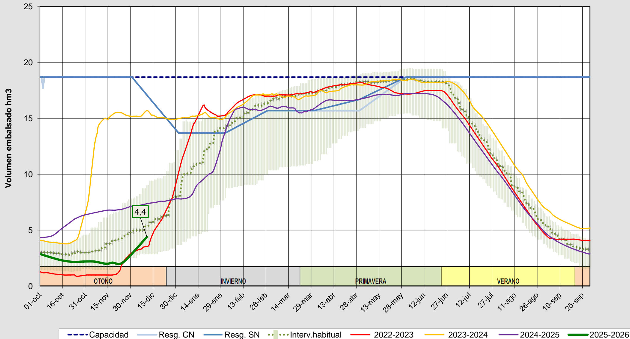
Evolución del volumen almacenado en el embalse de Villameca a fecha 11/12/2025
