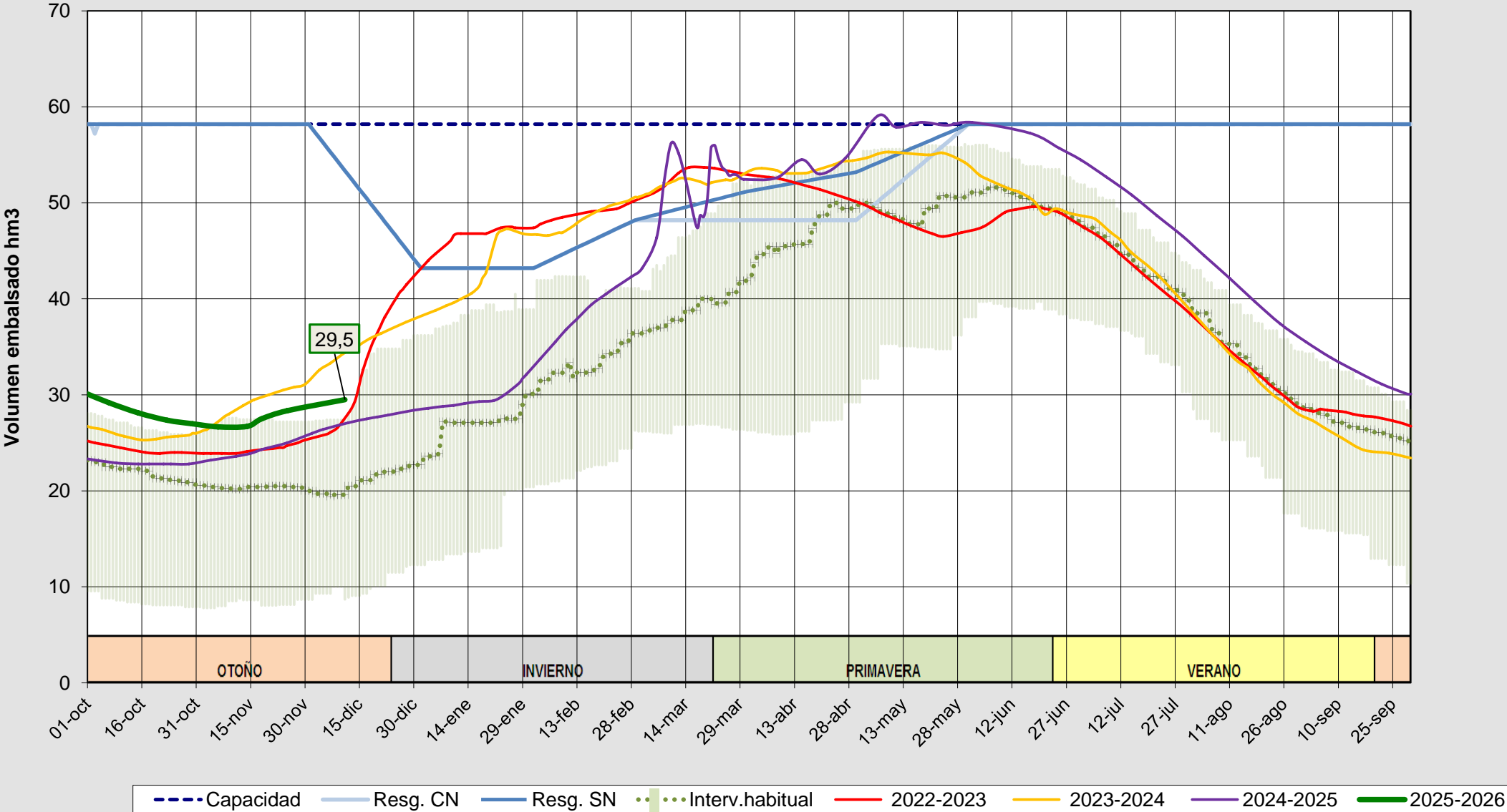
Evolución del volumen almacenado en el embalse de Las Cogotas a fecha 11/12/2025
