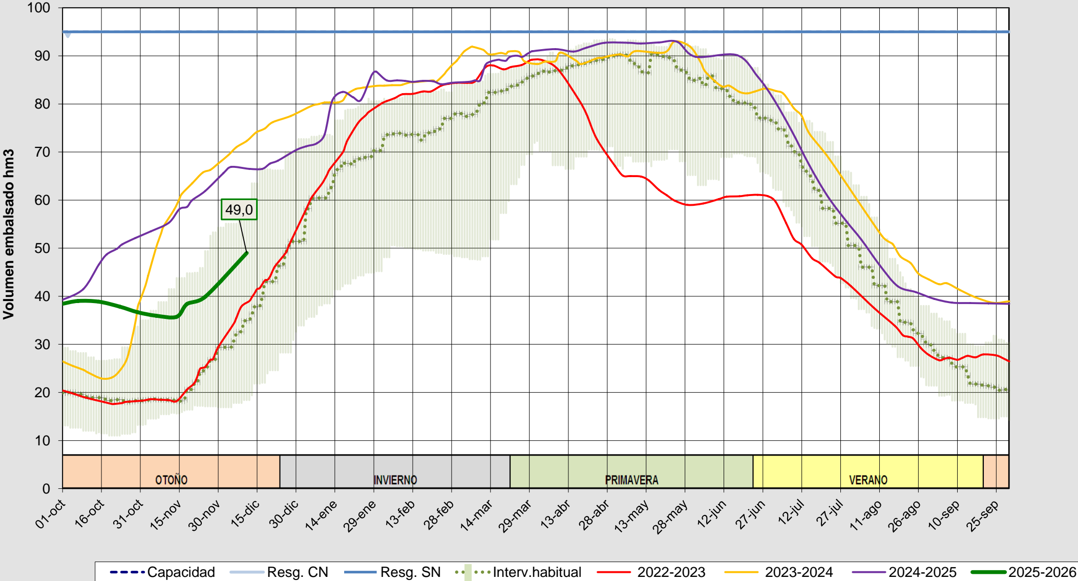
Evolución del volumen almacenado en el embalse de Compuerto a fecha 11/12/2025
