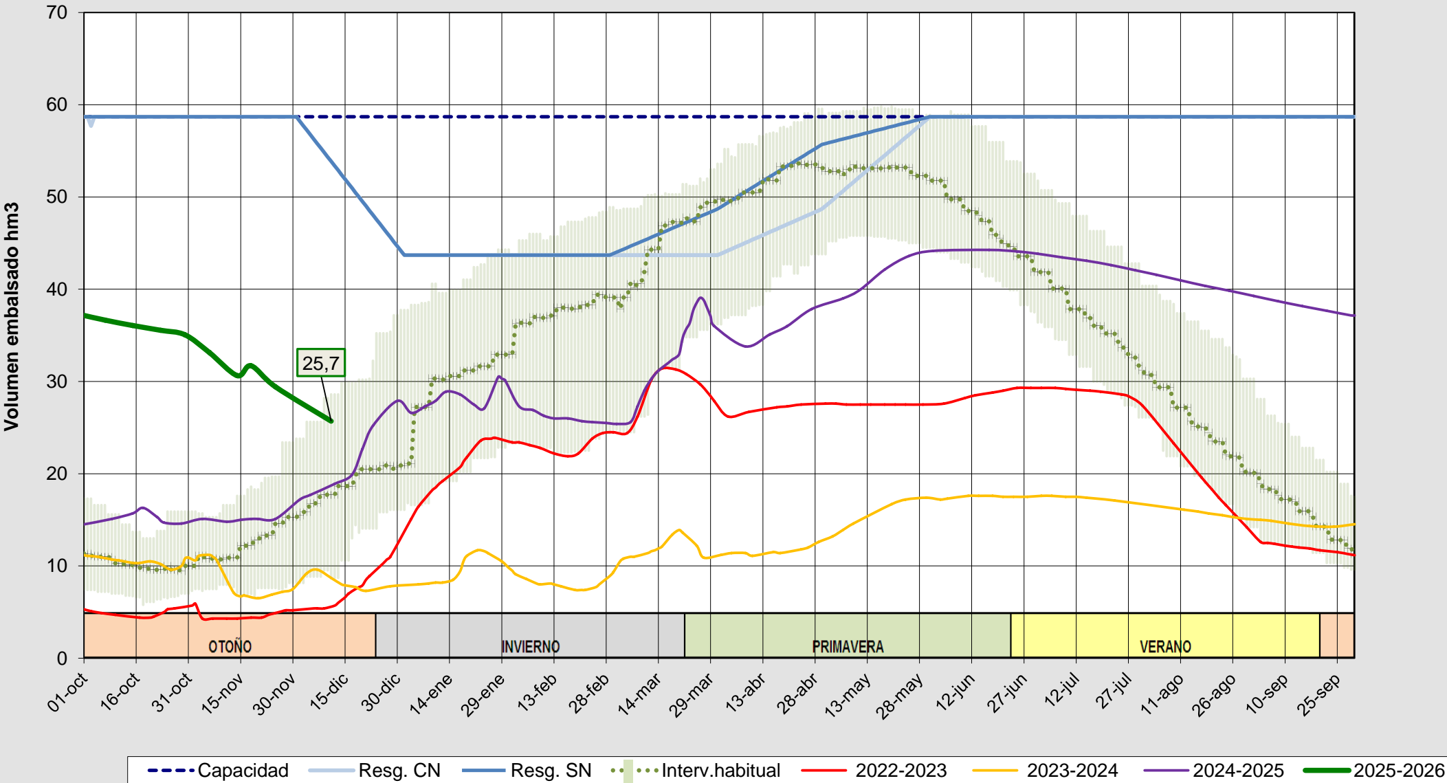
Evolución del volumen almacenado en el embalse de Requejada a fecha 11/12/2025
