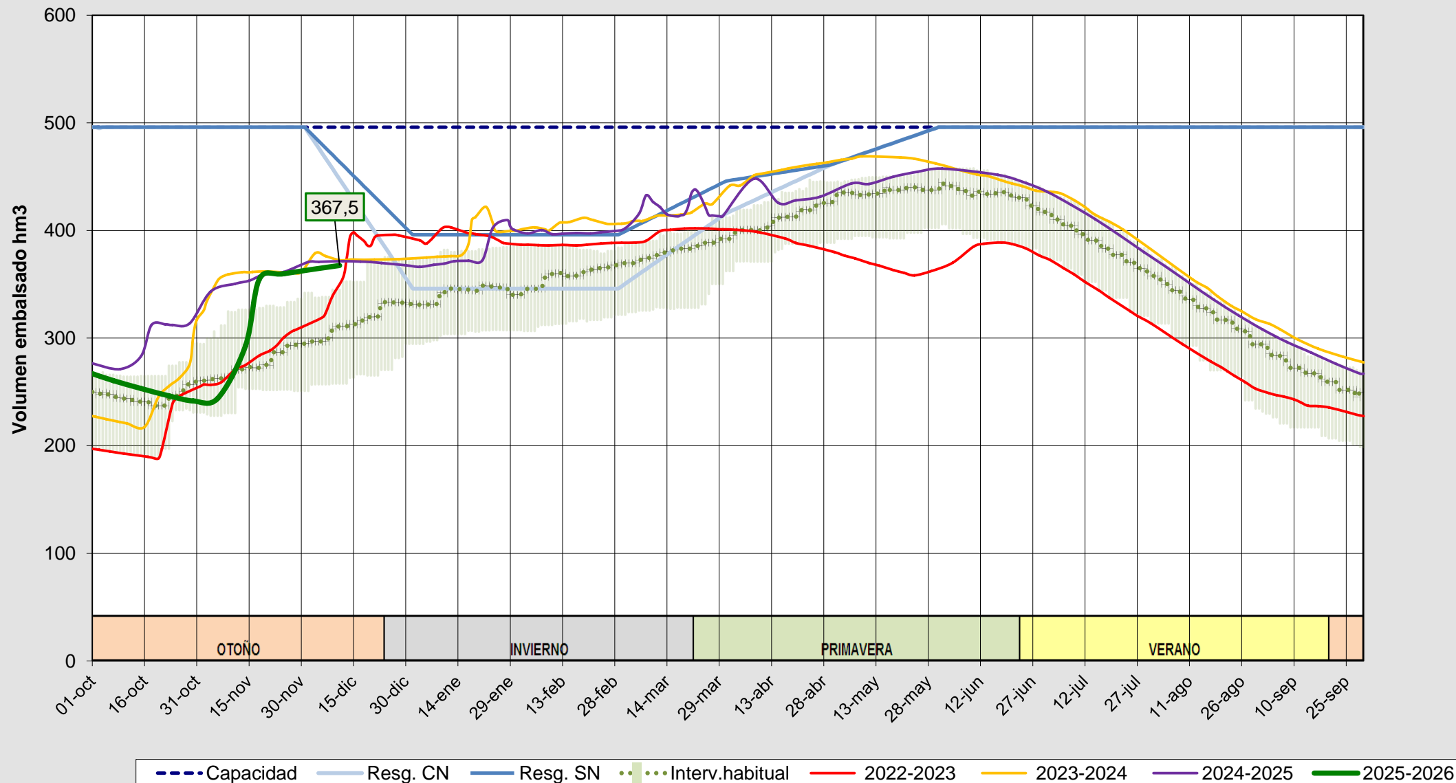
Evolución del volumen almacenado en el embalse de Santa Teresa a fecha 11/12/2025
