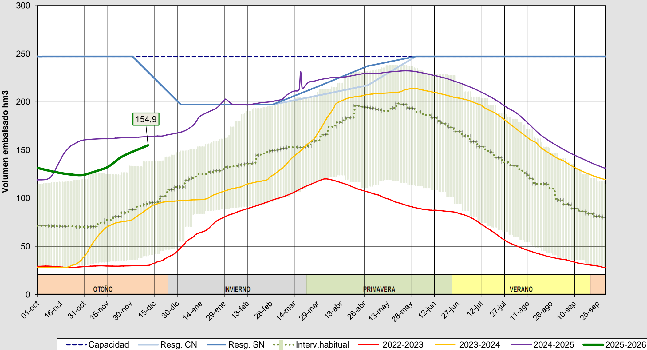
Evolución del volumen almacenado en el embalse de Aguilar a fecha 11/12/2025
