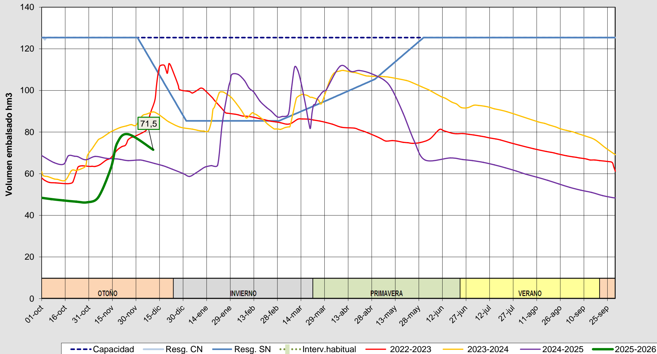
Evolución del volumen almacenado en el sistema del ÁGUEDA a fecha 11/12/2025
