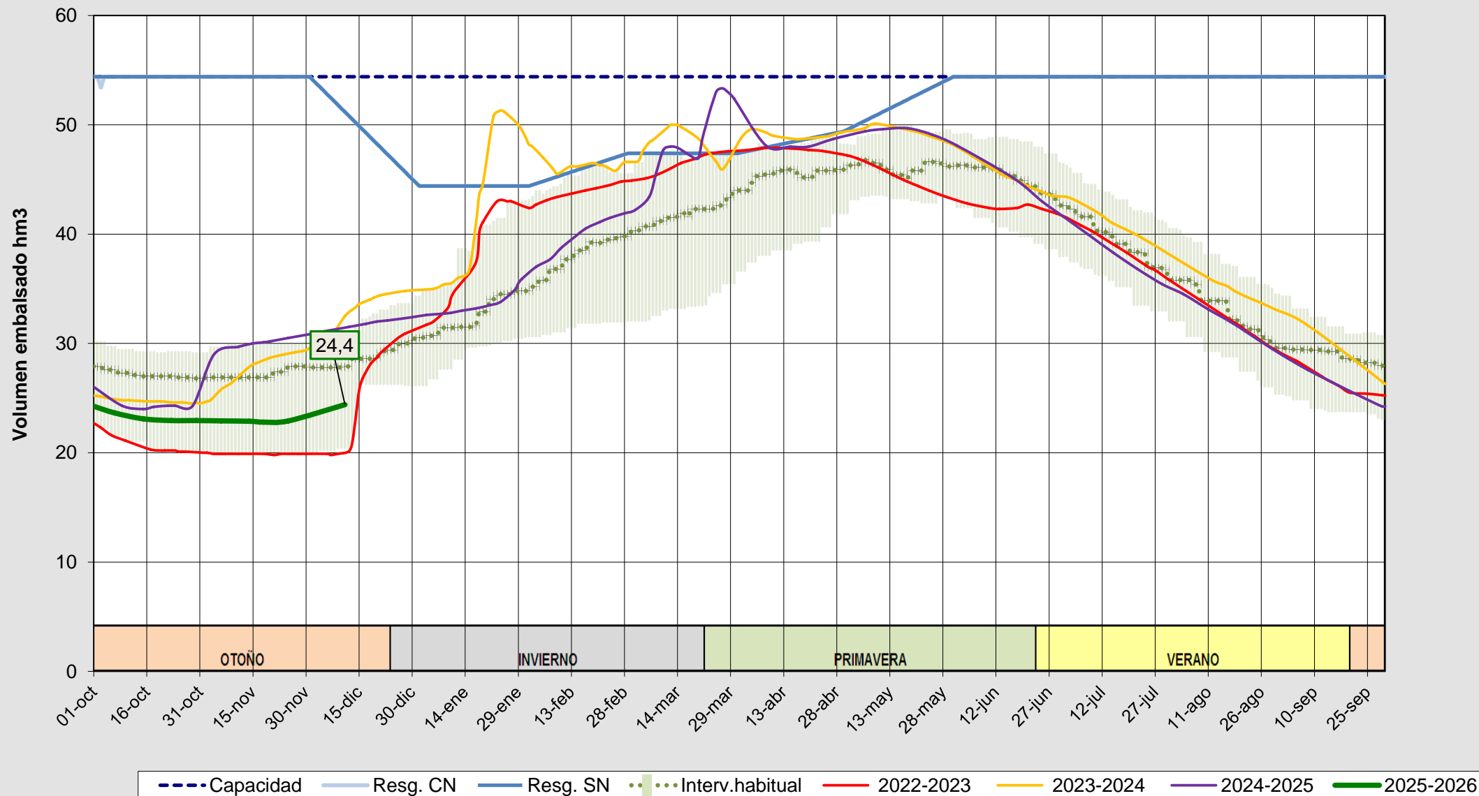
Evolución del volumen almacenado en el embalse de Linares del Arroyo a fecha 11/12/2025
