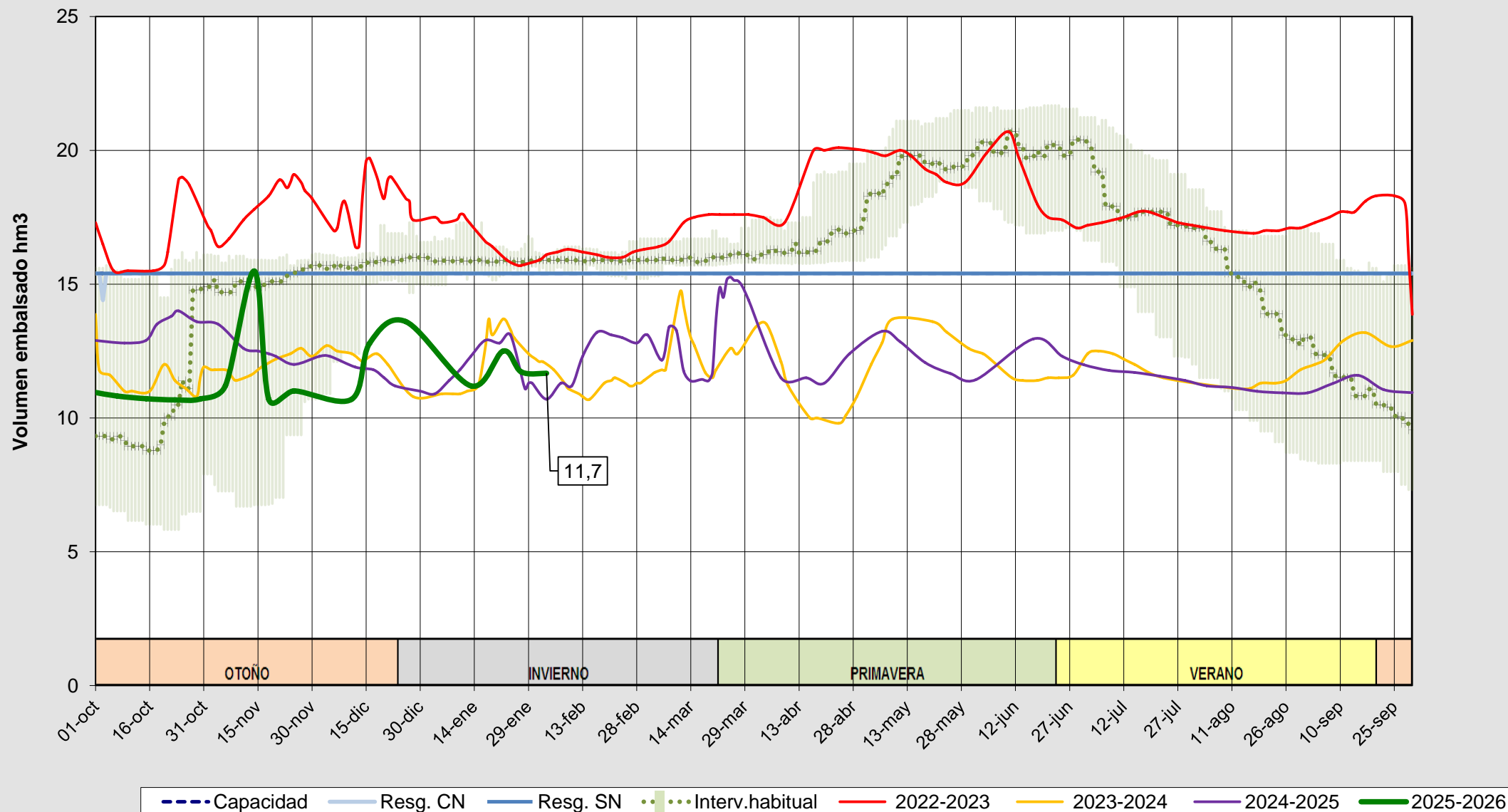
Evolución del volumen almacenado en el embalse de Águeda a fecha 03/02/2026
