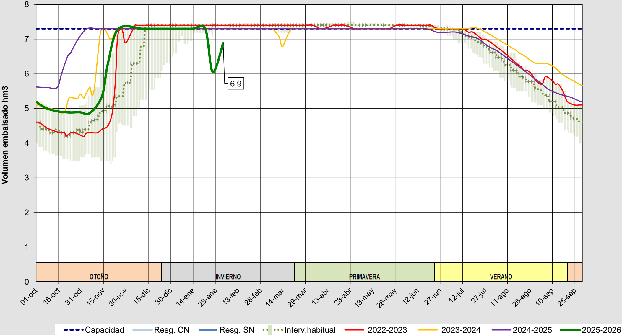
Evolución del volumen almacenado en el embalse de Pontón Alto a fecha 03/02/2026
