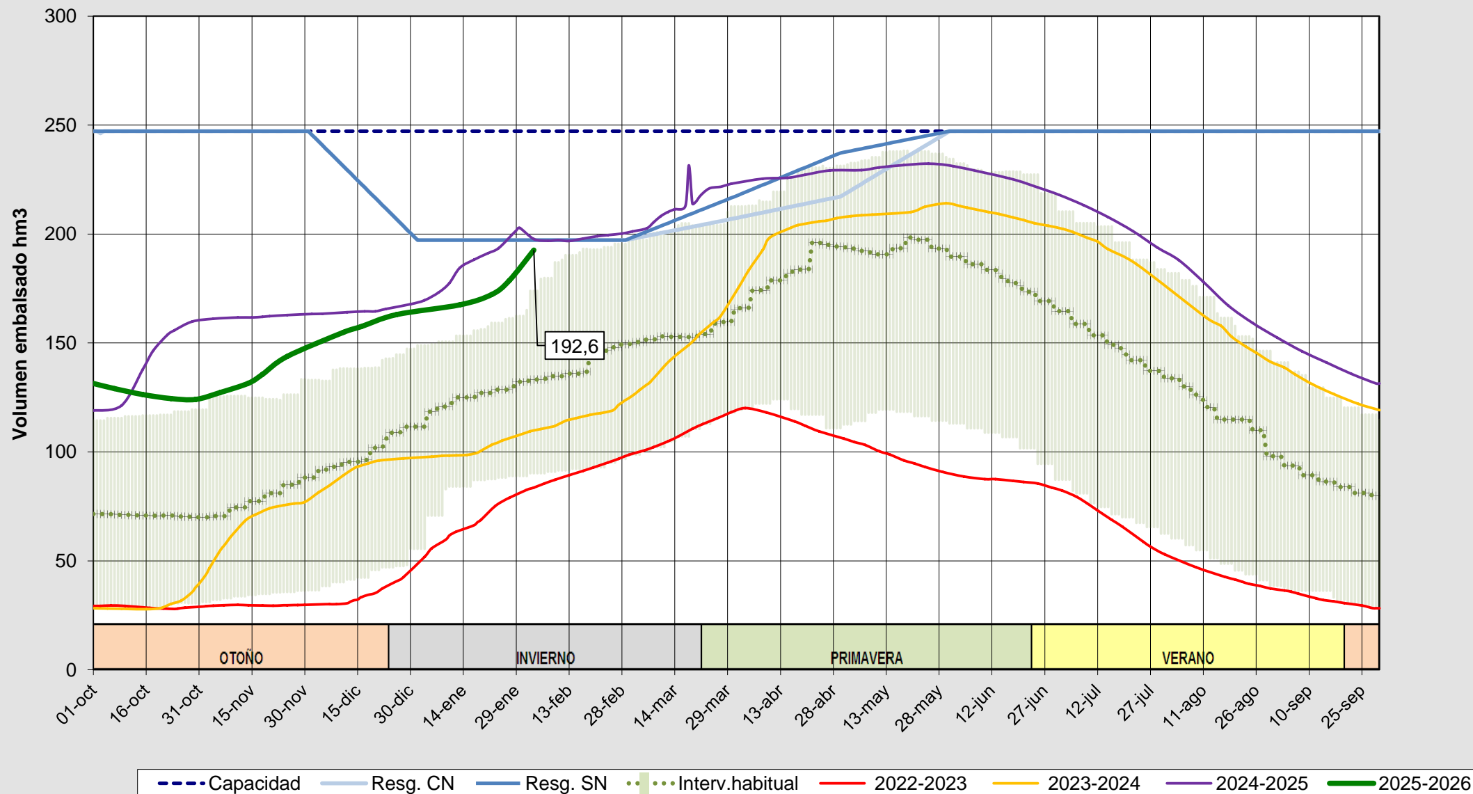
Evolución del volumen almacenado en el embalse de Aguilar a fecha 03/02/2026
