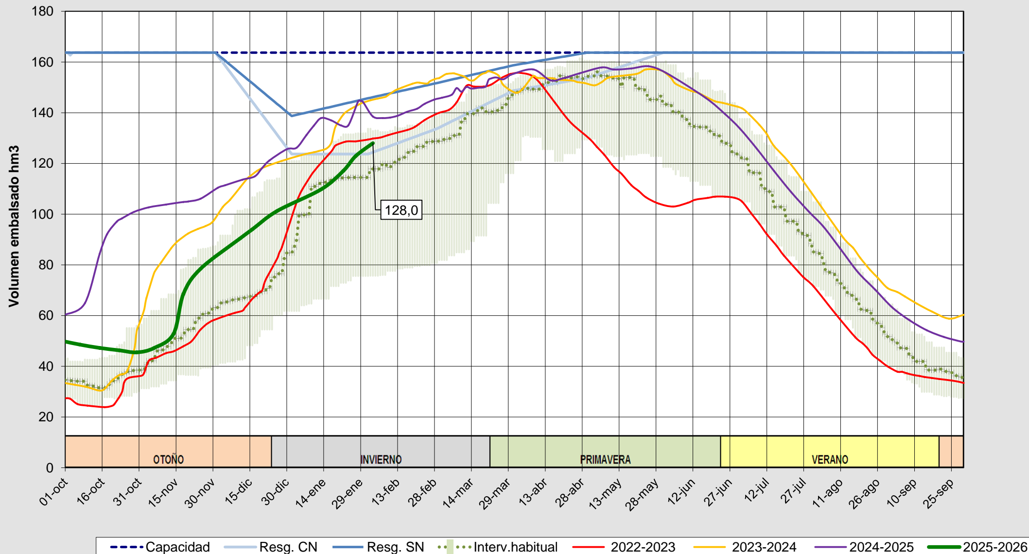
Evolución del volumen almacenado en el sistema del CARRIÓN a fecha 03/02/2026
