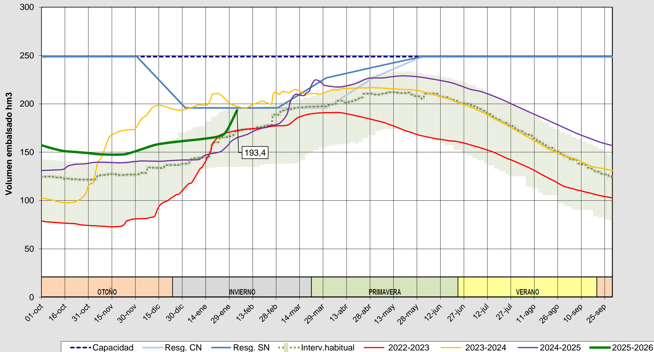
Evolución del volumen almacenado en el embalse de Cuerda del Pozo a fecha 03/02/2026
