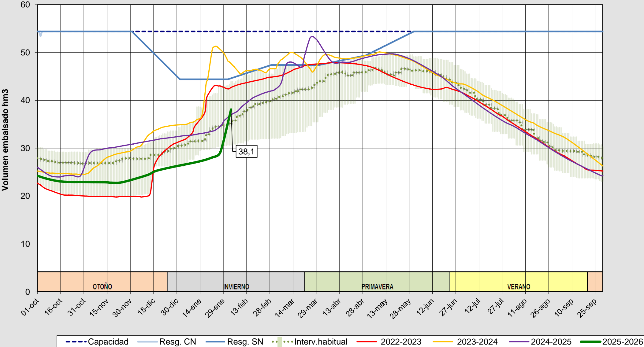
Evolución del volumen almacenado en el embalse de Linares del Arroyo a fecha 03/02/2026
