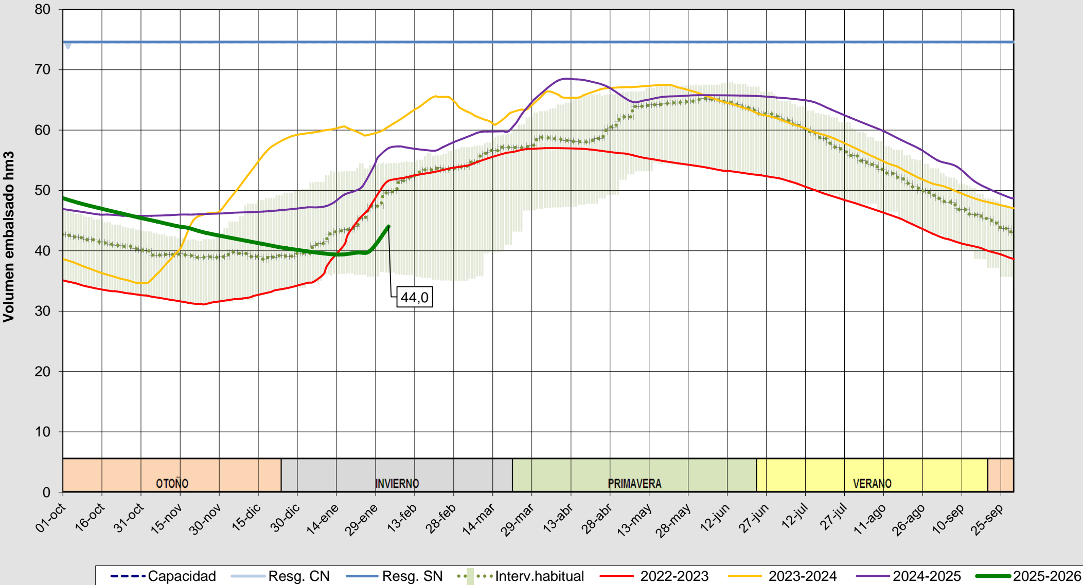
Evolución del volumen almacenado en el embalse de Úzquiza a fecha 03/02/2026
