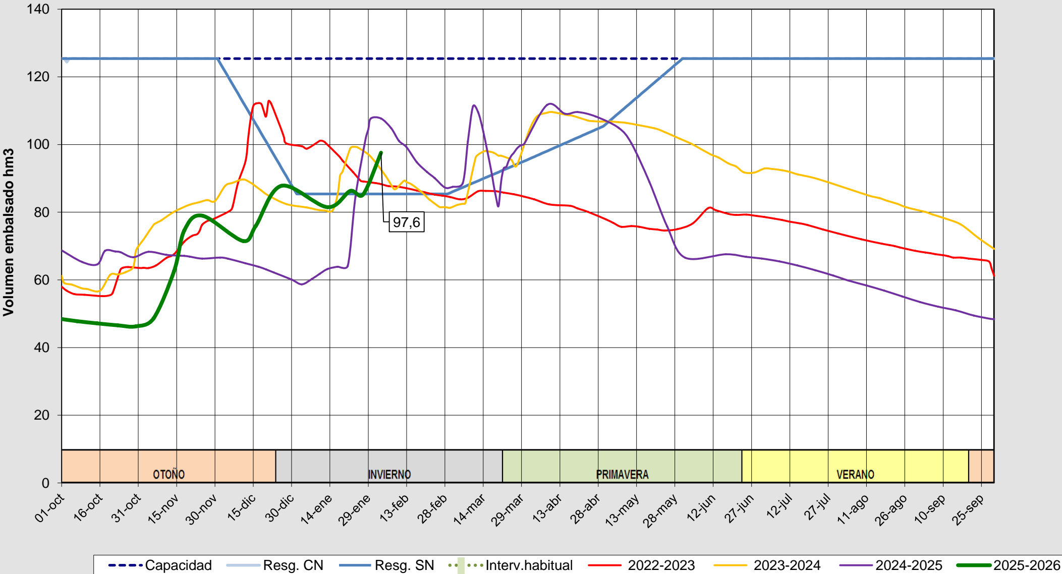
Evolución del volumen almacenado en el sistema del ÁGUEDA a fecha 03/02/2026
