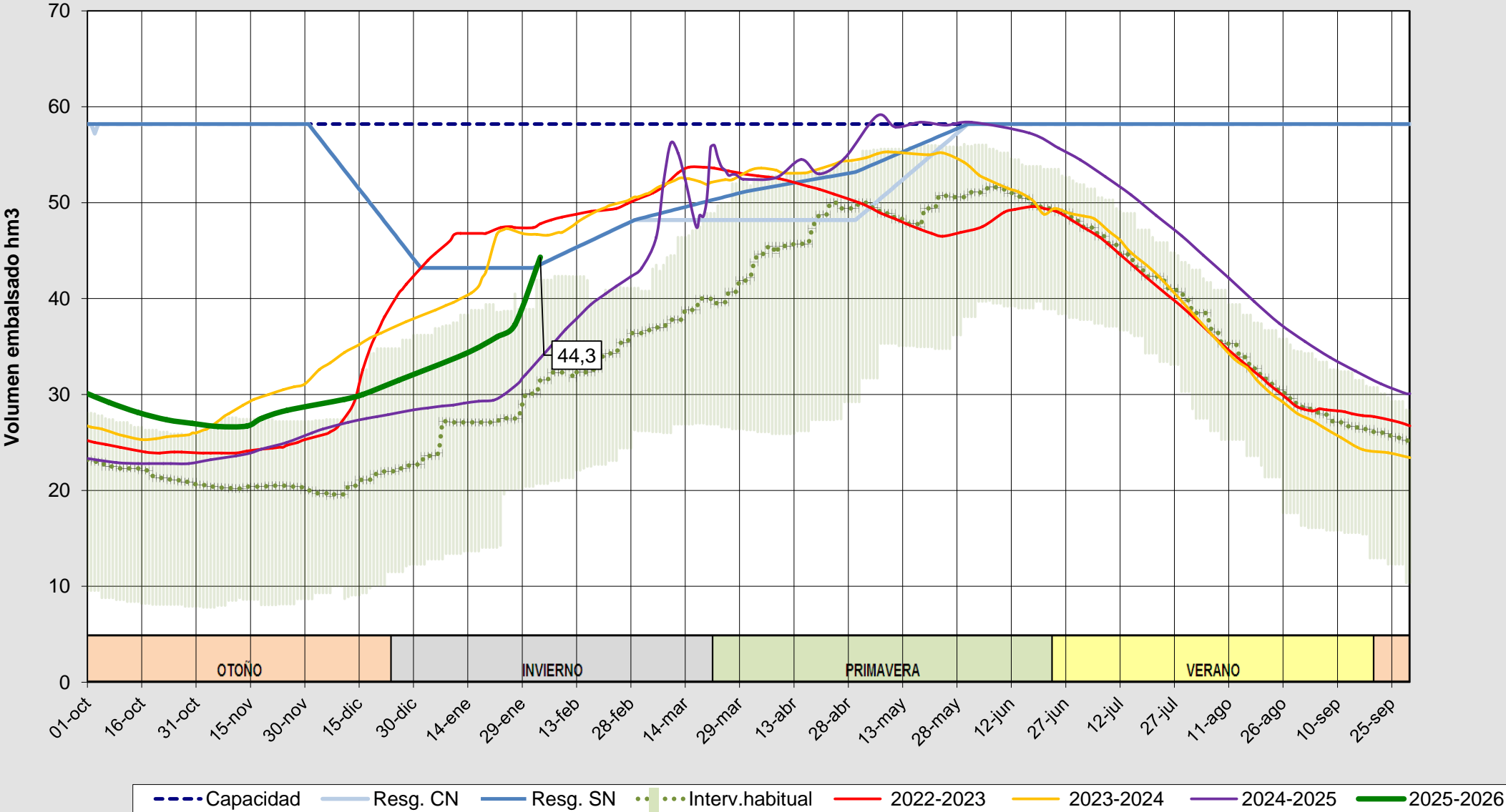
Evolución del volumen almacenado en el embalse de Las Cogotas a fecha 03/02/2026
