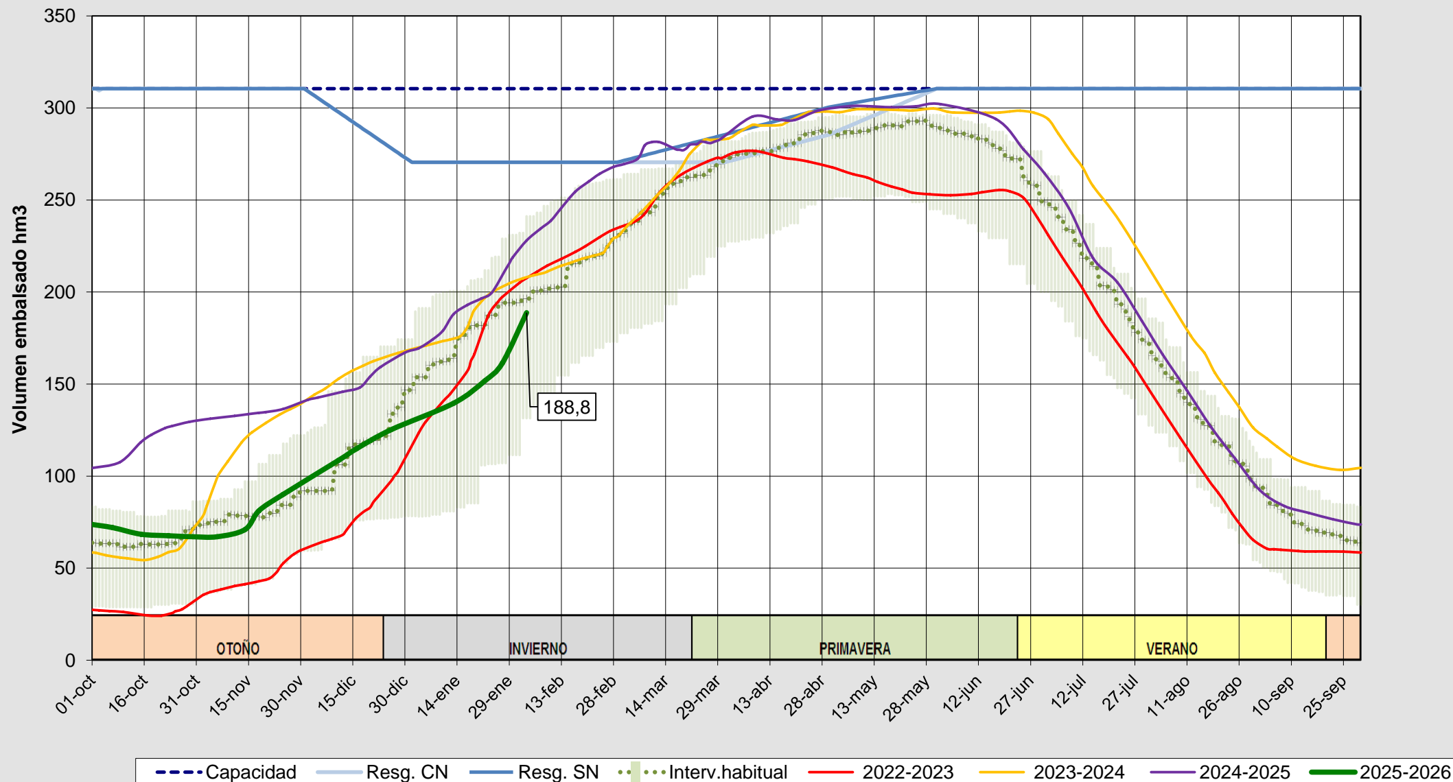
Evolución del volumen almacenado en el embalse de Barrios de Luna a fecha 03/02/2026
