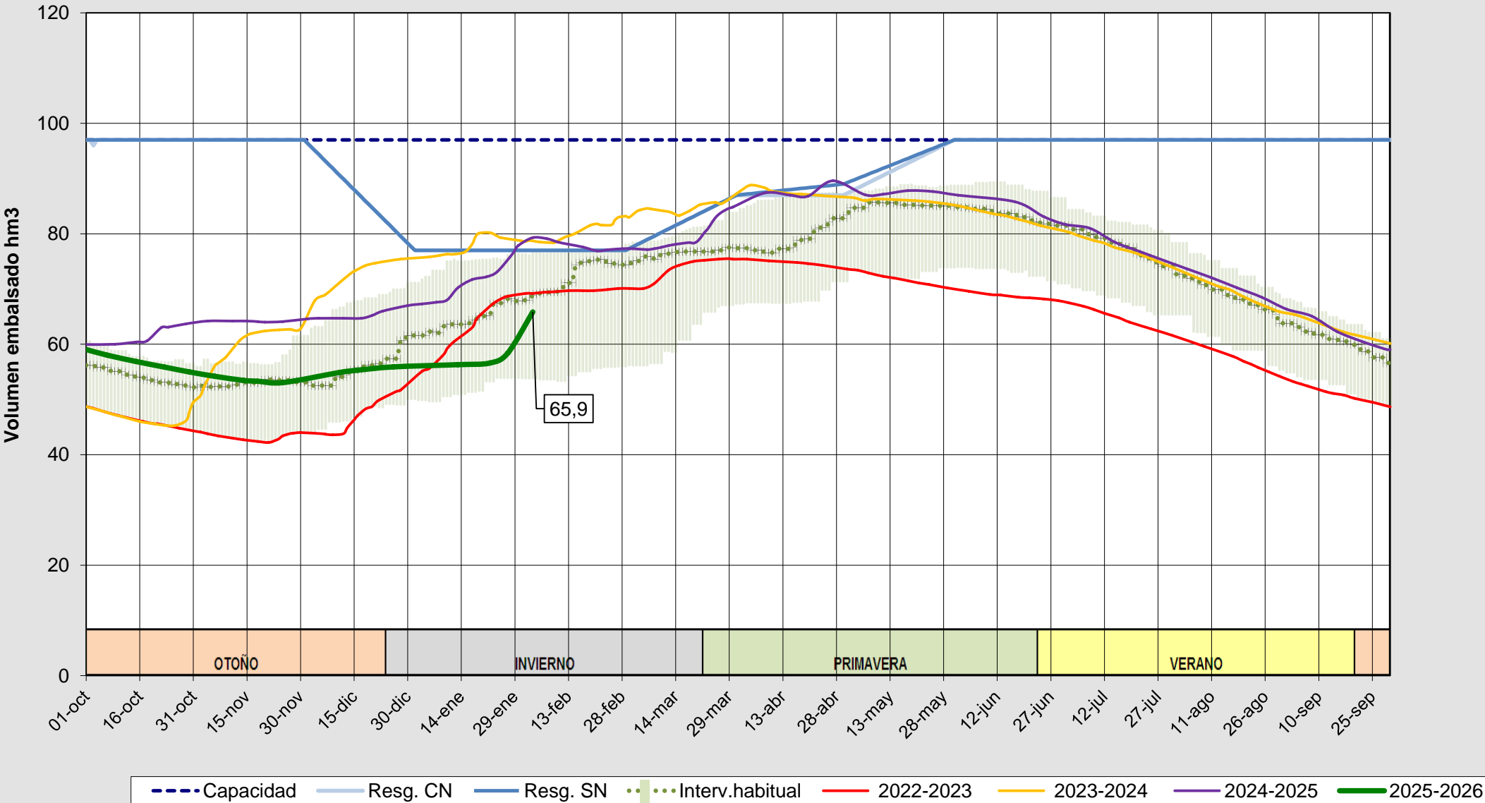
Evolución del volumen almacenado en el sistema del ARLANZÓN a fecha 03/02/2026
