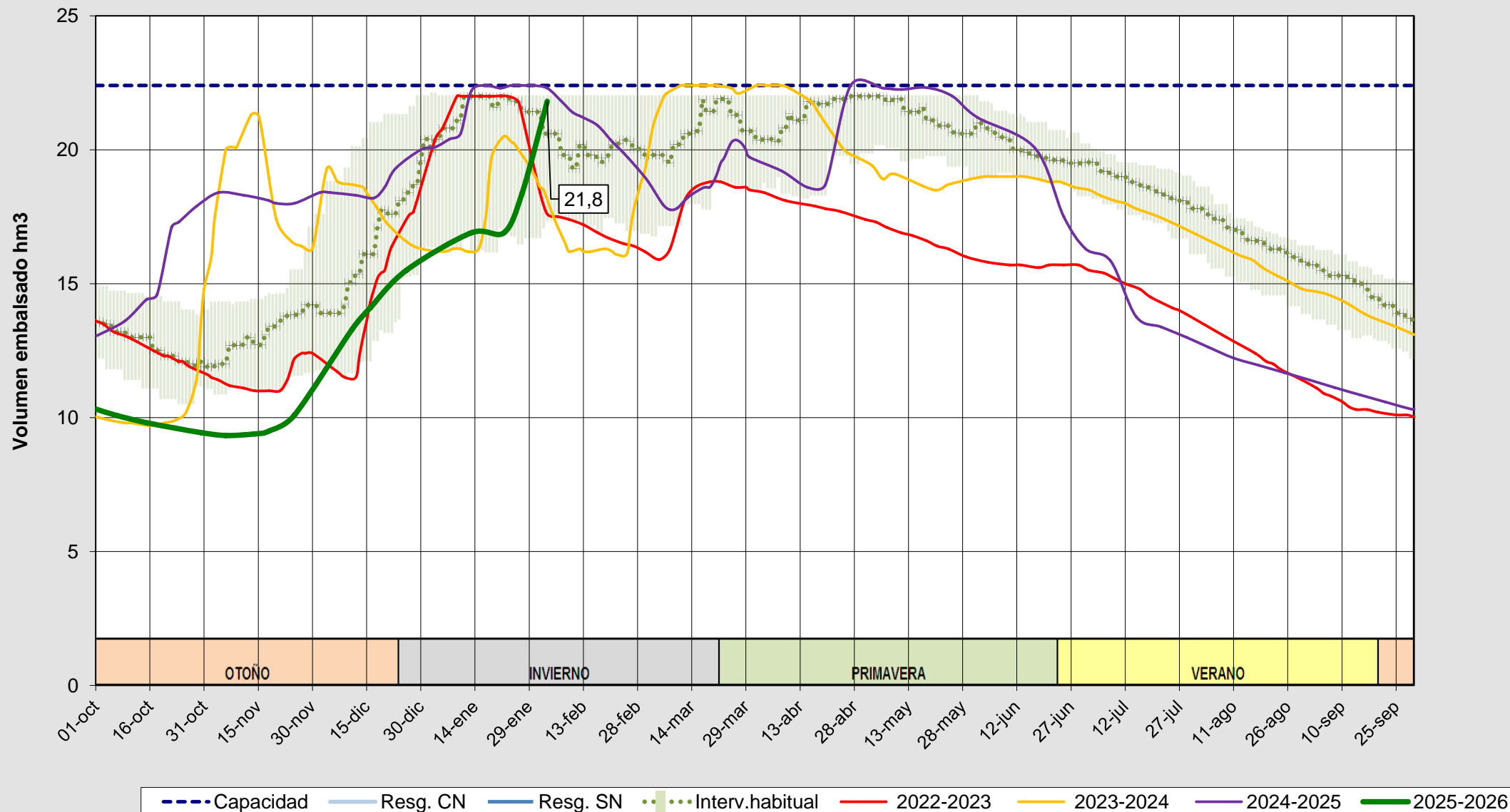
Evolución del volumen almacenado en el embalse de Arlanzón a fecha 03/02/2026
