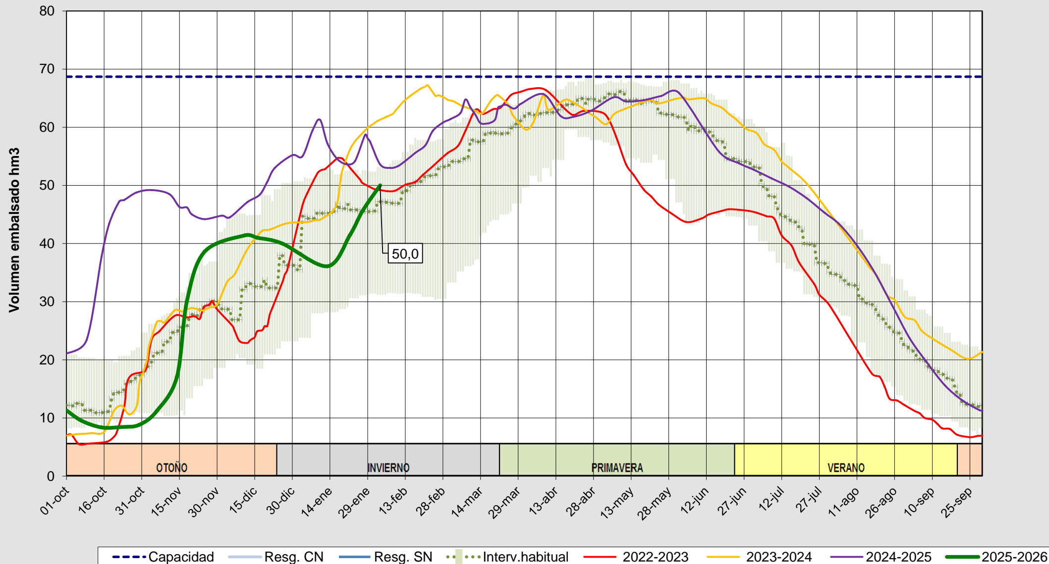
Evolución del volumen almacenado en el embalse de Camporredondo a fecha 03/02/2026
