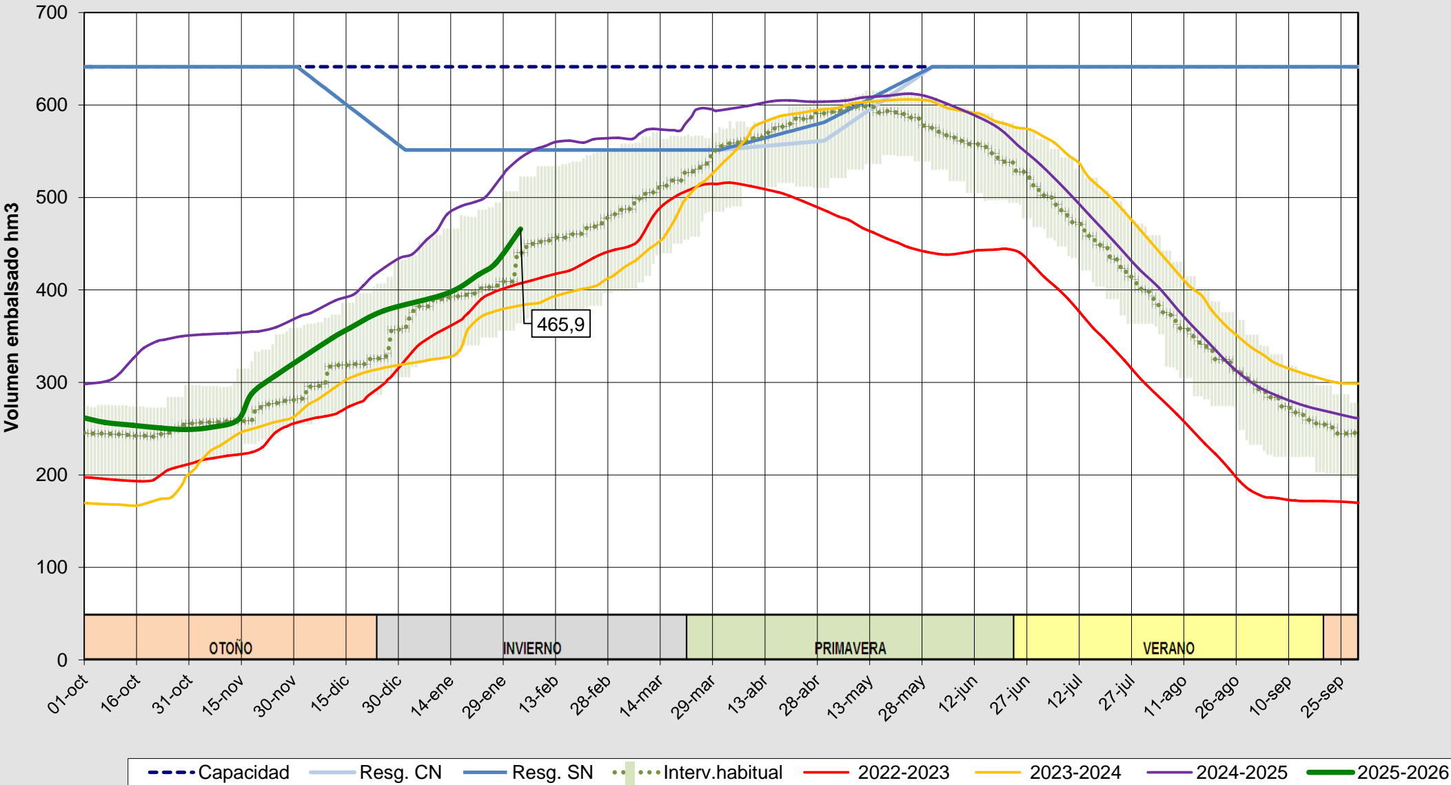
Evolución del volumen almacenado en el embalse de Riaño a fecha 03/02/2026
