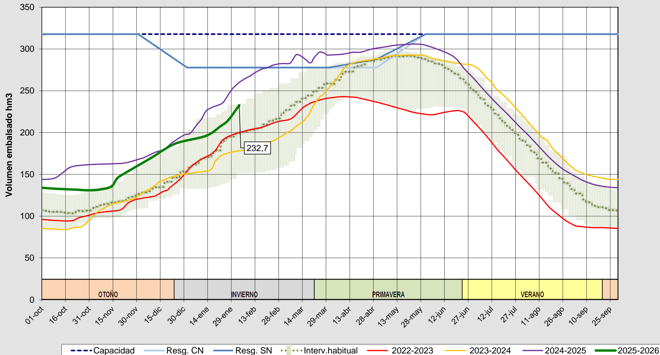
Evolución del volumen almacenado en el embalse de Porma a fecha 03/02/2026
