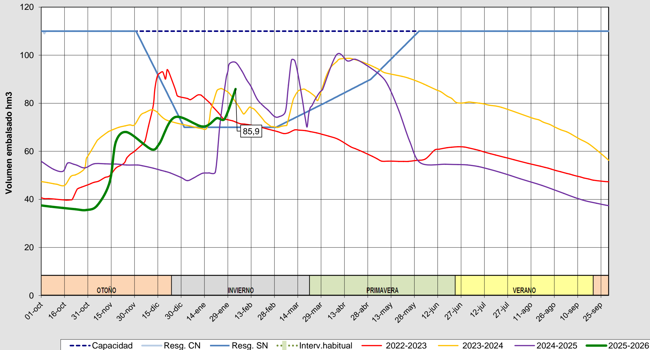
Evolución del volumen almacenado en el embalse de Irueña a fecha 03/02/2026
