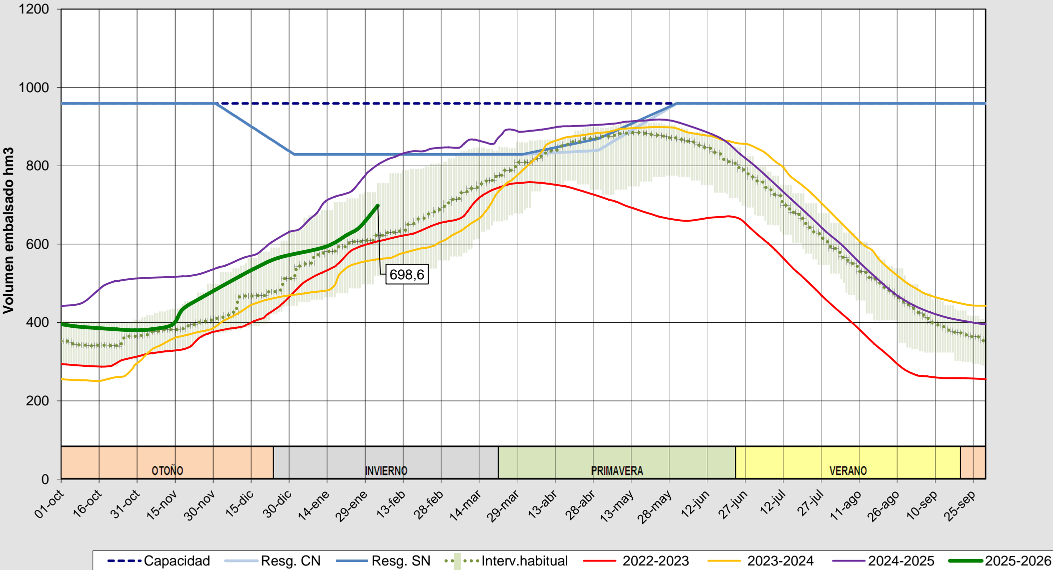
Evolución del volumen almacenado en el sistema del PORMA-ESLA a fecha 03/02/2026
