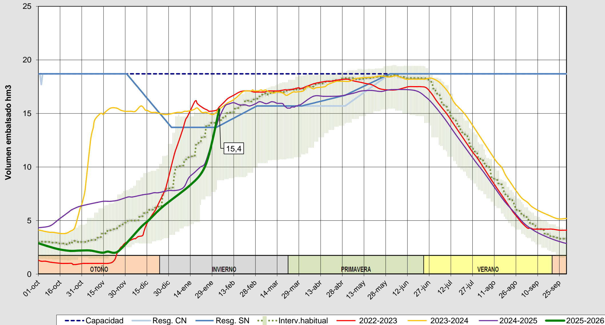
Evolución del volumen almacenado en el embalse de Villameca a fecha 03/02/2026
