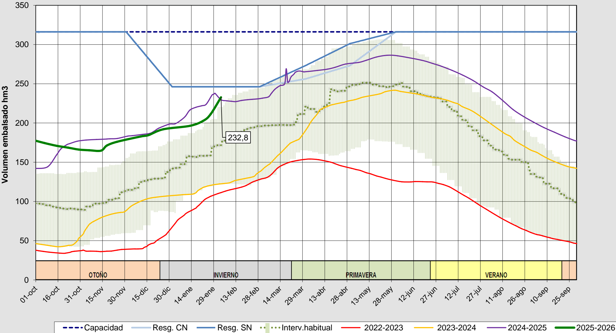
Evolución del volumen almacenado en el sistema del PISUERGA a fecha 03/02/2026
