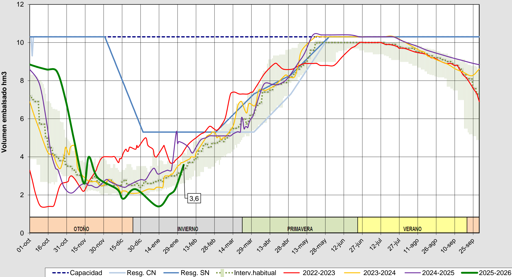
Evolución del volumen almacenado en el embalse de Cervera a fecha 03/02/2026
