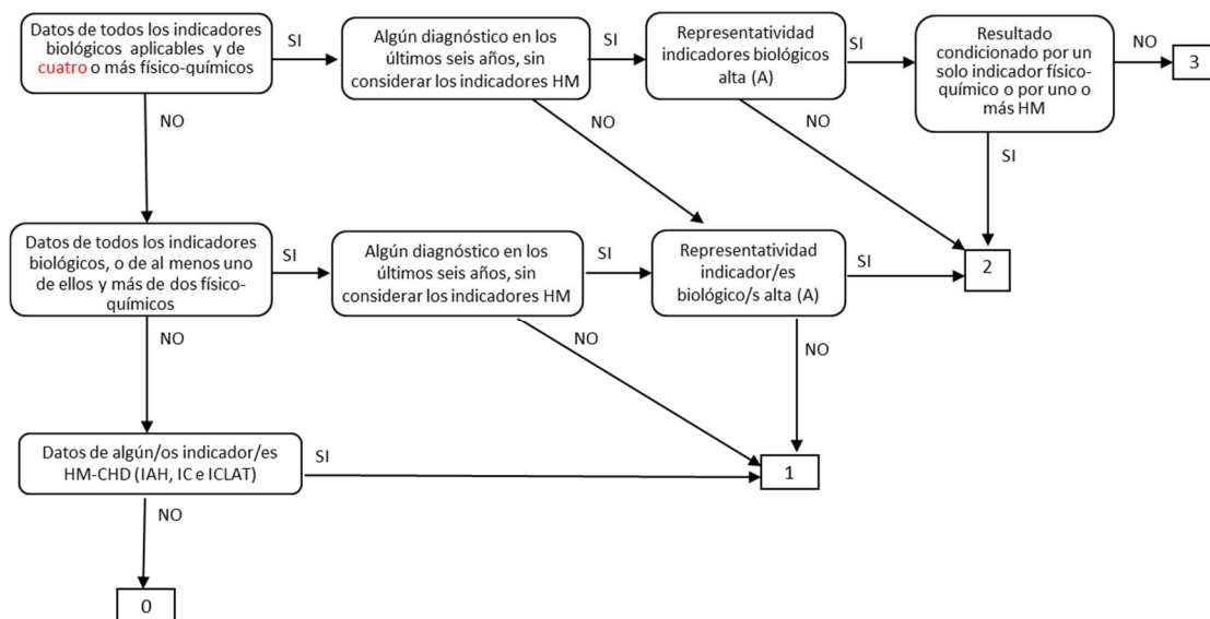
Figura 3. Esquema de estimación del nivel de confianza asociado al estado o potencial ecológico.
