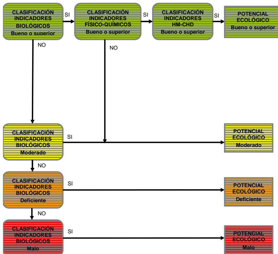
Figura 4. Esquema de clasificación del potencial ecológico en masas de agua embalse.
