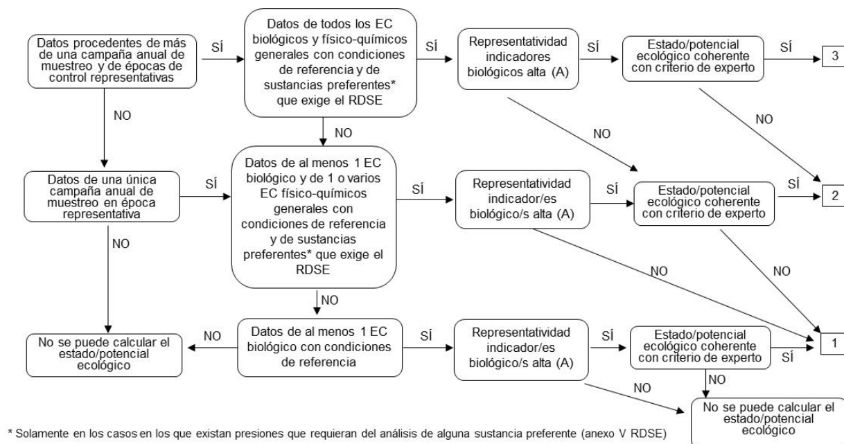
Figura 9. Esquema estimación nivel de confianza en lagos.
