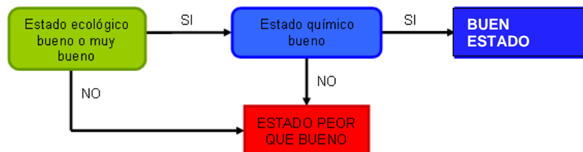
Figura 11. Esquema de clasificación del estado de las masas de agua superficial naturales.
