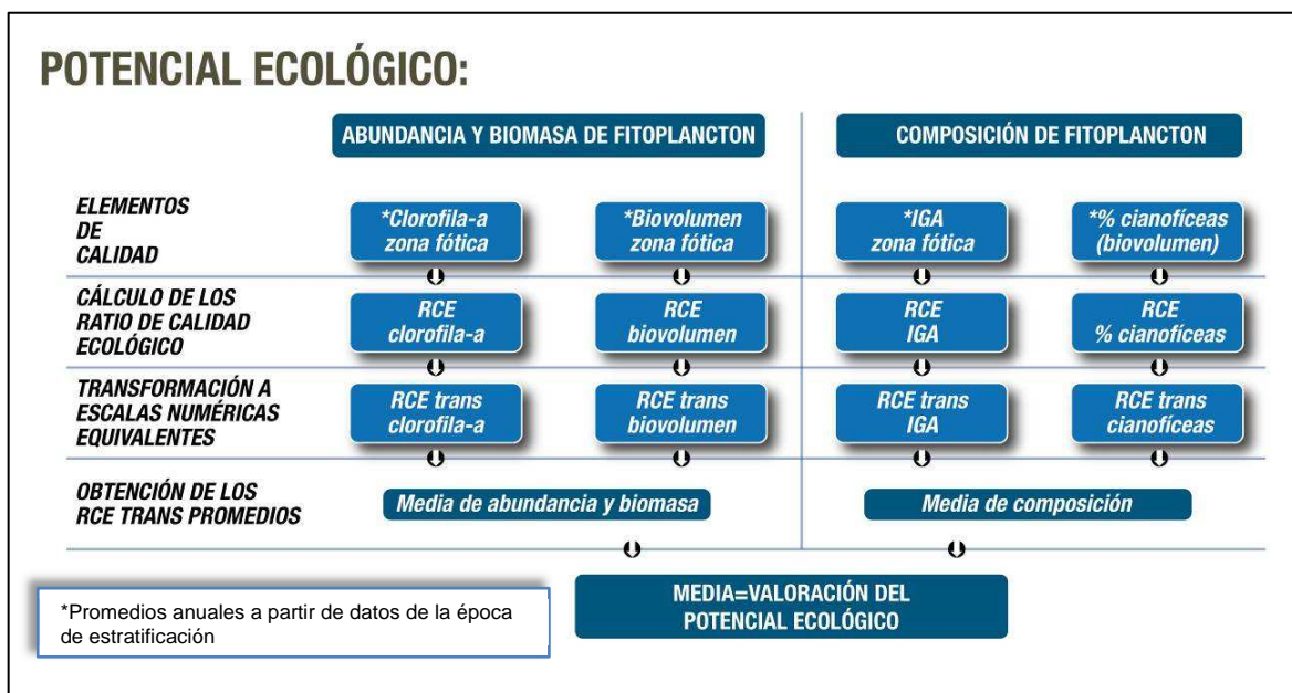
Figura 5. Esquema del procedimiento a seguir para la valoración del potencial ecológico.
