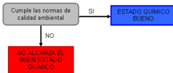
Figura 10. Esquema de clasificación del estado químico para masas de agua superficial.
