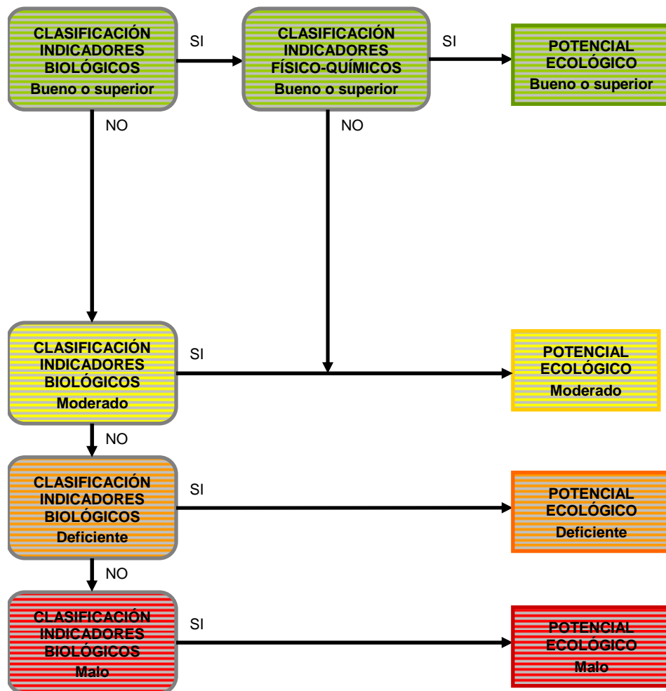
Figura 2. Esquema de clasificación del potencial ecológico en masas de agua artificiales asimilables a ríos.
