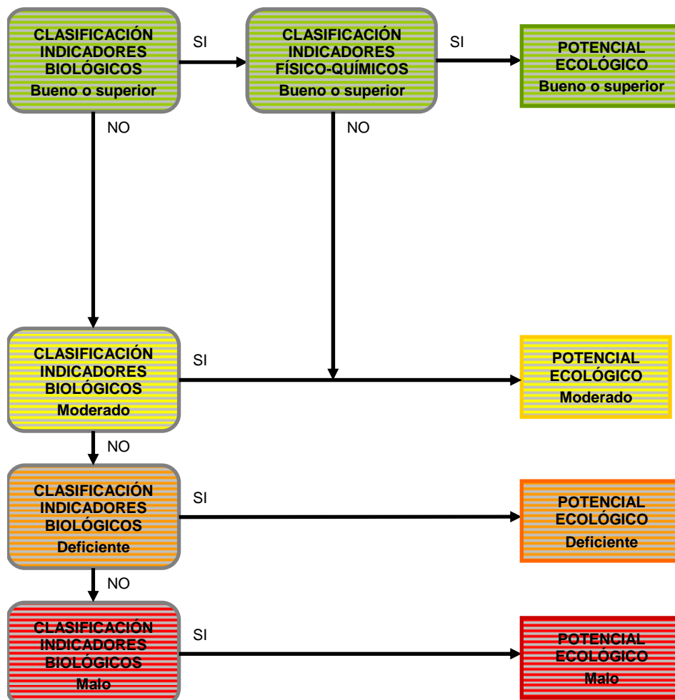
Figura 8. Esquema clasificación del potencial ecológico en lagos muy modificados.
