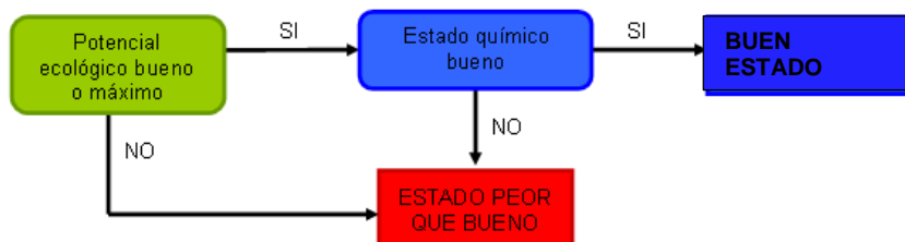
Figura 12. Esquema de clasificación del estado de las masas de agua superficial artificiales o muy modificadas.
