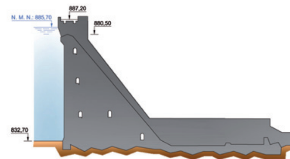
SECCIÓN TIPO
