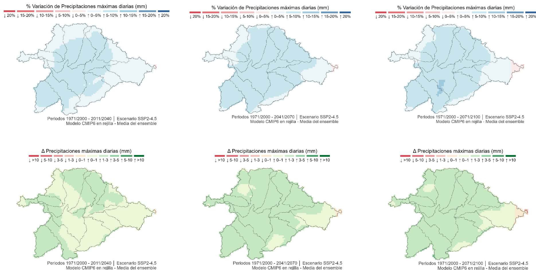
Figura 63. Variación de las precipitaciones máximas diarias proyectadas bajo el escenario intermedio de emisiones (SSP2-4.5), para los horizontes temporales 2011-2040, 2041-2070 y 2071-2100, en comparación con el periodo de control 1971-2000. Fuente: elaboración propia a partir de información de AdaptecCa
