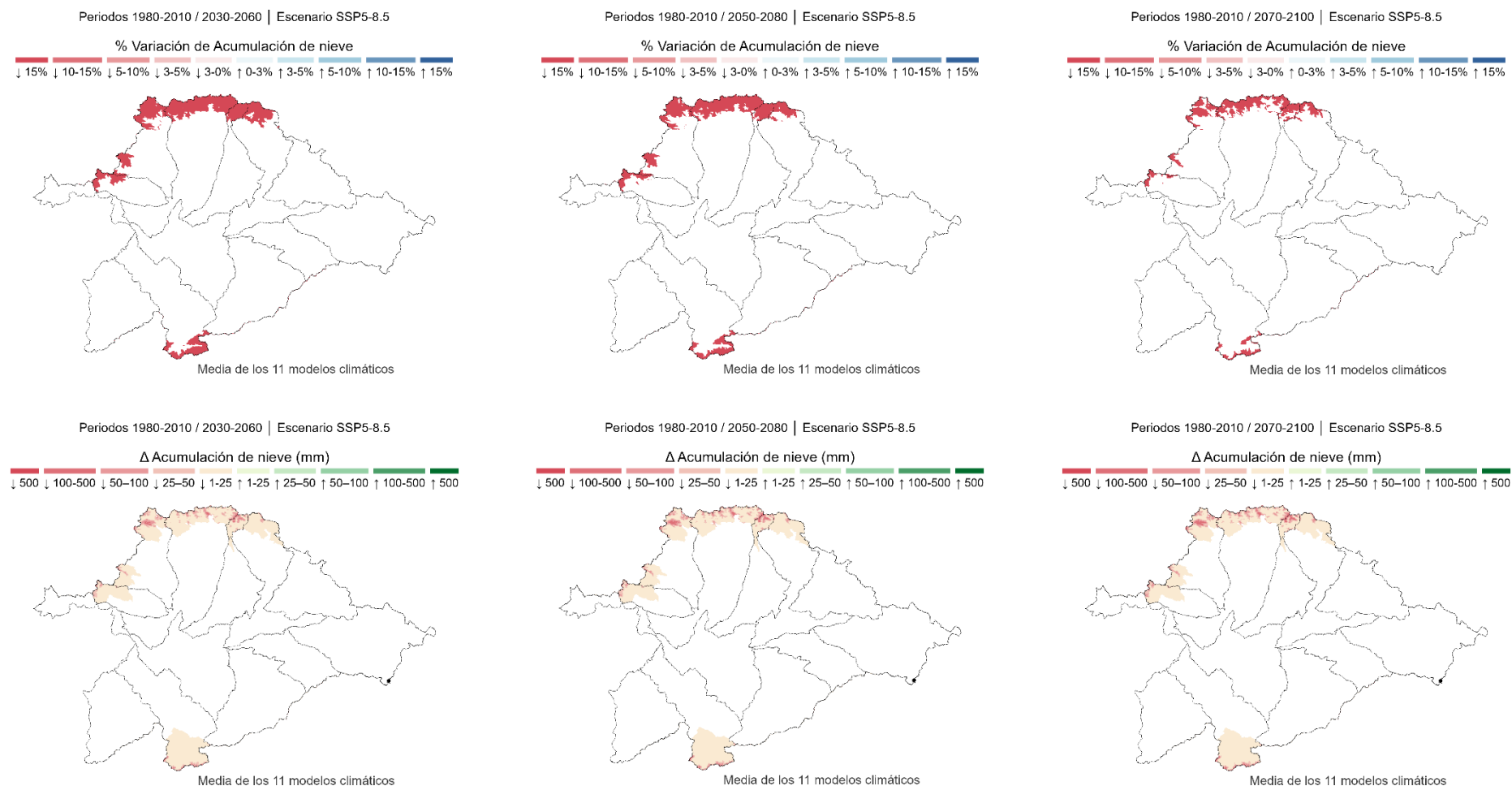
Figura 55. Variación del volumen de nieve almacenado proyectado bajo el escenario pesimista de emisiones (SSP5-8.5), para los horizontes temporales 2030-2060, 2050-2080 Y 2070-2100, en comparación con el periodo de control 1980-2010. Fuente: Elaboración propia a partir de información del CEDEX, 2025.
