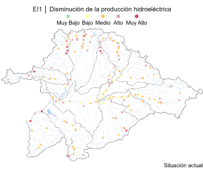
Figura 132. Riesgo EI1: Mapa de situación actual (periodo 1980/81 – 2022/23)
