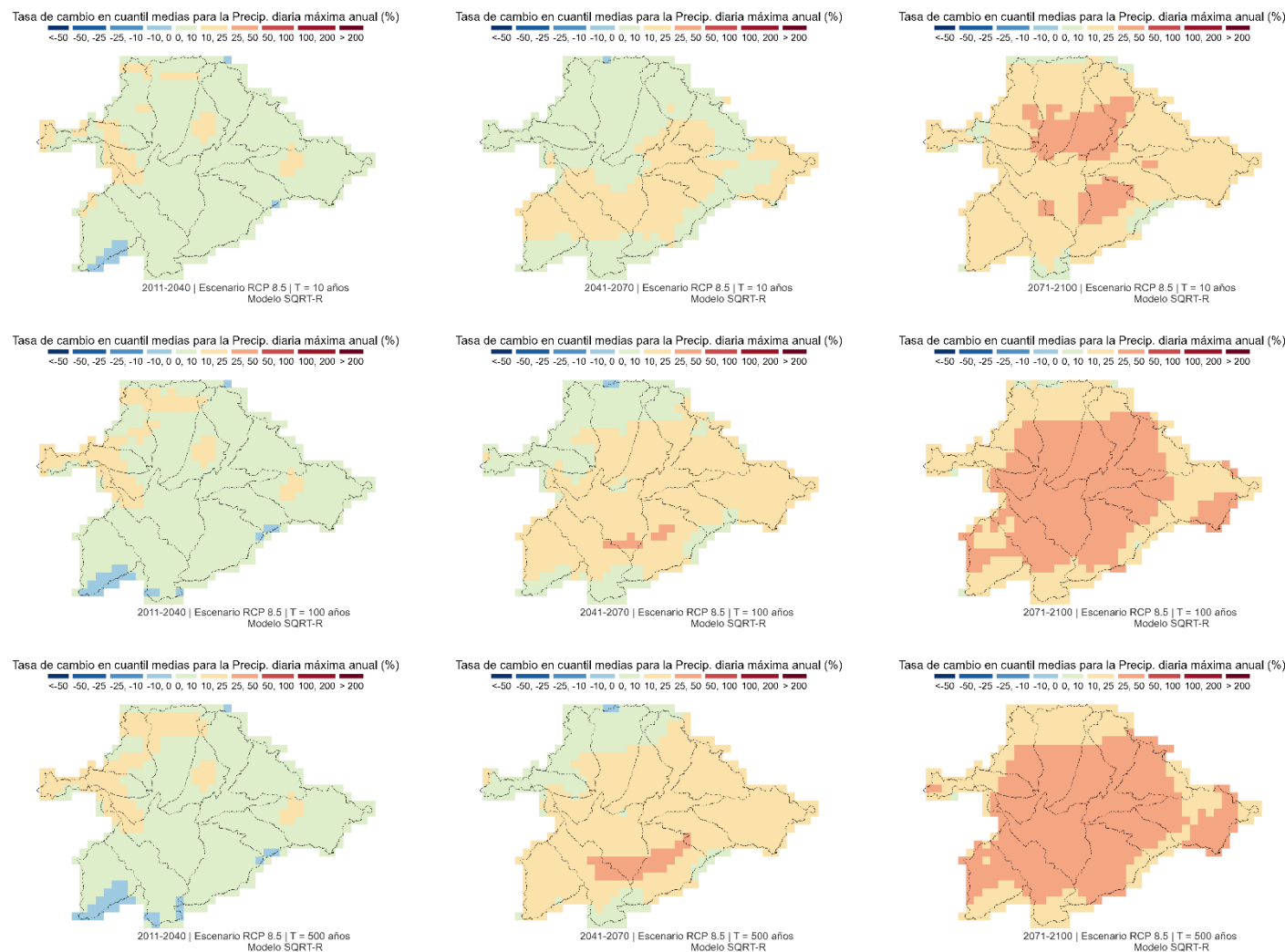
Figura 61. Tasa de cambio de la precipitación diaria máxima anual proyectada bajo el escenario de altas emisiones (SSP5-8.5) (RCP 8.5) para los horizontes temporales 2011-2040, 2041-2070 y 2071-2100, y para los periodos de retorno de 10, 100 y 500 años, calculada respecto al periodo de control (1971-2000). Fuente: elaboración propia a partir de información del CEDEX
