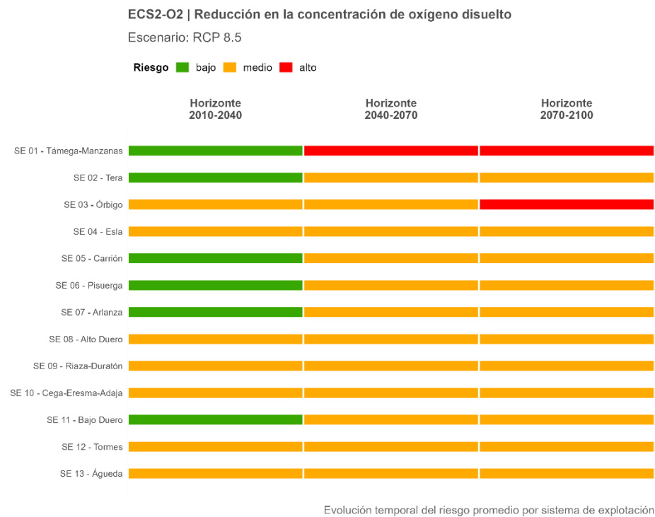
Figura 100. Trayectoria temporal del riesgo ECS2-O2 promedio por sistema de explotación, proyectado bajo el escenario de altas emisiones (RCP 8.5).
