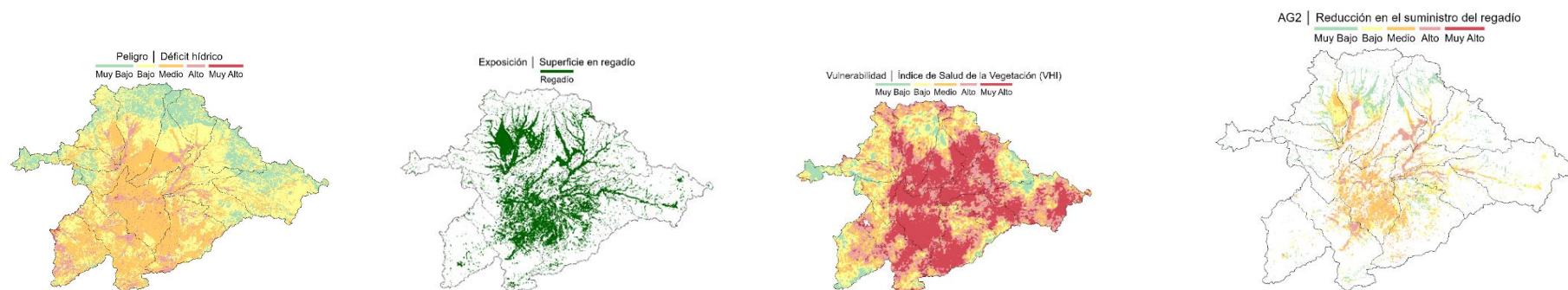
Figura 5. Riesgo AG2. Reducción de la garantía de suministro del regadío. Mapas de los indicadores de peligro, exposición y vulnerabilidad Mapa de situación (periodo 1980/81-2022/23)
