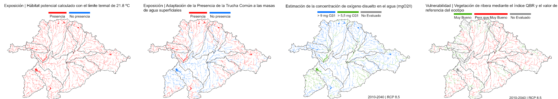
Figura 93. Riesgo ECS2. Mapas de Exposición: hábitat potencial calculado con el límite térmico de 21.8 °C y adaptación de la presencia de la Trucha común a las masas de agua superficiales (Atlas y Libro Rojo de los Peces, MMA, 2001). Mapa de la estimación de la concentración de oxígeno disuelto en agua (mgO 2 /l) calculada en función de la temperatura y la altitud en el mes de agosto. Mapa de Vulnerabilidad en base a la vegetación de ribera mediante el índice QBR y el valor de referencia del ecotipo.
