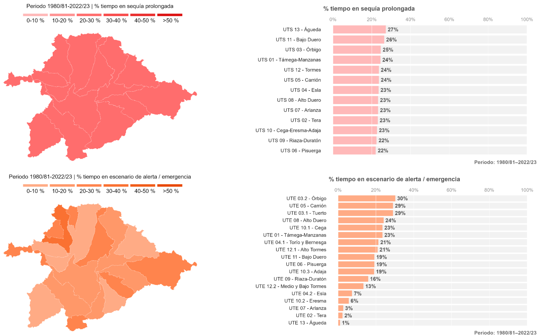
Figura 36. Caracterización espacial y temporal de la sequía prolongada y escasez coyuntural. Fuente: elaboración a partir de los informes mensuales de seguimiento de los PES. La UTS con mayor porcentaje de tiempo en sequía prolongada es la UTS 13 - Águeda (27%), mientras que las que presentan el menor porcentaje son las UTS 09 y UTS 06. En cuanto a los escenarios de alerta o emergencia, la UTE con mayor porcentaje de tiempo en estas situaciones es la UTE 03.2 (30%) y la que registra el menor porcentaje es la UTE 13 (1%).
