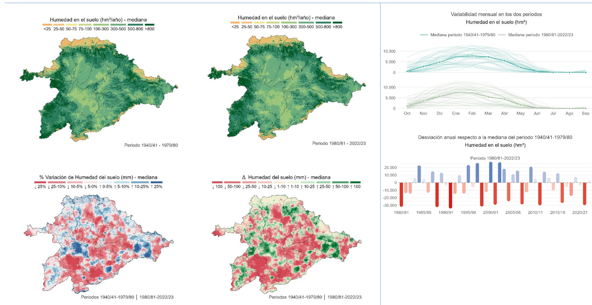
Figura 26. Caracterización espacial y temporal de la humedad en el suelo. Comparación entre los periodos 1940/41–1979/80 y 1980/81–2022/23. Fuente: Elaboración propia a partir de información de SIMPA (CEDEX).
