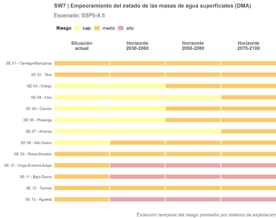
Figura 86. Trayectoria temporal del riesgo SW7 promedio por sistema de explotación, proyectado bajo el escenario de altas emisiones (SSP5-8.5).
