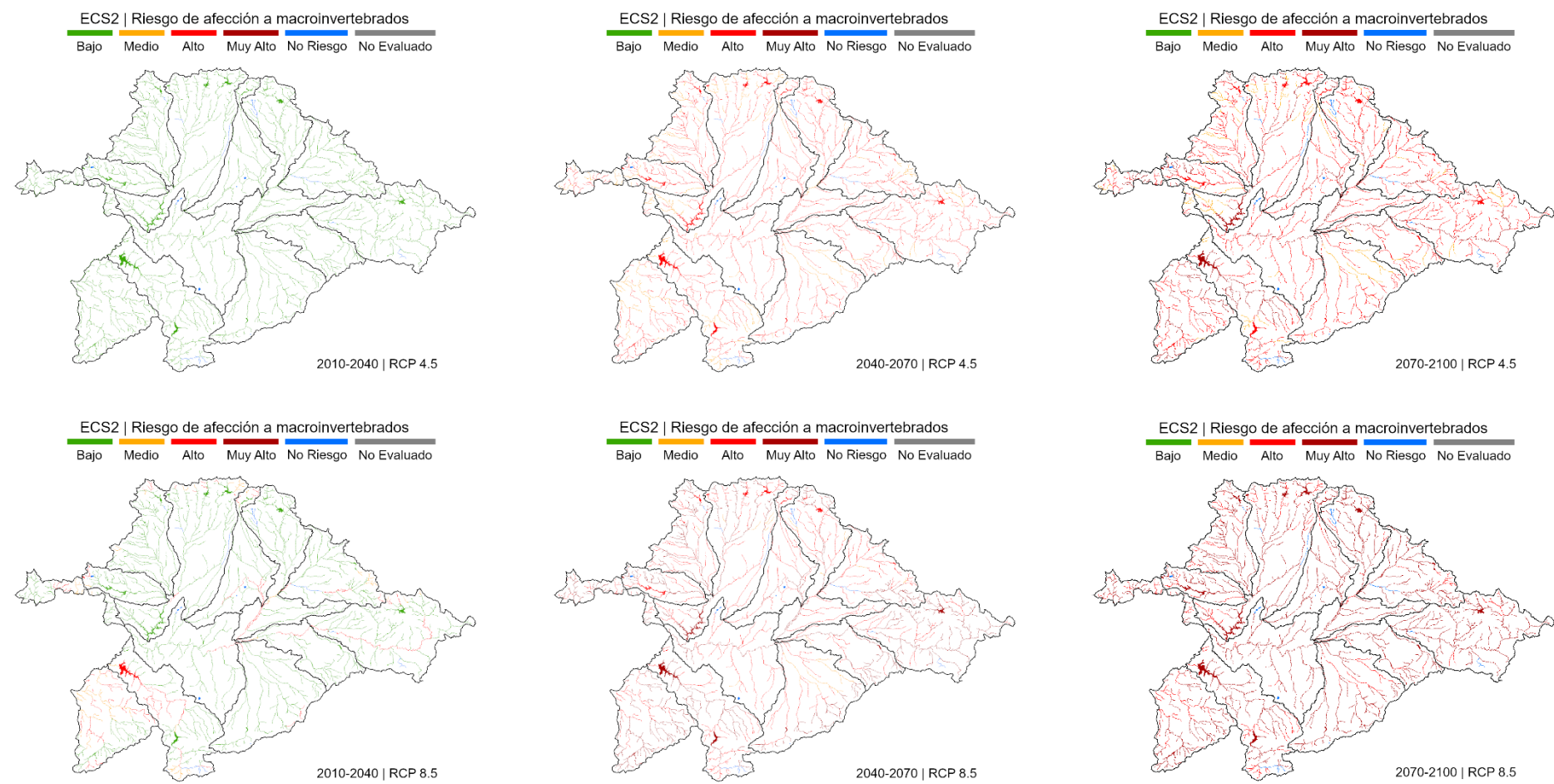
Figura 96. Evaluación del riesgo ECS2 proyectado bajo los escenarios RCP 4.5 y RCP 8.5, para los horizontes temporales 2010-2040, 2040-2070 y 2070/2100. Riesgo de afección a macroinvertebrados.
