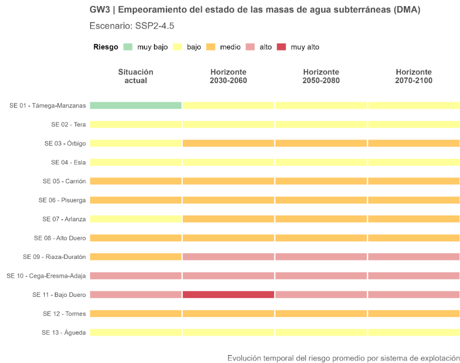
Figura 91. Trayectoria temporal del riesgo GW3 promedio por sistema de explotación, proyectado bajo el escenario intermedio (SSP2-4.5).
