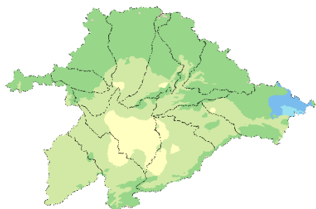
Clasificación climática de Köppen-Geiger (2011-2040) | Escenario SSP5-8.5
