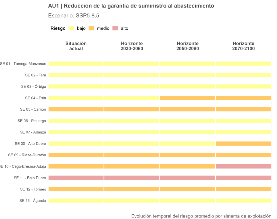
Figura 124. Trayectoria temporal del riesgo AU1 promedio por sistema de explotación, proyectado bajo el escenario de altas emisiones (SSP5-8.5).
