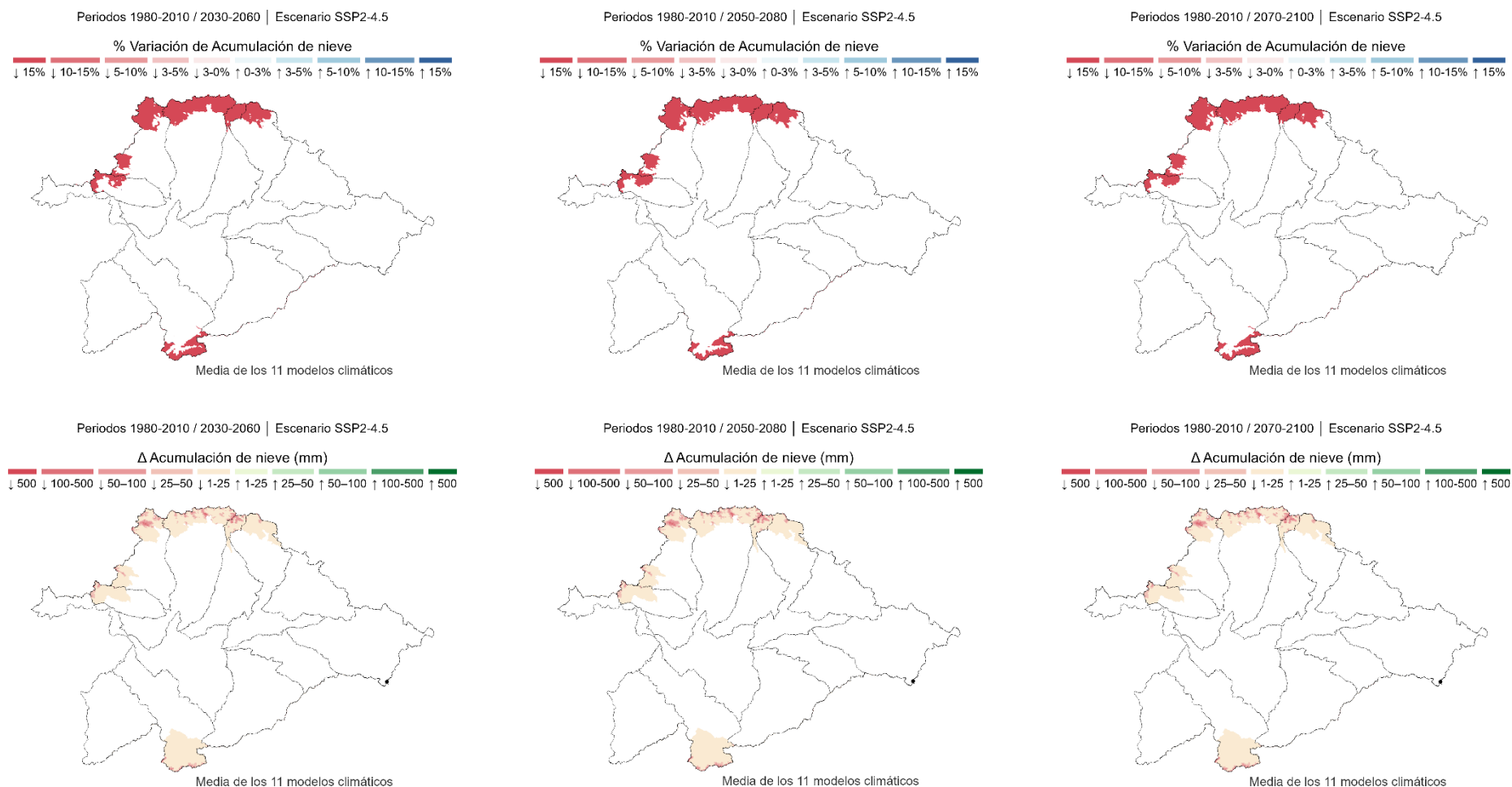
Figura 54. Variación del volumen de nieve almacenado proyectado bajo el escenario intermedio de emisiones (SSP2-4.5), para los horizontes temporales 2030-2060, 2050-2080 Y 2070-2100, en comparación con el periodo de control 1980-2010. Fuente: Elaboración propia a partir de información del CEDEX, 2025.
