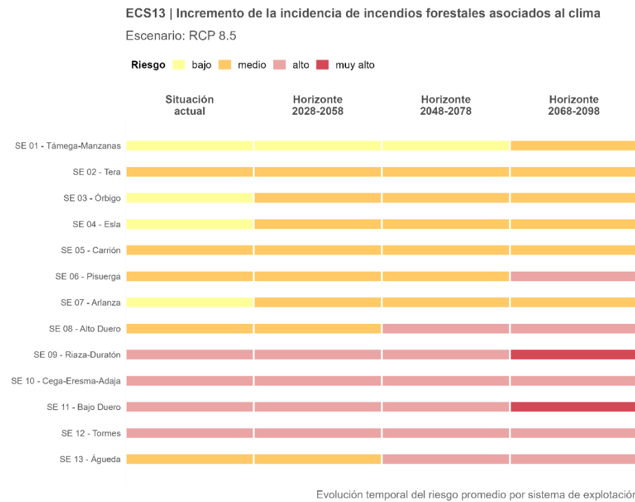
Figura 118. Trayectoria temporal del riesgo ECS13 promedio por sistema de explotación, proyectado bajo el escenario de altas emisiones (SSP5-8.5).
