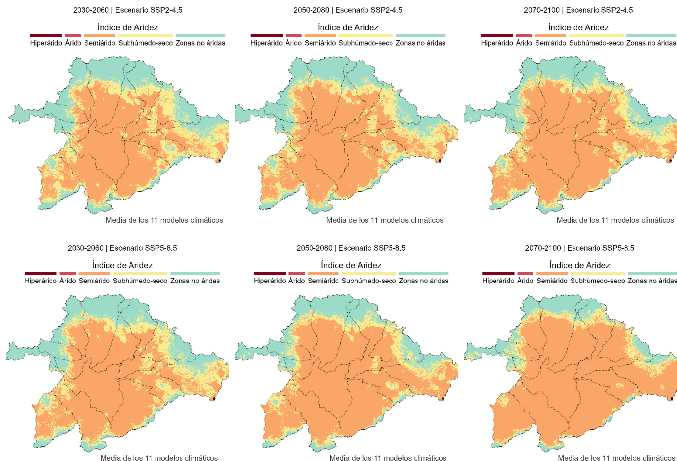
Figura 67. Variación del índice de aridez para diversos horizontes temporales y escenarios climáticos. Fuente: elaboración propia a partir de proyecciones SIMPA (CEDEX)
