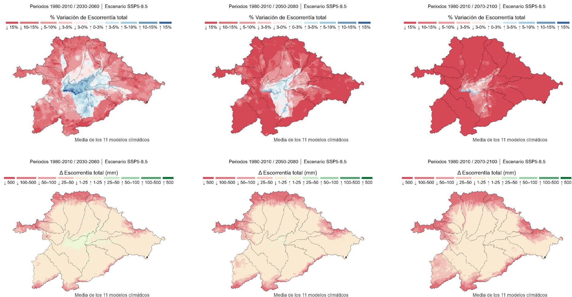
Figura 59. Variación de las aportaciones totales proyectadas bajo el escenario de altas emisiones (SSP5-8.5), para los horizontes temporales 2030-2060, 2050-2080 Y 2070-2100, en comparación con el periodo de control 1980-2010. Fuente: Elaboración propia a partir de información del CEDEX, 2025.
