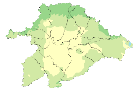
Clasificación climática de Köppen-Geiger (2071-2100) | Escenario SSP5-8.5
