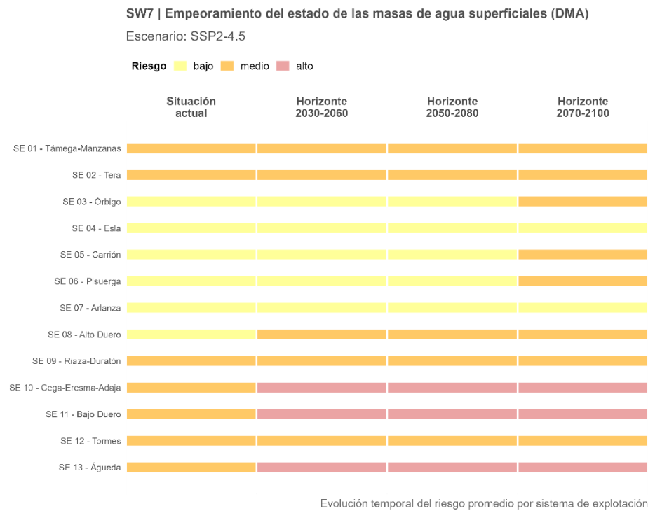
Figura 85. Trayectoria temporal del riesgo SW7 promedio por sistema de explotación, proyectado bajo el escenario intermedio (SSP2-4.5).
