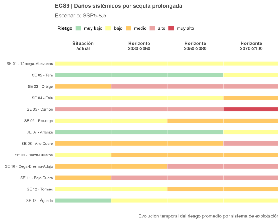
Figura 110. Trayectoria temporal del riesgo ECS9 promedio por sistema de explotación, proyectado bajo el escenario de altas emisiones (SSP5-8.5).
