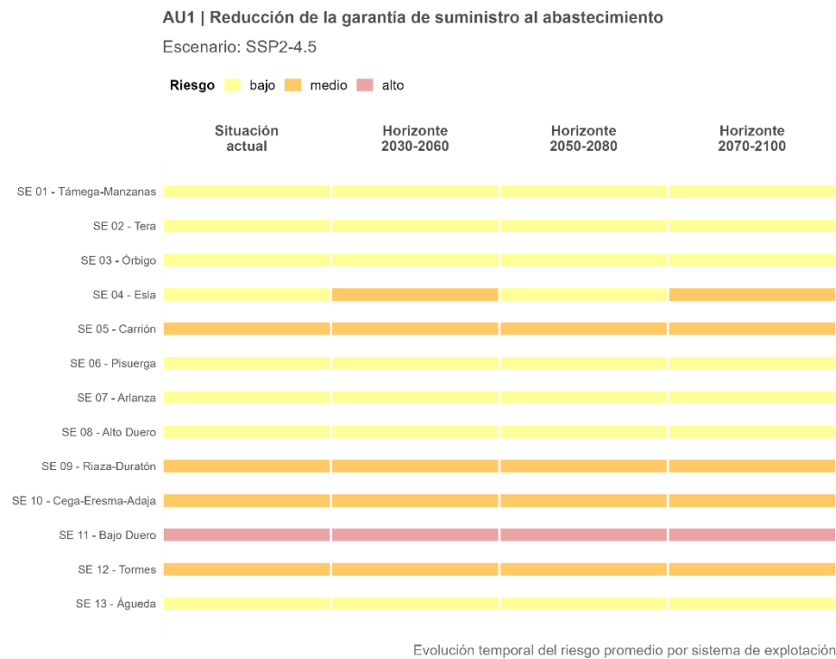
Figura 123. Trayectoria temporal del riesgo AU1 promedio por sistema de explotación, proyectado bajo el escenario intermedio (SSP2-4.5).
