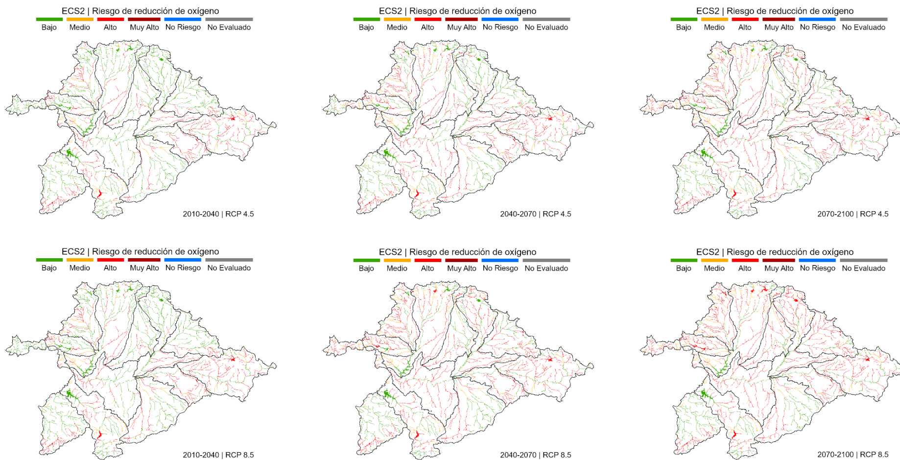
Figura 95. Evaluación del riesgo ECS2 proyectado bajo los escenarios RCP 4.5 y RCP 8.5, para los horizontes temporales 2010-2040, 2040-2070 y 2070/2100. Riesgo de reducción de oxígeno.
