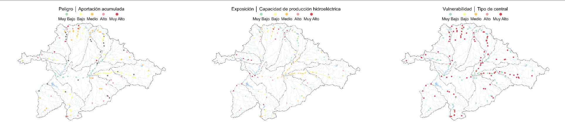
Figura 131. Riesgo EI1. Mapas de los indicadores de peligro, exposición y vulnerabilidad
