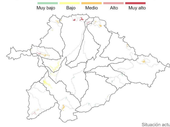
Figura 104. Riesgo ECS8: Mapa de situación actual (periodo 1980/81 – 2022/23)
