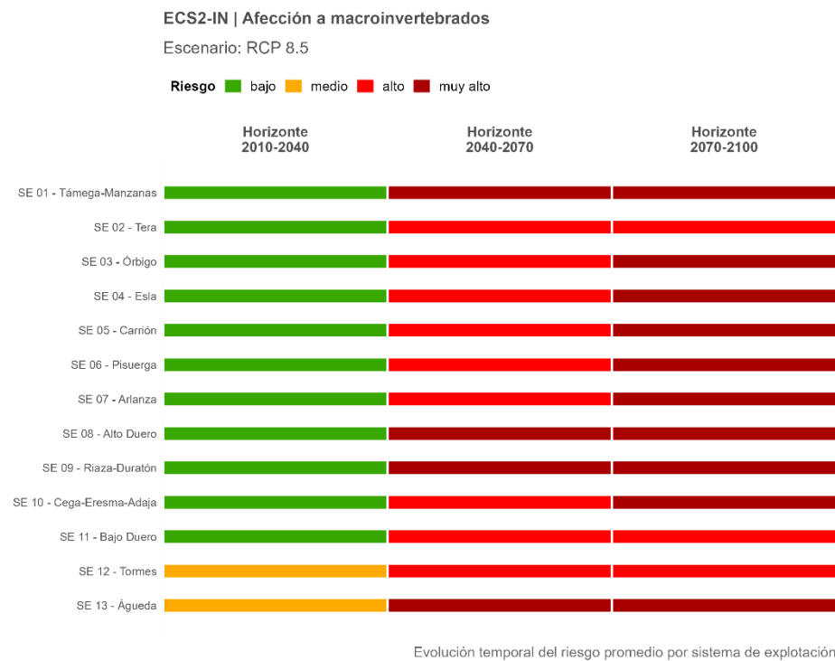
Figura 102. Trayectoria temporal del riesgo ECS2-IN promedio por sistema de explotación, proyectado bajo el escenario de altas emisiones (RCP 8.5).
