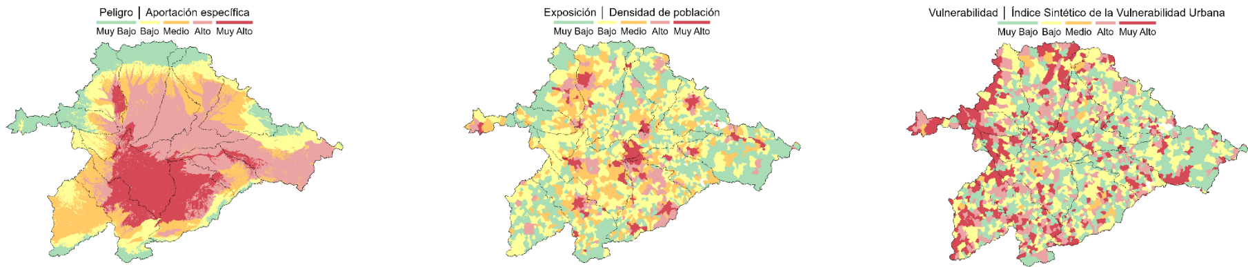
Figura 119. Riesgo AU1. Mapas de los indicadores de peligro, exposición y vulnerabilidad, sin tener en cuenta el efecto de regulación de las infraestructuras existentes.
