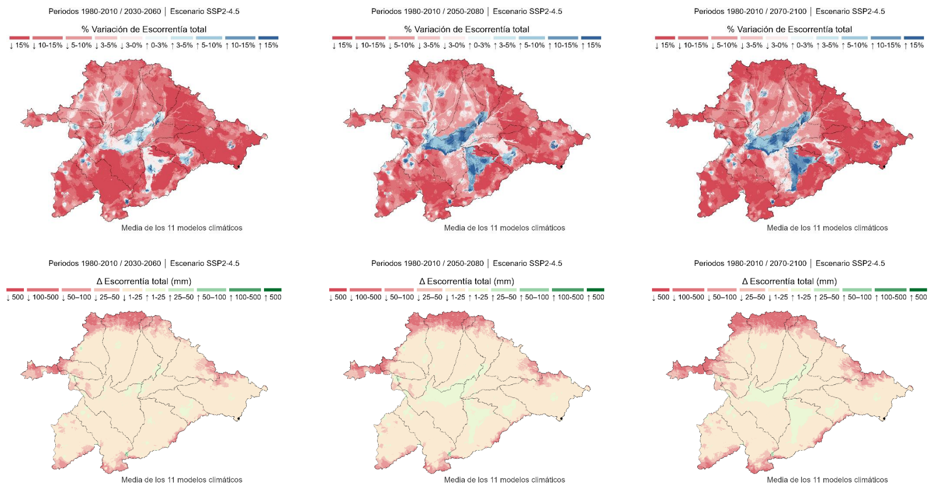
Figura 58. Variación de las aportaciones totales proyectadas bajo el escenario intermedio de emisiones (SSP2-4.5), para los horizontes temporales 2030-2060, 2050-2080 Y 2070-2100, en comparación con el periodo de control 1980-2010. Fuente: Elaboración propia a partir de información del CEDEX, 2025.
