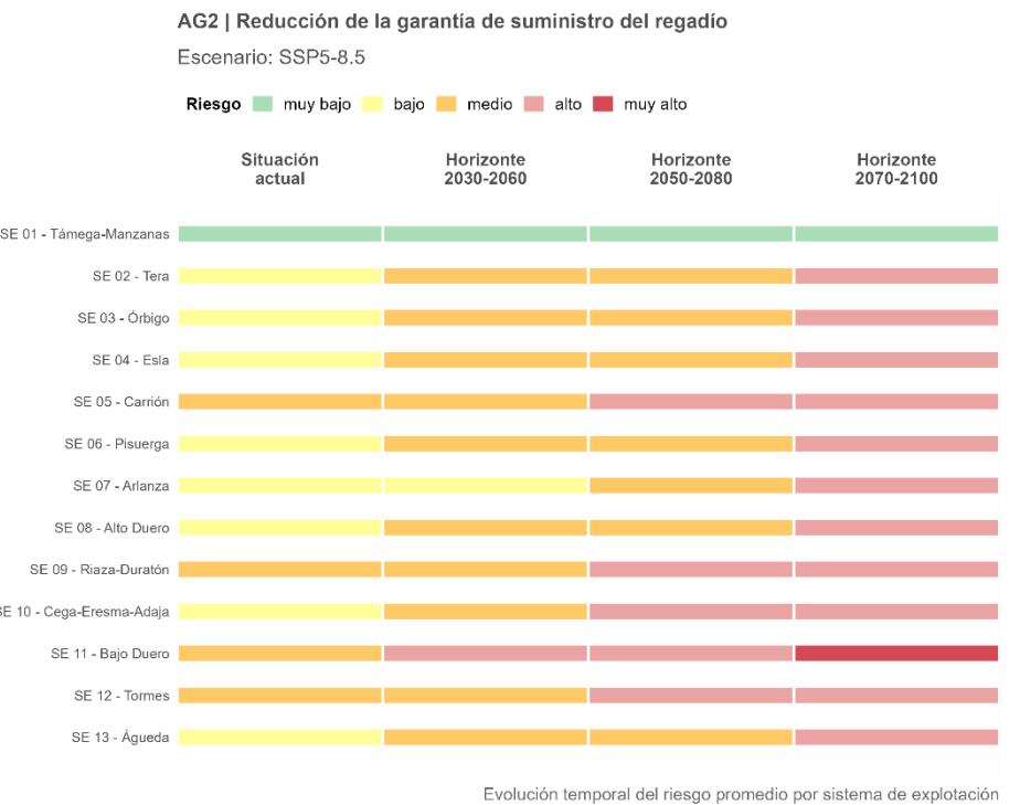
Figura 130. Trayectoria temporal del riesgo AG2 promedio por sistema de explotación, proyectado bajo el escenario de altas emisiones (SSP5-8.5).
