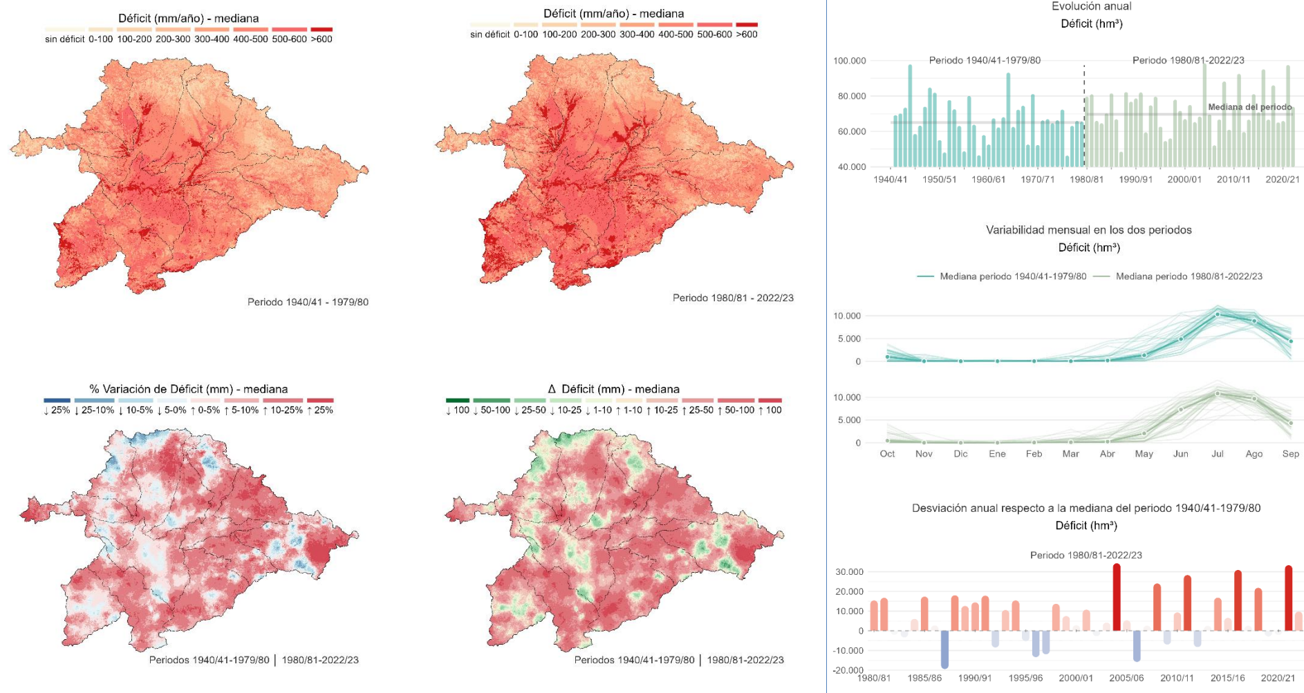
Figura 28. Caracterización espacial y temporal del estrés hídrico (ETP-ETR). Comparación entre los periodos 1940/41-1979/80 y 1980/81-2022/23. Fuente: Elaboración propia a partir de información de SIMPA (CEDEX).
