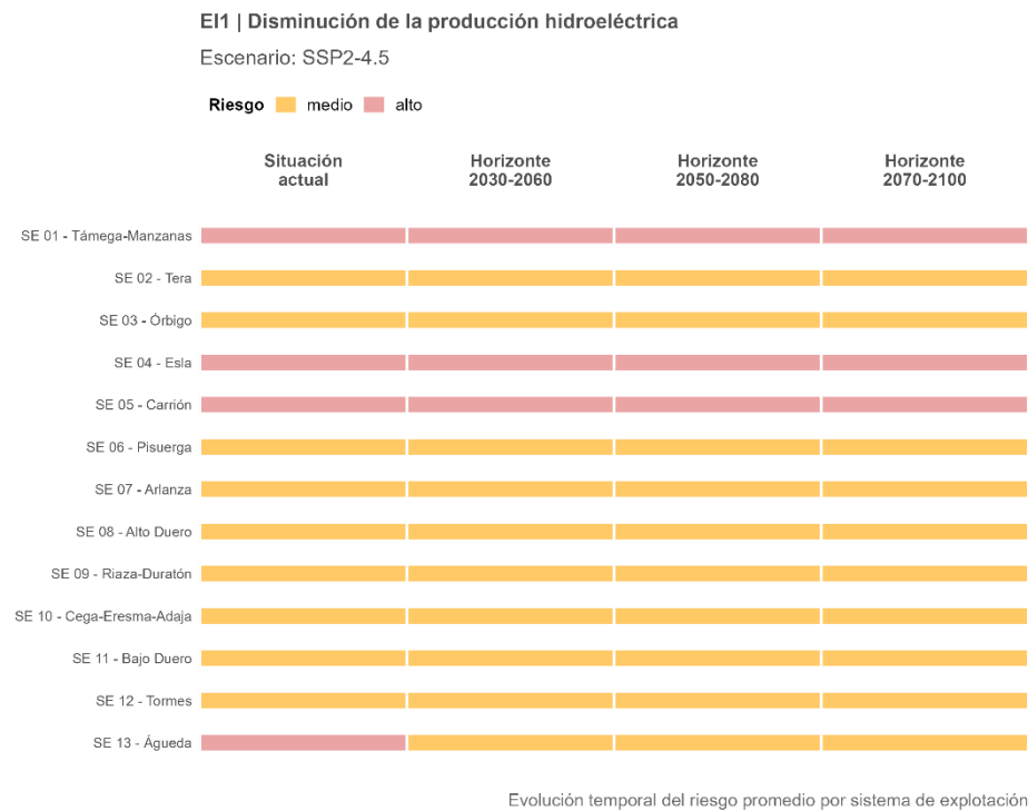
Figura 135. Trayectoria temporal del riesgo EI1 promedio por sistema de explotación, proyectado bajo el escenario intermedio (SSP2-4.5).
