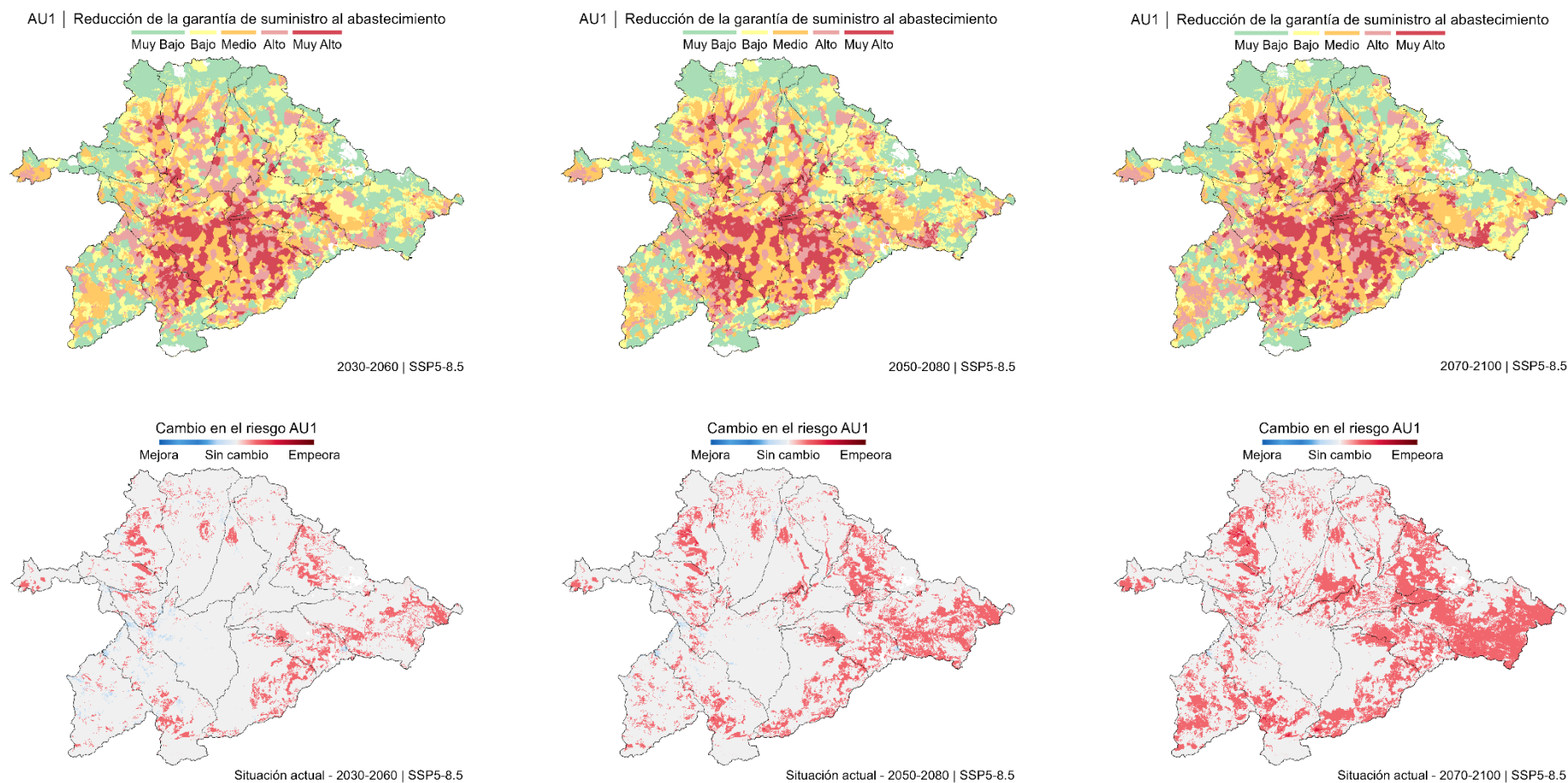
Figura 122. Evaluación del riesgo AU1 proyectado bajo el escenario de altas emisiones (SSP5-8.5), para los horizontes temporales 2030/2060, 2050/2080 y 2070/2100 respecto a la situación de riesgo actual, sin tener en cuenta el efecto de regulación de las infraestructuras existentes.
