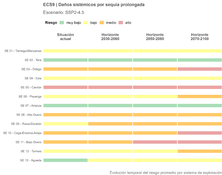
Figura 109. Trayectoria temporal del riesgo ECS9 promedio por sistema de explotación, proyectado bajo el escenario intermedio (SSP2-4.5).
