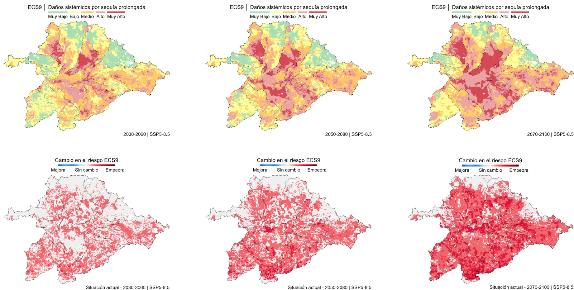
Figura 108. Evaluación del riesgo ECS9 proyectado bajo el escenario de altas emisiones (SSP5-8.5), para los horizontes temporales 2030/2060, 2050/2080 y 2070/2100 respecto a la situación de riesgo actual.
