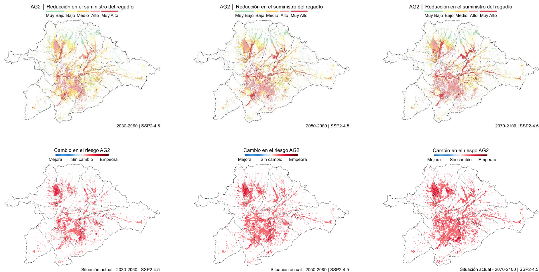
Figura 127. Evaluación del riesgo AG2 proyectado bajo el escenario intermedio (SSP2-4.5), para los horizontes temporales 2030/2060, 2050/2080 y 2070/2100 respecto a la situación de riesgo actual, sin tener en cuenta el efecto de regulación de las infraestructuras existentes.
