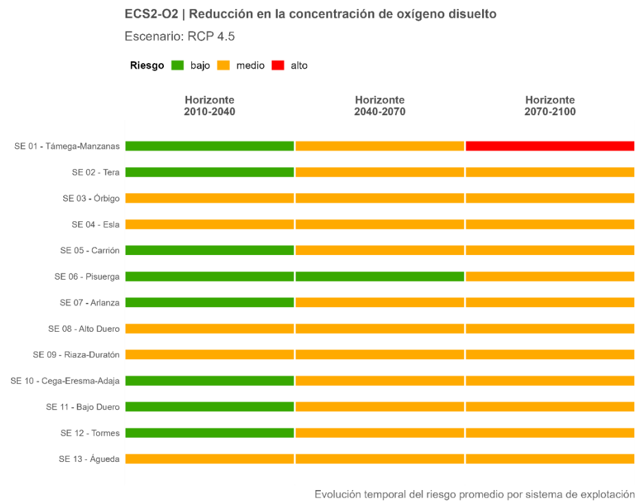
Figura 99. Trayectoria temporal del riesgo ECS2-O2 promedio por sistema de explotación, proyectado bajo el escenario intermedio (RCP 4.5)
