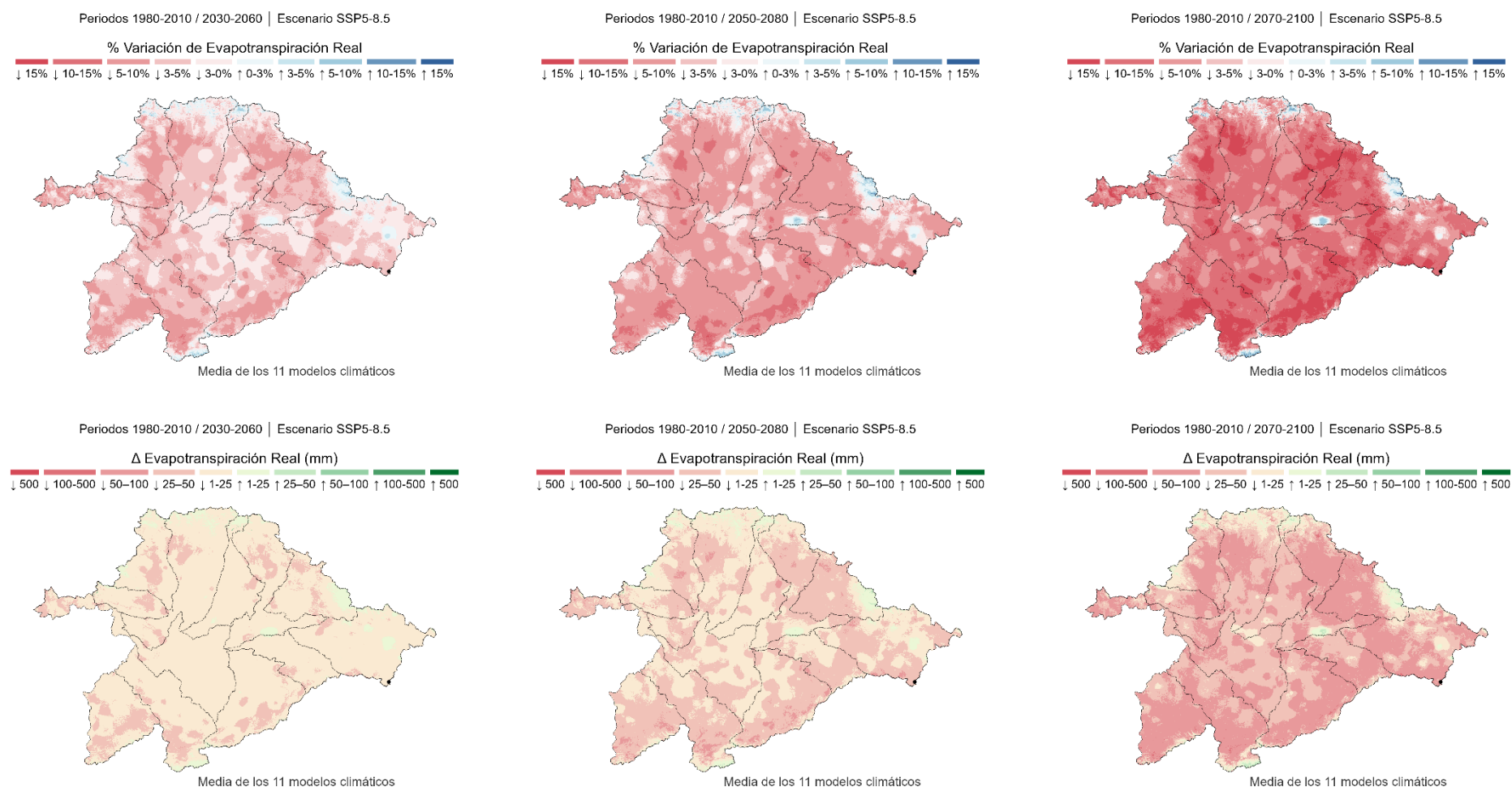
Figura 57. Variación de la evapotranspiración real proyectada bajo el escenario de altas emisiones (SSP5-8.5), para los horizontes temporales 2030-2060, 2050-2080 Y 2070-2100, en comparación con el periodo de control 1980-2010. Fuente: Elaboración propia a partir de información del CEDEX, 2025.
