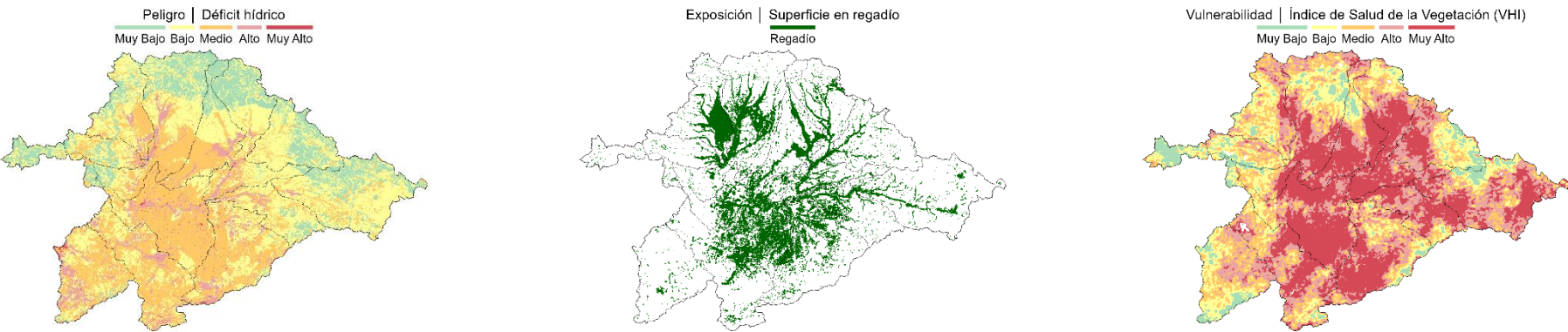
Figura 125. Riesgo AG2. Mapas de los indicadores de peligro, exposición y vulnerabilidad, sin tener en cuenta el efecto de regulación de las infraestructuras existentes
