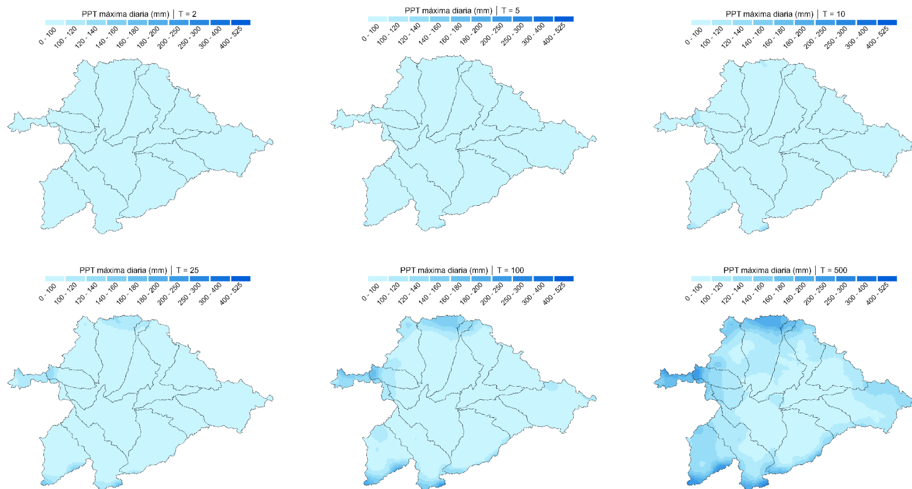
Figura 34. Caracterización espacial de las precipitaciones máximas diarias para los periodos de retorno de 2, 5, 10, 25, 100 y 500 años. Fuente: CAUMAX, 2014.
