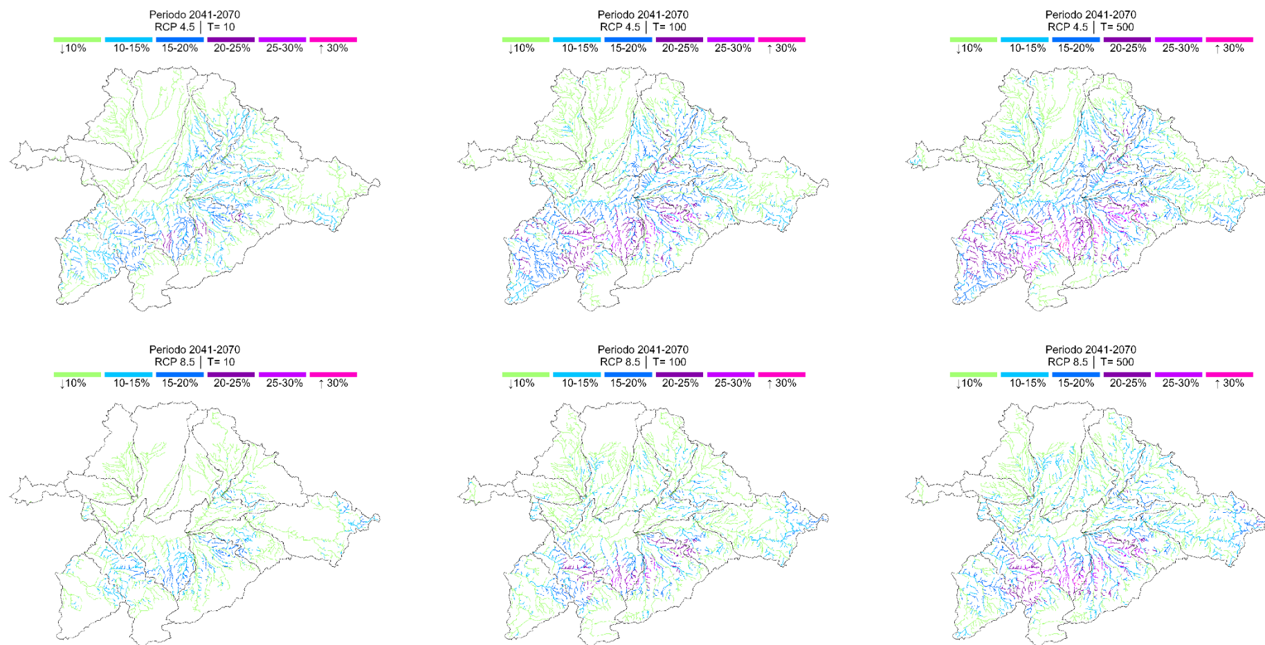
Figura 62. Tasa de cambio de la precipitación máxima acumulada en la red fluvial proyectada bajo los escenarios medio (RCP 4.5) y pesimista (RCP 8.5) de emisiones para el horizonte temporal 2041-2070, y para los periodos de retorno de 10, 100 y 500 años, calculada respecto al periodo de control (1971-2000). Fuente: Elaboración propia a partir de información del CEDEX
