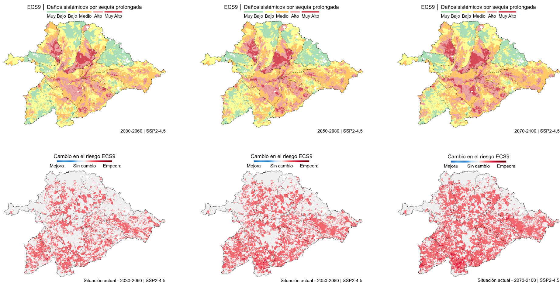
Figura 107. Evaluación del riesgo ECS9 proyectado bajo el escenario intermedio (SSP2-4.5), para los horizontes temporales 2030/2060, 2050/2080 y 2070/2100 respecto a la situación de riesgo actual.
