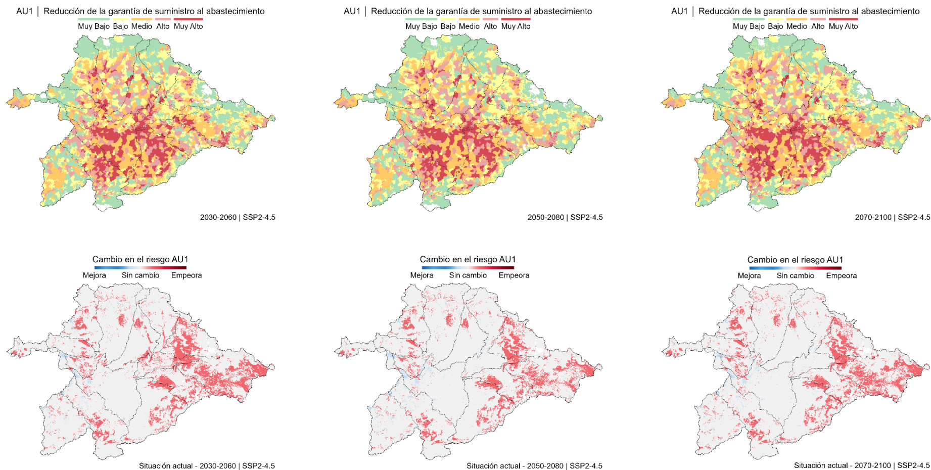
Figura 121. Evaluación del riesgo AU1 proyectado bajo el escenario intermedio (SSP2-4.5), para los horizontes temporales 2030/2060, 2050/2080 y 2070/2100 respecto a la situación de riesgo actual, sin tener en cuenta el efecto de regulación de las infraestructuras existentes.
