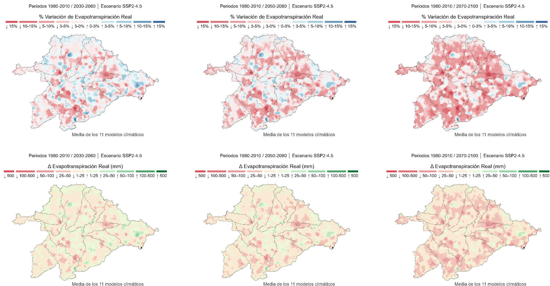
Figura 56. Variación de la evapotranspiración real proyectada bajo el escenario intermedio de emisiones (SSP2-4.5), para los horizontes temporales 2030-2060, 2050-2080 Y 2070-2100, en comparación con el periodo de control 1980-2010. Fuente: Elaboración propia a partir de información del CEDEX, 2025.
