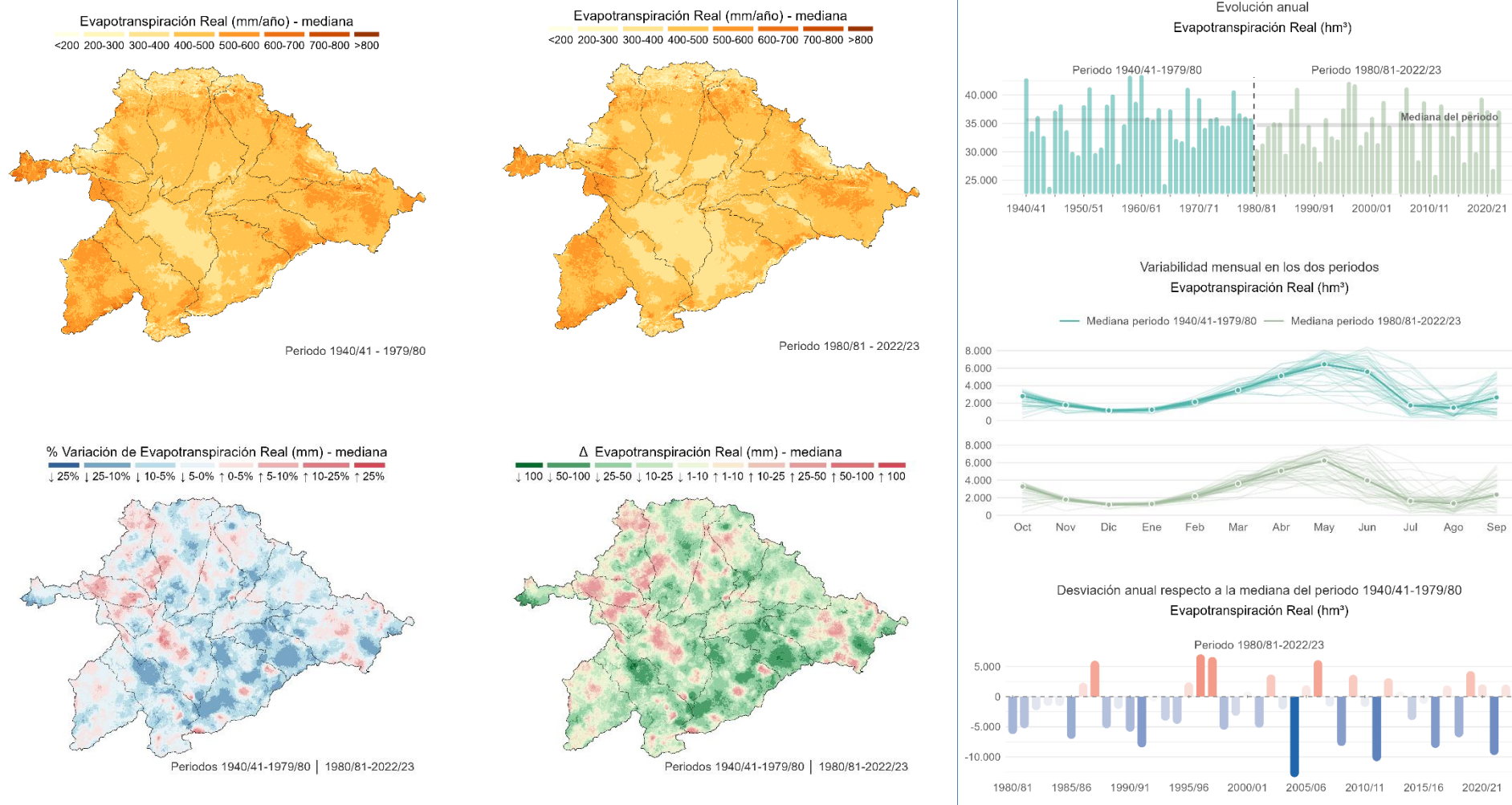
Figura 29. Caracterización espacial y temporal de la evapotranspiración real. Comparación entre los periodos 1940/41–1979/80 y 1980/81–2022/23. Fuente: Elaboración propia a partir de información de SIMPA (CEDEX).
