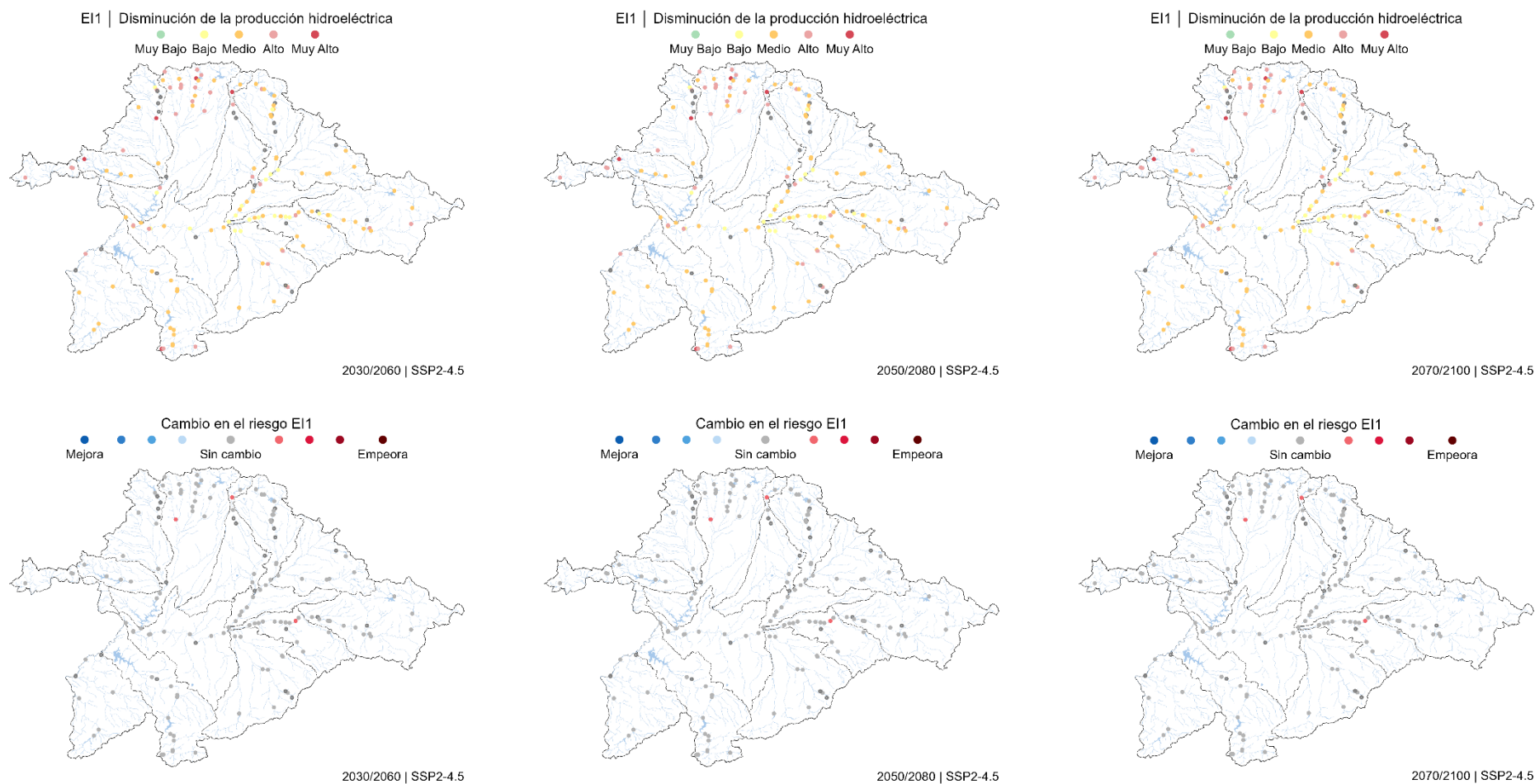
Figura 133. Evaluación del riesgo EI1 proyectado bajo el escenario intermedio (SSP2-4.5), para los horizontes temporales 2030/2060, 2050/2080 y 2070/2100 respecto a la situación de riesgo actual.
