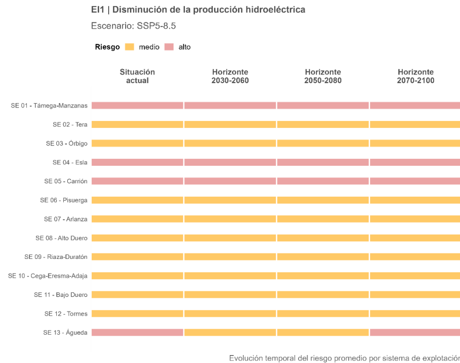
Figura 136. Trayectoria temporal del riesgo EI1 promedio por sistema de explotación, proyectado bajo el escenario de altas emisiones (SSP5-8.5).
