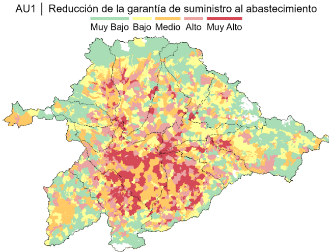
Figura 120. Riesgo AU1: Mapa de situación actual (periodo 1980/81 – 2022/23)
