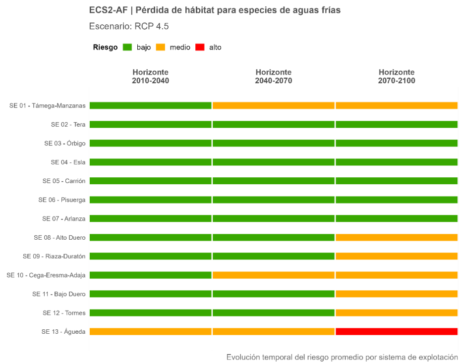
Figura 97. Trayectoria temporal del riesgo ECS2-AF promedio por sistema de explotación, proyectado bajo el escenario intermedio (RCP 4.5).
