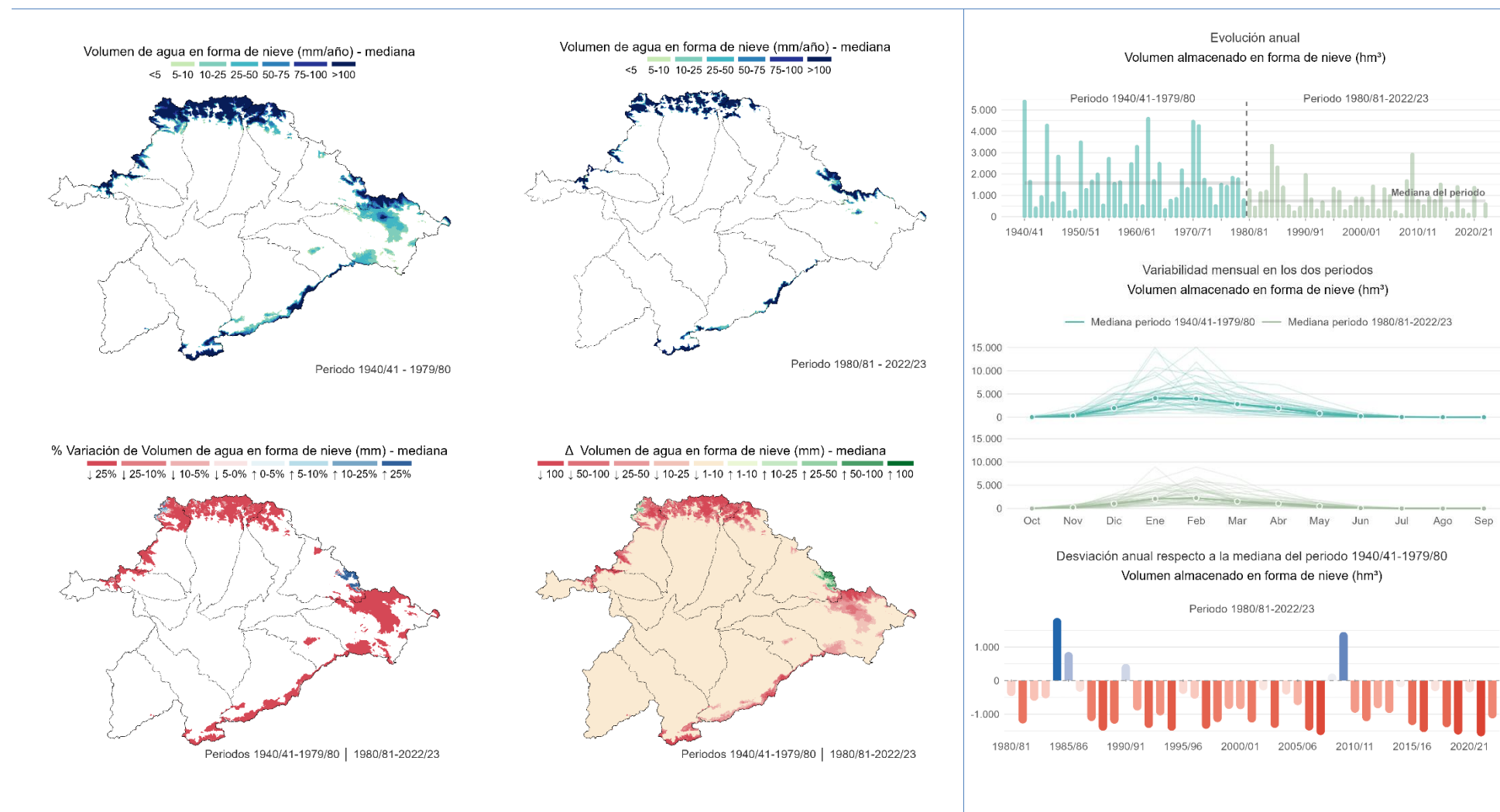
Figura 25. Caracterización espacial y temporal del régimen nival. Comparación entre los periodos 1940/41–1979/80 y 1980/81–2022/23. Fuente: Elaboración propia a partir de información de SIMPA (CEDEX).
