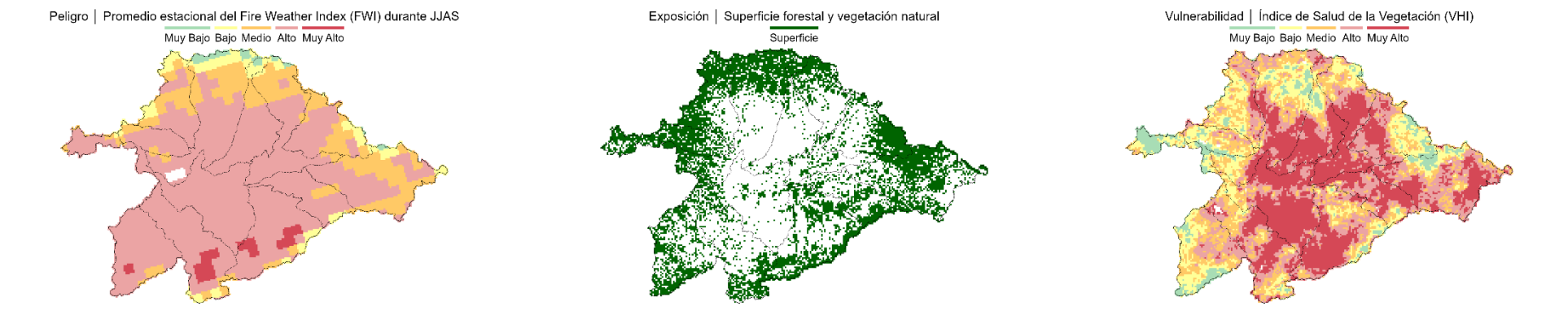
Figura 113. Riesgo ECS13. Mapas de los indicadores de peligro, exposición y vulnerabilidad
