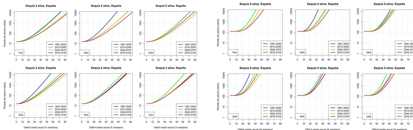
Figura 65. Periodo de retorno de sequías en España para diferentes déficits medios anuales y duración 2 años (izquierda) y 5 años (derecha) para el periodo de control (1961-2000) y tres periodos futuros (2010-2040, 2040-2070 y 2070-2100) con el escenario climático intermedio (RCP 4.5)
