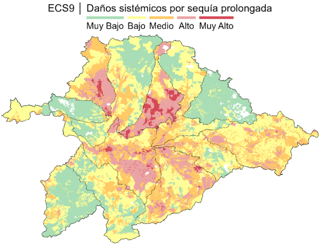
Figura 106. Riesgo ECS9: Mapa de situación actual (periodo 1980/81 – 2022/23)
