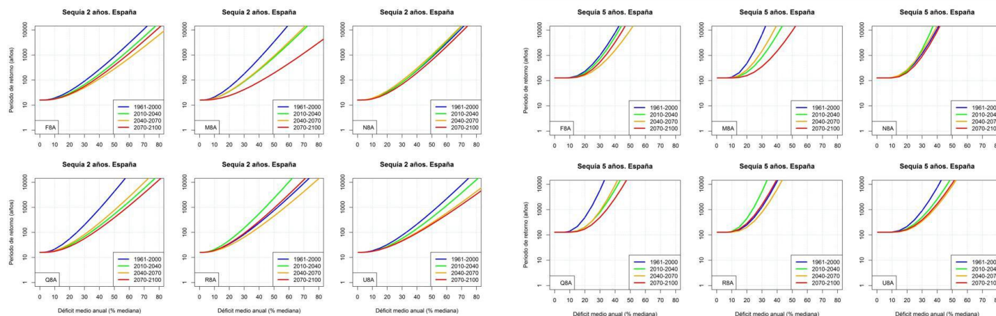
Figura 66. Periodo de retorno de sequías en España para diferentes déficits medios anuales y duración 2 años (izquierda) y 5 años (derecha) para el periodo de control (1961-2000) y tres periodos futuros (2010-2040, 2040-2070 y 2070-2100) con el escenario climático de altas emisiones (RCP 8.5)
