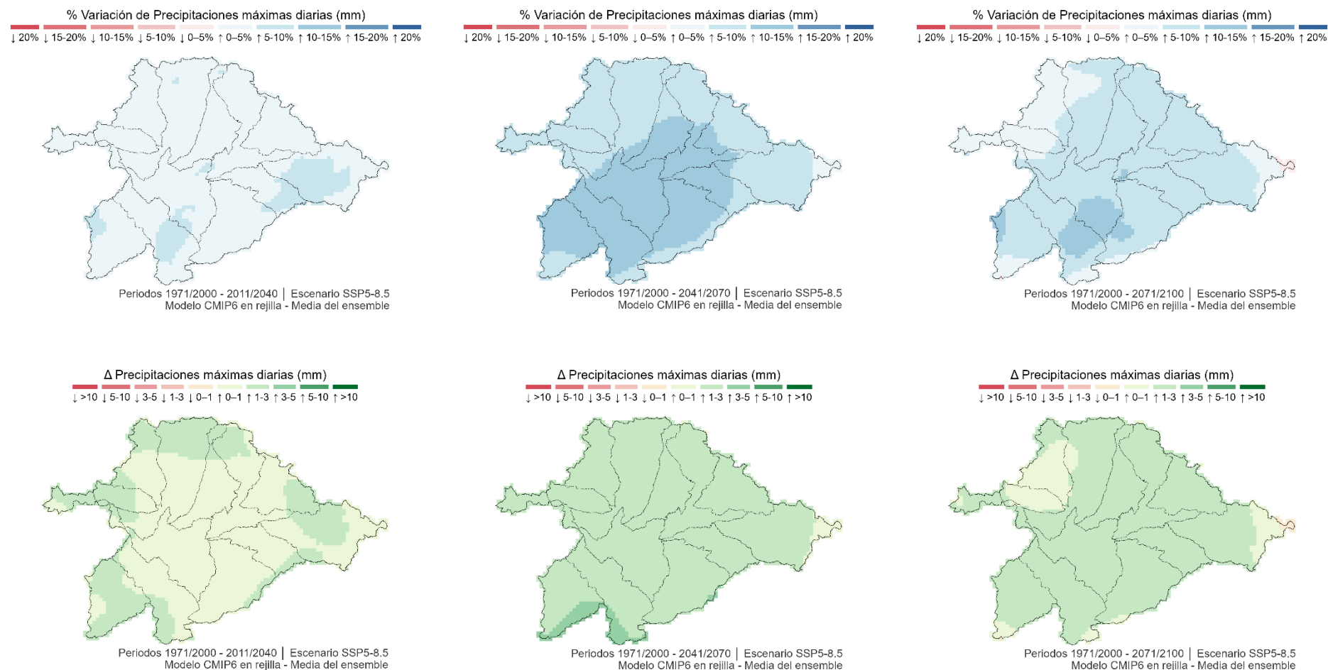
Figura 64. Variación de las precipitaciones máximas diarias proyectadas bajo el escenario de altas emisiones (SSP5-8.5), para los horizontes temporales 2011-2040, 2041-2070 y 2071-2100, en comparación con el periodo de control 1971-2000. Fuente: Elaboración propia a partir de información de Adaptecca.
