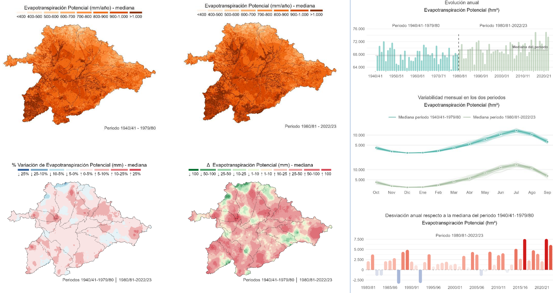
Figura 23. Caracterización espacial y temporal de la evapotranspiración potencial. Comparación entre los periodos 1940/41–1979/80 y 1980/81–2022/23. Fuente: Elaboración propia a partir de información de SIMPA (CEDEX). La mediana del periodo 1980/81–2022/23 (69.350,78 hm 3 ) supera a la del periodo 1940/41–1979/80 (67.619,12 hm 3 ) en 1731,66 hm 3 , lo que supone un incremento del 2,56%. La mayor desviación se produce en el año hidrológico 2021/22, siendo esta de +7.169,20 hm 3 .
