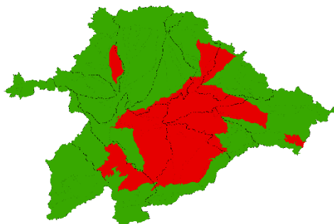
Figura 13. Estado químico de las masas de agua subterránea
