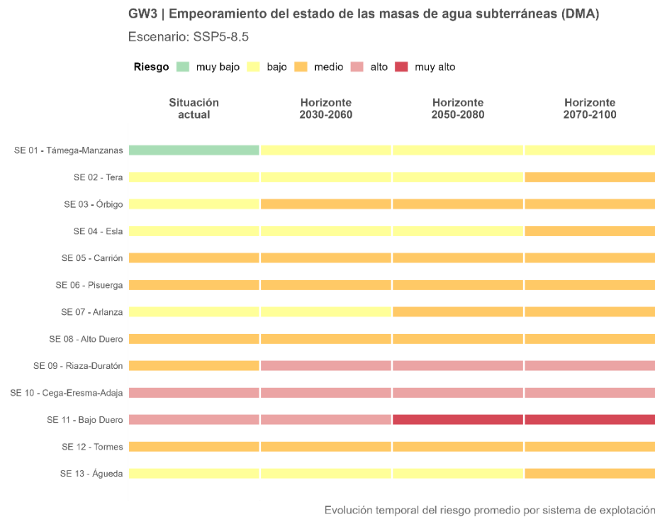
Figura 92. Trayectoria temporal del riesgo GW3 promedio por sistema de explotación, proyectado bajo el escenario de altas emisiones (SSP5-8.5).
