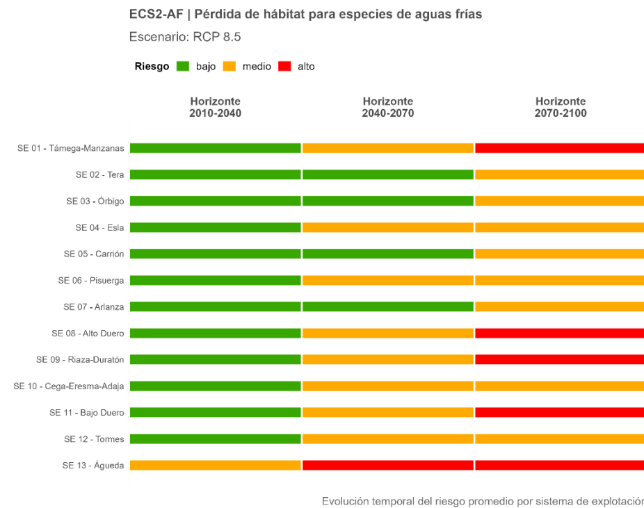
Figura 98. Trayectoria temporal del riesgo ECS2-AF promedio por sistema de explotación, proyectado bajo el escenario de altas emisiones (RCP 8.5).
