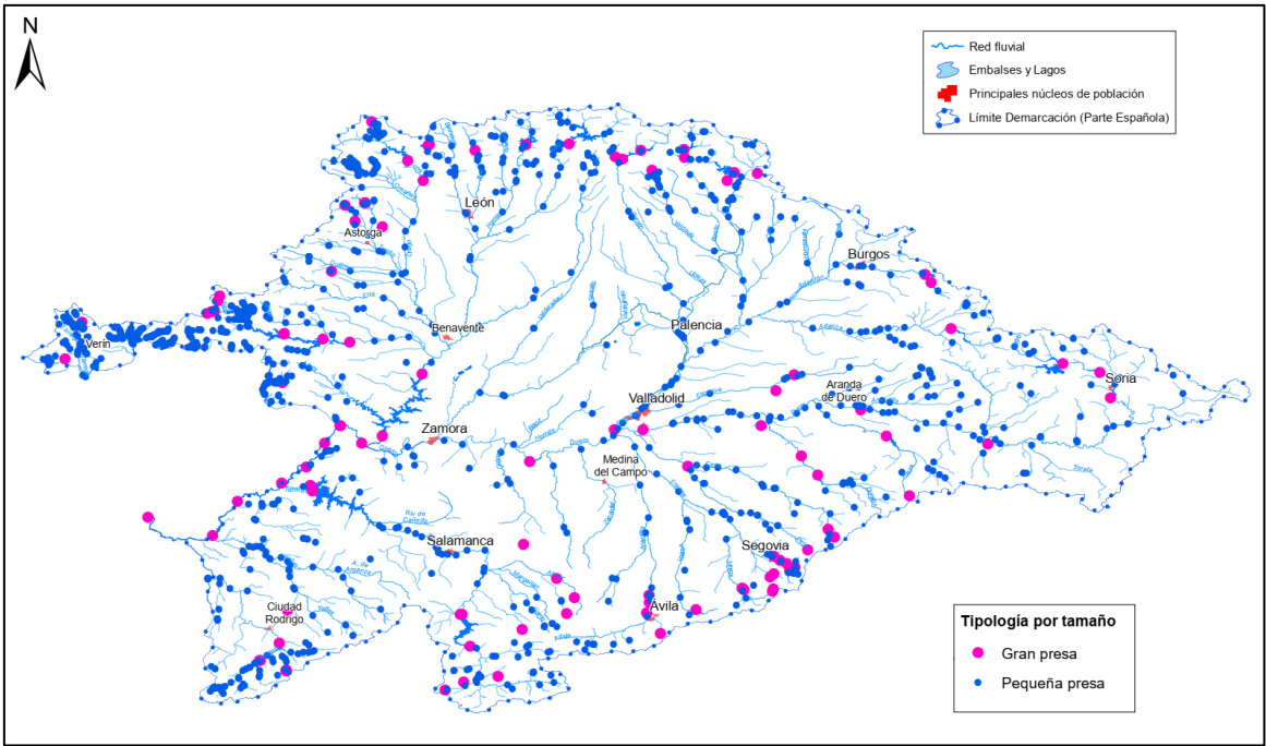
Figura 19. Distribución geográfica de presiones morfológicas por presas y azudes
