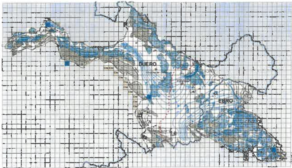
Figura 7.1. Superficie piezométrica flujo subterráneo y manantiales de la MASCH Araviana-Borobla (acuífero jurásico) en régimen natural permanente.
