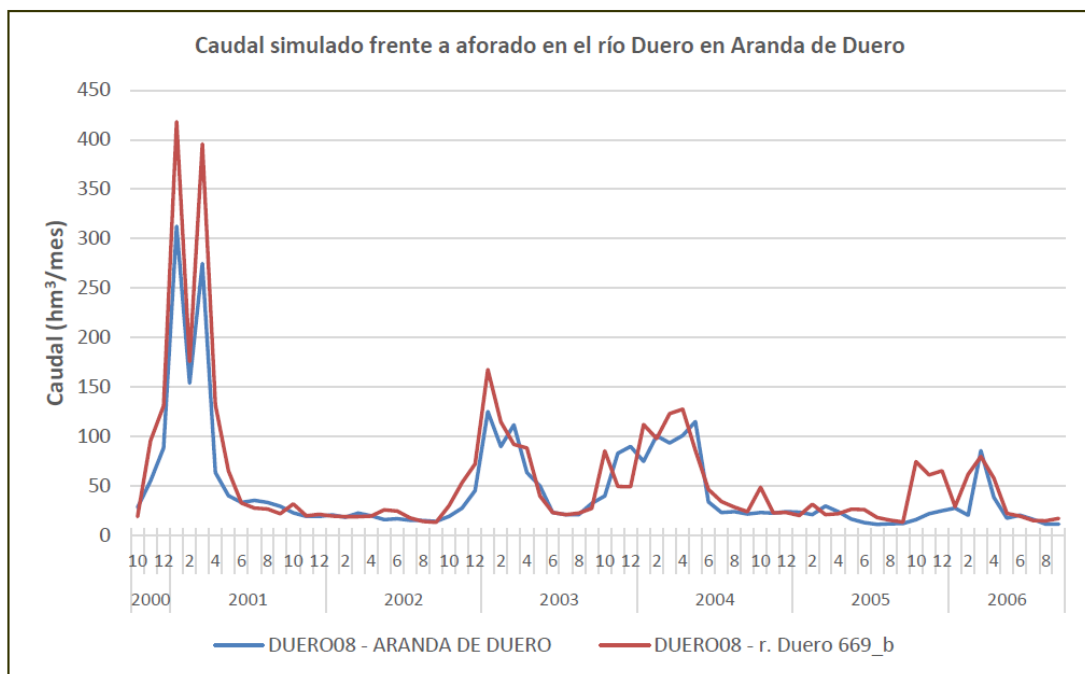
Figura 4.1.5 Comparación entre los caudales medios del río Duero aforados (en azul) y los simulados en la estación de Aranda de Duero (en rojo).
