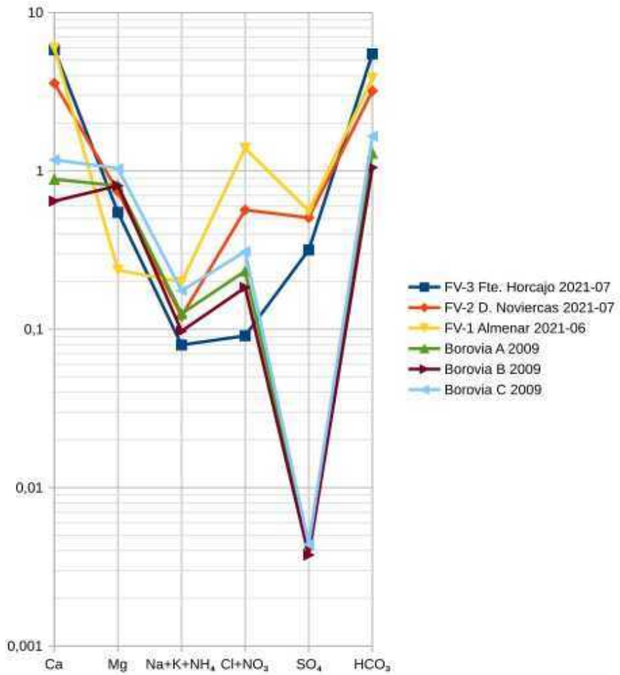
Figura 5.7.3 Diagrama de columnas verticales logarítmicas (Schoeller-Barkaloff) de las muestras de agua adicionales y del río Manubles (Borobia).
