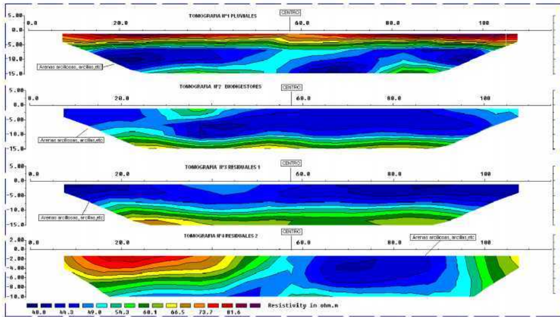
Figura 6.2 Tomografía eléctrica de los 15 primeros metros en la zona de las balsas. (Geoterra, 2020 b). Las áreas de baja resistividad eléctrica (colores azules) se interpretan como presencia dominante de arcillas y arcillas arenosas.
