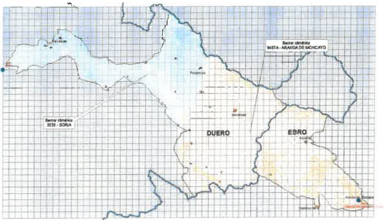
Figura 5.7. Sectores climáticos por polígonos de Thiessen ajustados al mallaado aplicado en el código RENATA
