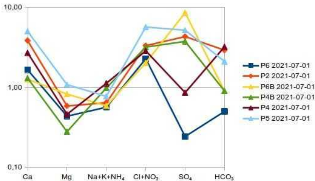
Figura 5.7.2 Diagrama de columnas verticales logarítmicas (Schoeller-Barkaloff) de las muestras de agua de la limpieza de los piezómetros de la ubicación de las balsas de la futura Vaquería de Noviercas.
