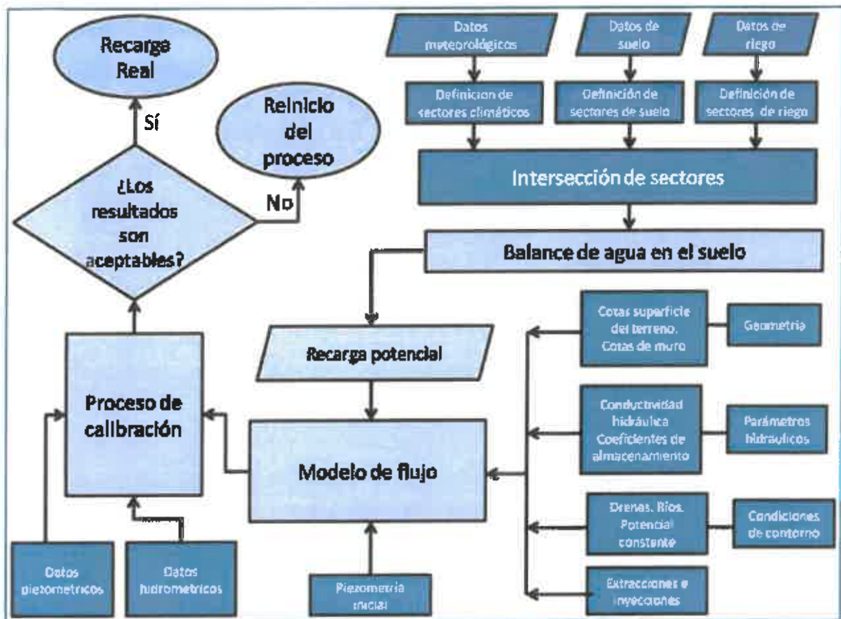
Figure 5.8. Diagrama de flujo del código RENATA detallando los datos que se tienen que aportar al programa.
