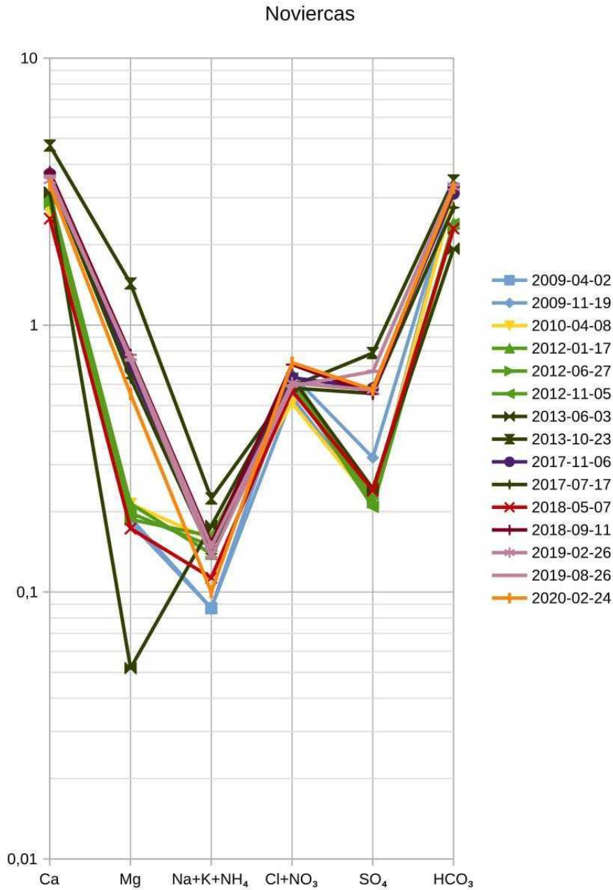
Figura 5.7.7 Representación de los análisis iónicos mayoritarios del pozo de Noviercas a partir de los datos de la red de calidad del agua de la CHD.
