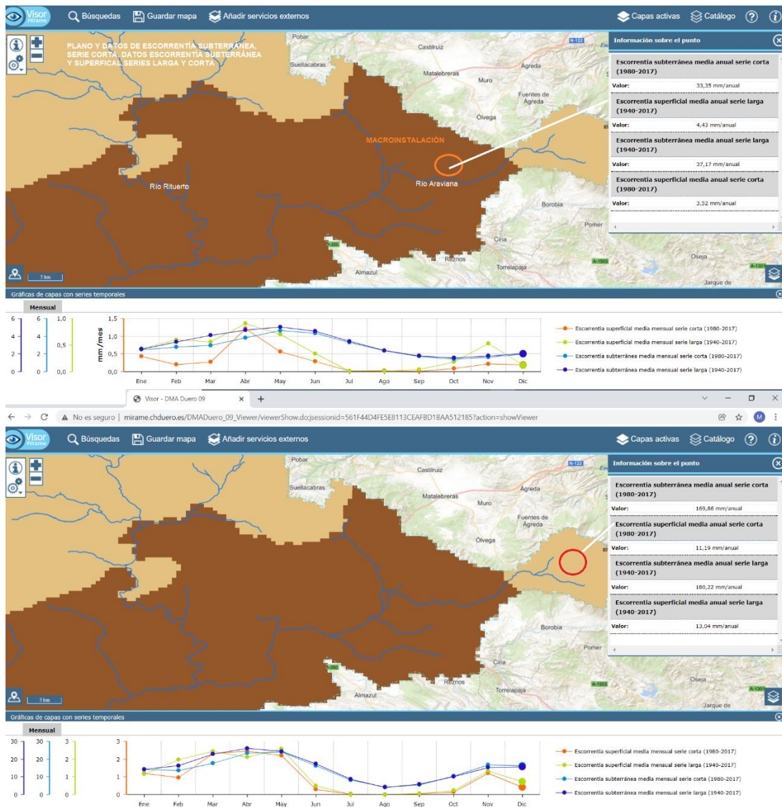
Figura 1: Planos de precipitación media subterránea de la serie corta. Los gráficos y los datos incluyen tanto escorrentía superficial como subterránea, series larga y corta. Se incluyen dos zonas, Río Araviana a la altura de Noviercas (1a) y Cabecera del Río Araviana, (1b).
