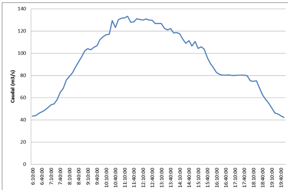
Figura 2. Hidrograma real (EA 2102. Embalse de Riaño)
