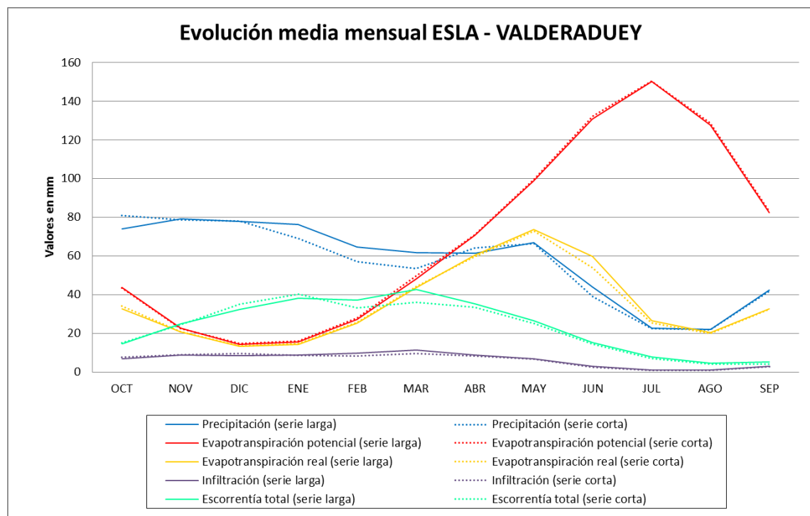
Figura 68. Evolución media mensual de las principales variables hidrológicas, subzona Esla-Valderaduey
