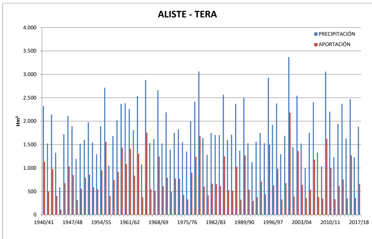
Figura 52. Serie de precipitaciones y aportaciones anuales en la subzona Aliste-Tera
