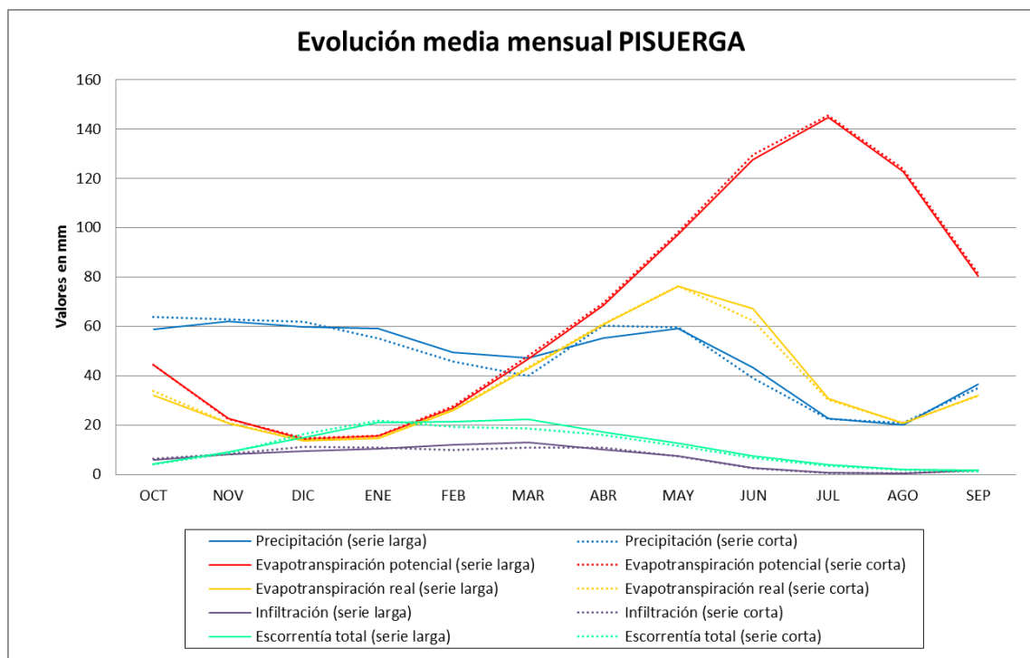
Figura 70. Evolución media mensual de las principales variables hidrológicas, subzona Pisuergra
