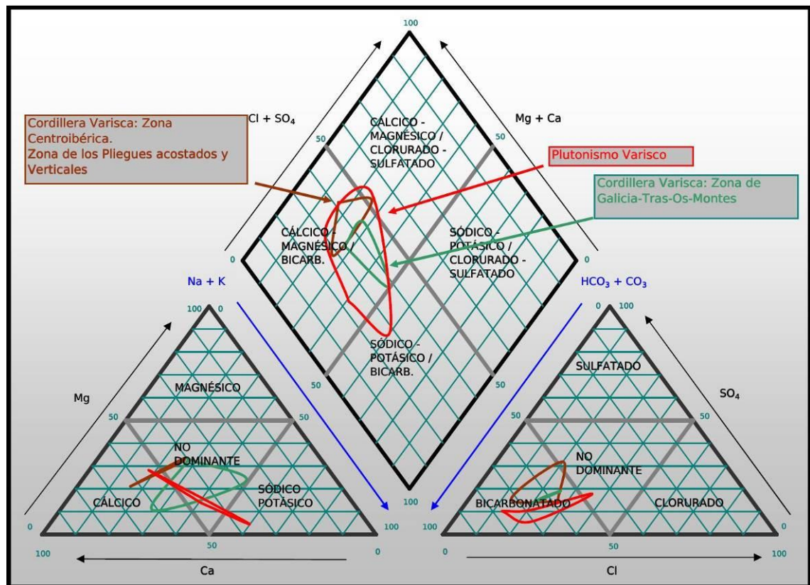
Figura 92. Diagrama de Piper para los contextos geológicos metamórficos e ígneos de la cuenca
