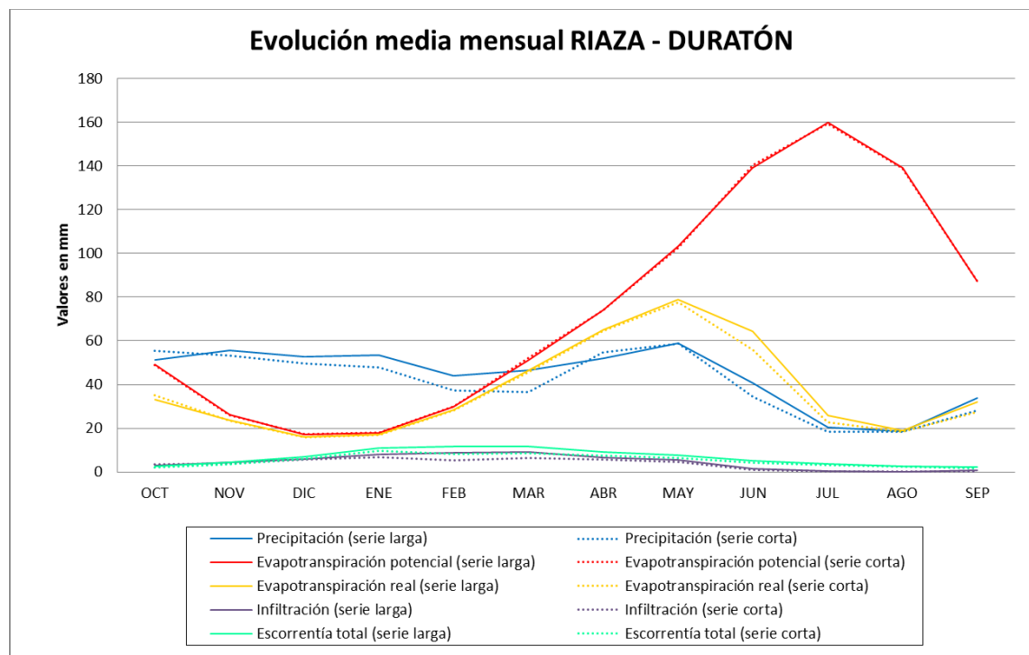
Figura 73. Evolución media mensual de las principales variables hidrológicas, subzona Riaza-Duración
