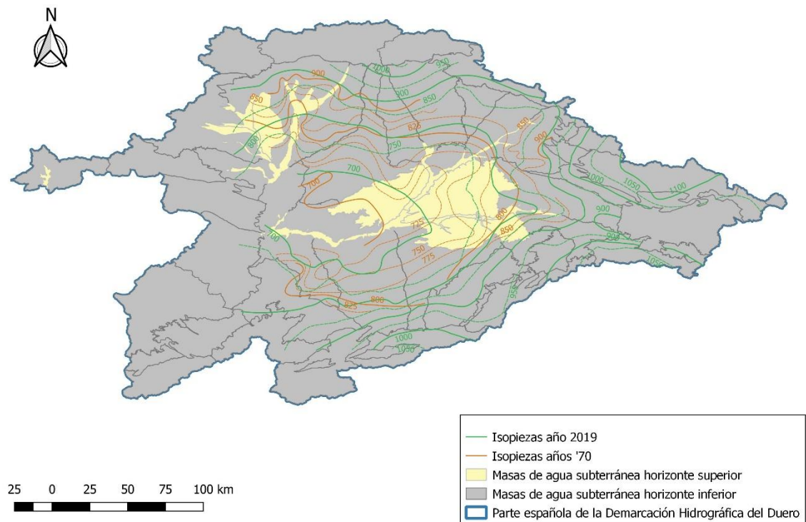
Figura 15. Piezometría de referencia e isopiezías del año 2019
