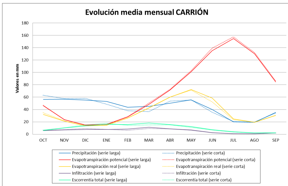
Figura 69. Evolución media mensual de las principales variables hidrológicas, subzona Carrión
