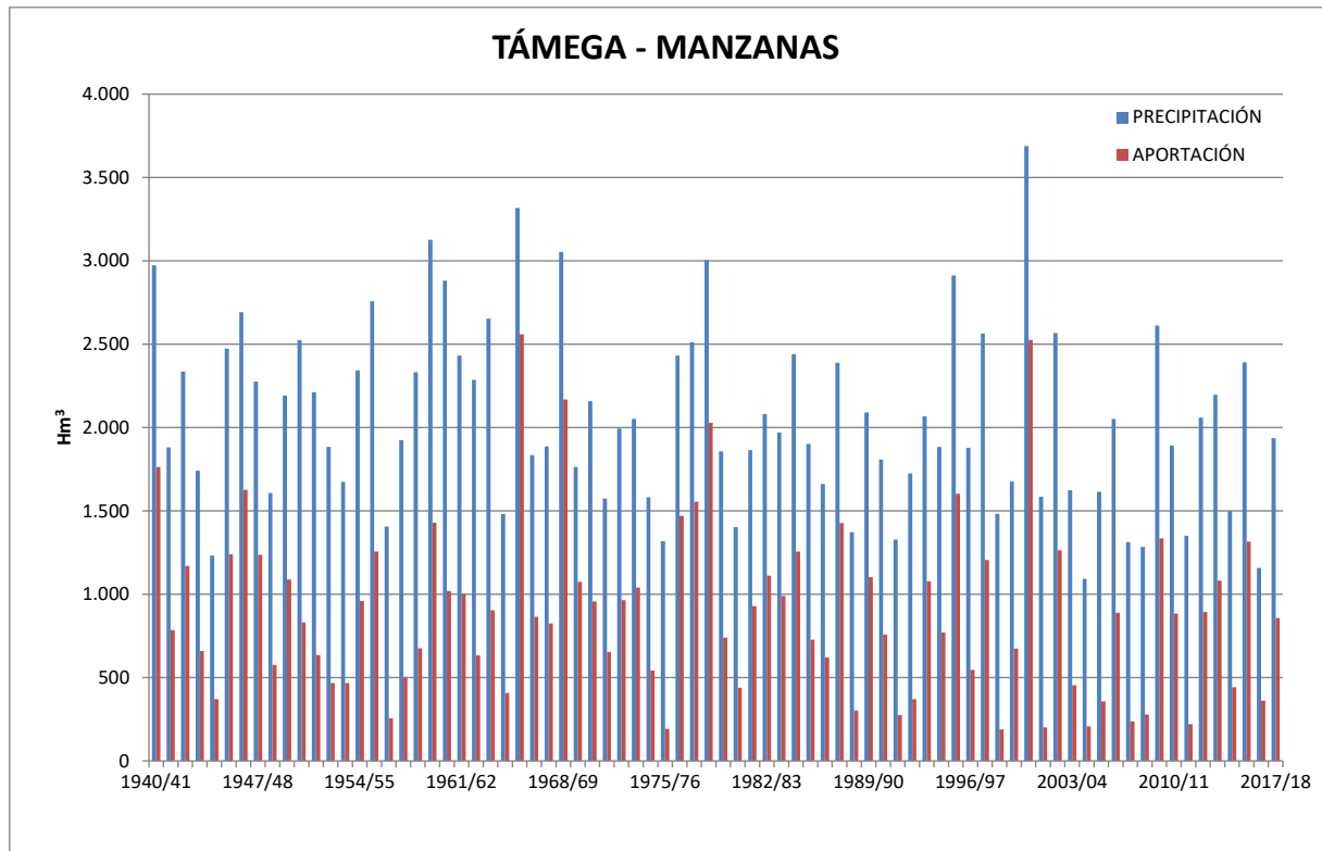
Figura 51. Serie de precipitaciones y aportaciones anuales en la subzona Támege-Manzanas
