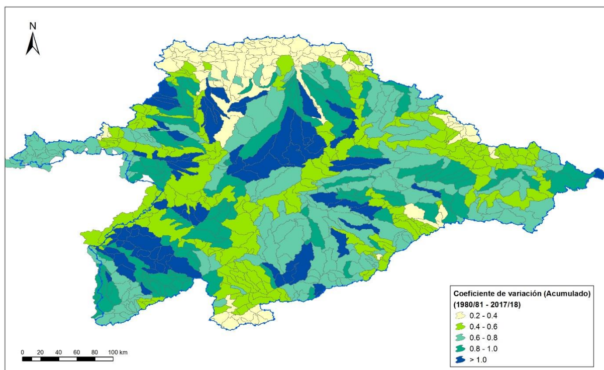
Figura 46. Distribución espacial del coeficiente de variación (Serie 1980/81 a 2017/18)
