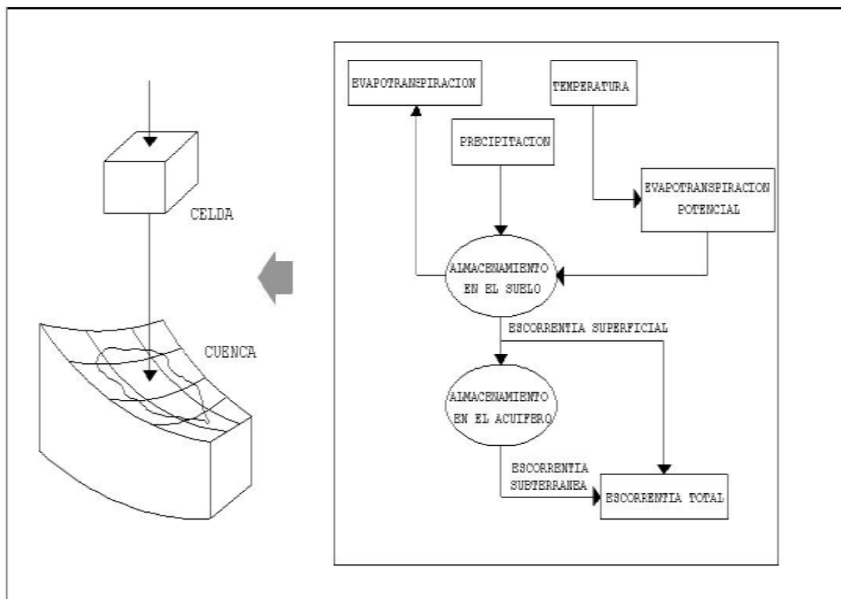
Figura 9. Esquema de funcionamiento de SIMPA
