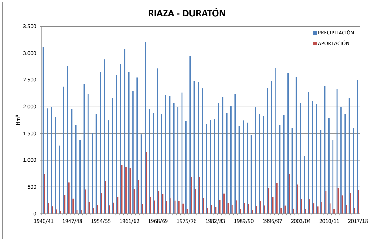
Figura 59. Serie de precipitaciones y aportaciones anuales en la subzona Riza-Duraton
