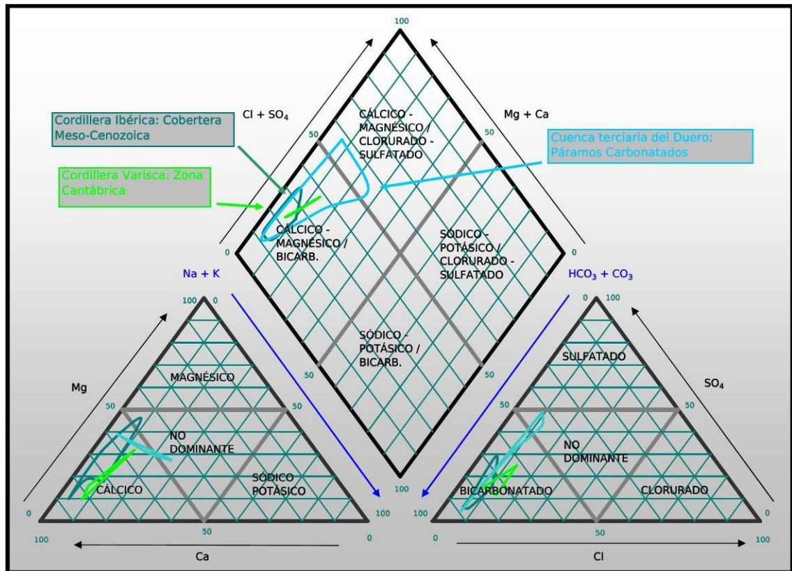
Figura 94. Diagrama de Piper para los contextos geológicos carbonatados de la cuenca
