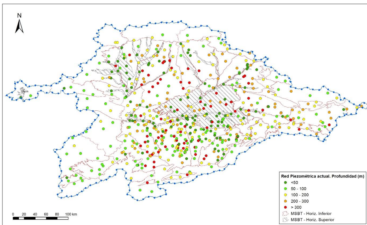
Figura 14. Red piezométrica de la cuenca del Duero
