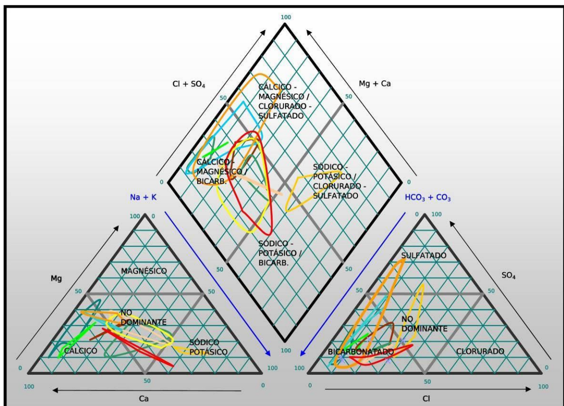
Figura 95. Características químicas de las aguas naturales de la cuenca española del Duero
