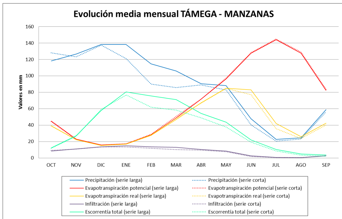
Figura 65. Evolución media mensual de las principales variables hidrológicas, subzona Táme-ga-Manzanas
