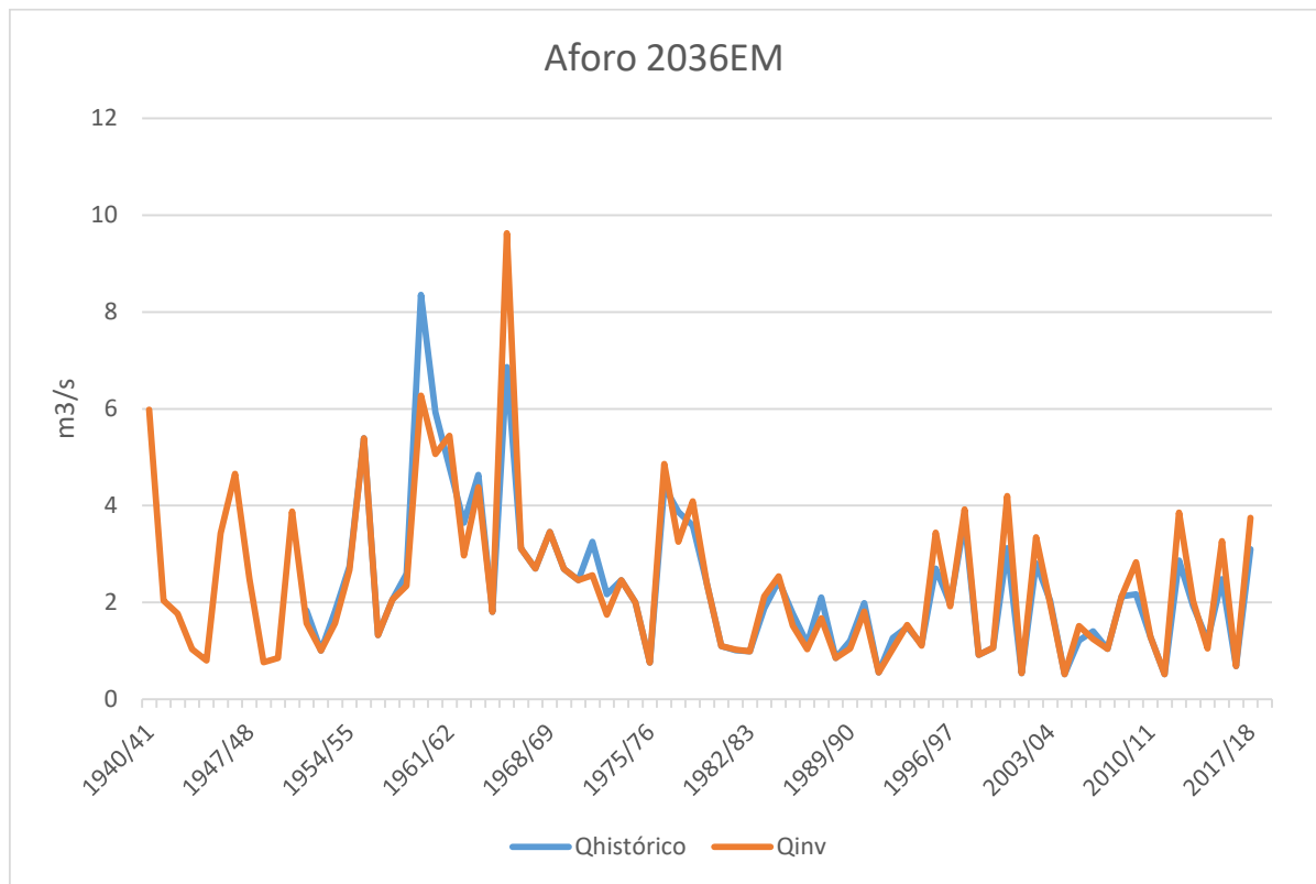
Figura 88. Valores de aportación (caudales medios anuales) del Riaza en E. Linares del Arroyo
