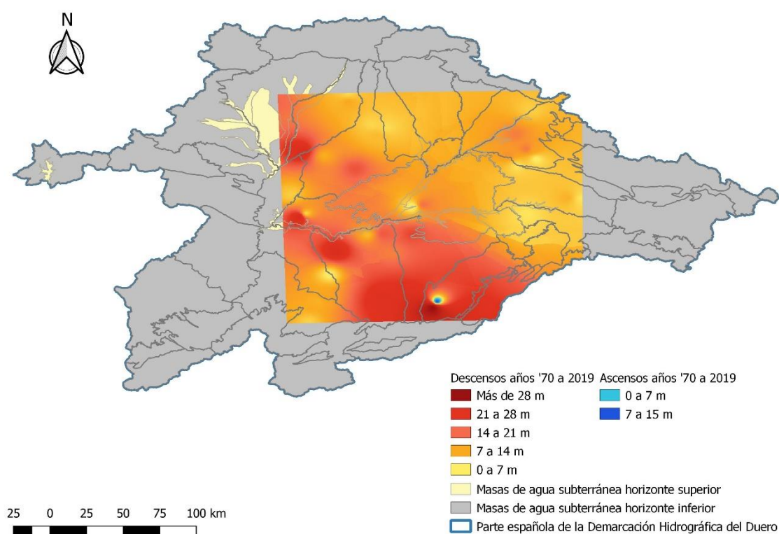
Figura 16. Mapa de isodescensos
