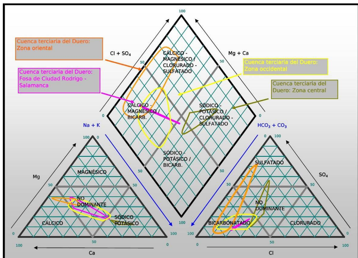
Figura 93. Diagrama de Piper para los contextos geológicos detríticos de la cuenca
