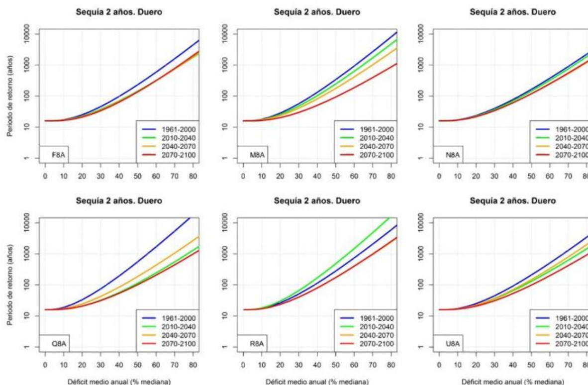
Figura 106. Variación en el periodo de retorno de las sequías de dos años según las proyecciones del escenario RCP8.5 (CEDEX, 2017)
