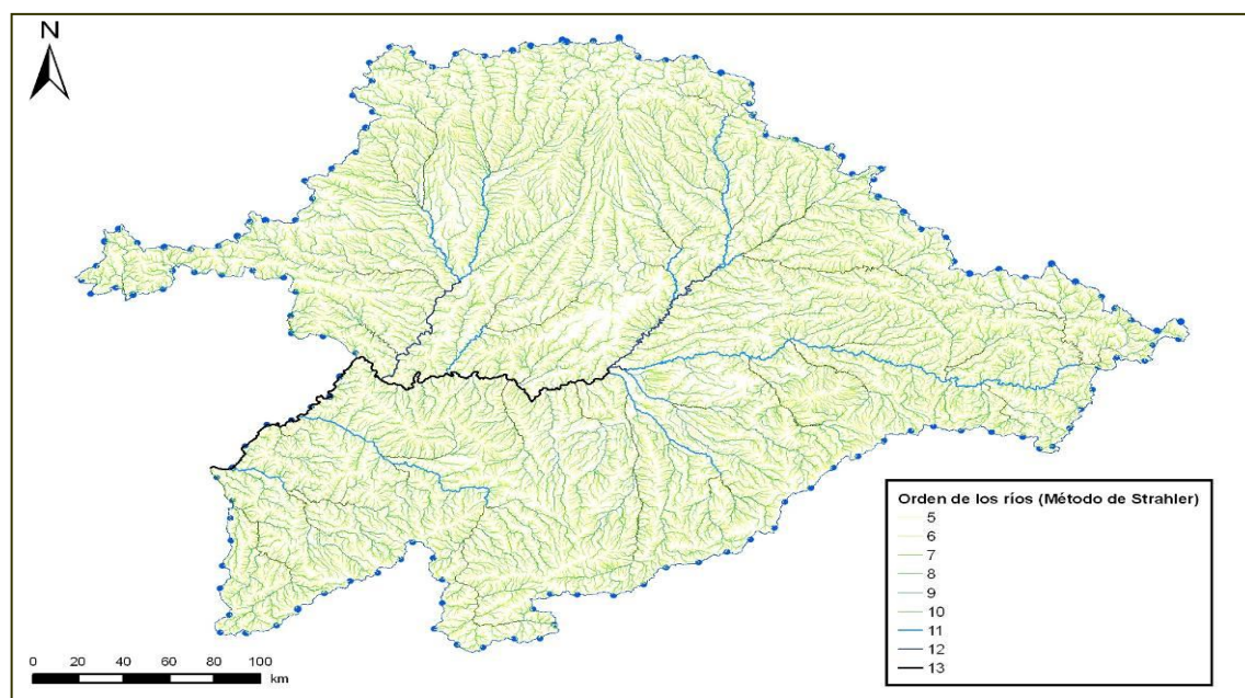
Figura 5. Órdenes Strahler
