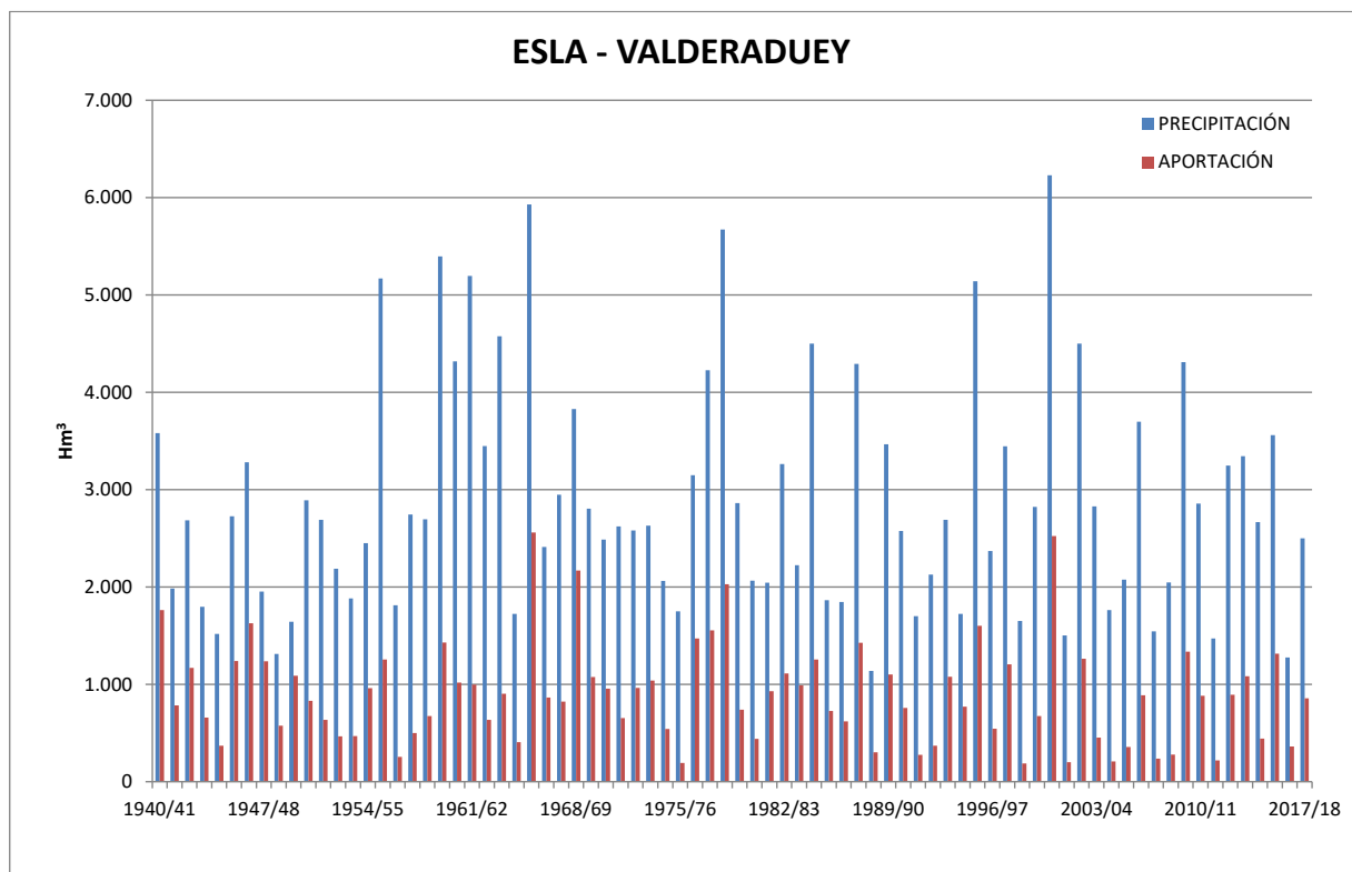
Figura 54. Serie de precipitaciones y aportaciones anuales en la subzona Esla-Valderaduey
