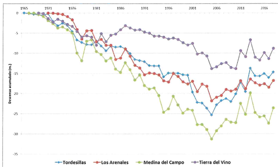
Imagen 1. Gráfico de variación de niveles piezométricos en las masas con mayores descensos acumulado. Fuente: CHD
