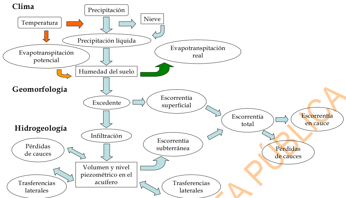
Figura 6. Esquema de flujo del modelo conceptual del ciclo hidrológico Patricial
