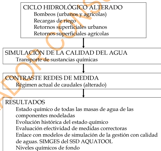
Figura 4. Metodología para la simulación de la calidad del agua, resultados y aplicaciones
