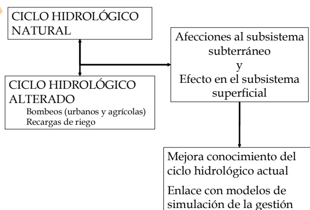
Figura 3. Régimen natural y régimen alterado en la componente subterránea y evaluación de afecciones
