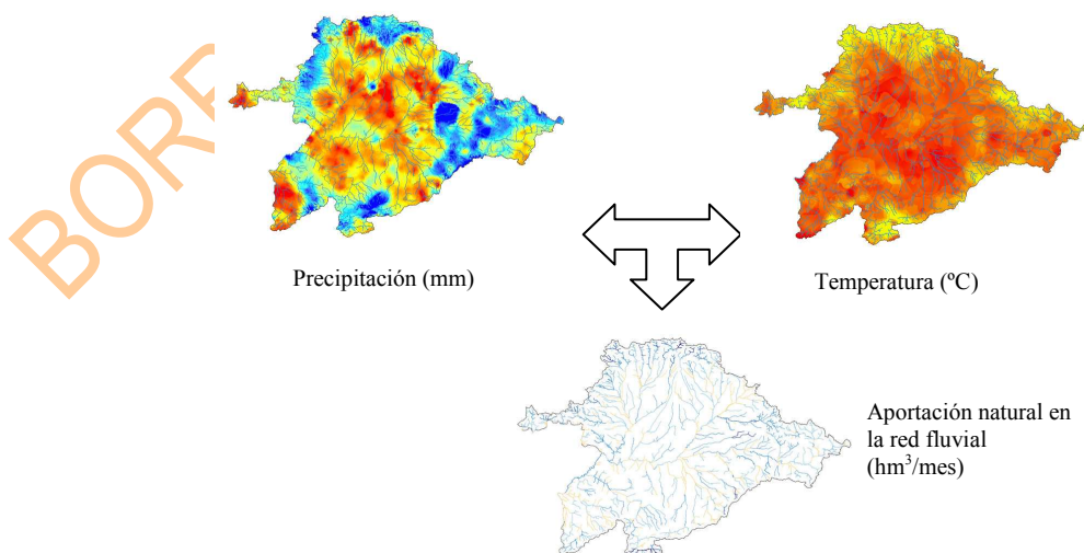
Figura 7. Precipitación temperatura y aportación en la red fluvial en mayo de 2006 en la parte española de la DHD
