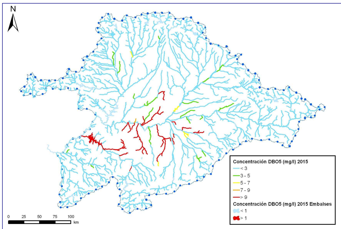
Figura 12. Concentración de DBO 5 (mg/l) en las masas de agua superficiales en el escenario 2015 con mejoras en el tratamiento de los efluentes
