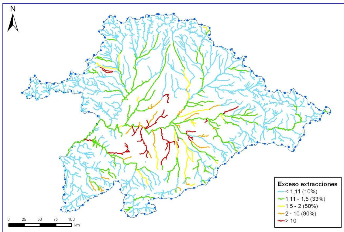
Figura 6. Extracción de caudal sobre las masas de agua superficiales
