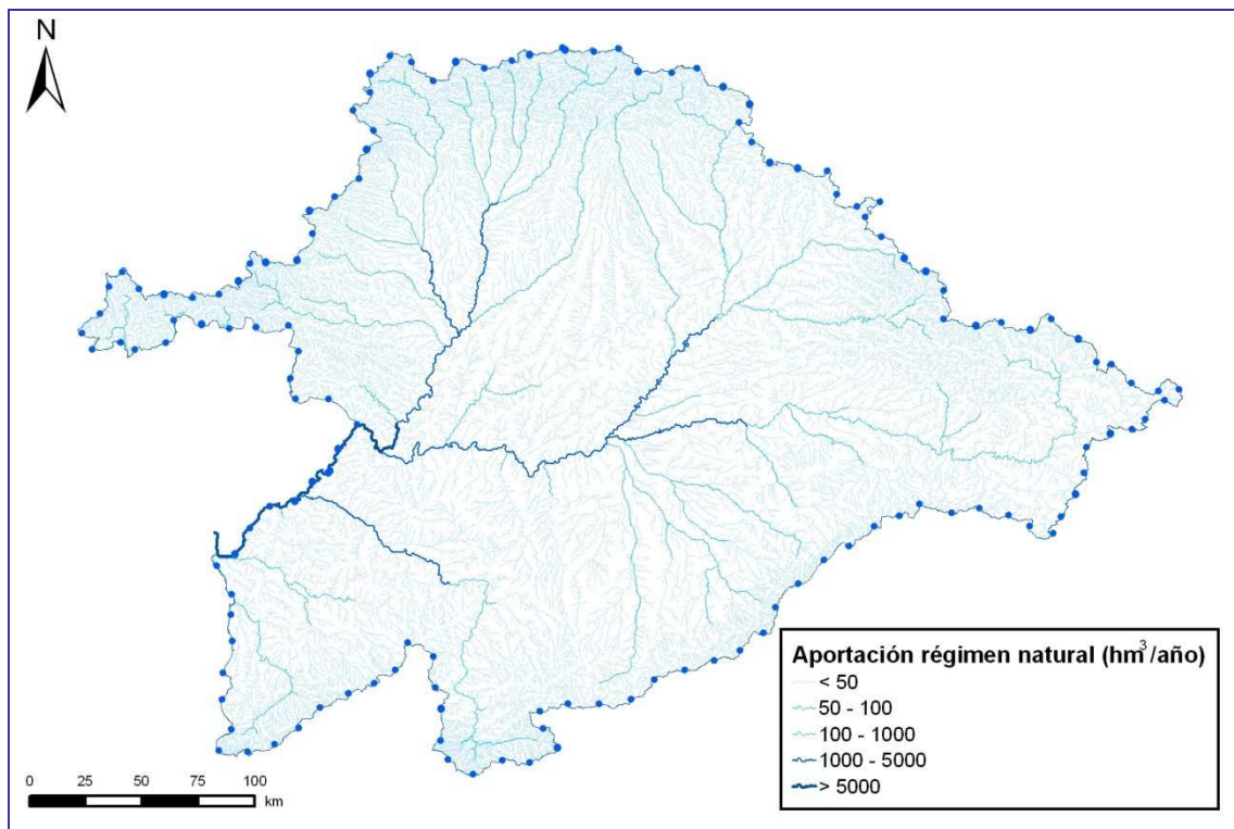
Figura 3. Aportación acumulada en régimen natural (1980/81-2005/06)
