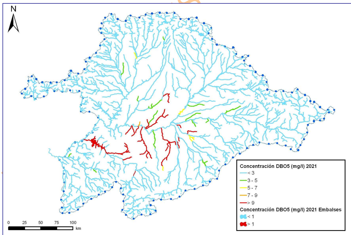
Figura 14. Concentración de materia orgánica (mg/l) en las masas de agua superficiales en el escenario 2021 con medidas adicionales
