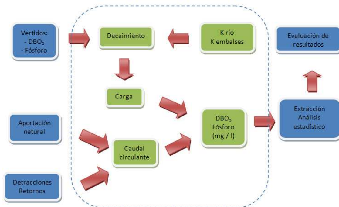
Figura 1. Esquema general de la modelación en GEOIMPRESS
