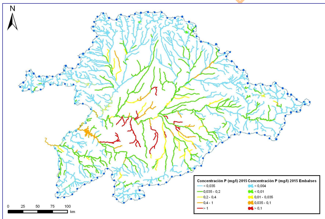
Figura 11. Concentración de fósforo (mg/l) en las masas de agua superficiales en el escenario 2015 con mejoras en el tratamiento de los efluentes
