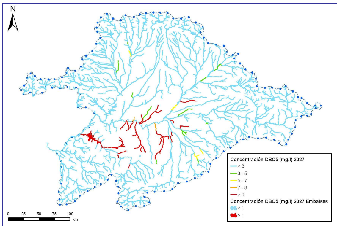
Figura 16. Concentración de materia orgánica (mg/l) en las masas de agua superficiales en el escenario 2027 con medidas adicionales
