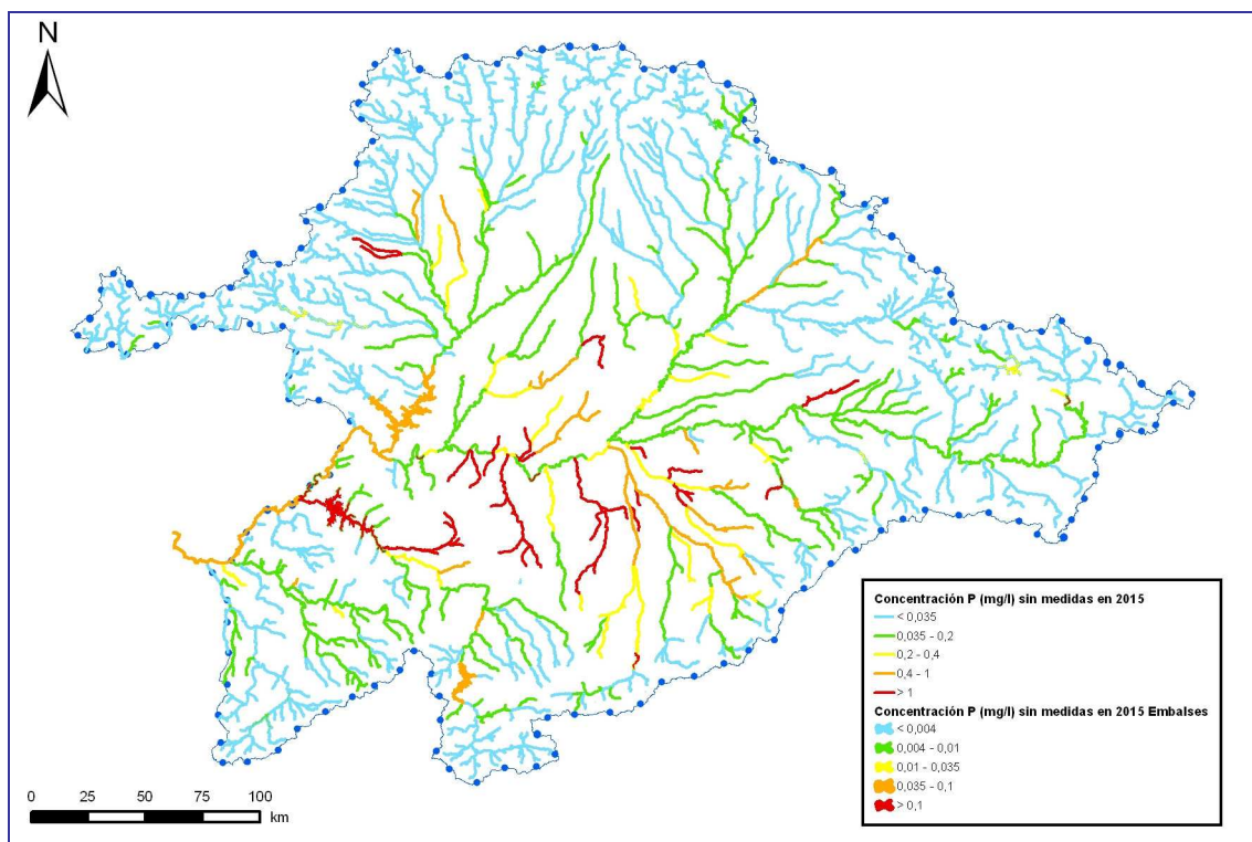
Figura 9. Concentración de fósforo (mg/l) en las masas de agua superficiales en el escenario 2015 sin mejoras en el tratamiento de los efluentes
