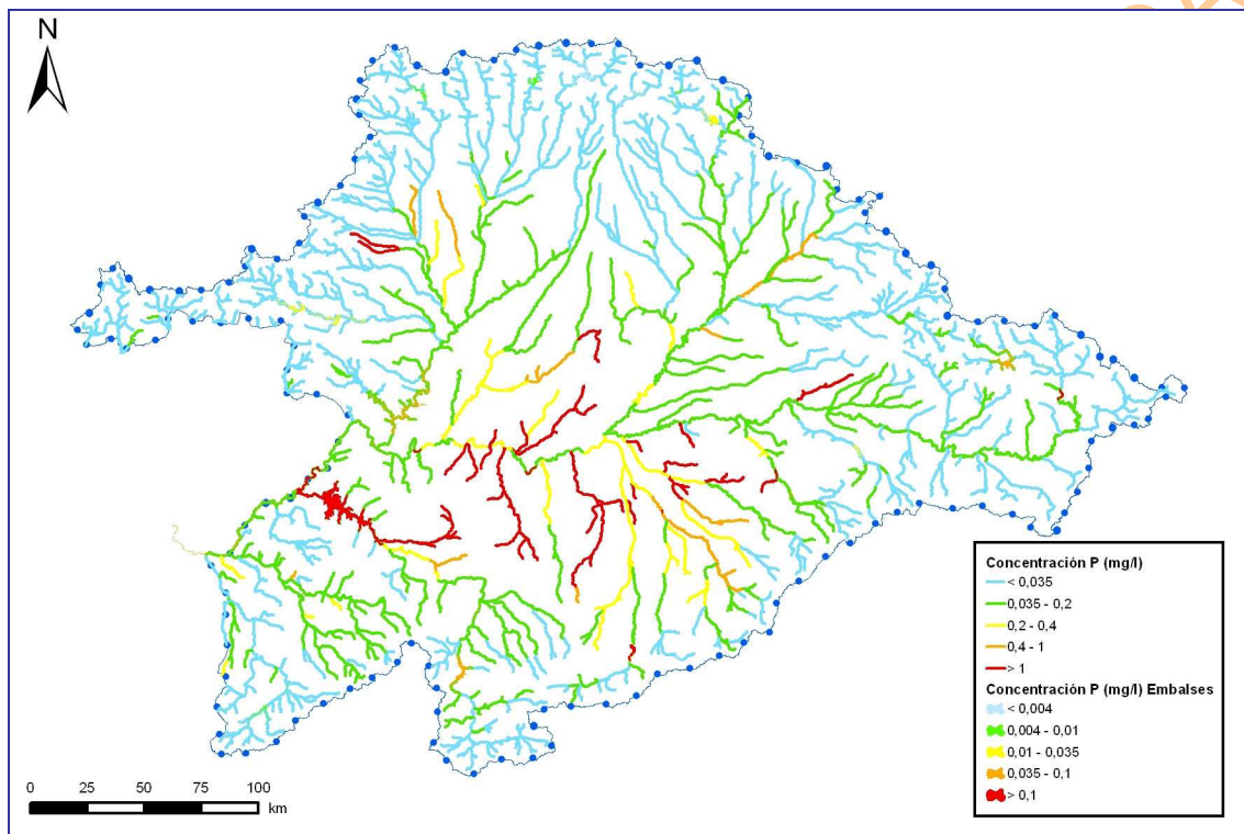
Figura 7. Concentración de fósforo (mg/l) en las masas de agua superficiales en la situación actual
