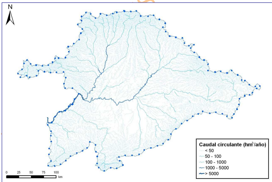
Figura 4. Aportación acumulada en régimen alterado (1980/81-2005/06)
