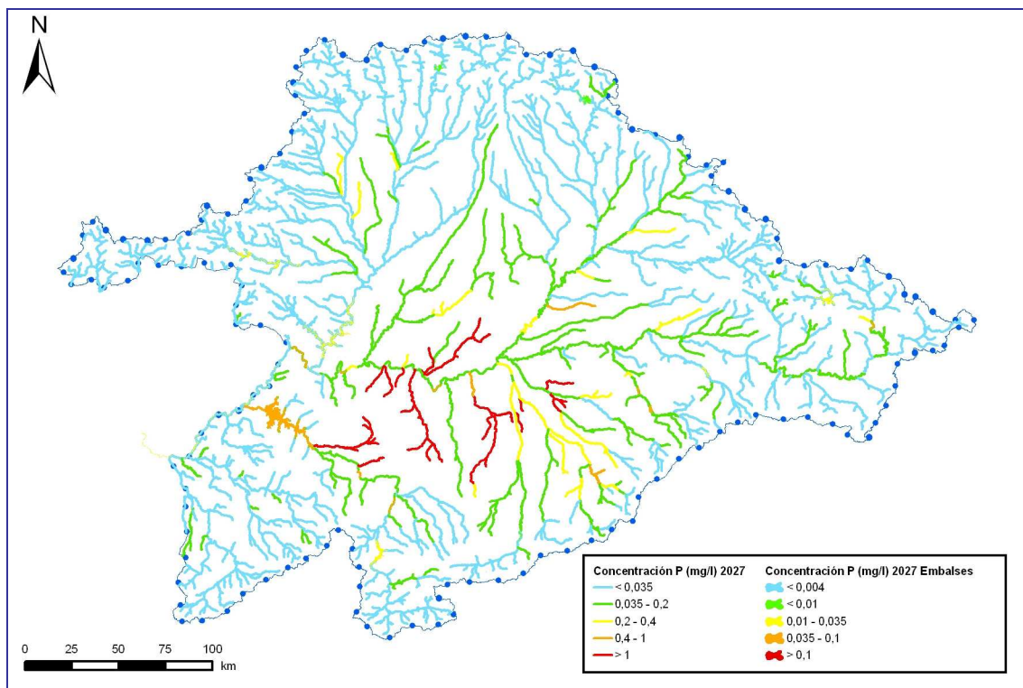
Figura 15. Concentración de fósforo (mg/l) en las masas de agua superficiales en el escenario 2027 con medidas adicionales
