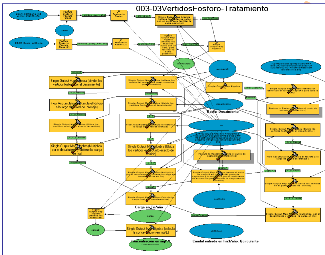
Figura 5. Script gráfico del modelo de simulación del fósforo en el escenario actual
