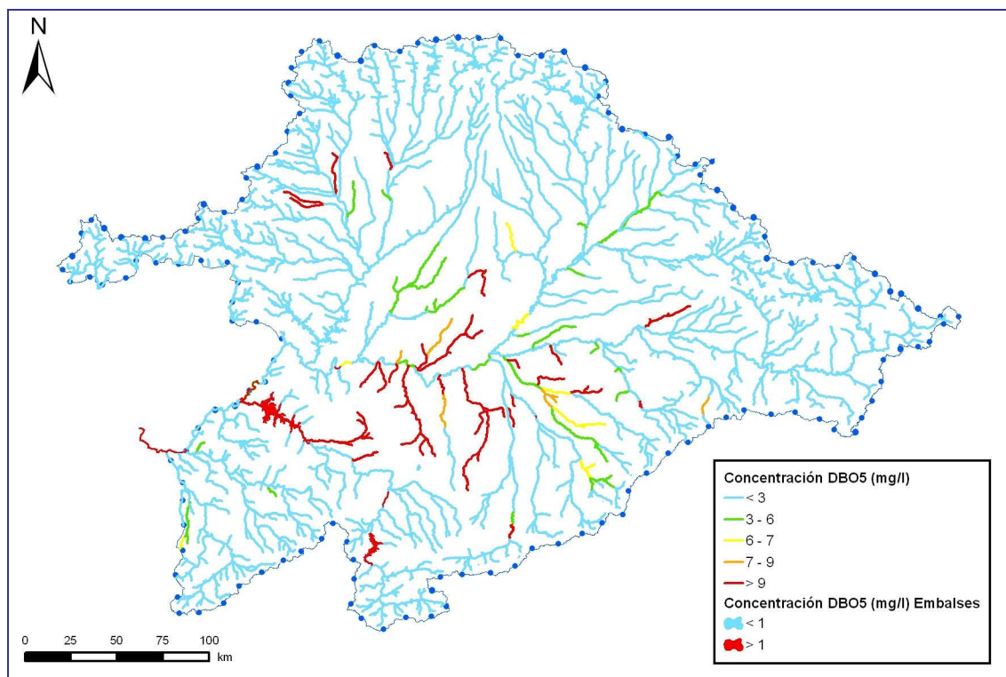
Figura 8. Concentración de materia orgánica (mg/l) en las masas de agua superficiales en la situación actual
