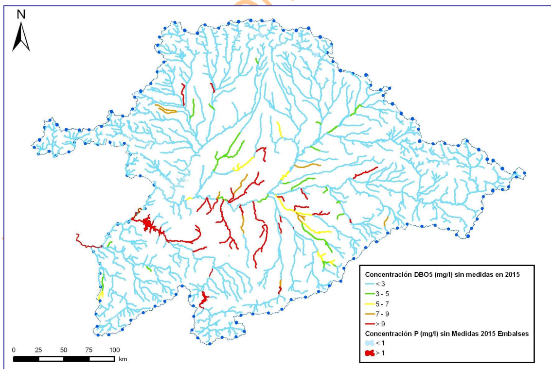
Figura 10. Concentración de DBO 5 (mg/l) en las masas de agua superficiales en el escenario 2015 sin mejoras en el tratamiento de los efluentes
