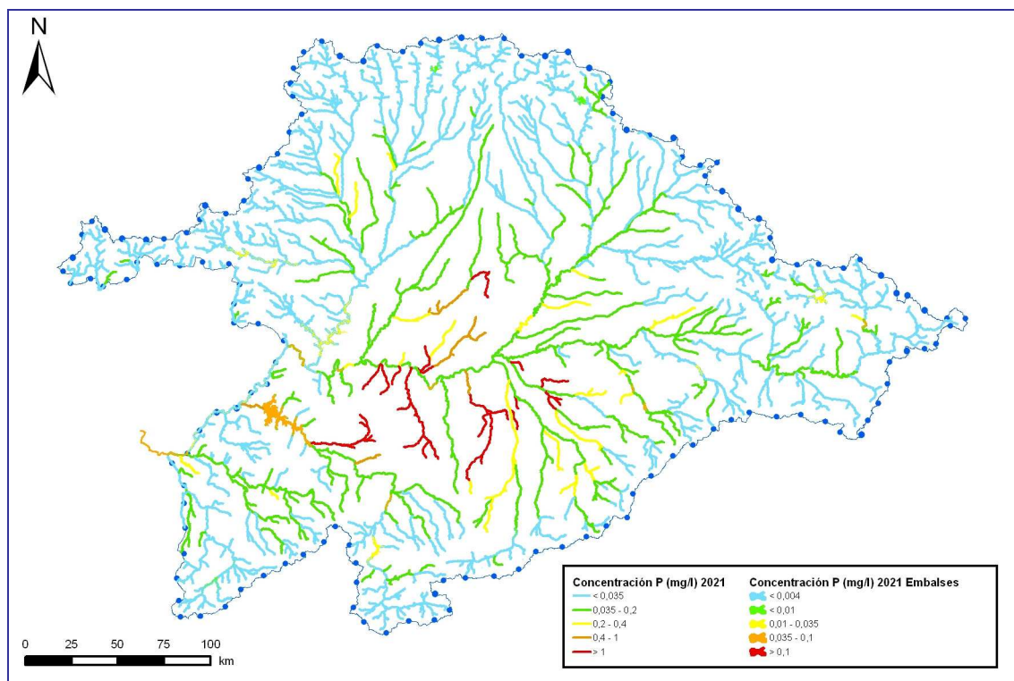
Figura 13. Concentración de fósforo (mg/l) en las masas de agua superficiales en el escenario 2021 con medidas adicionales
