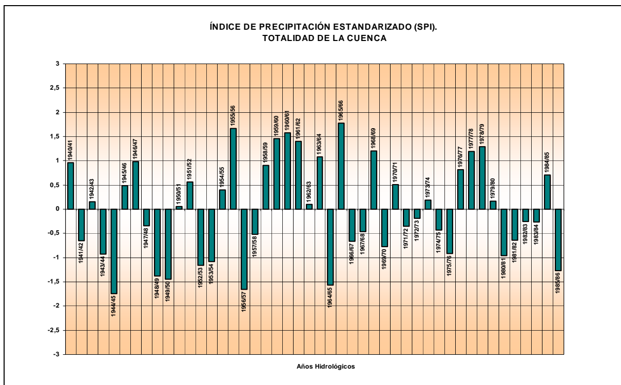
Figura 3. Evolución del Índice SPI en el ámbito de la cuenca del Duero
