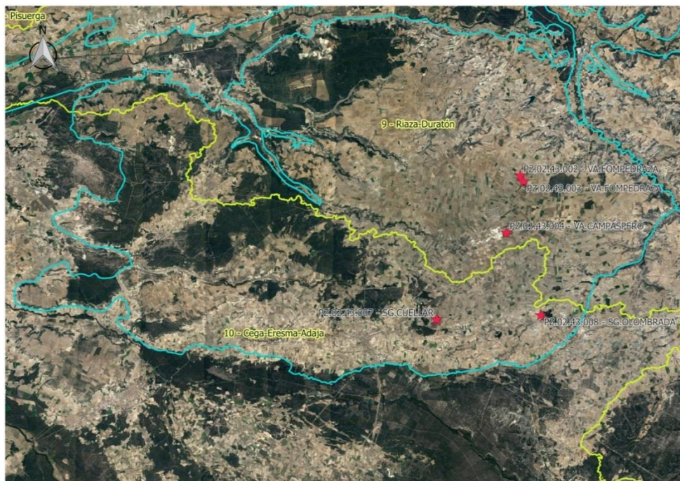
Figura 6. Distribución geográfica de los piezómetros seleccionados (masa 400043)
